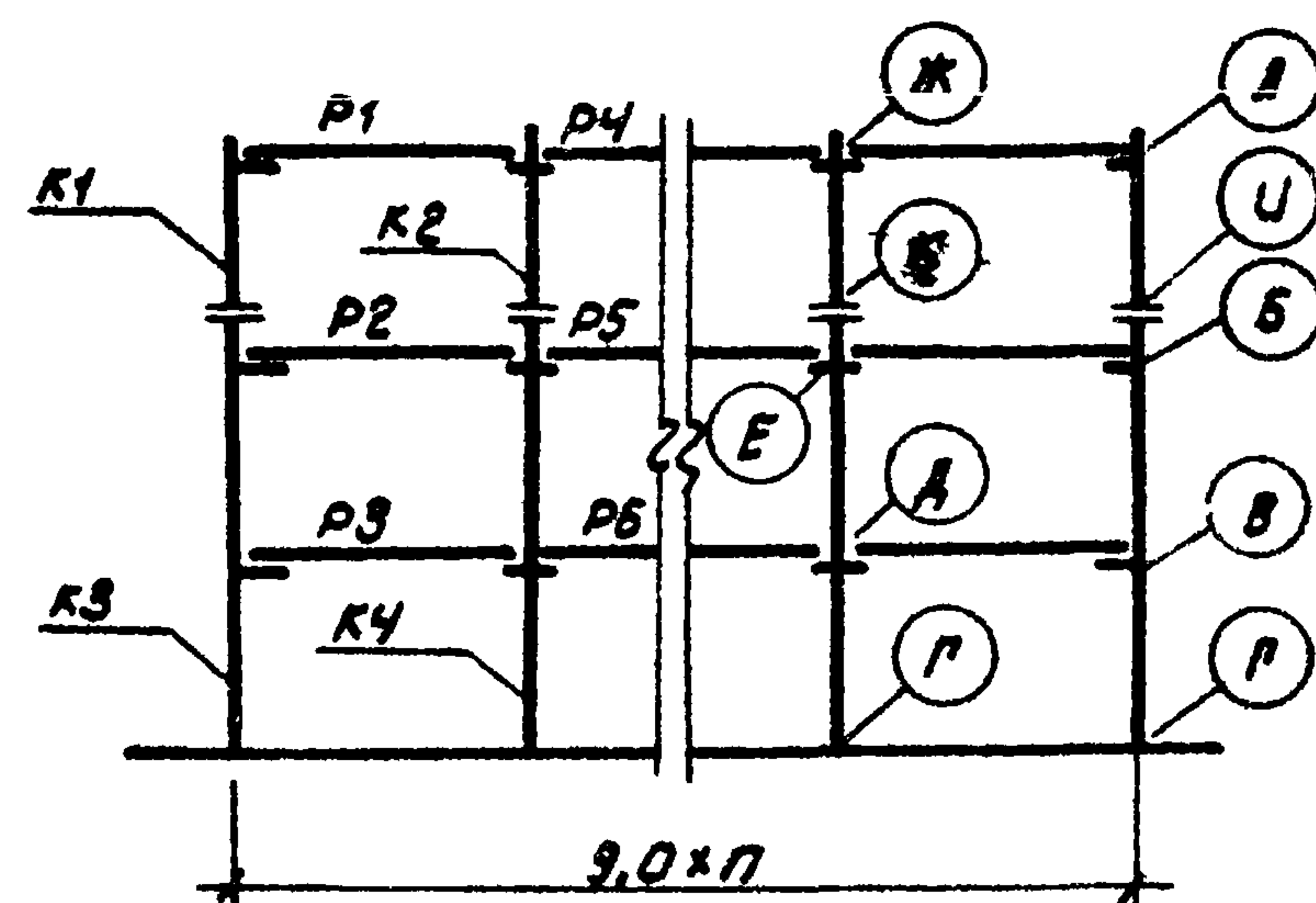
Схема рамы п-9-3 (60;48)
