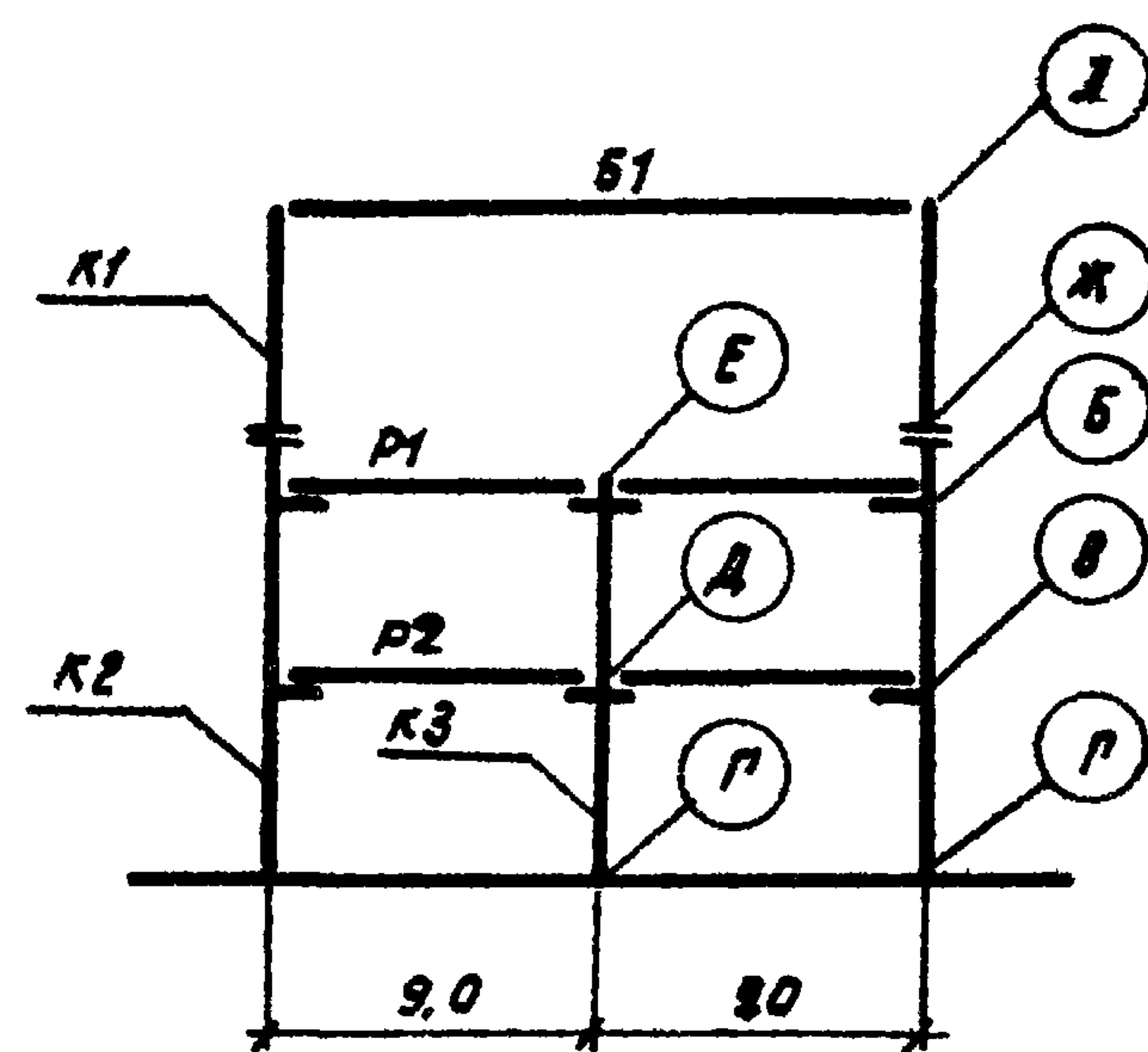
Схема рамы 2-9-3 (48; 48; 72)
