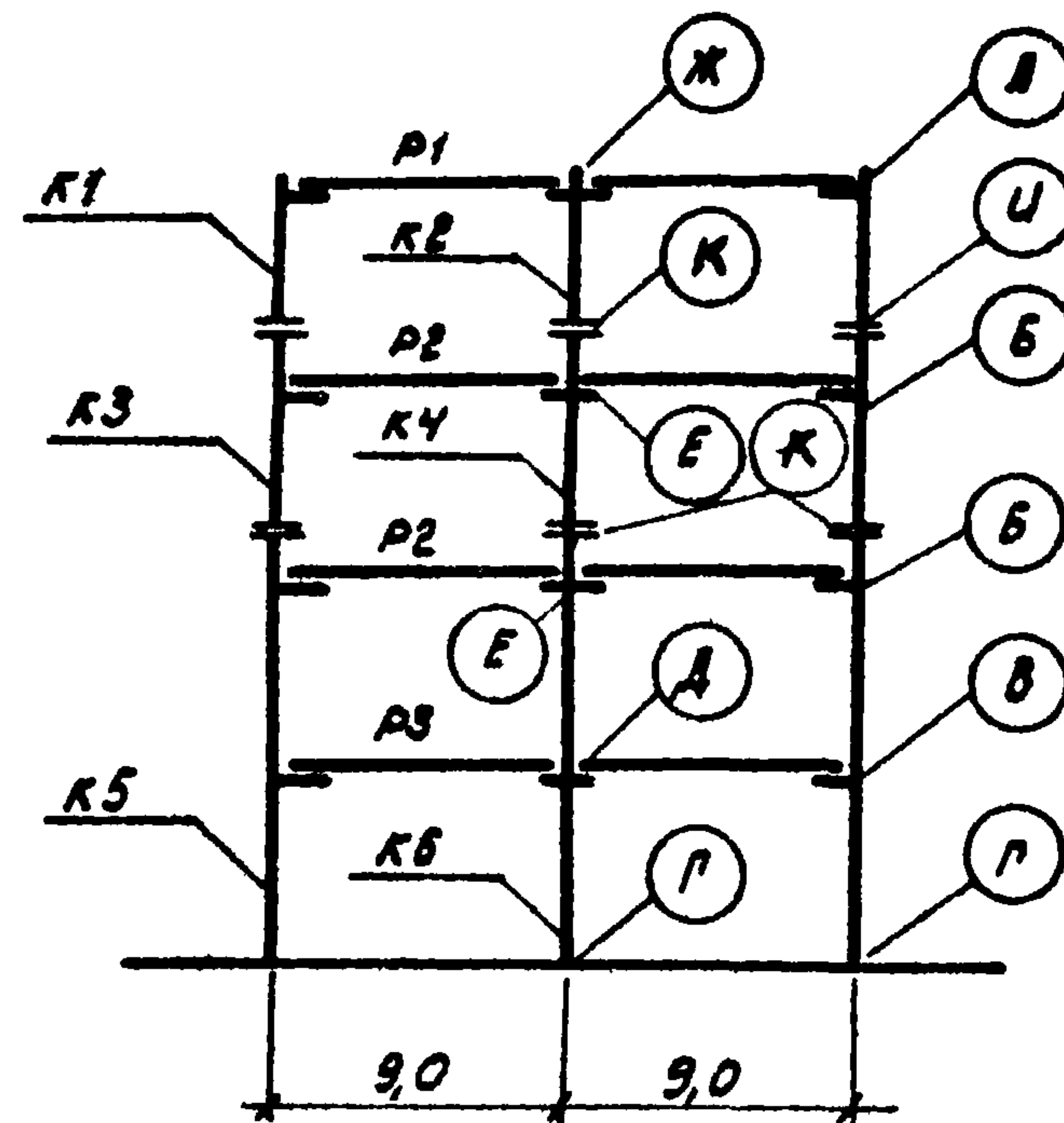
Схема рамы 2-9-4 (72; 60)
