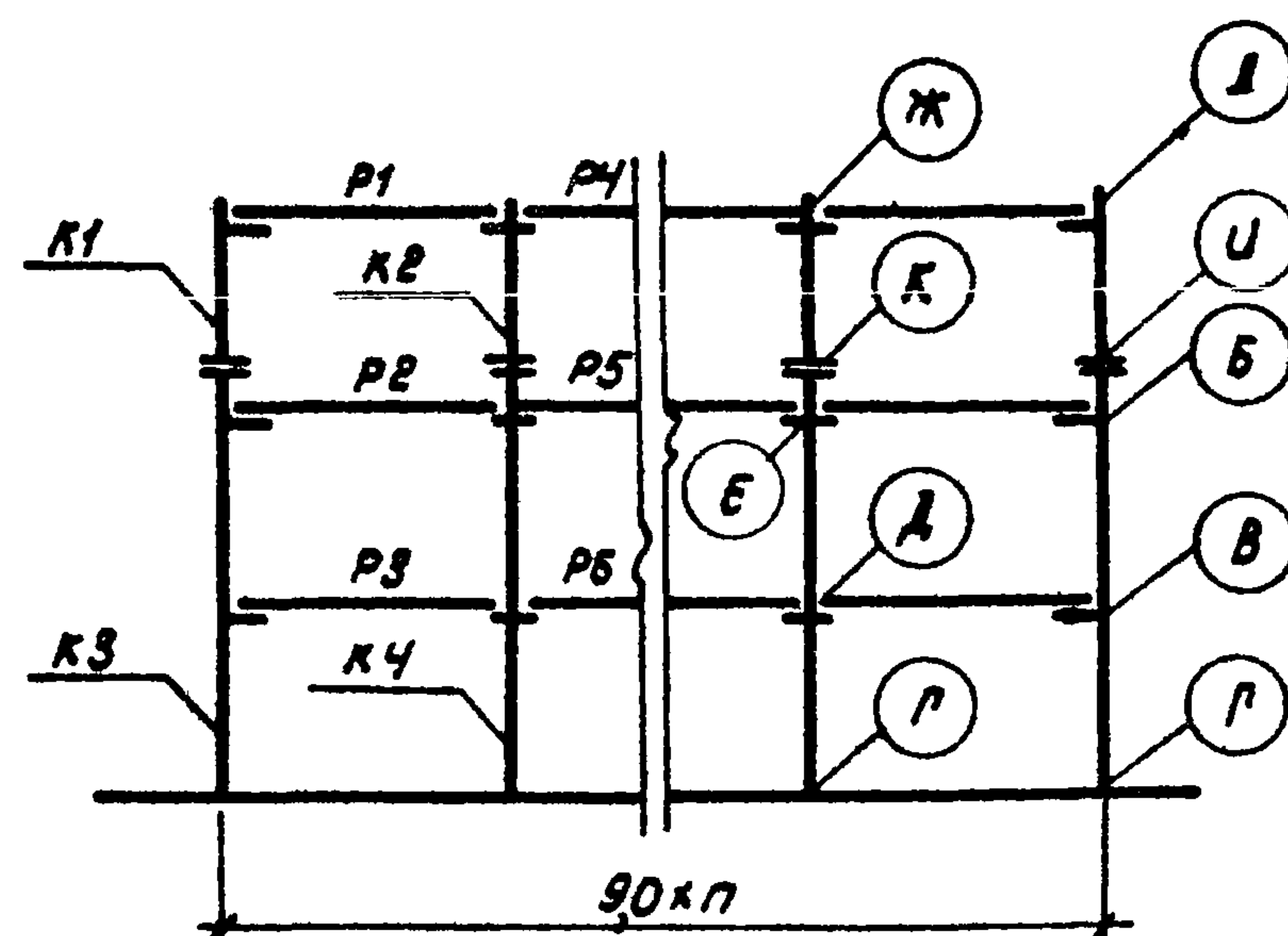
Схема рамы п-9-3 (48)
