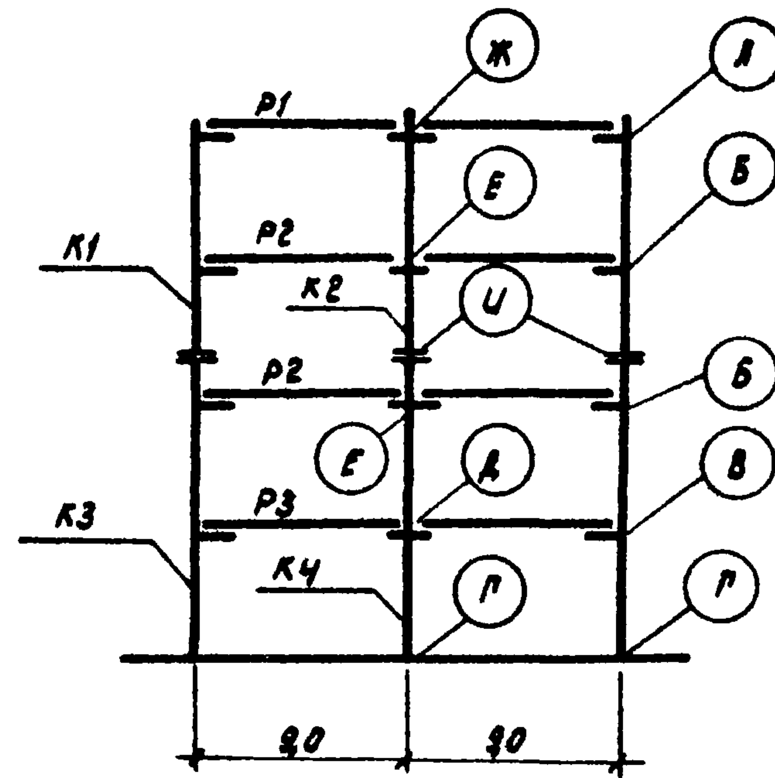
Схема рамы 2-9-4 (48)
