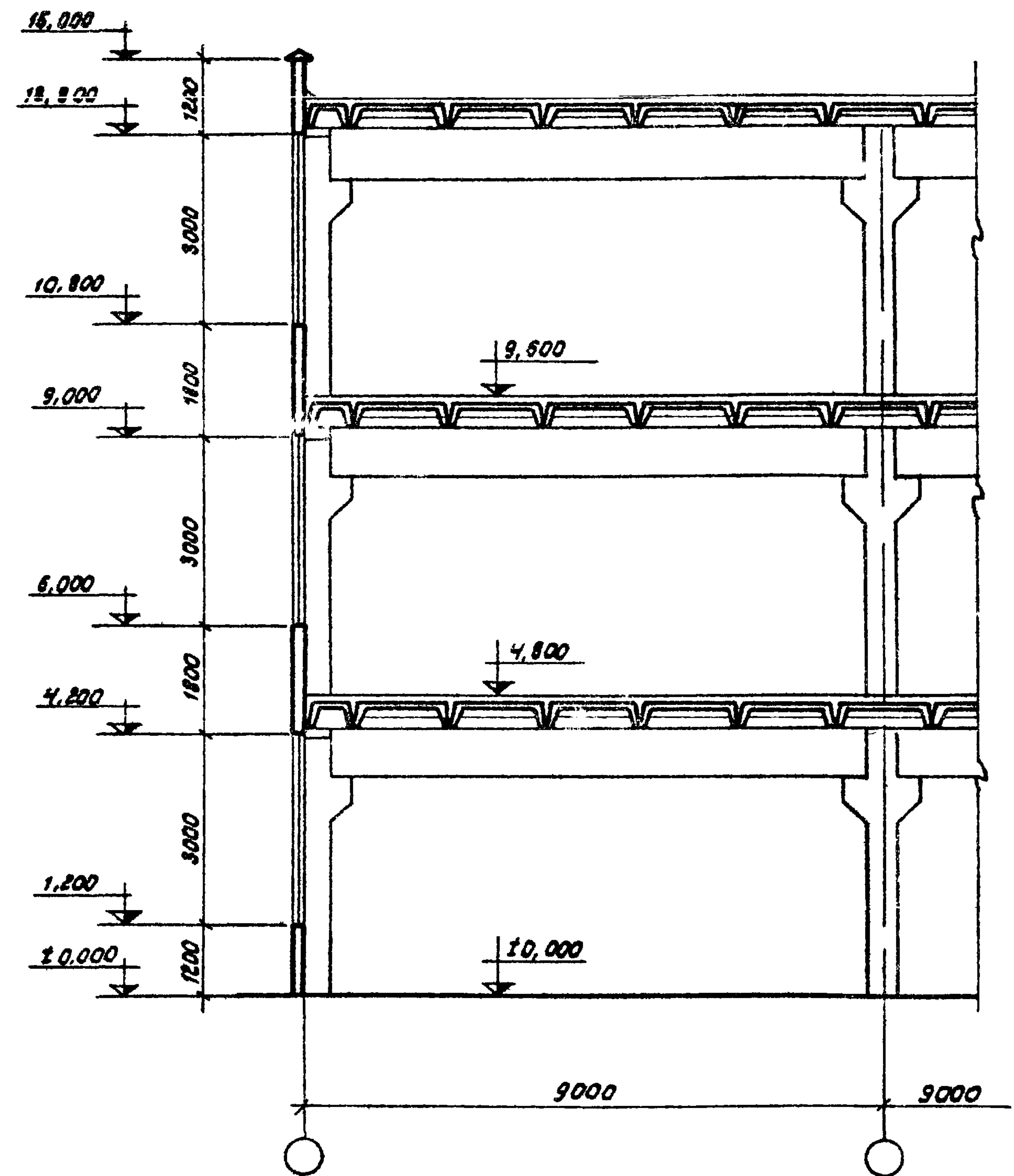
Поперечный разрез (пример)
