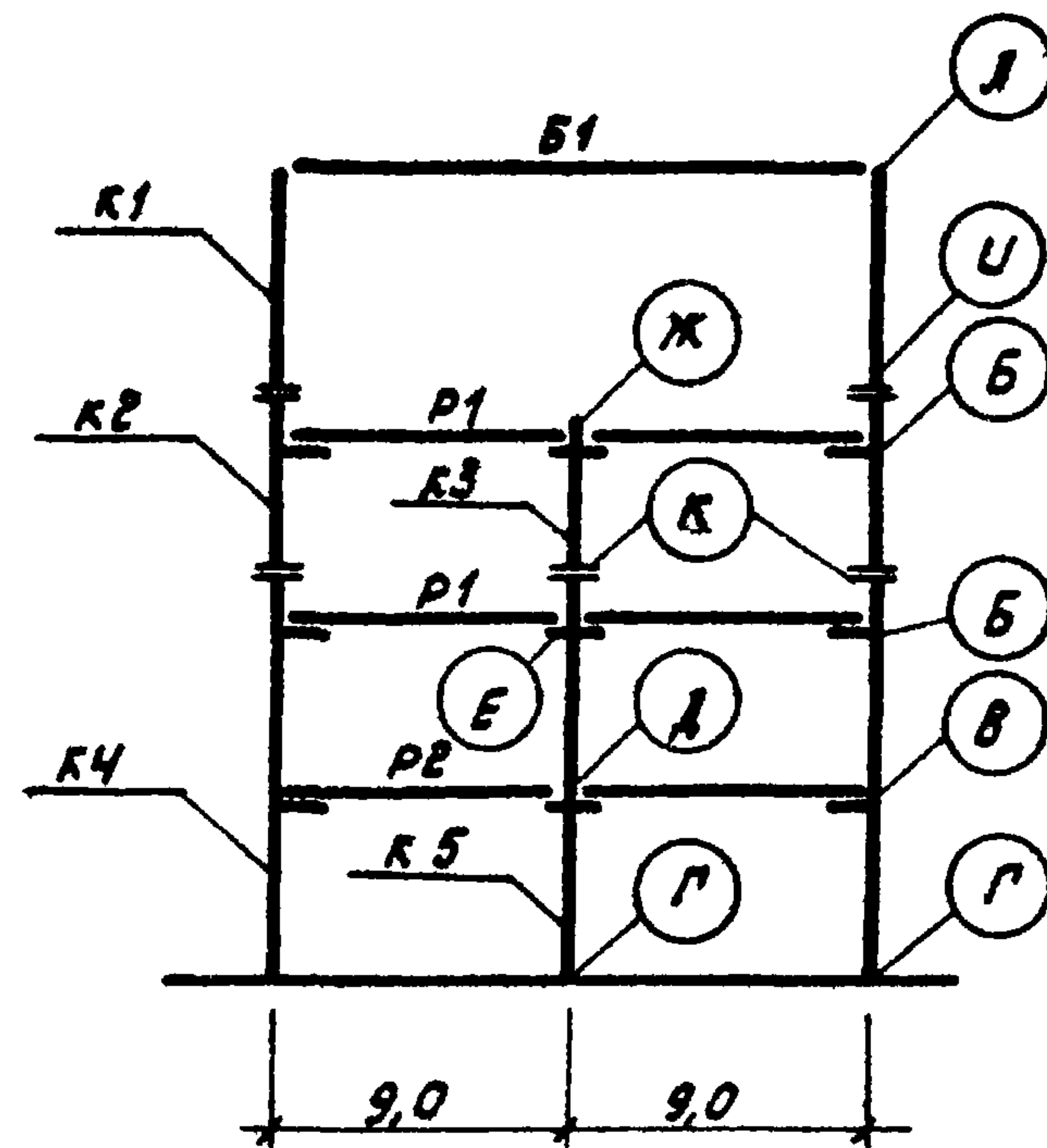
Схема рамы 2-9-4 (48; 48; 72)
