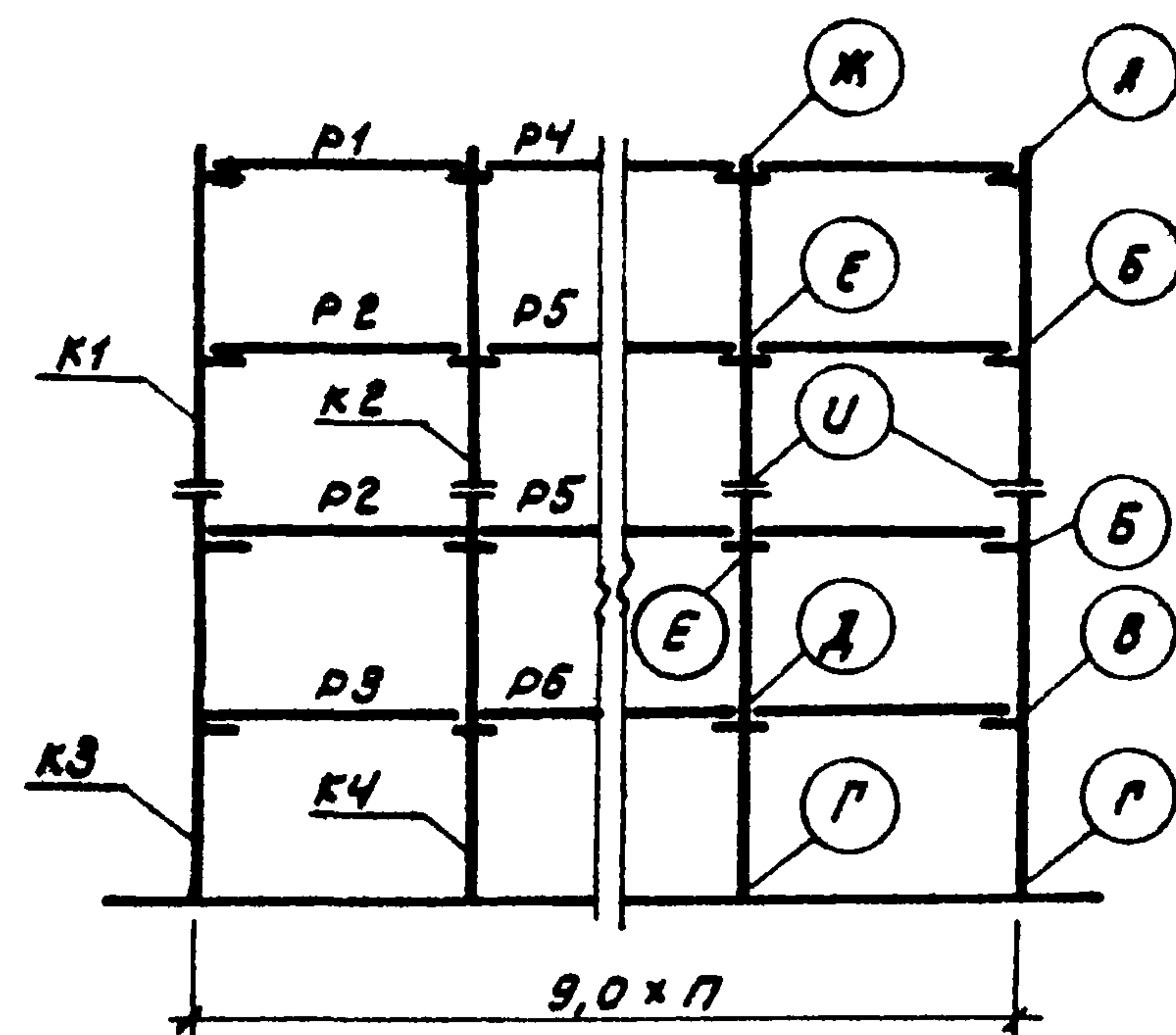
Схема рамы п-9-4 (60, 48)
