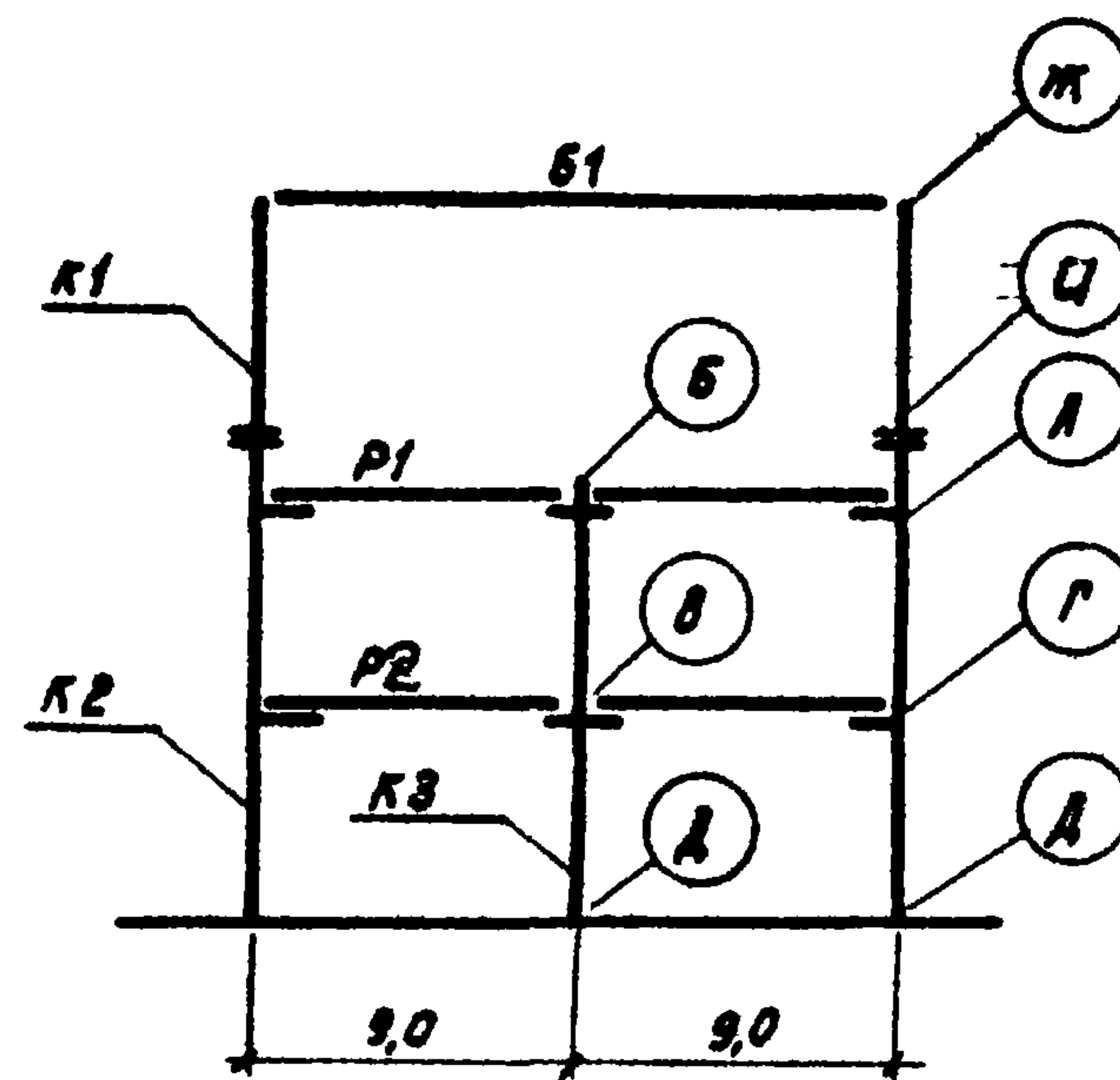
Схема рамы 2-9-3 (60; 60; 72)
