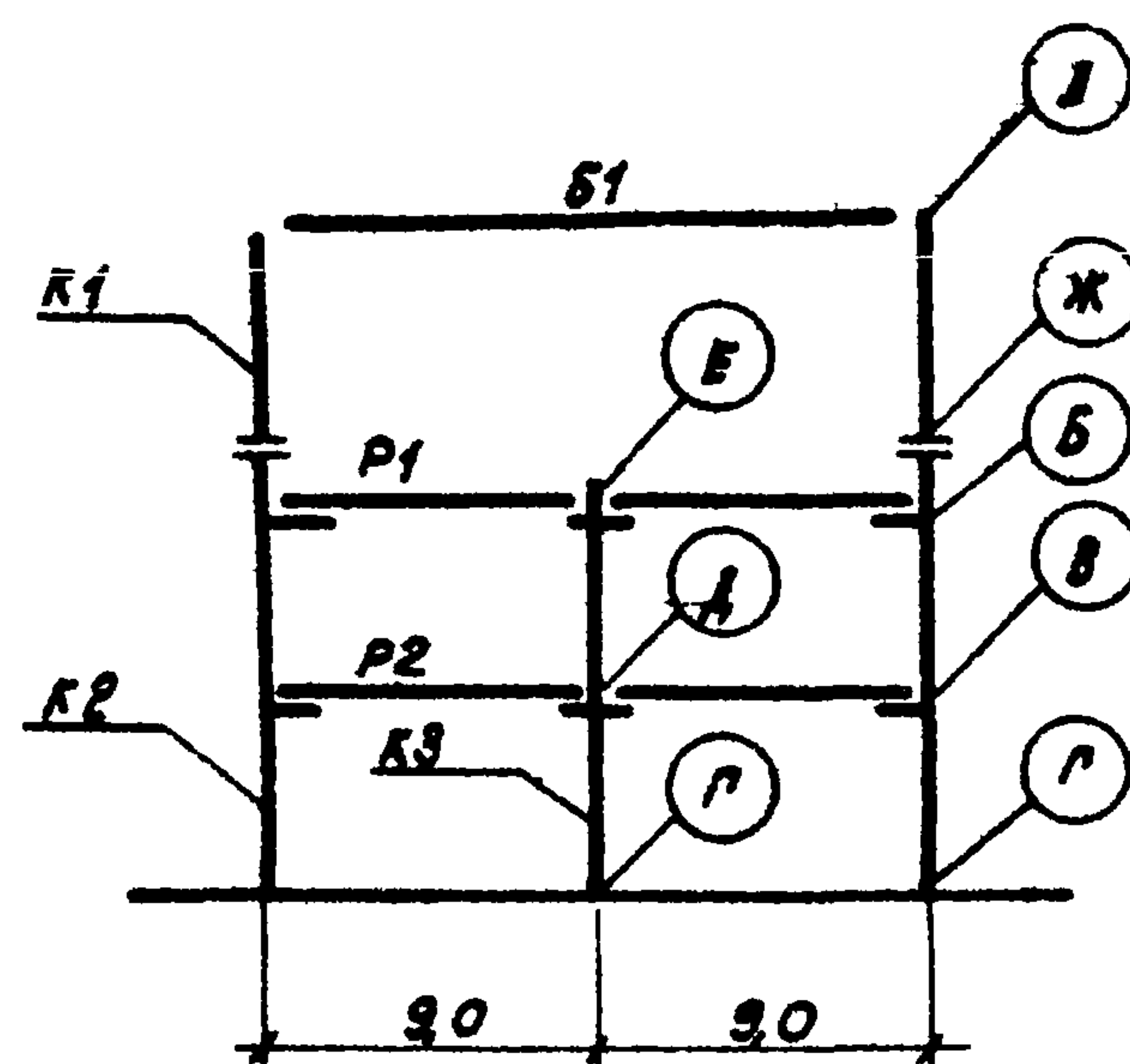
Схема рамы 2-9-3 (48; 48; 72)
