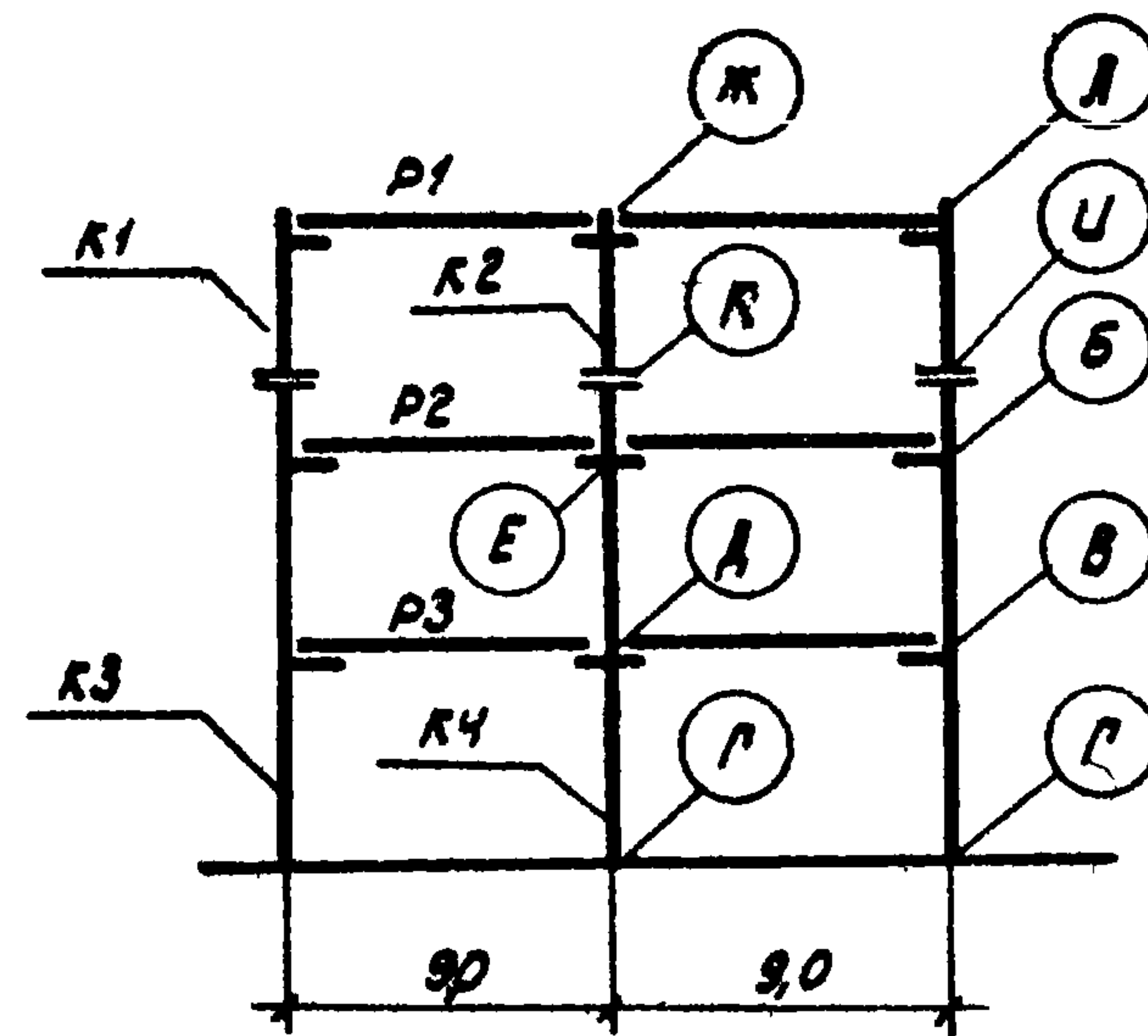
Схема рамы 2-9-3 (72; 60)
