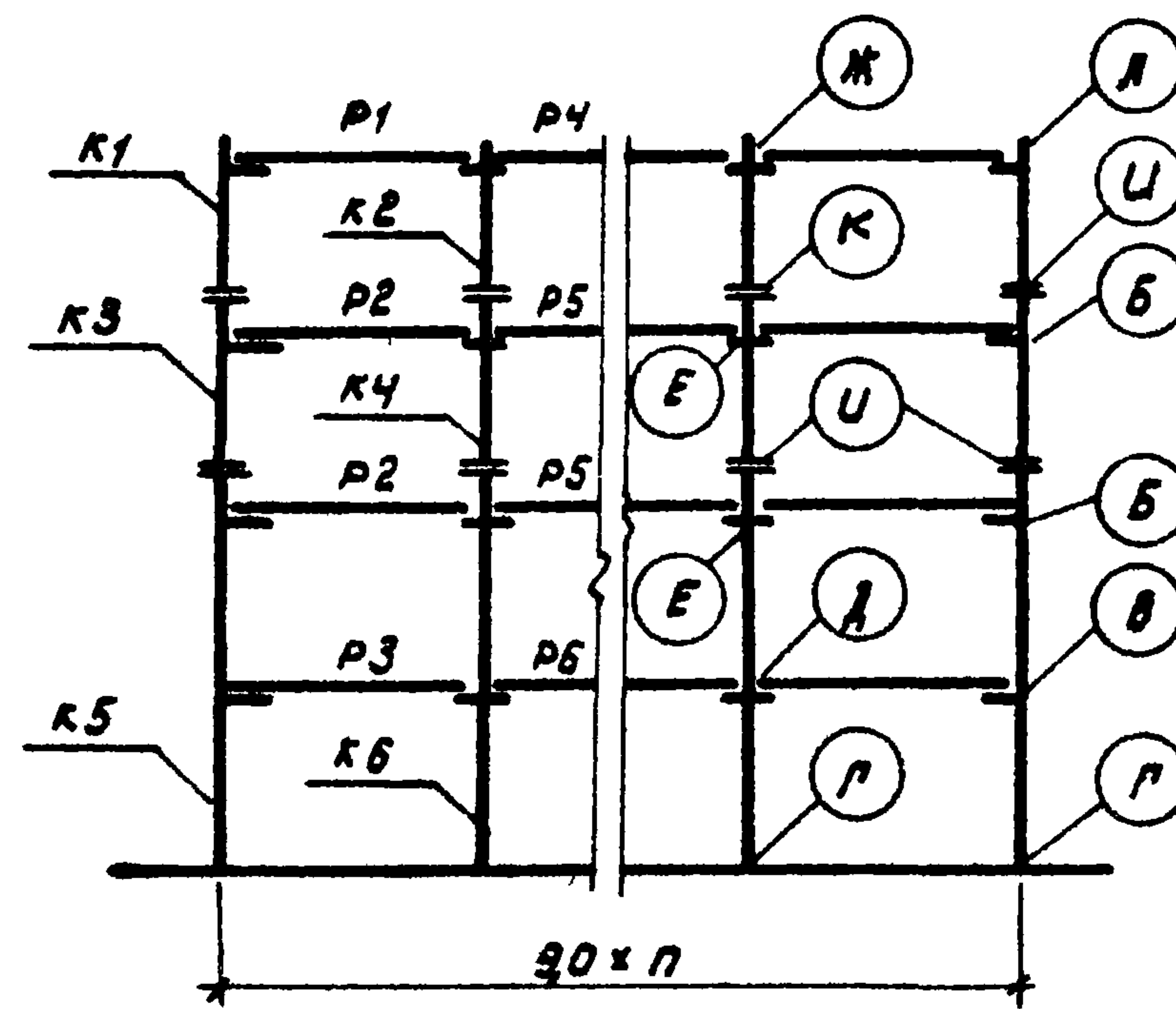
Схема рамы п-9-4 (72, 60)
