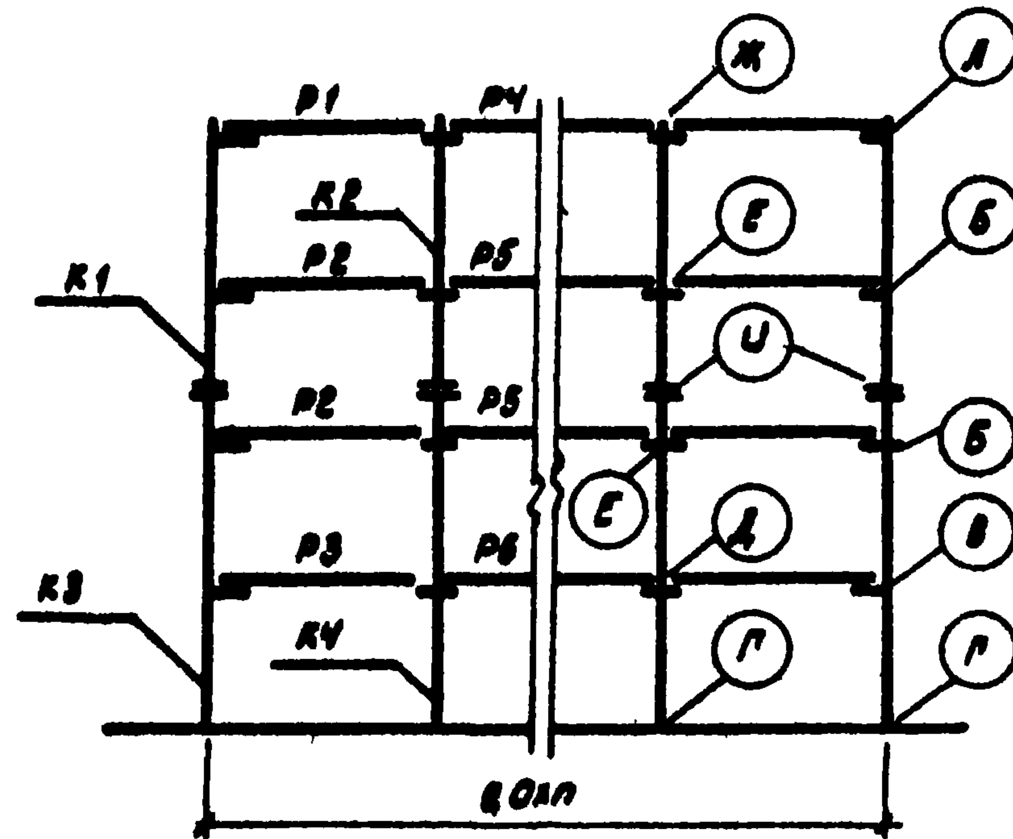
Схема рамы П-9-4 (48)
