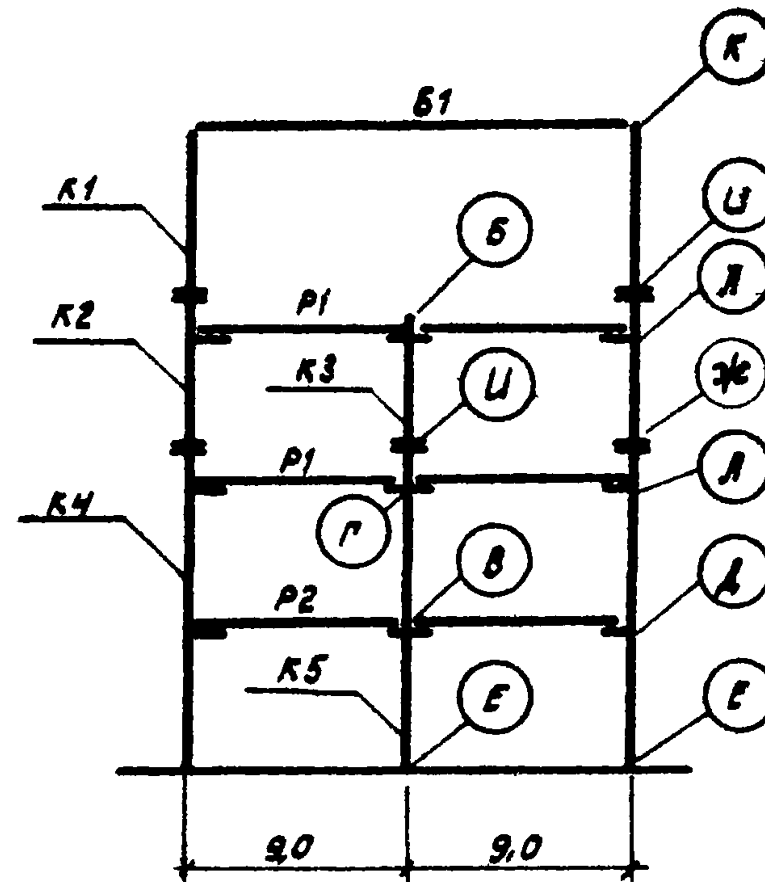
Схема рамы 2-9-4 (60; 60; 72)
