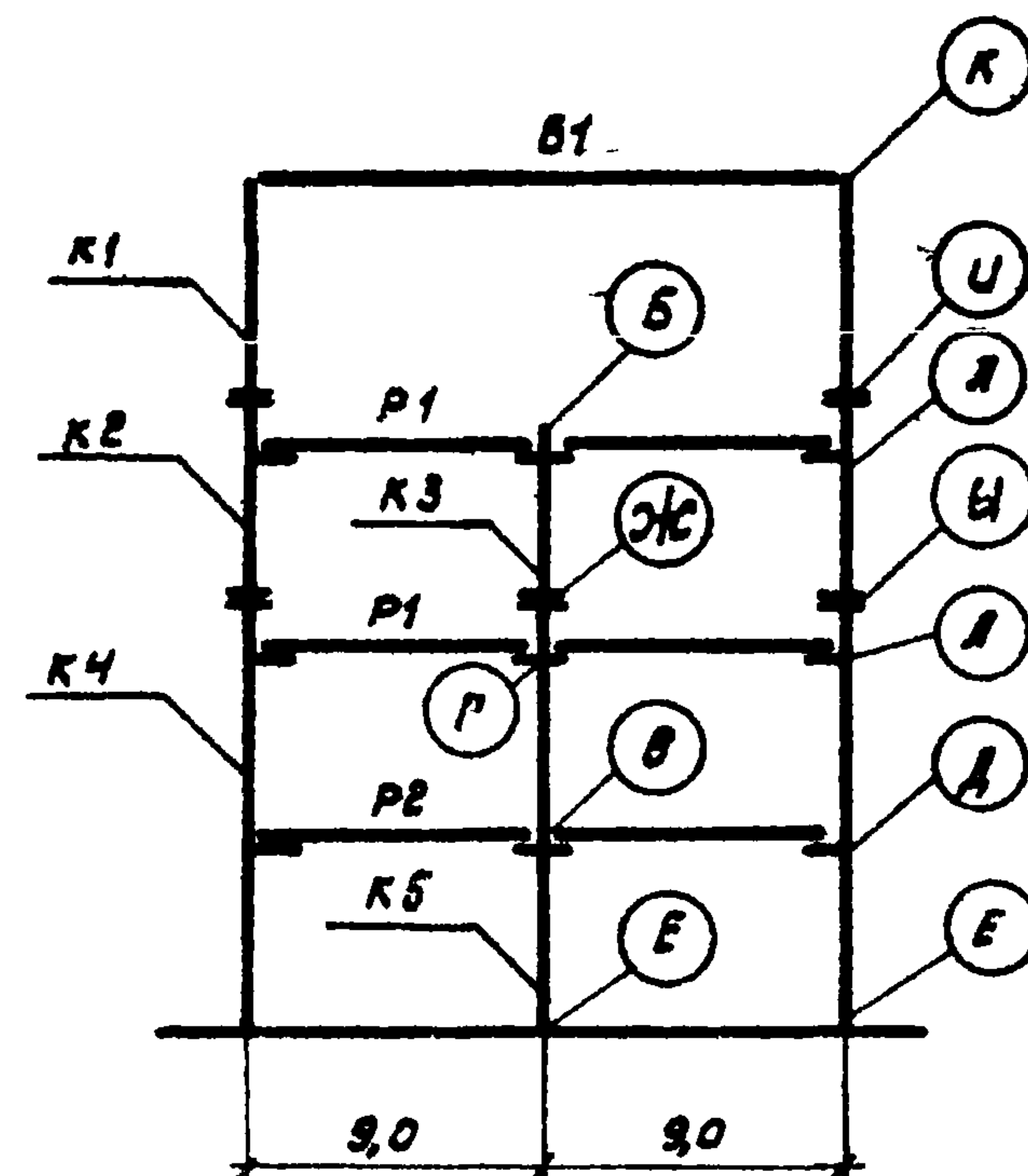
Схема рамы 2-9-4 (60; 60; 72)
