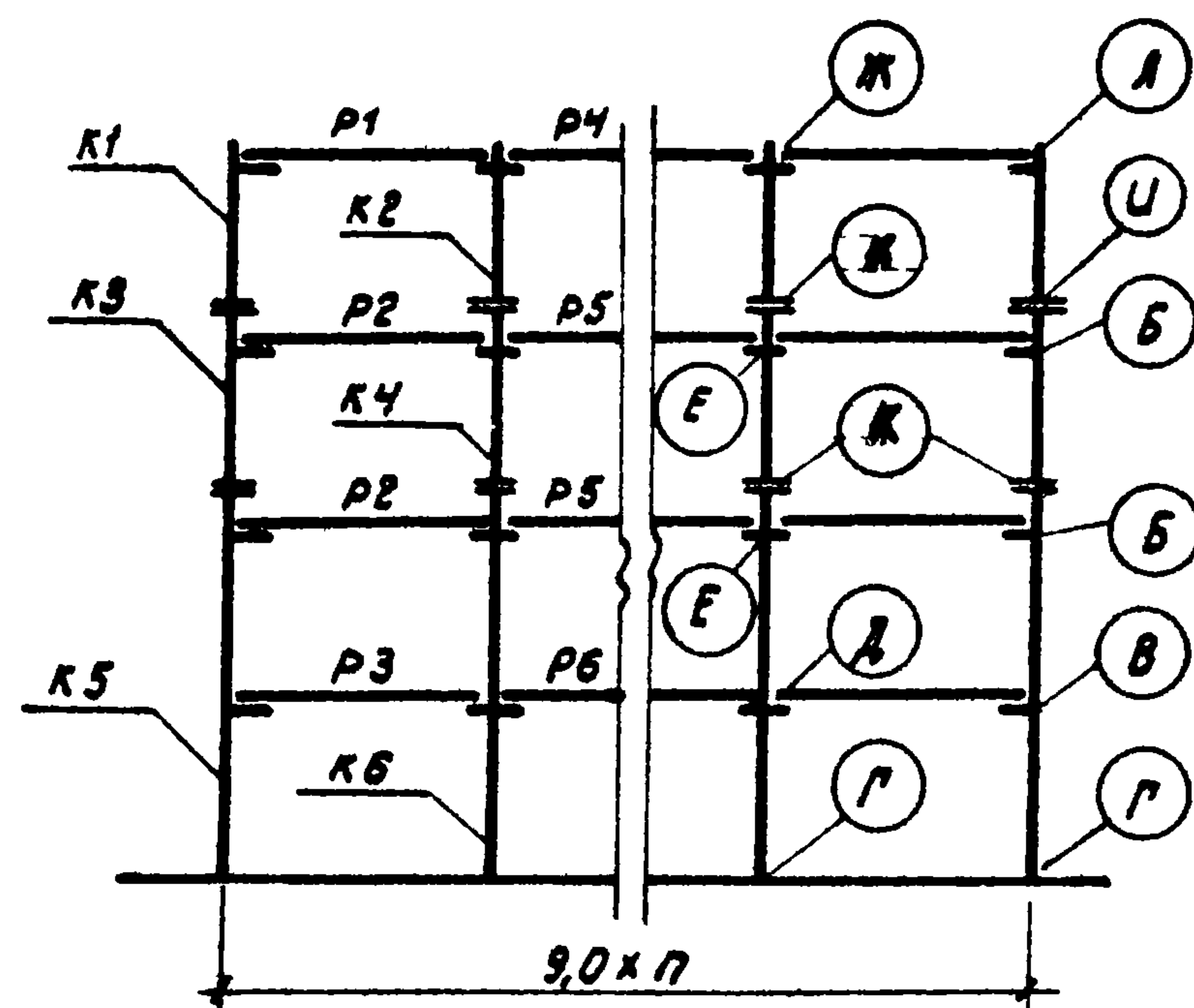
Схема рамы n-9-4 (60)
