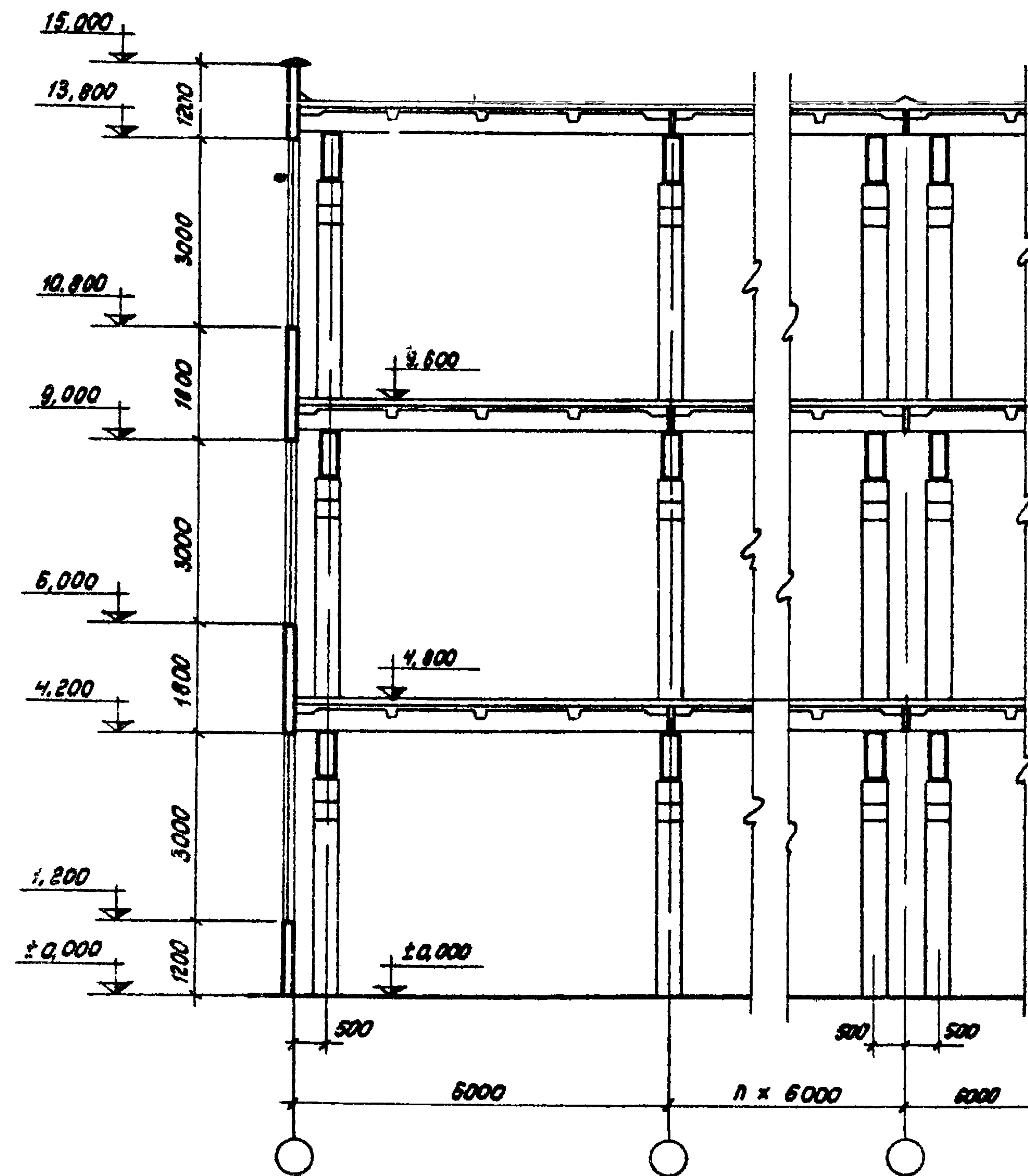
Продольный разрез (пример)
