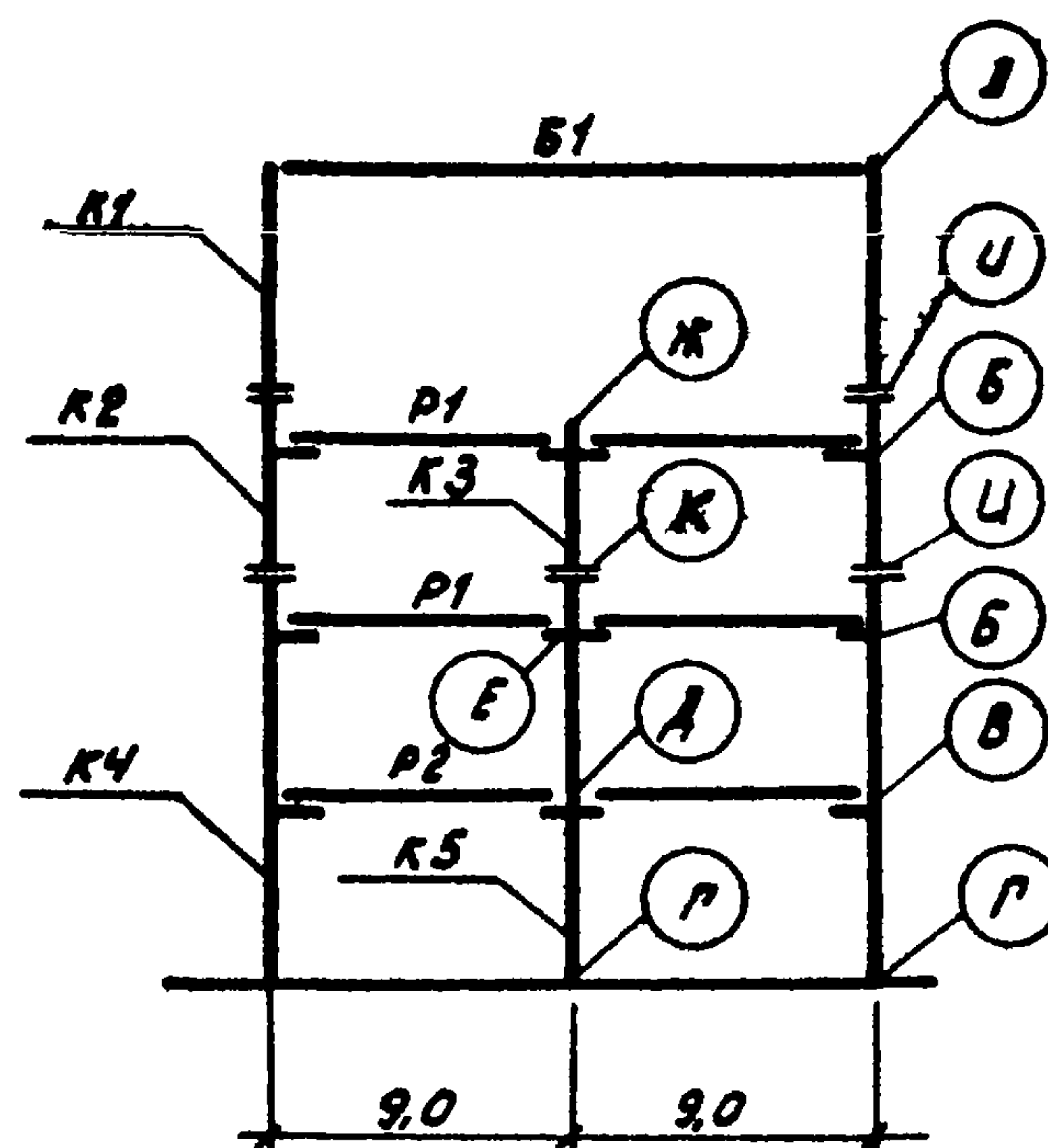
Схема рамы 2-9-4 (48; 48, 72)
