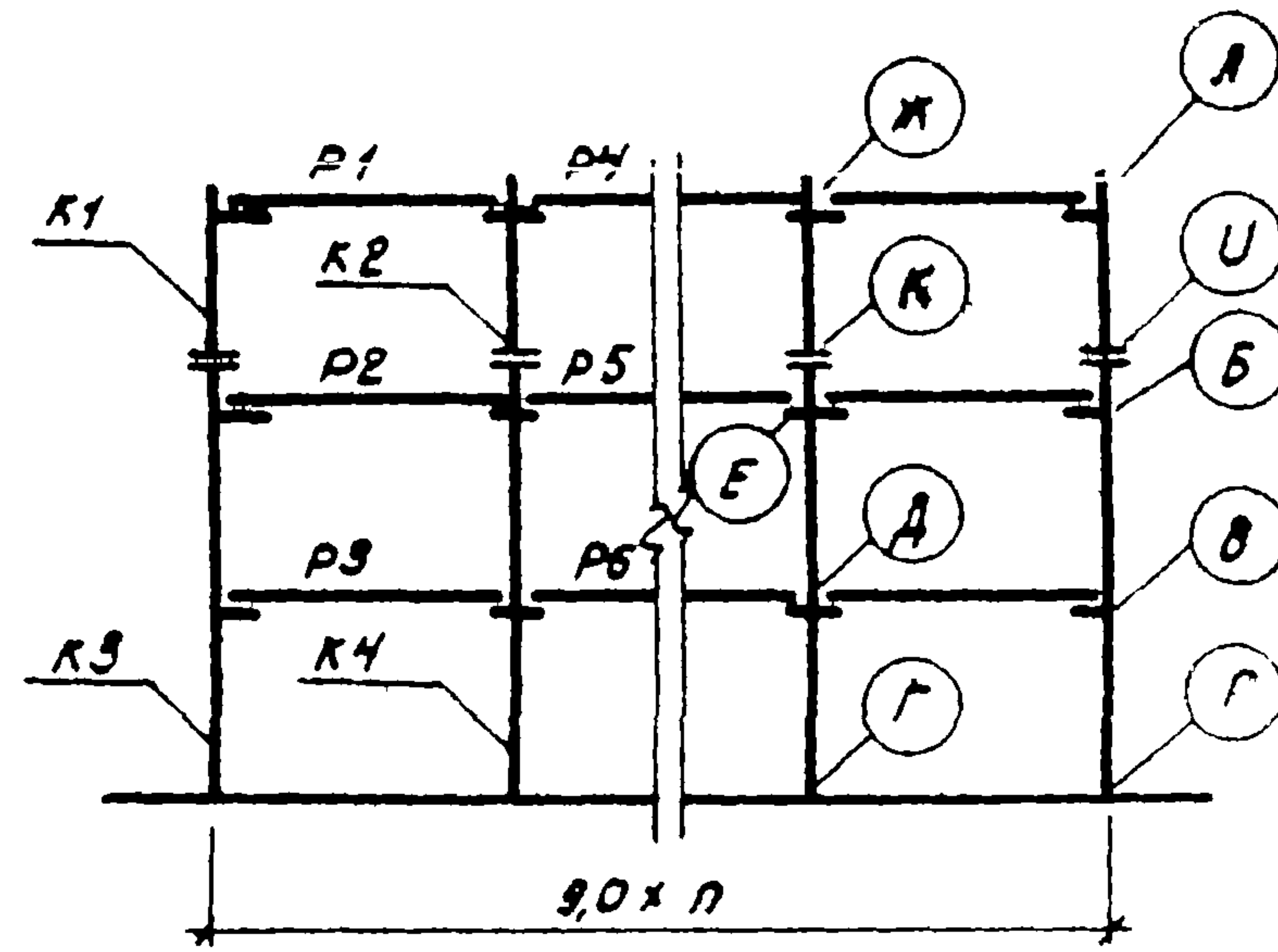
Схема рамы п-9-3 (60)
