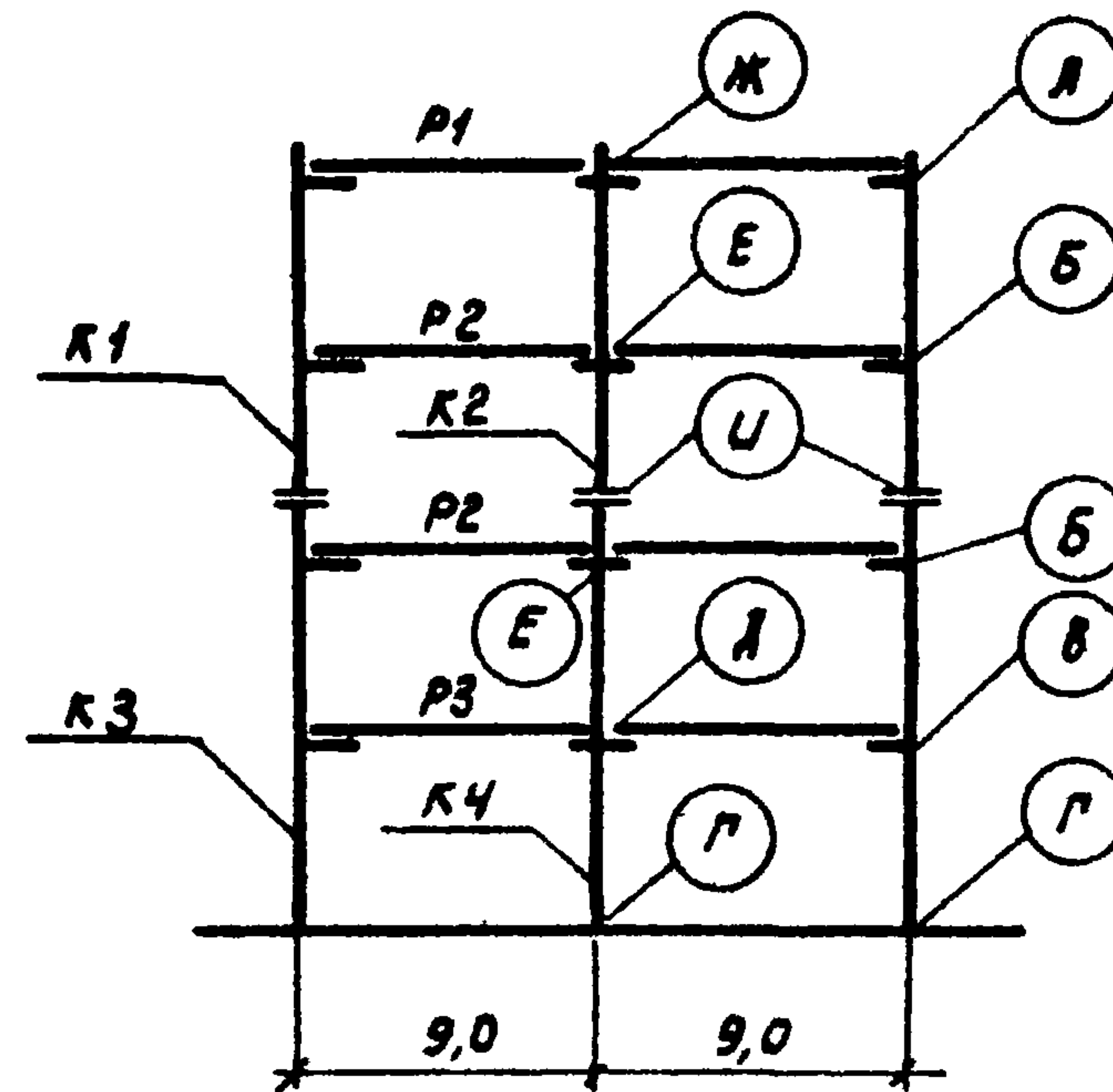
Схема рамы 2-9-4 (60; 48)
