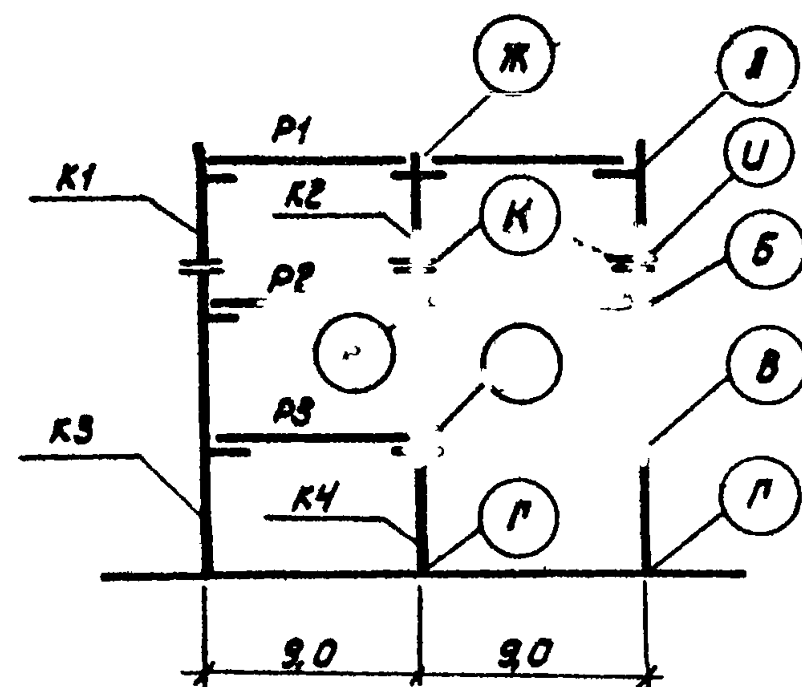
Схема рамы 2-9-3 (60; 48)
