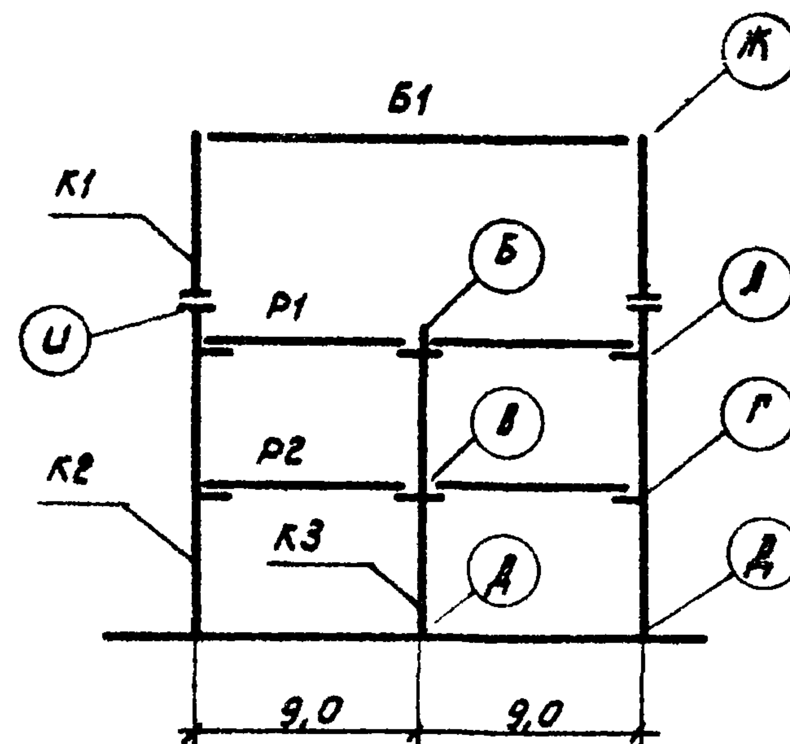
Схема рамы 2-9-3 (60; 60; 72)
