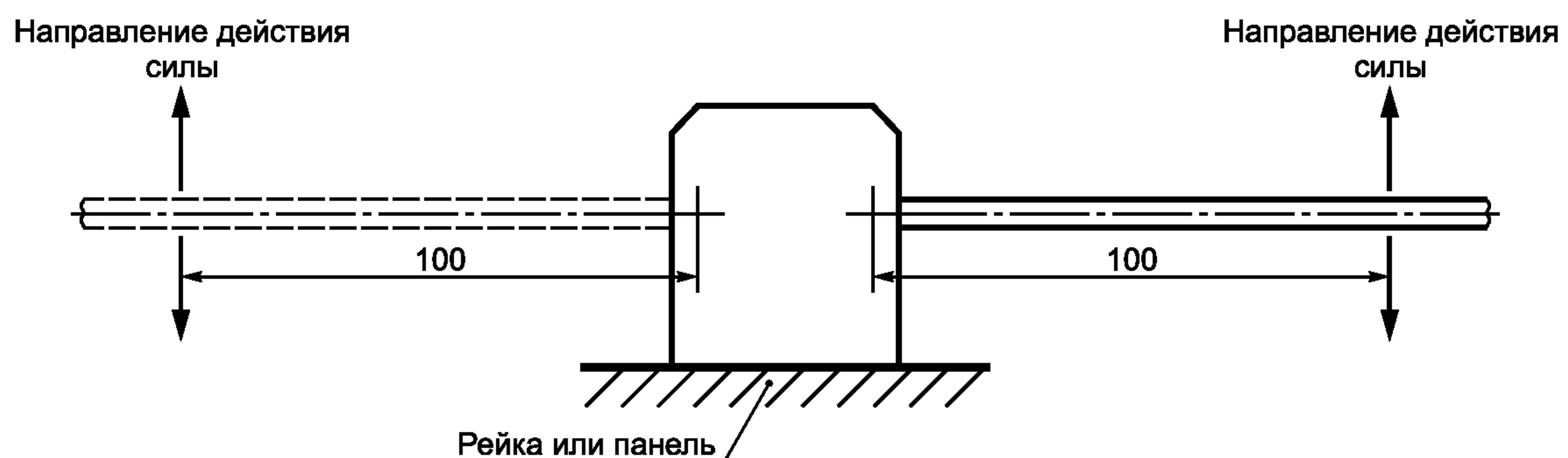
Рисунок 1 — Схема испытания по 8.3.2
