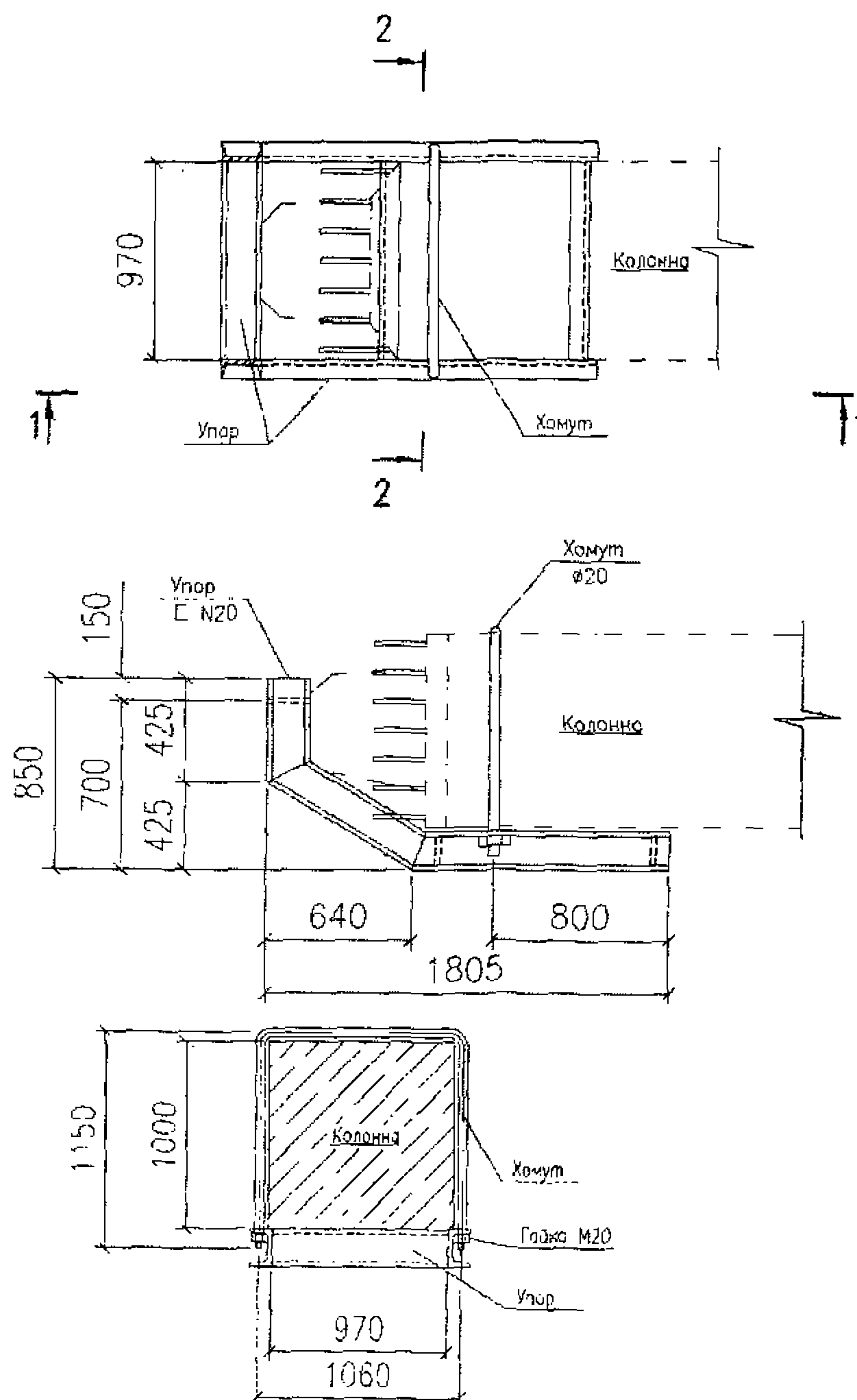
Рисунок 9.1 - Упор для колонн сечением 1000x1000 мм
