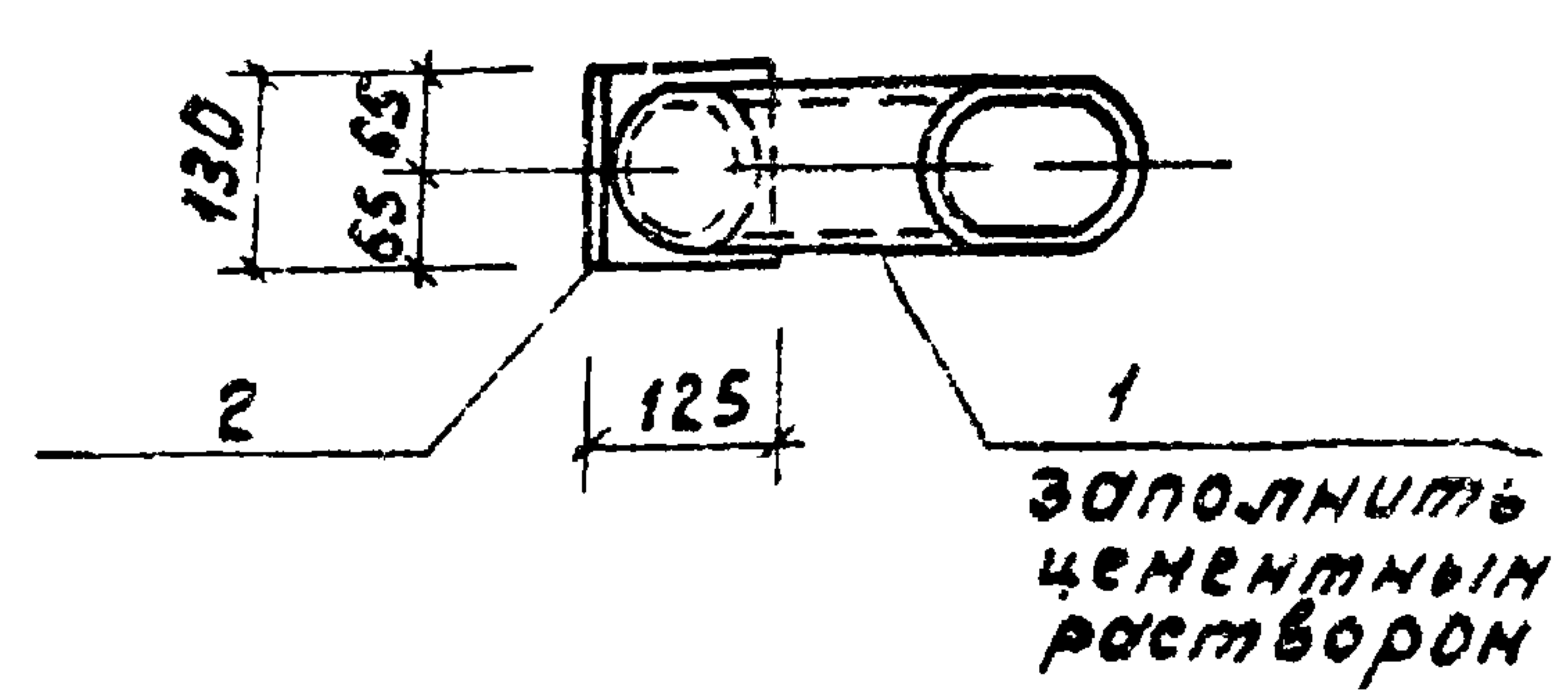
1-1 М 1:10
