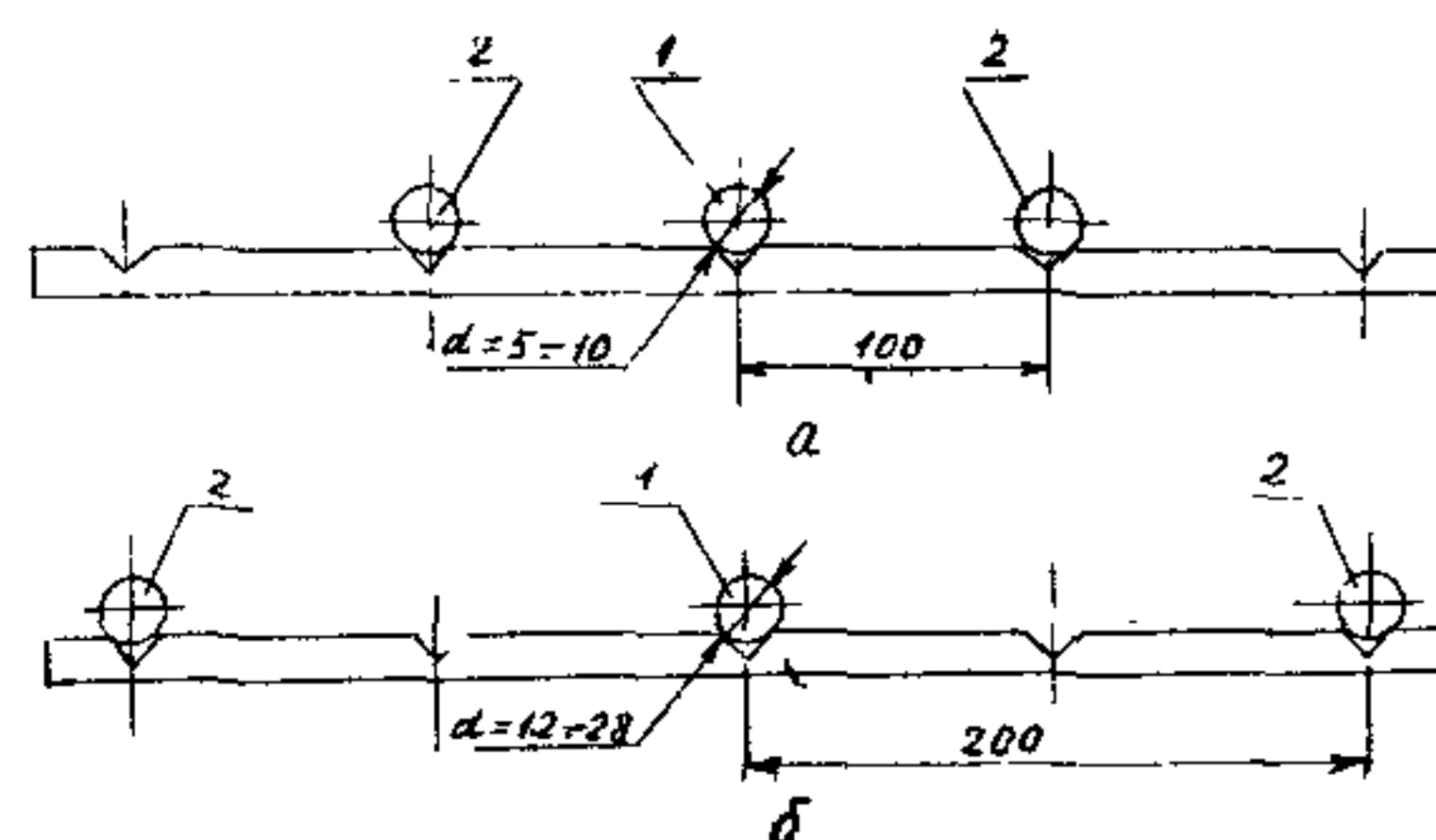
Рис.2. Схемы размещения образцов при испытании по п.6.4.5 1 - контролируемый образец; 2 - соседние образцы
