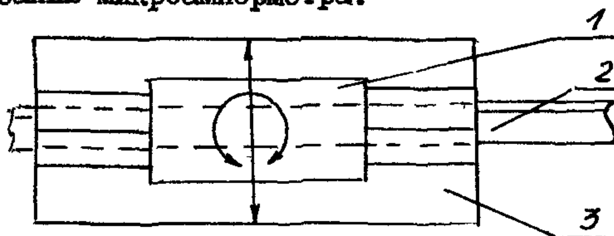
Рис. 3. Установка преобразователя на поверхности прокладки
