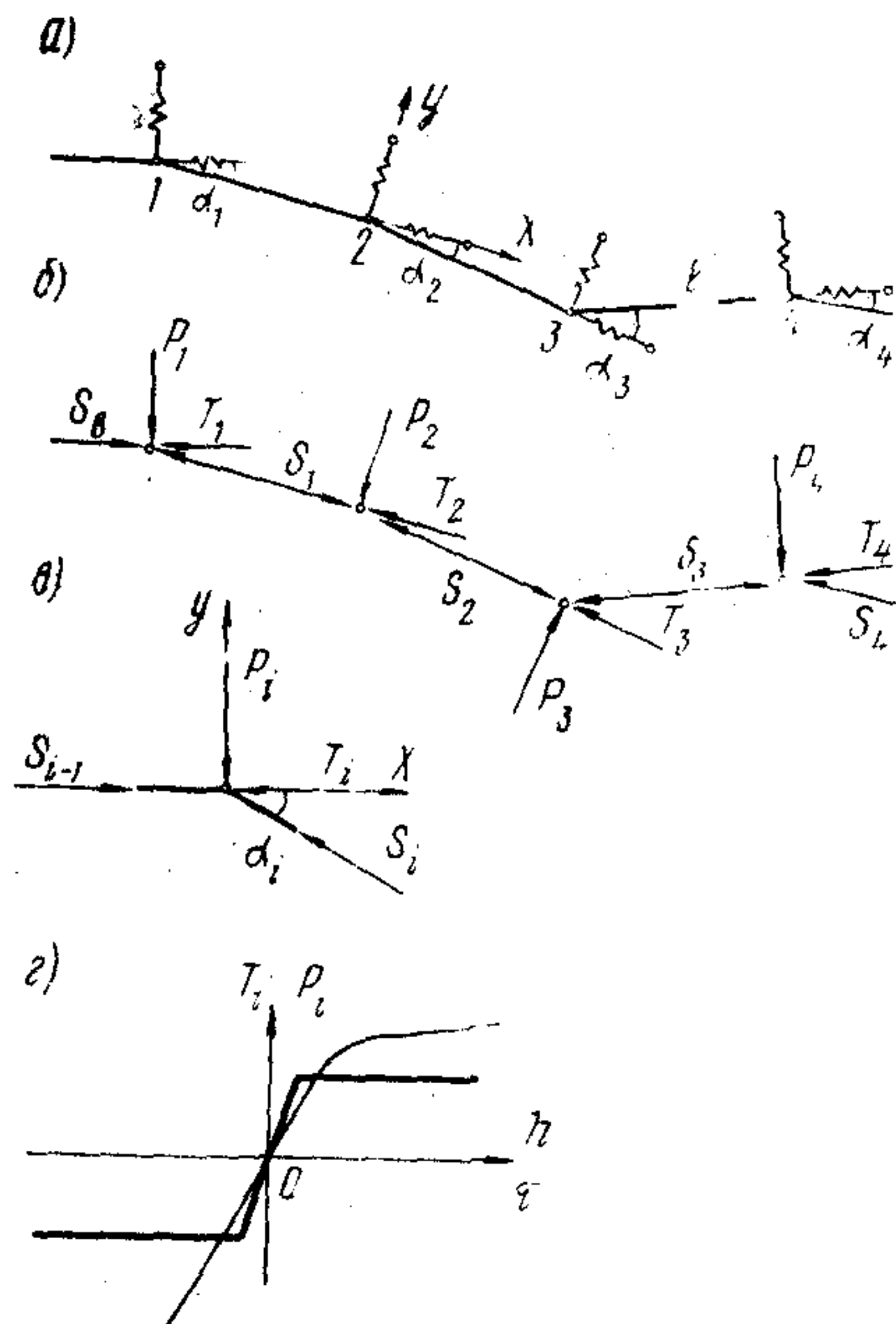
Рис.18. Расчетная схема безмоментного расчета кинематической цепи:
