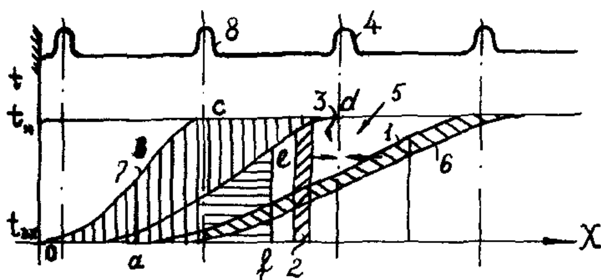
Рис.17. Схема нагружения компенсаторов подземного трубопровода продольными перемещениями при захлаживании:
