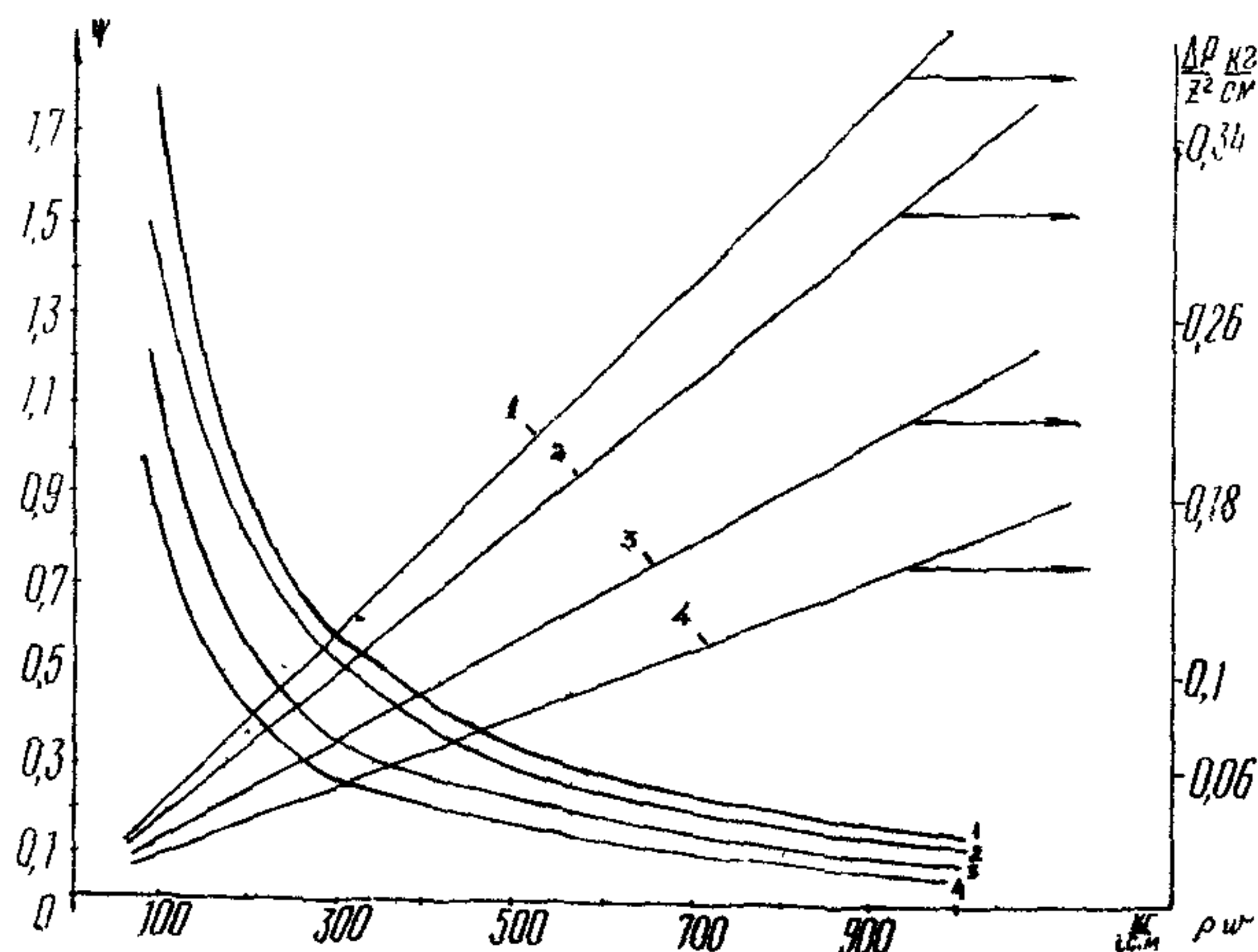
Рис.8. Значения f и \frac{\Delta P}{L^2} в зависимости от \rho w и w^2 :
