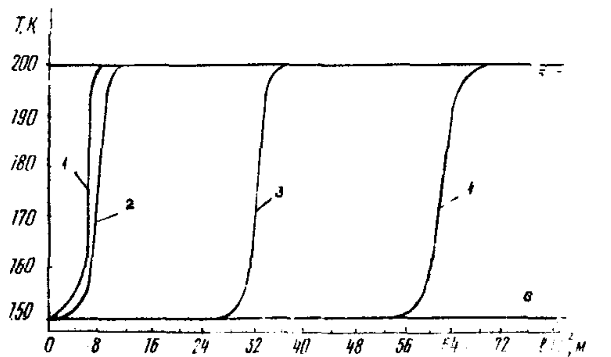
Рис. 4. Изменение температуры стенки трубопровода диаметром 1420 мм по длине при захолаживании его от 200 К до 150 К (второй этап захолаживания):
