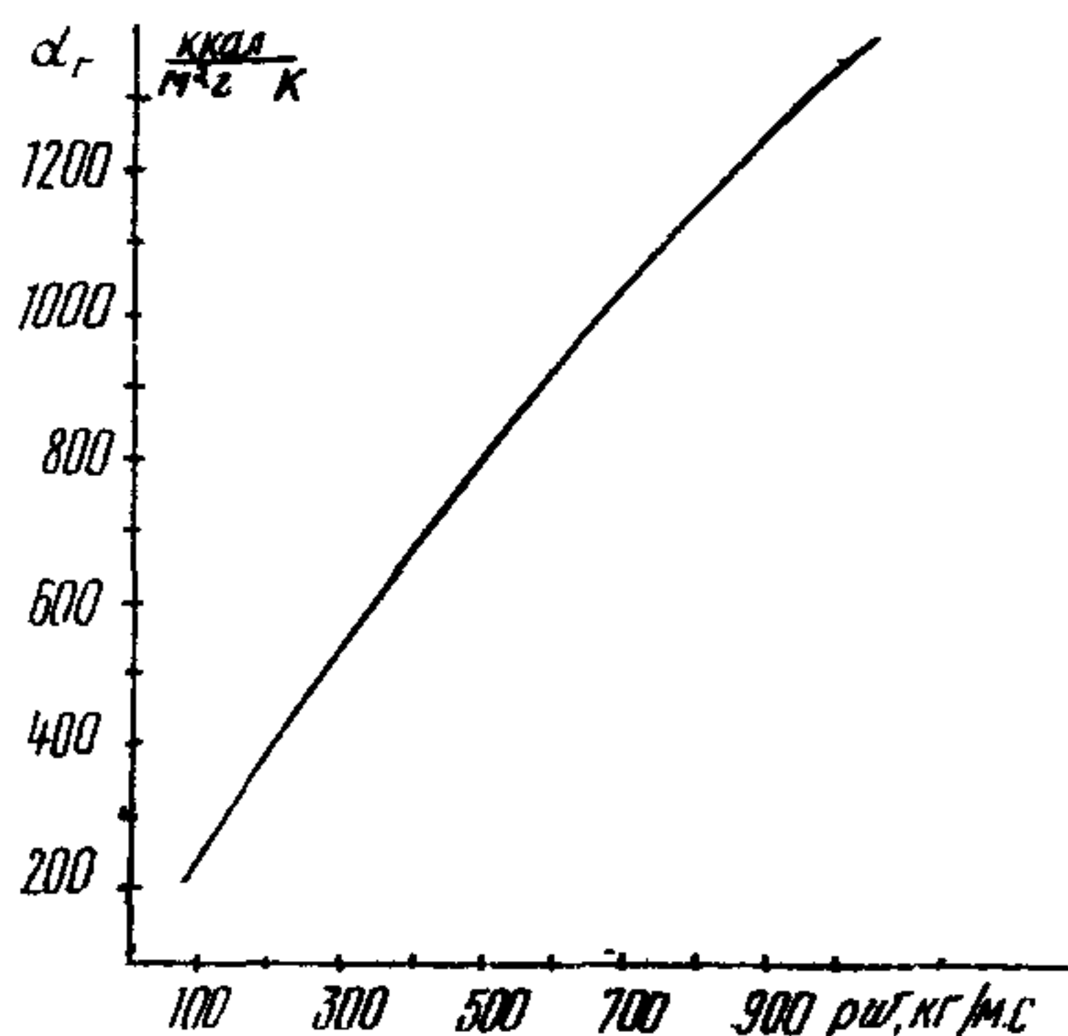
Рис. 6. Значения \alpha_r в зависимости от массовой скорости ( \rho w ) в процессе захлаживания участка трубопровода диаметром 1420 мм
