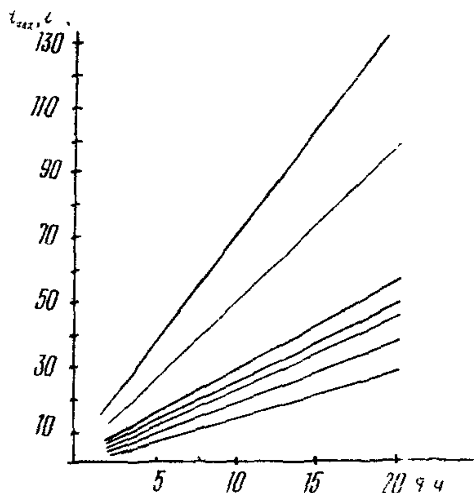
Рис.7. Диаграмма для приближенной оценки времени заохлаживания участка трубопровода диаметром 1420 мм протяженностью L при средней скорости газа w для разных значений f :
