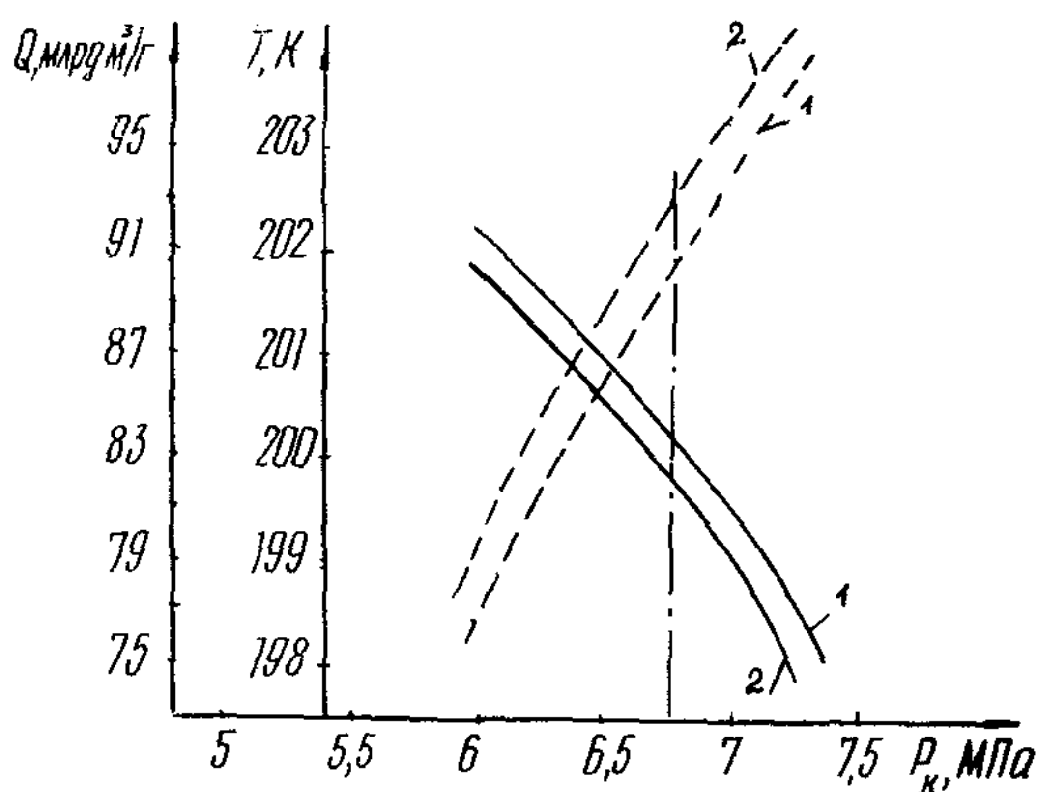
Рис.3. Зависимость производи- тельности трубо- провода ОПГ ( Q ) и температуры ОПГ ( T ) в конце участка от конеч- ного давления P_k = = 6,763 МПа; P_H = = 9,806 МПа; T_{H2} = 210 К; K = 0,43 Вт/м 2 ·К
