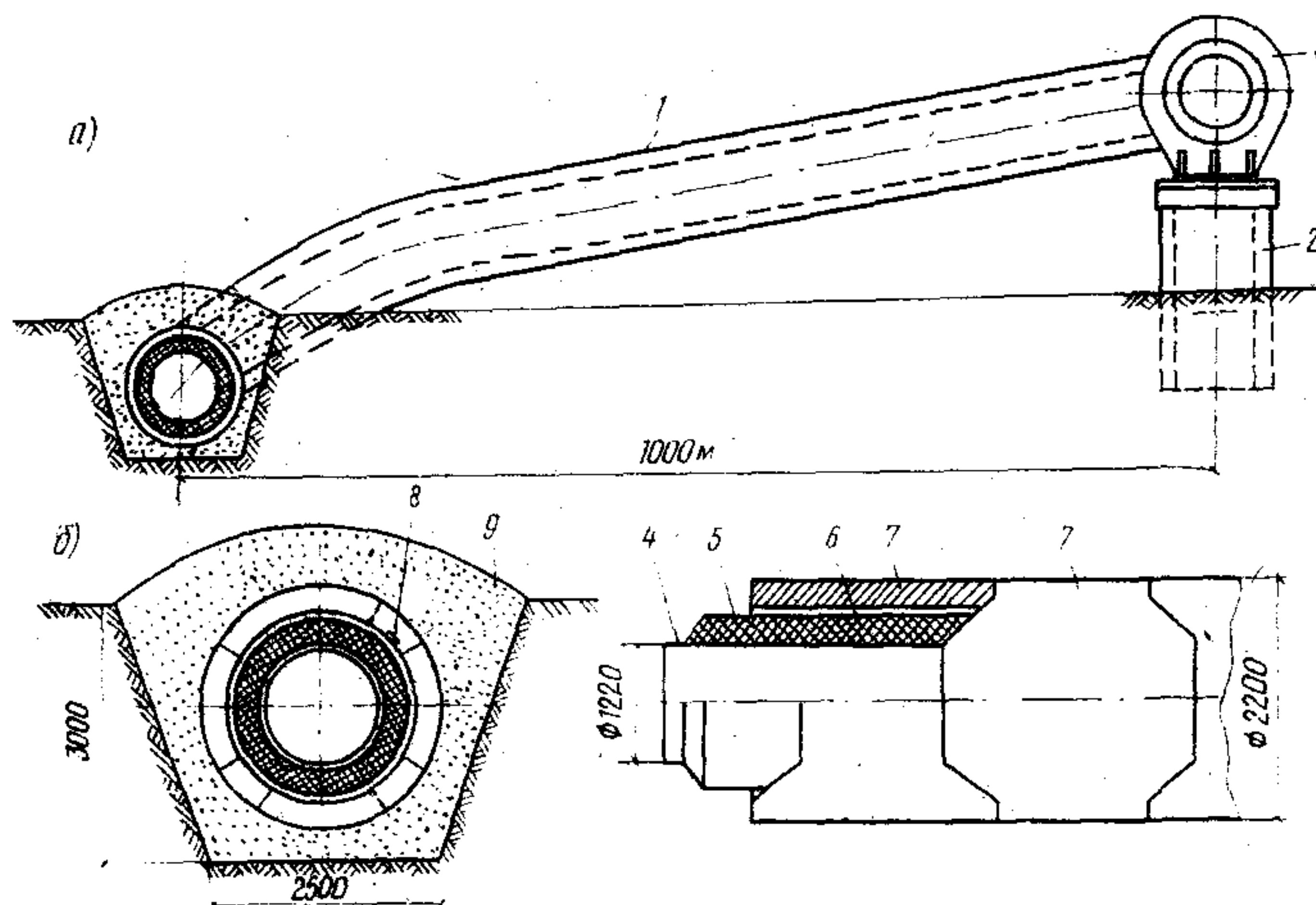
Рис. II. Узлы подземного трубопровода СПГ:
