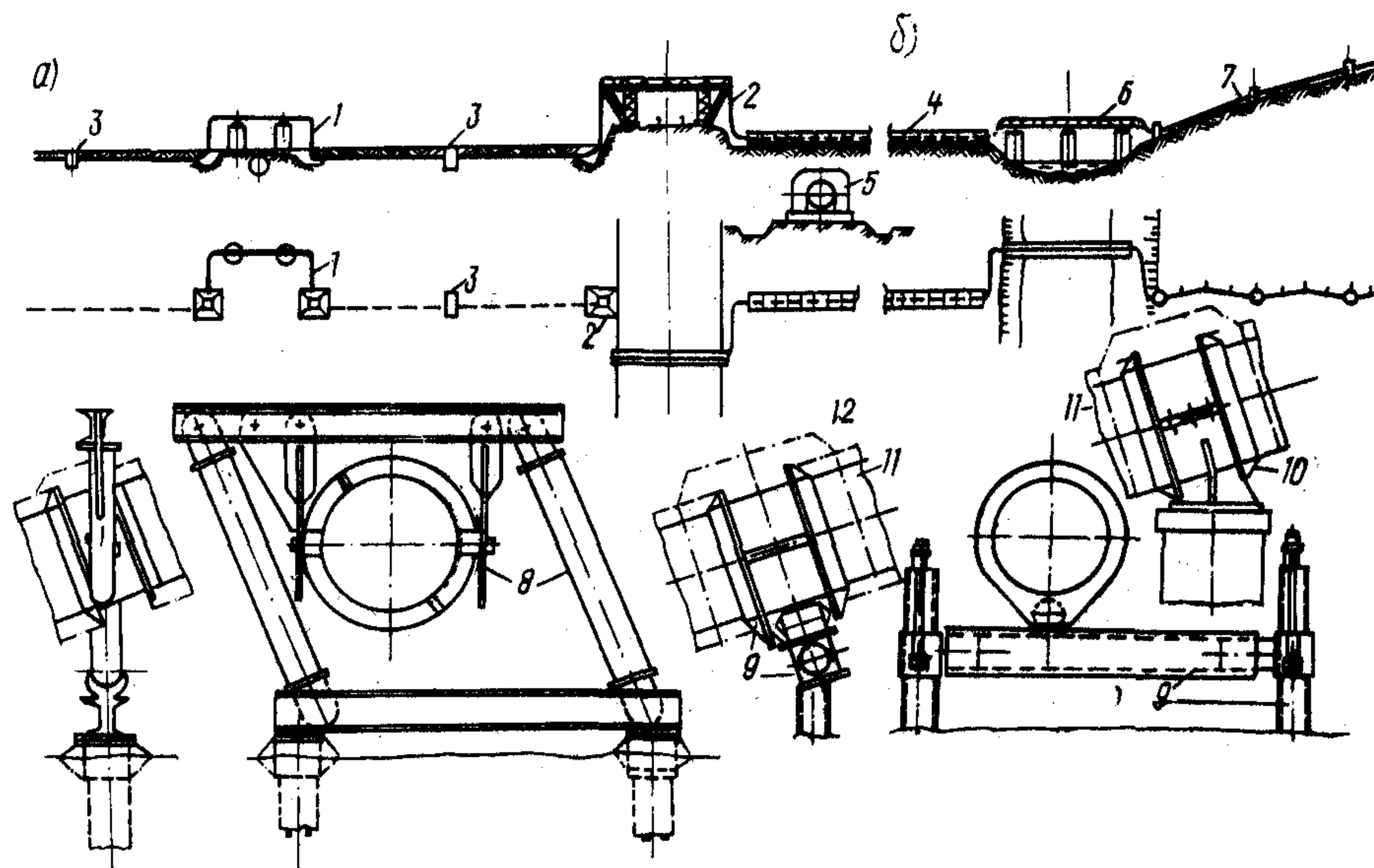
Рис.13. Схемы узлов подземного и надземного способов прокладки трубопровода СПГ:
