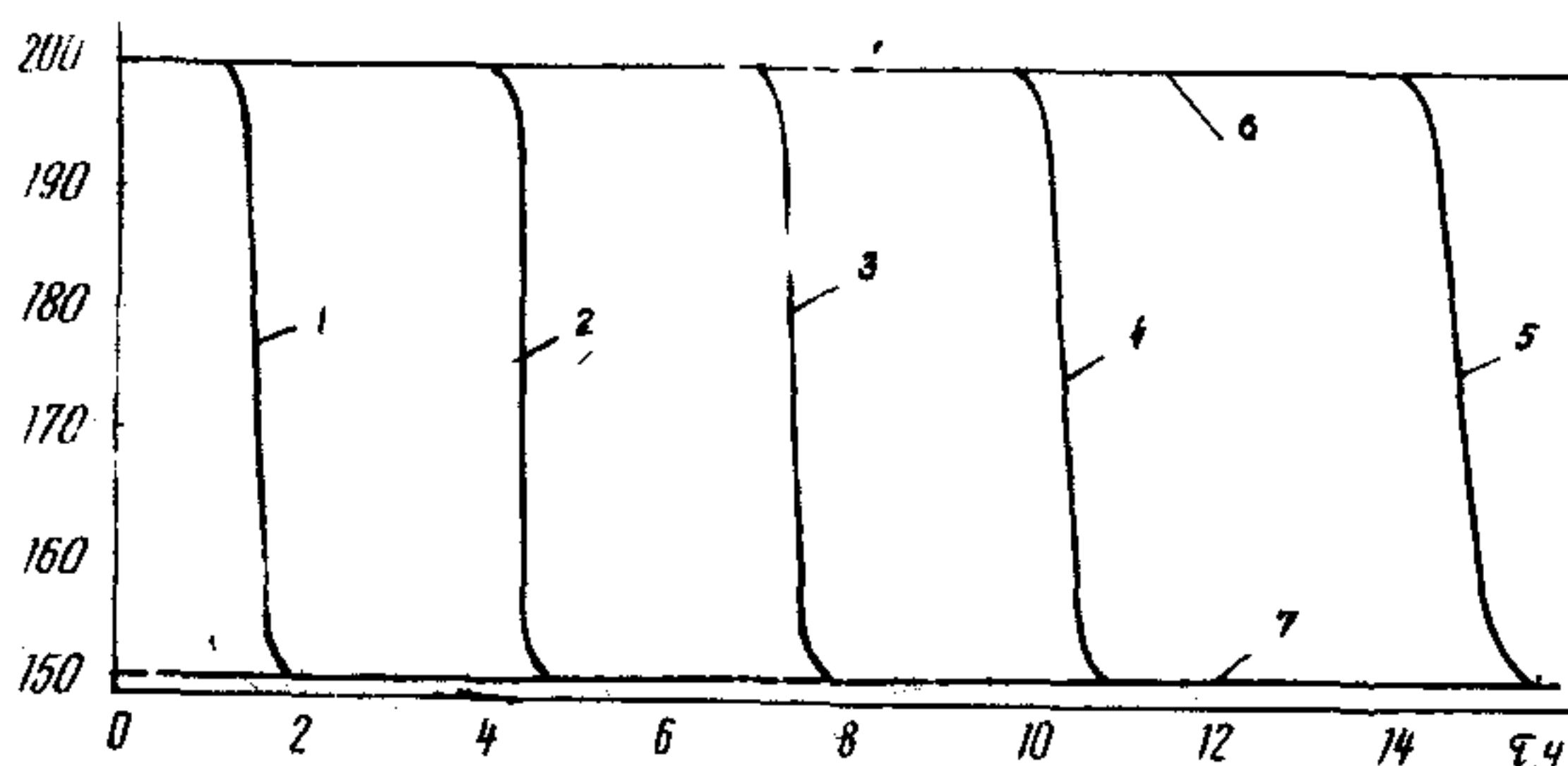
Рис. 3. Изменение температуры стенки трубопровода диаметром 1420 мм во времени при захолаживании его от 200 К до 150 К сжиженным природным газом (второй этап захолаживания)
