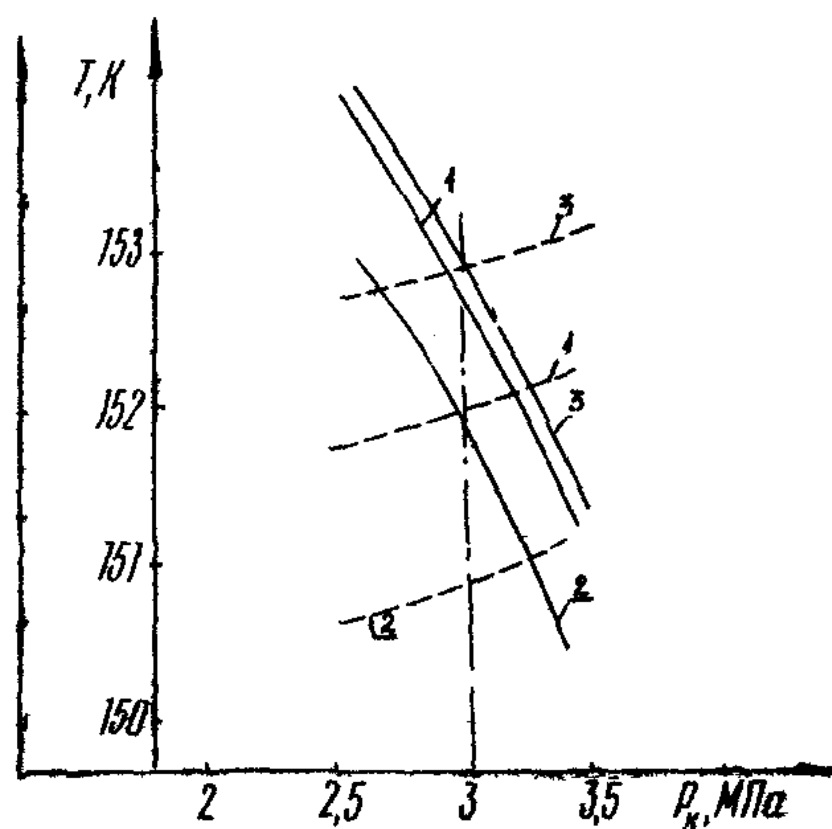
Рис.4. Зависимость производи- тельности трубопровода СПГ ( Q ) и температуры СПГ в конце участка от конечного давления P_k = 2,942 МПа; P_H = 5,393 МПа; T_{H2} = 150 К; K = 0,43 Вт/м 2 ·К
