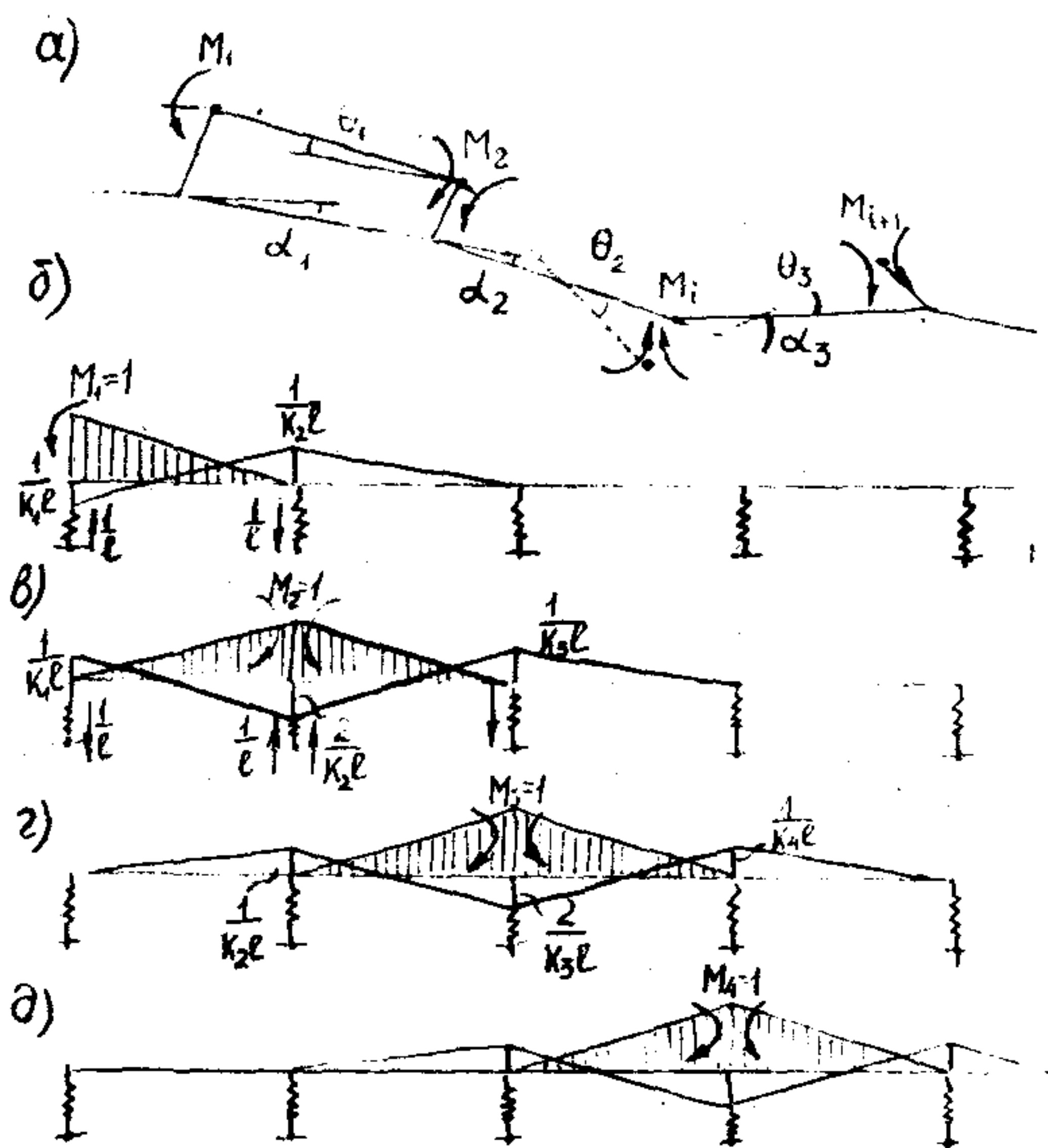
Рис.20. Основная система и единичные состояния расчета кинематической цепи на изгиб на разных этапах итерационного расчета:
