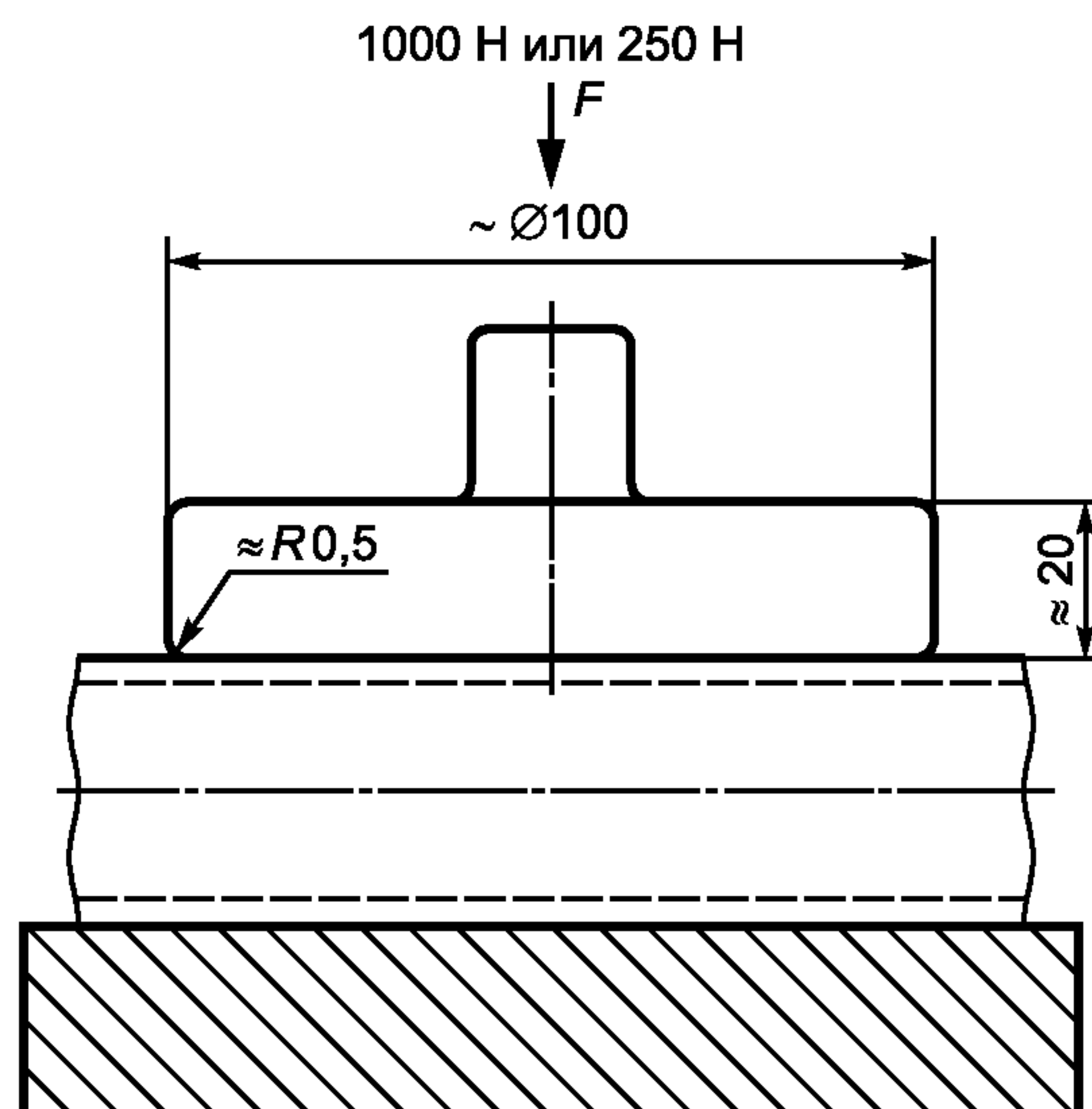
Рисунок 4 — Схема испытания на сплющивание шланга подачи воздуха
