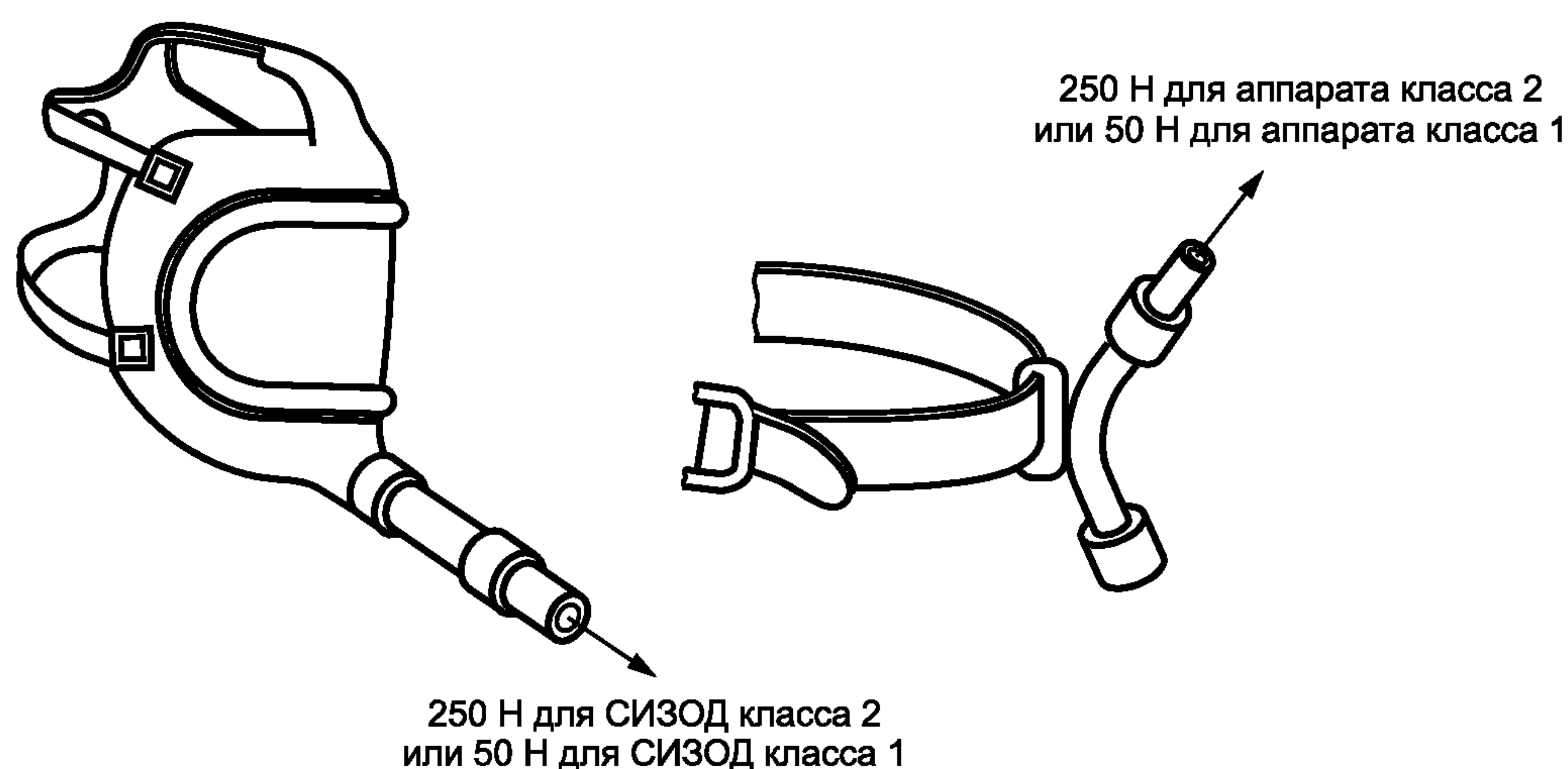
Рисунок 1 — Схема испытания прочности присоединения соединительного шланга
