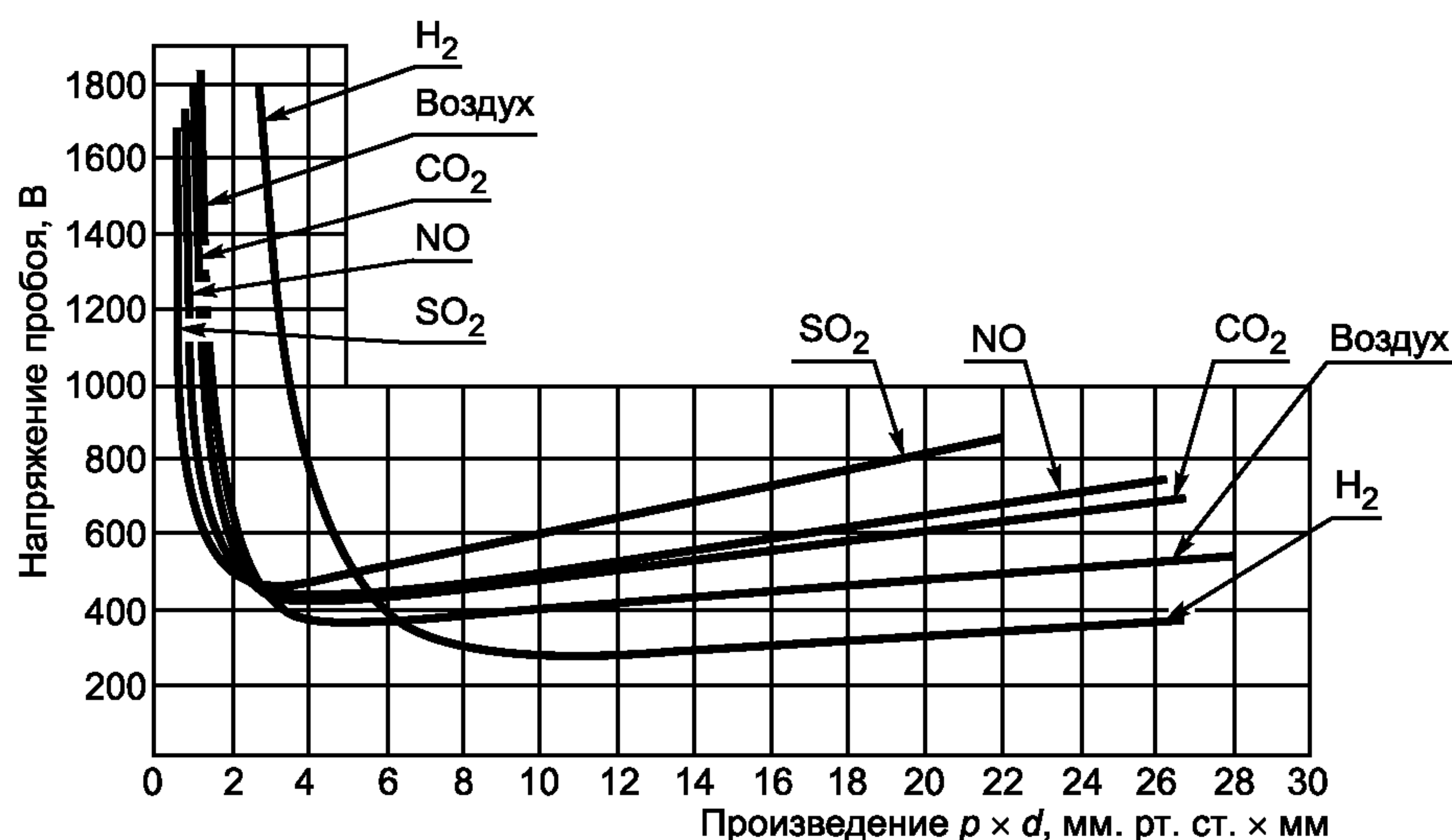
Рисунок 1 — Кривая Пашена
