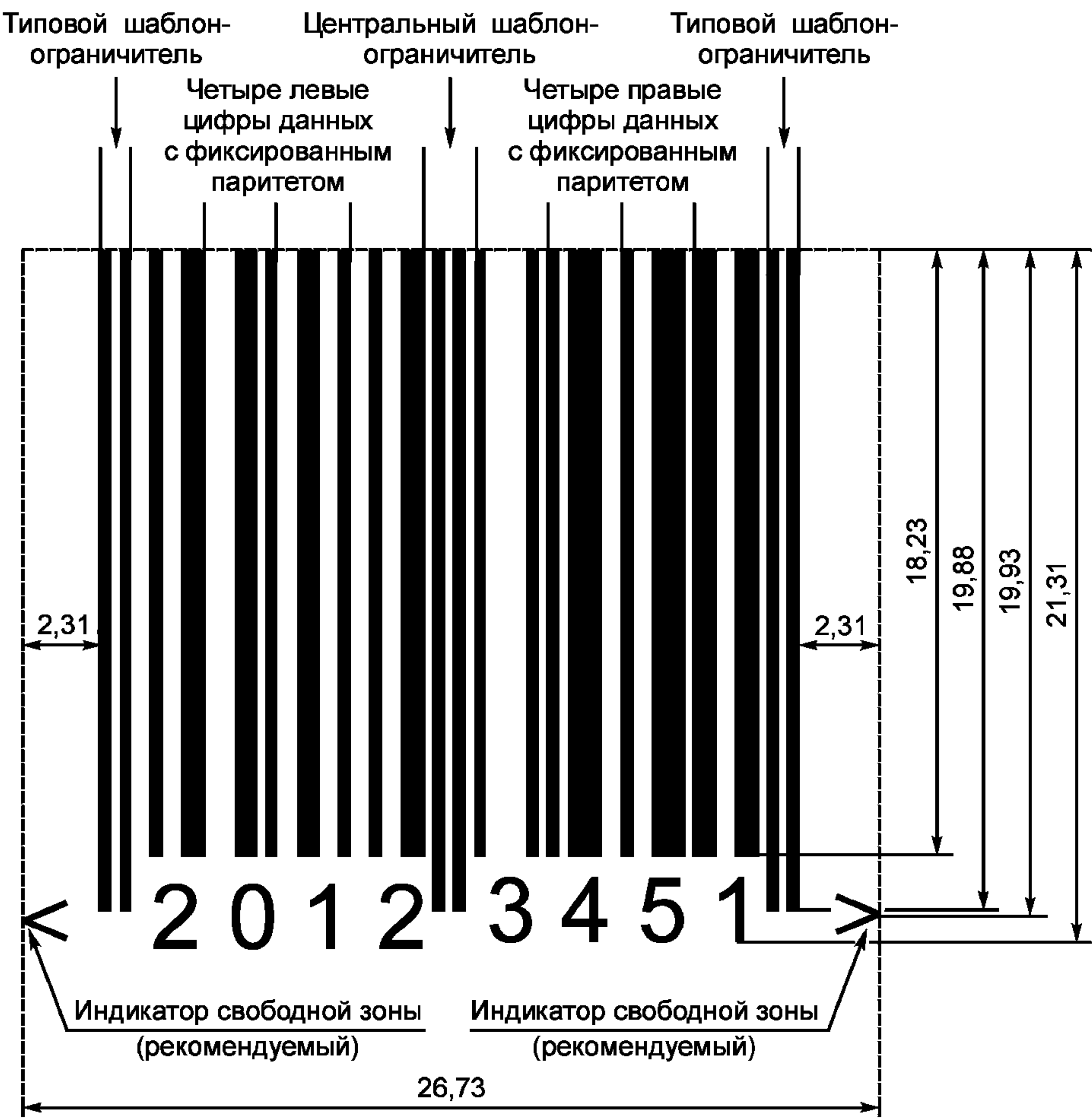
Рисунок Е.4 — Символ EAN-8
