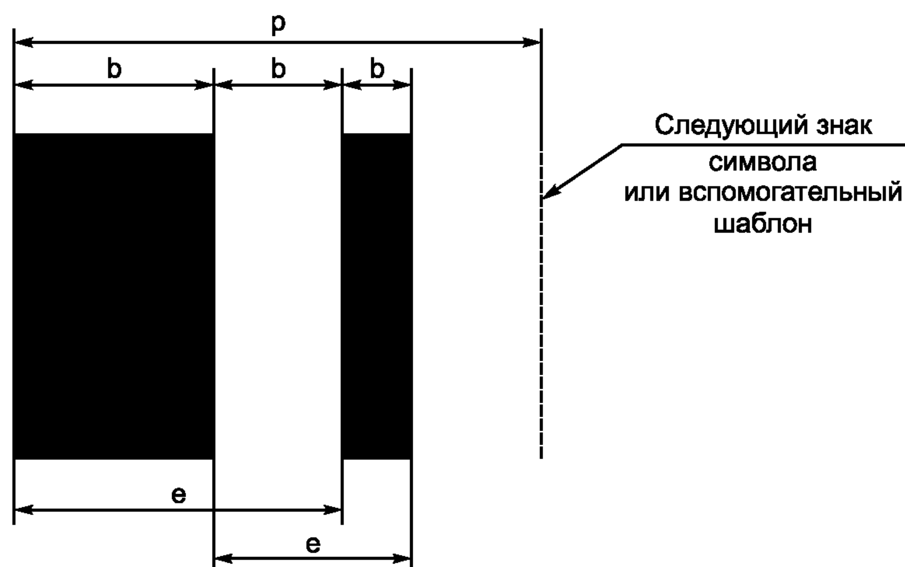
Рисунок F.1 — Размеры для определения допусков
