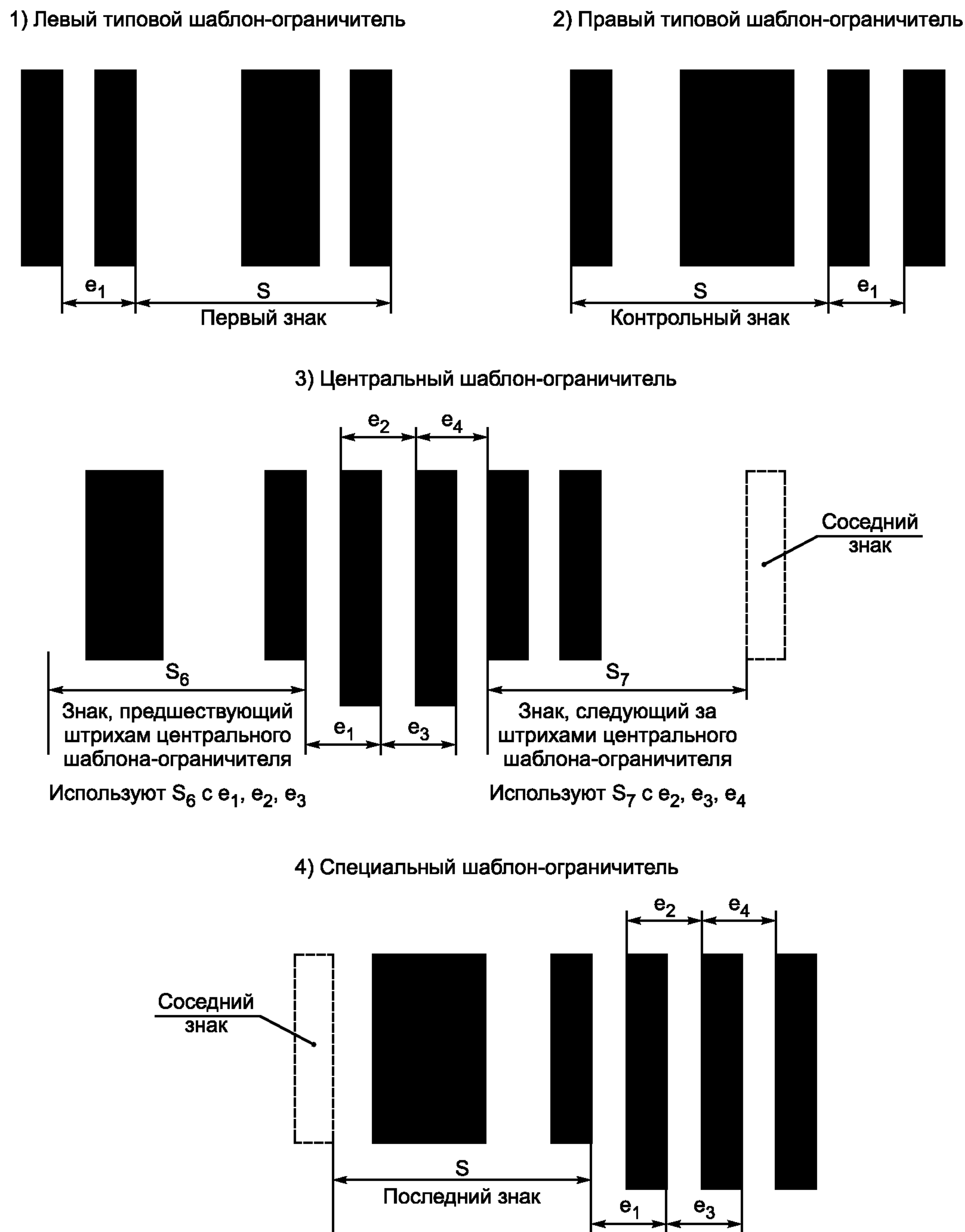
Рисунок 8 — Размеры вспомогательных шаблонов
