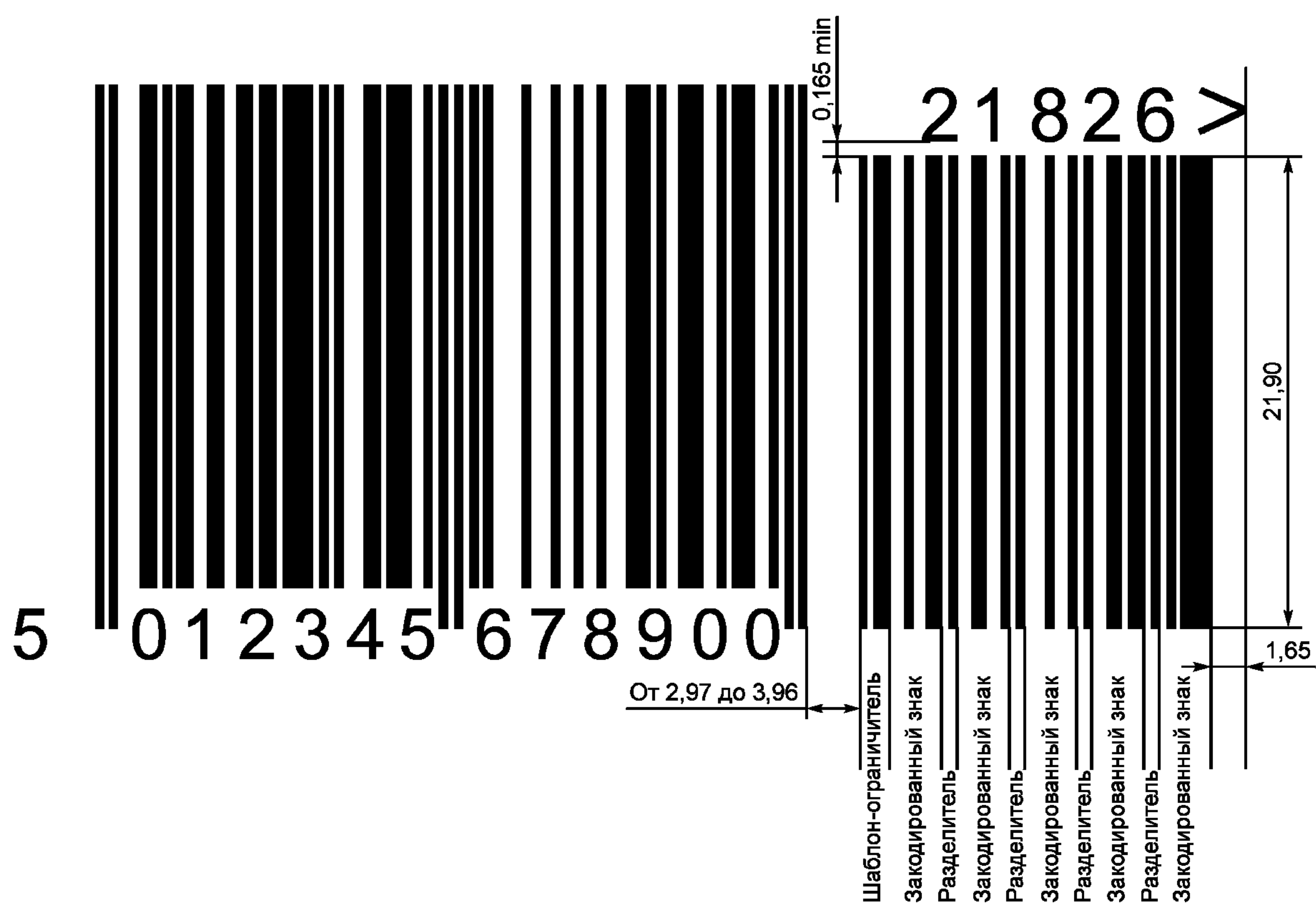
Рисунок Е.7 — Символ EAN-13 с 5-разрядным дополнительным символом
