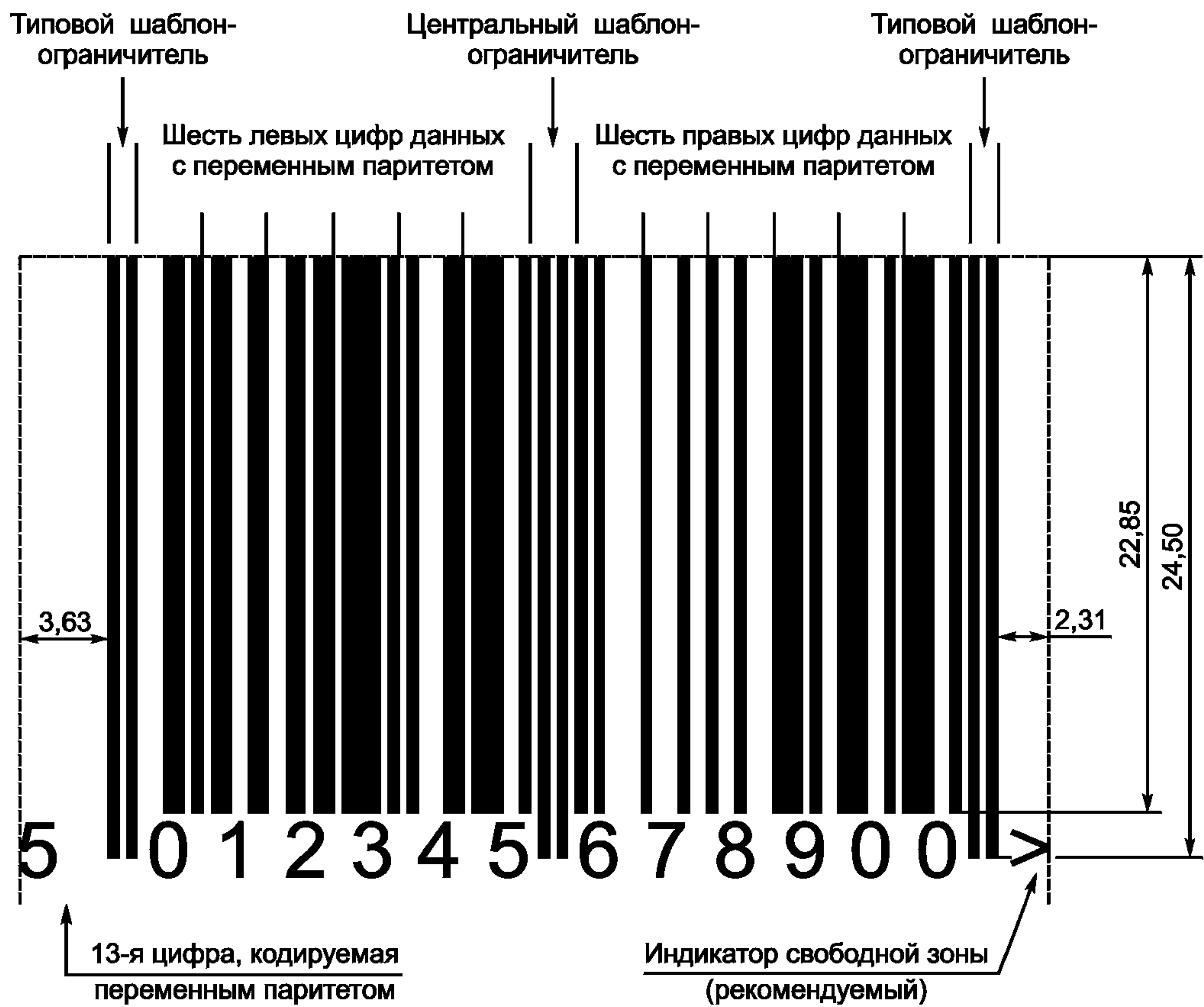
Рисунок Е.1 — Символ EAN-13
