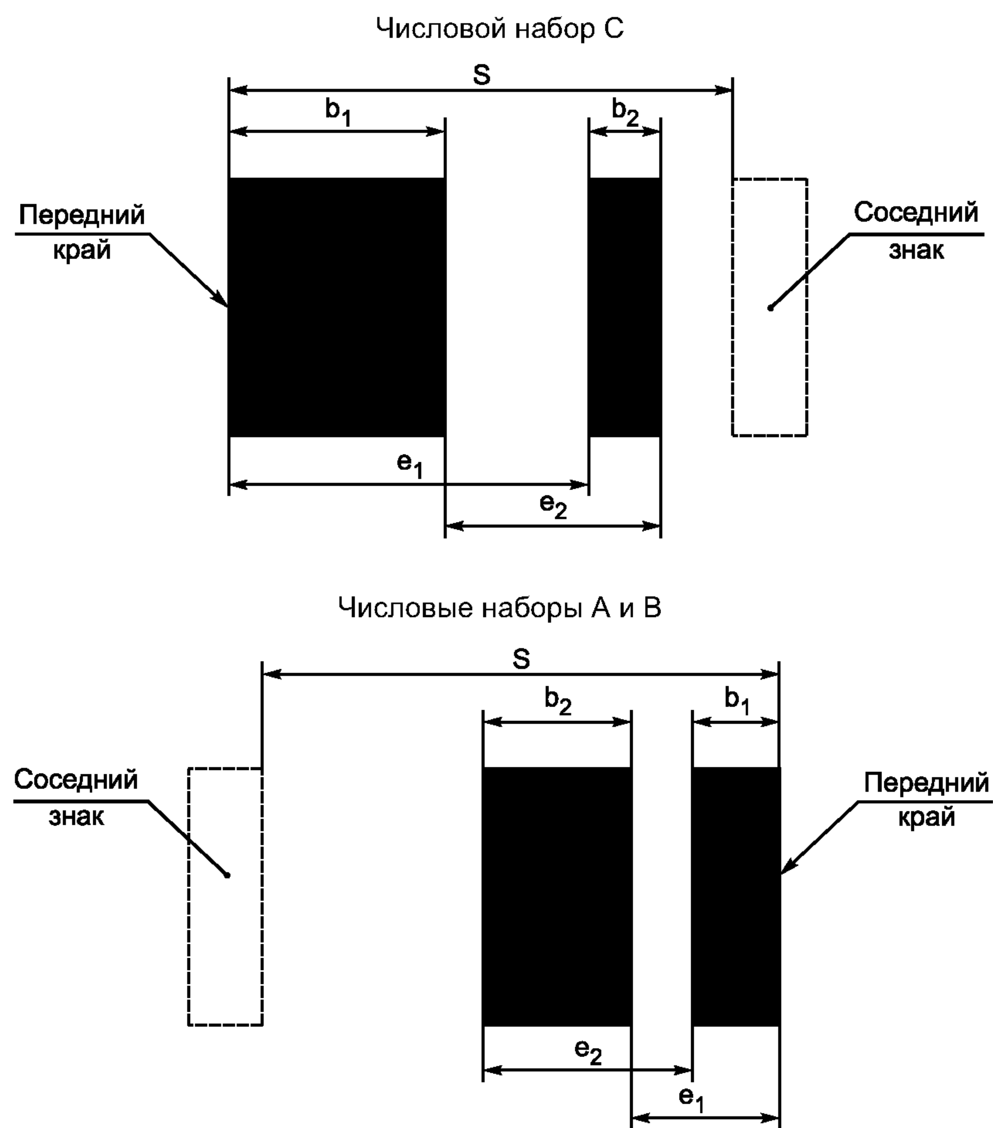
Рисунок 7 — Размеры для декодирования знаков символов
