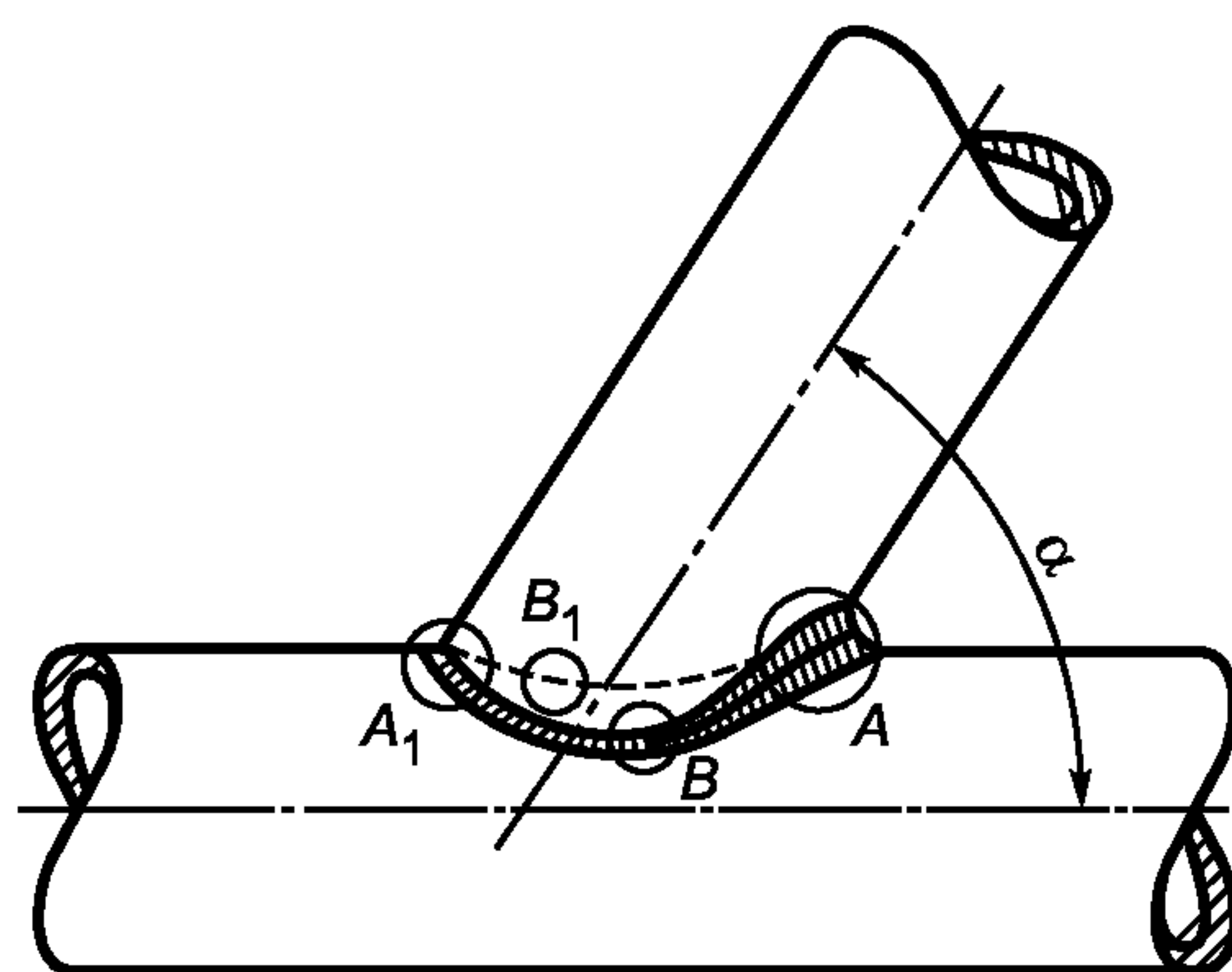
Рисунок 7 — Вырезка образцов для испытаний из таврового соединения
