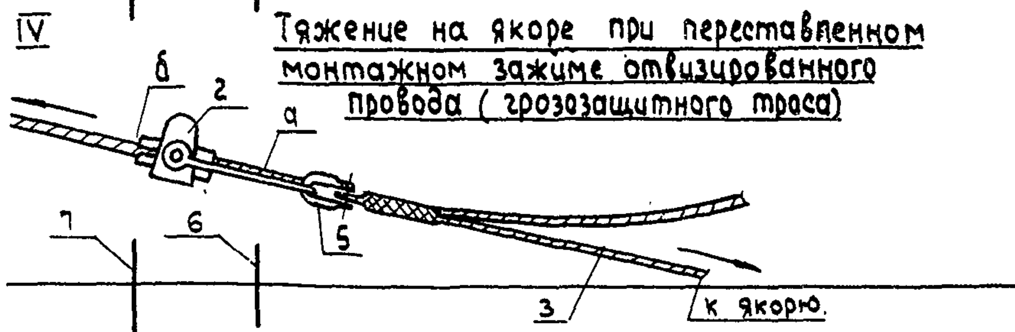
Рис.21. Передача тяжения отвизированного провода (грозозащитного троса) от трактора на якорь.
