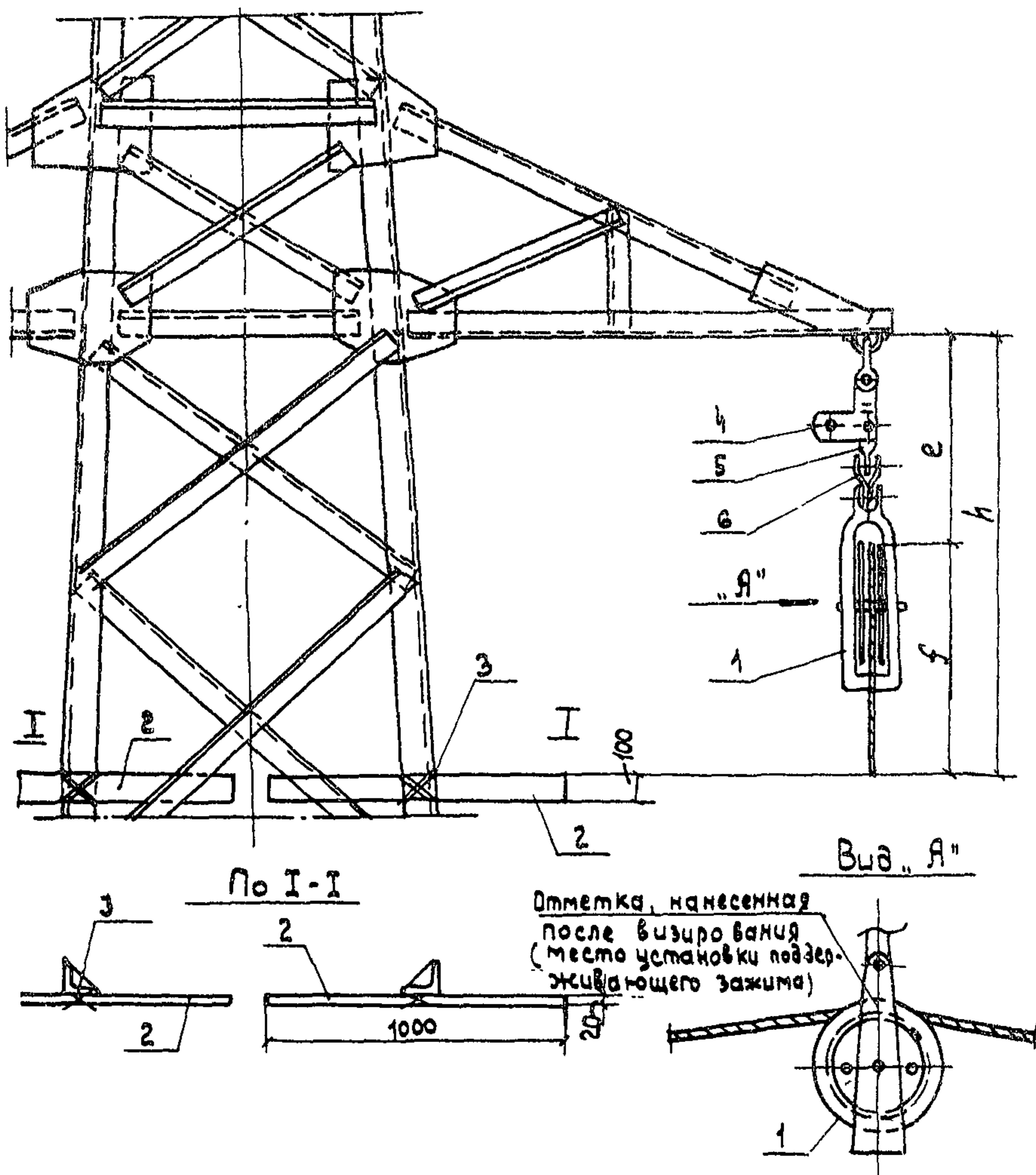
Рис. 4. Установка на опоре инвентарной визирной рейки при визировании провода.
