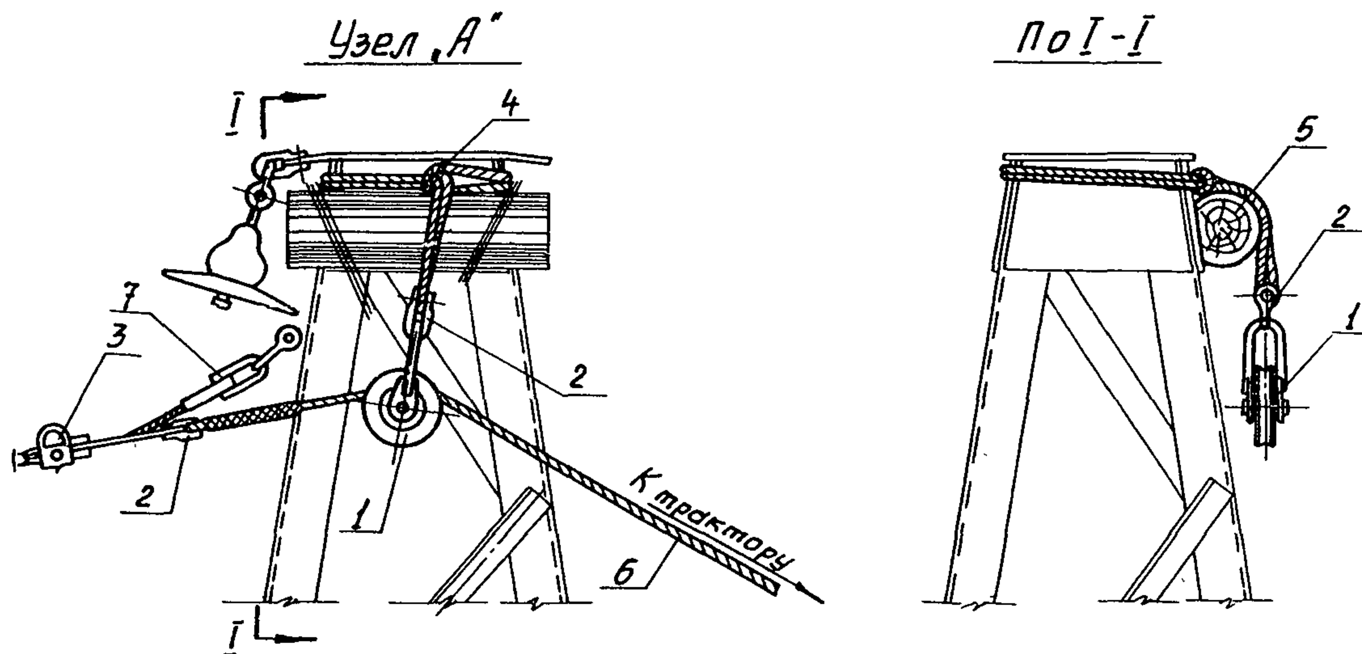
Рис. 14. Узел „А“ Подъем и крепление грозозащитного троса на анкерно-угловой опоре
