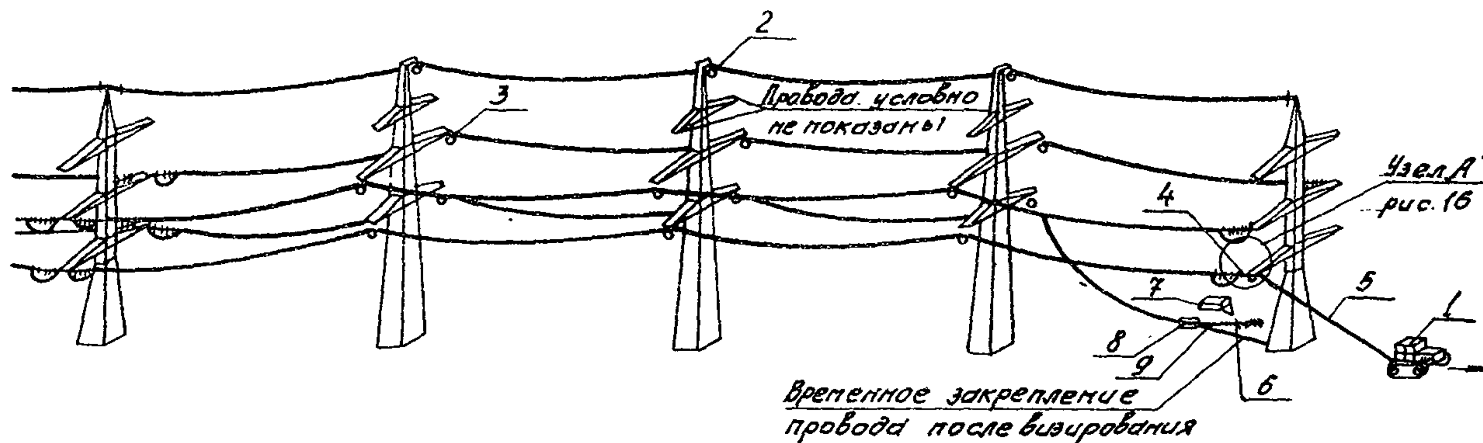
Рис. 15. Подъем проводов на анкерно-целовую опору
