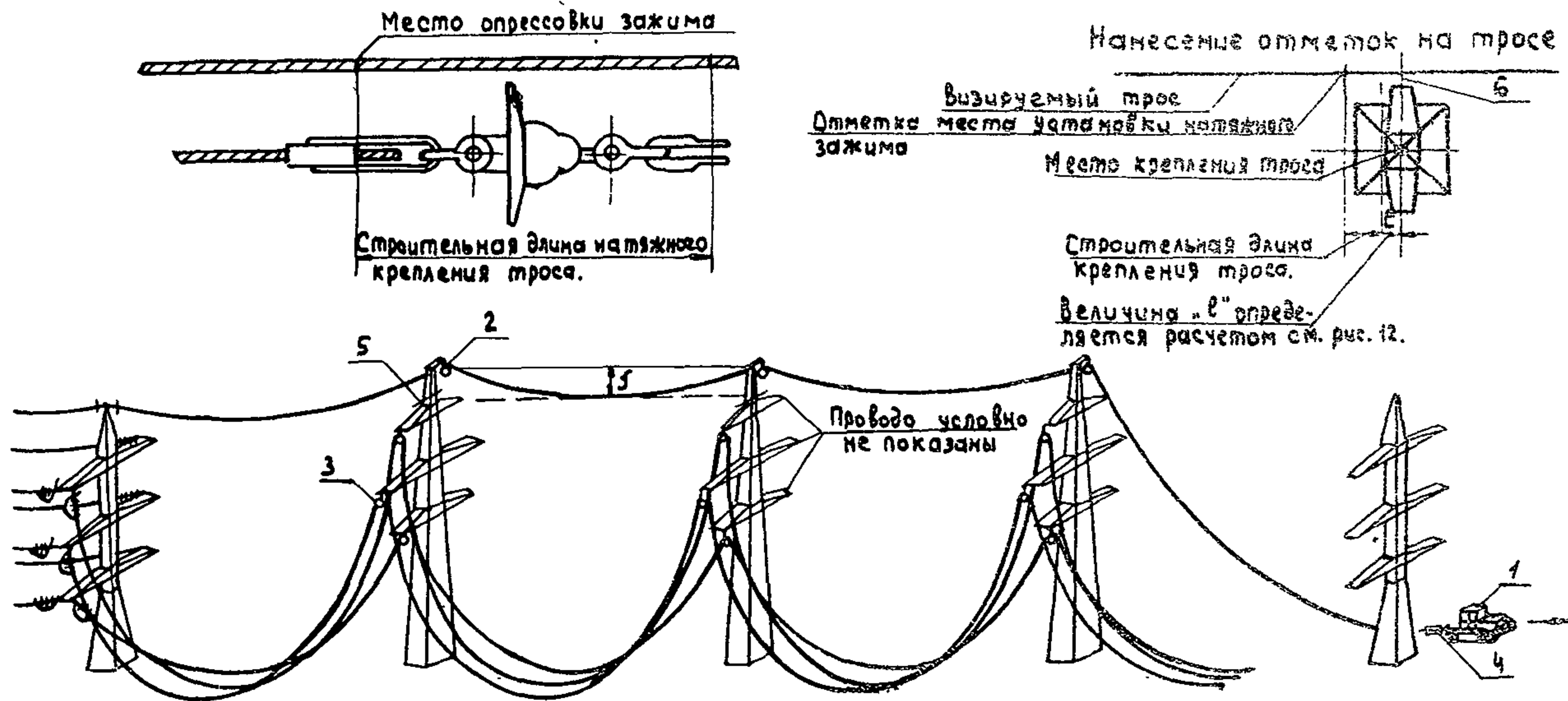
Рис. 5 Натягивание и визирование грозозащитного троса на участке ВА, ограниченном анкерно-угловыми опорами.
