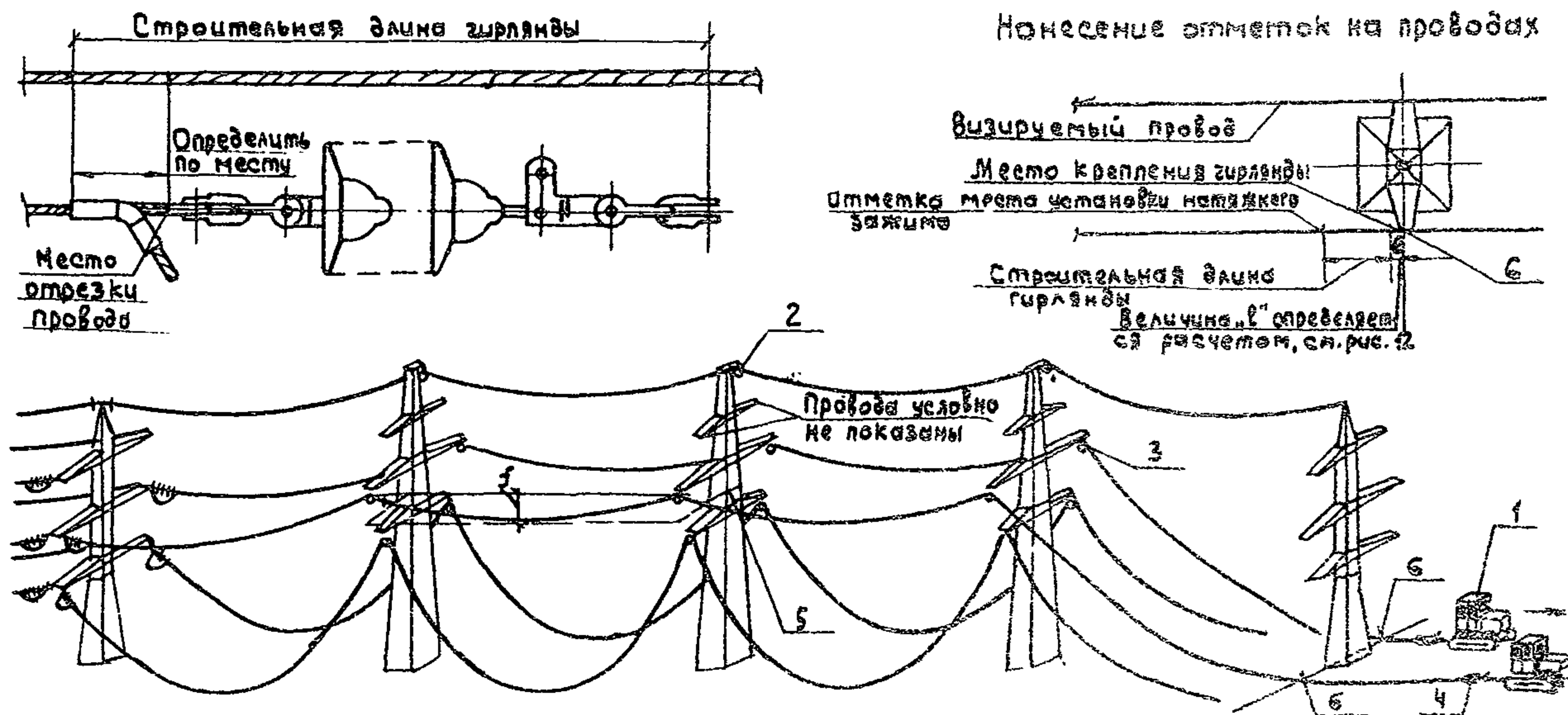
Рис. 6 Натягивание и визирирование проводов на участке 3л, ограниченном анкерно-угловыми опорами.
