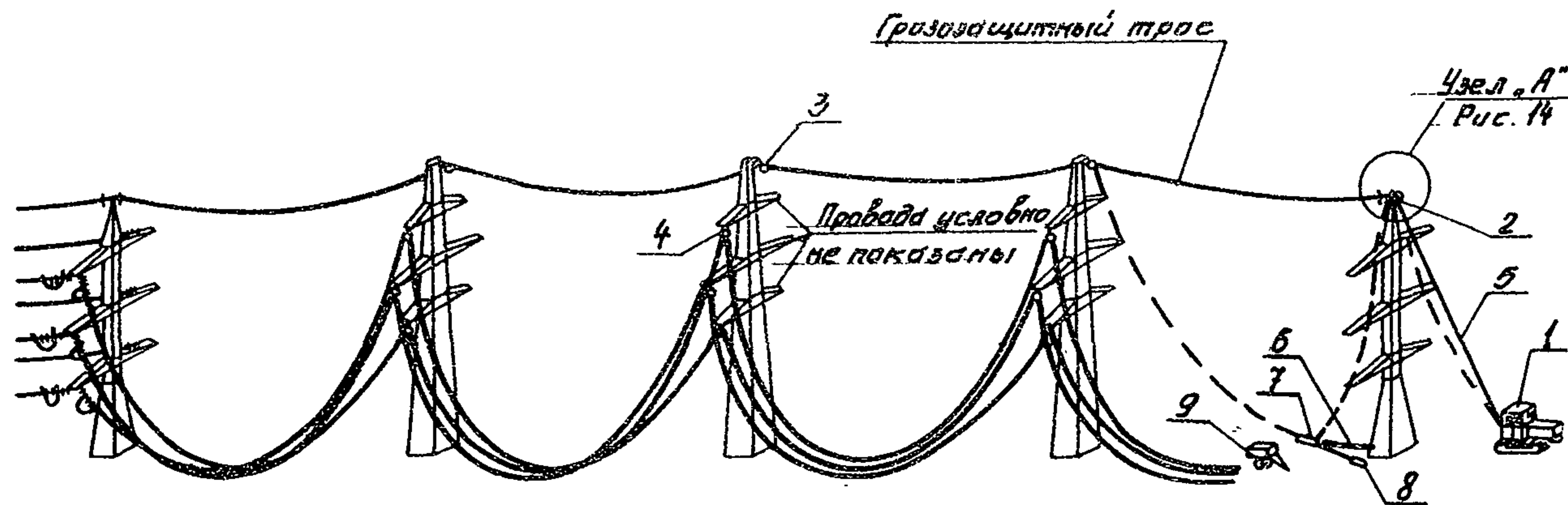
Рис. 13 Подъем и закрепление грозозащитного троса на анкерно-угловую опору
