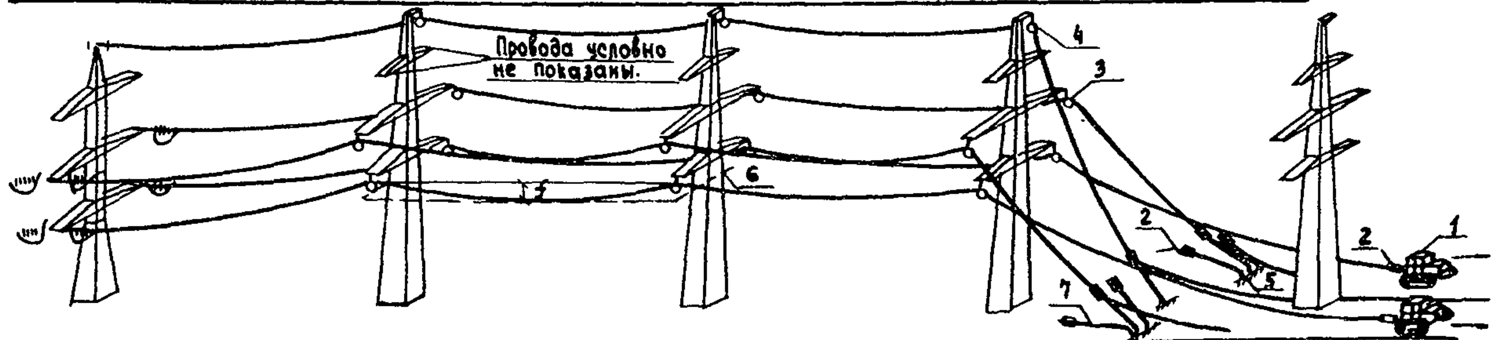
Рис.20 Натягивание, визирование и закрепление проводов на участке ВЛ, ограниченном анкерно-угловой и промежуточной опорами.
