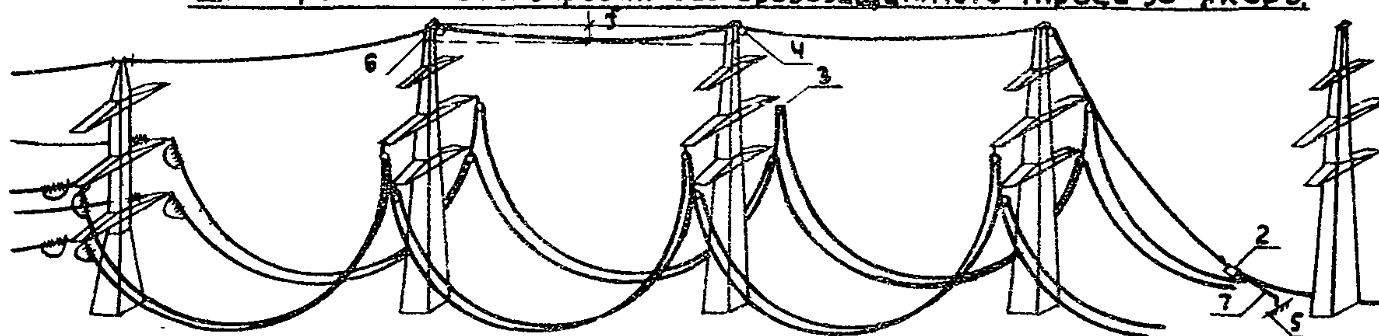
Рис. 19 Натягивание, визирование и закрепление грозозащитного троса на участке ВЛ. ограниченном анкерно-угловой и промежуточной опорами.
