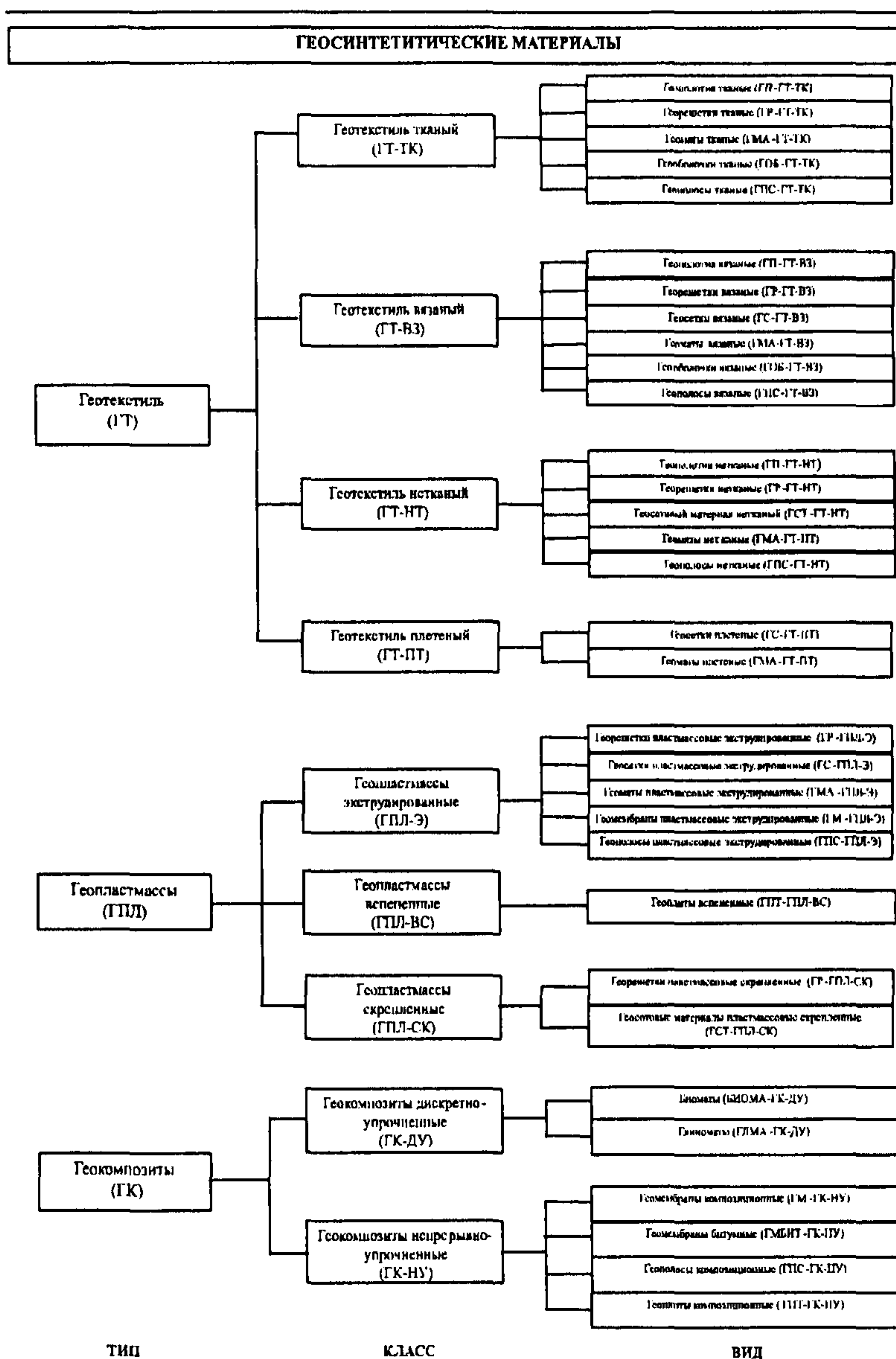
Рисунок 1 – Общая классификация геосинтетических материалов
