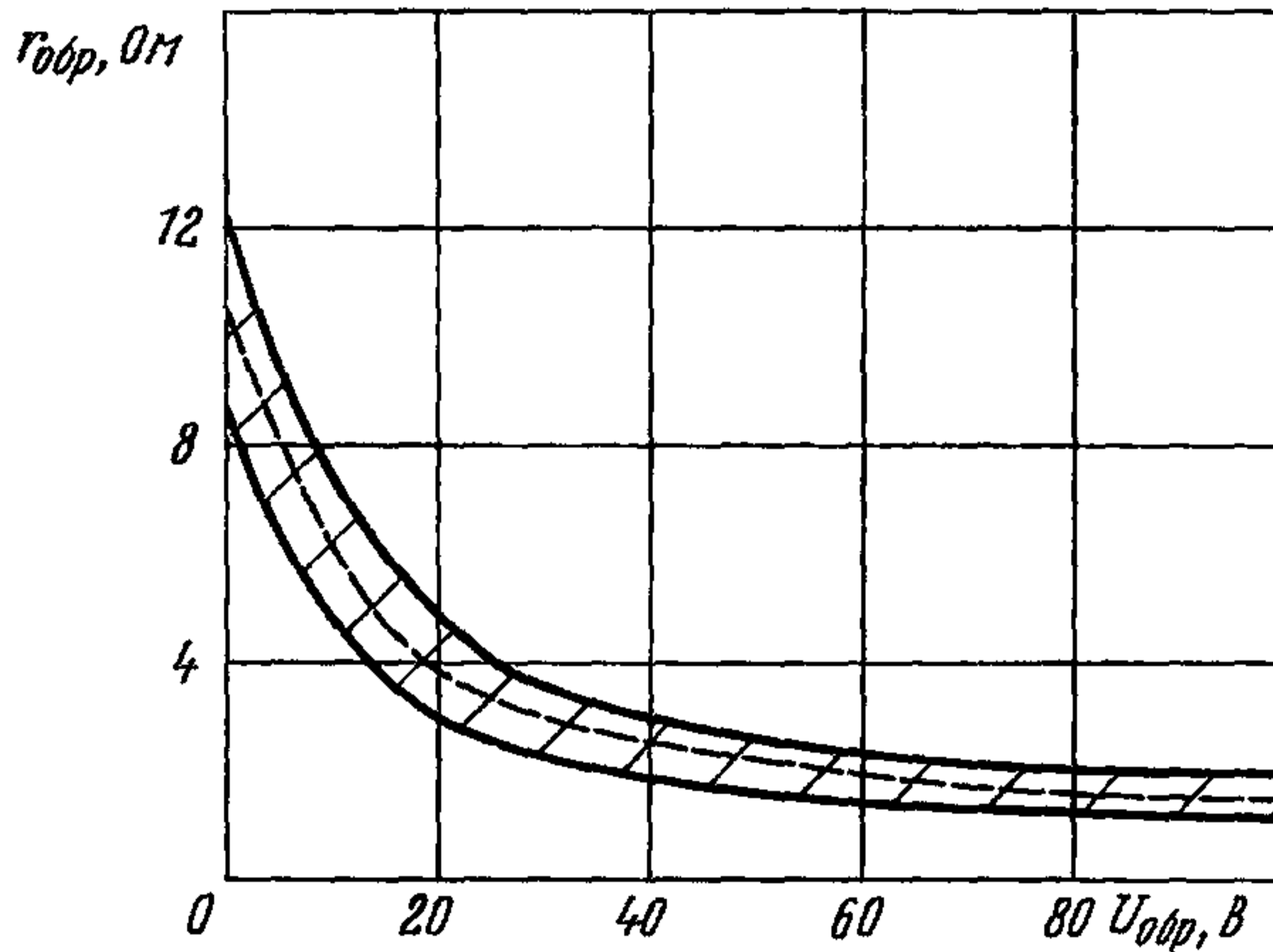
Область изменения обратного сопротивления потерь в зависимости от обратного напряжения
