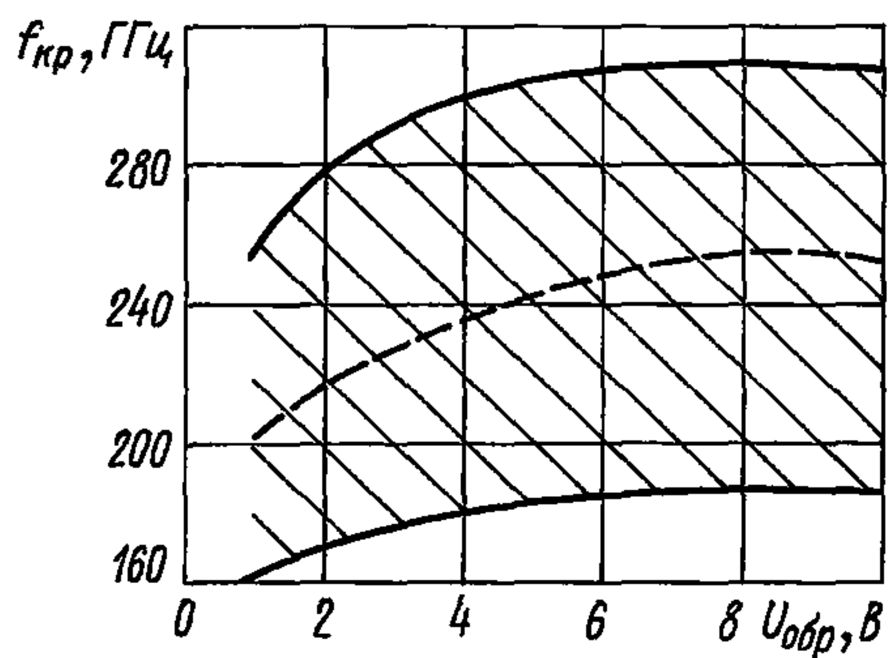
Область изменения критической частоты в зависимости от обратного напряжения смещения
