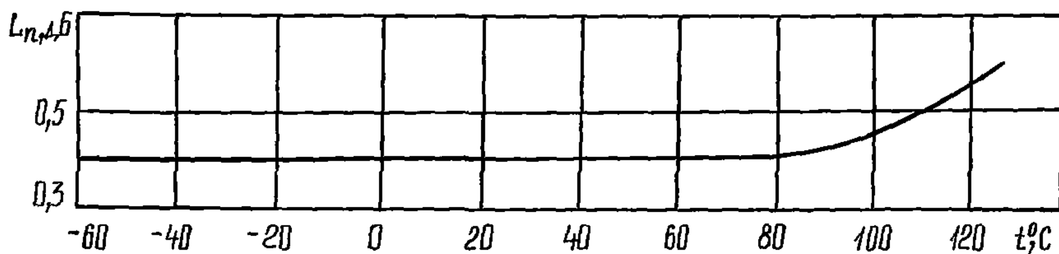
Характеристика потерь запирания в зависимости от температуры среды
