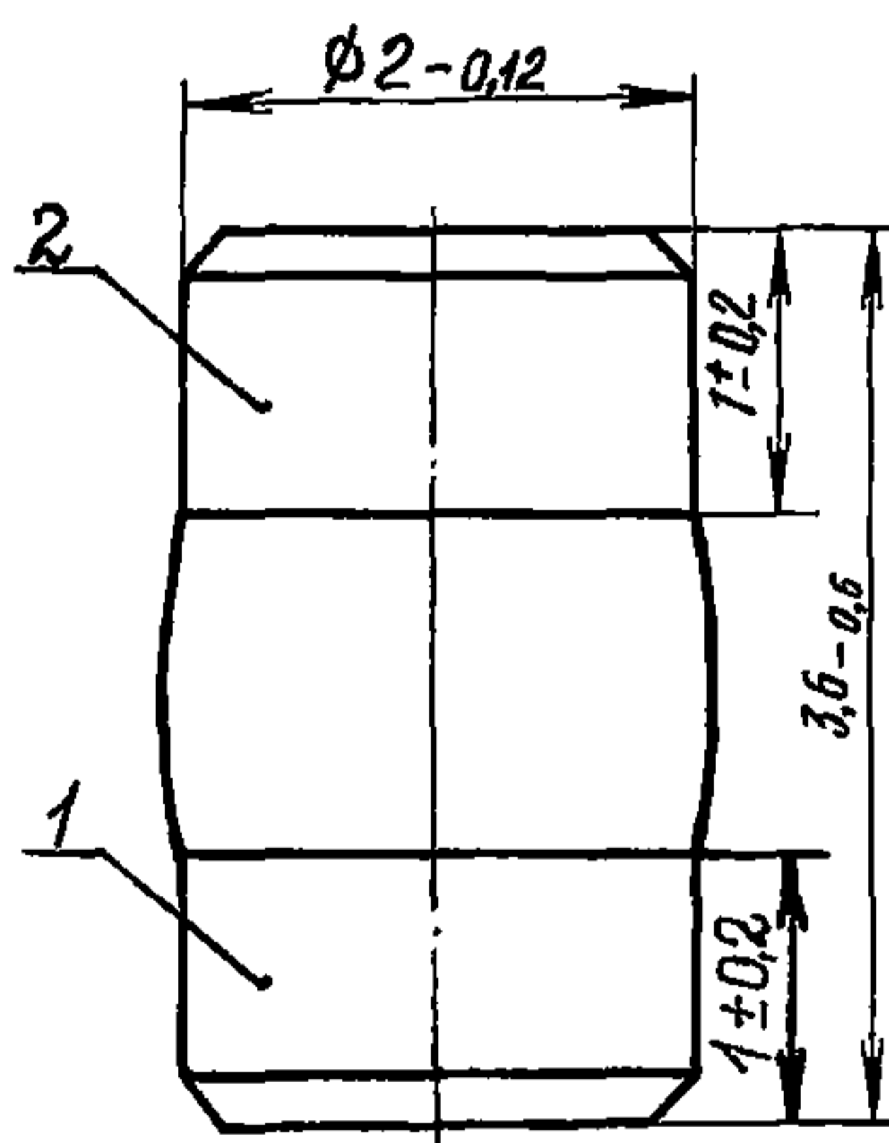
1 — вывод 1 «+»; 2 — вывод 2 «-»
