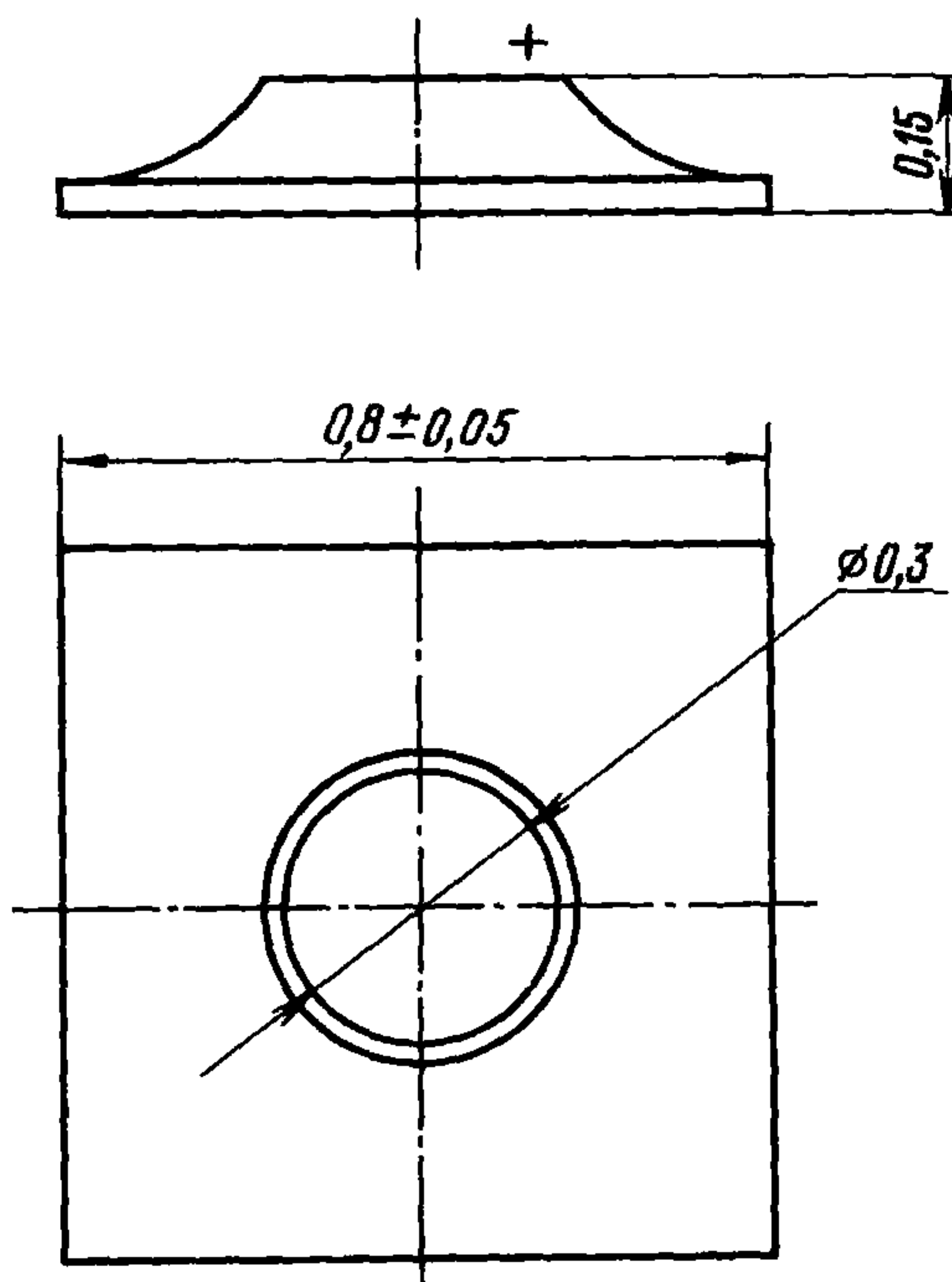
2A546A-5, 2A546Б-5
