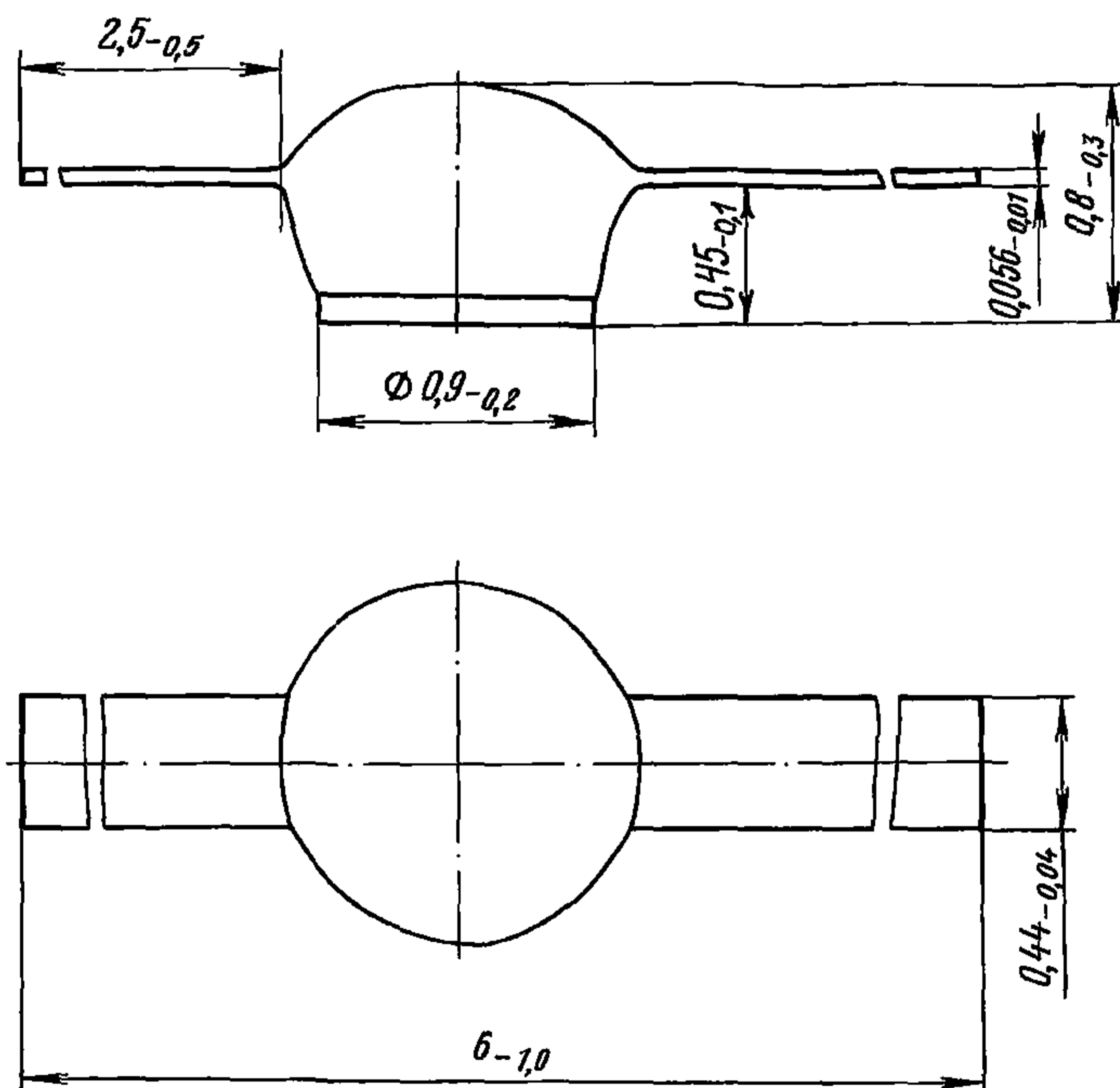
2A522A-2
