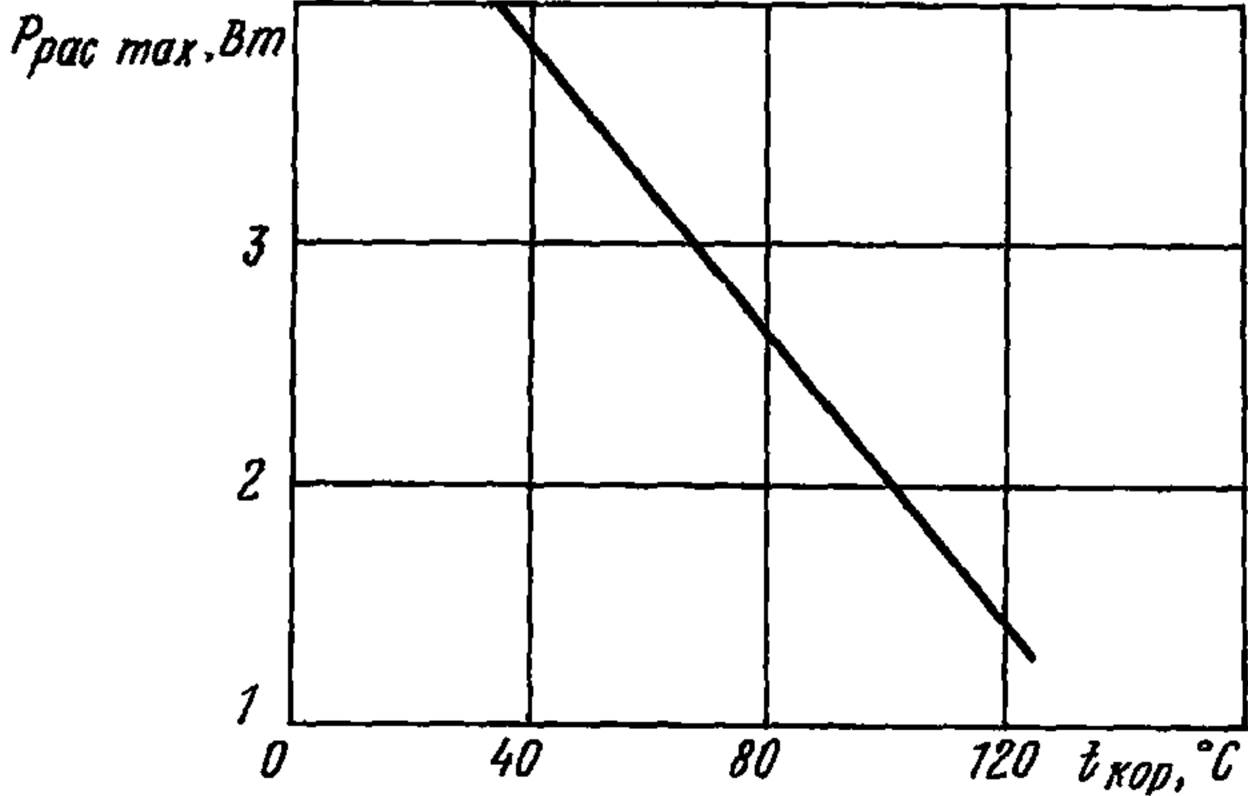
Характеристика максимально допустимой рассеиваемой мощности в зависимости от температуры корпуса
