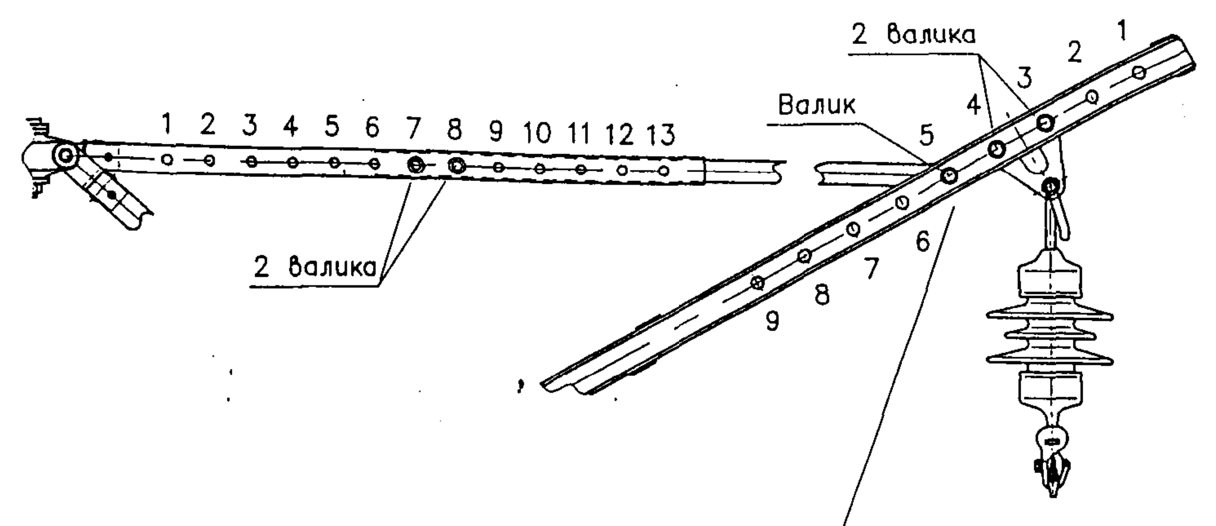
Нумерация отверстий кронштейна и тяги
