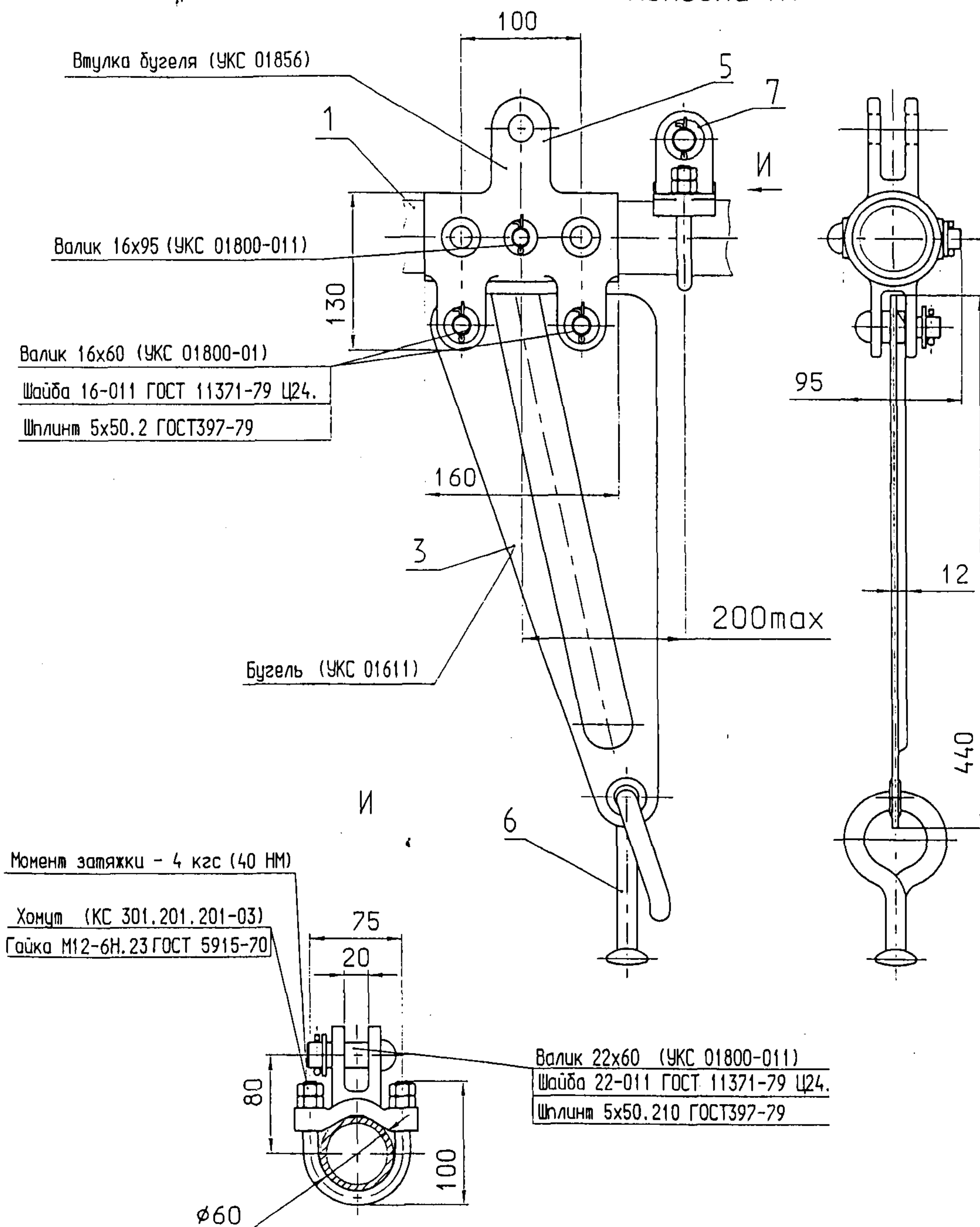
А (Листы 8, 9) Консоли НТ
