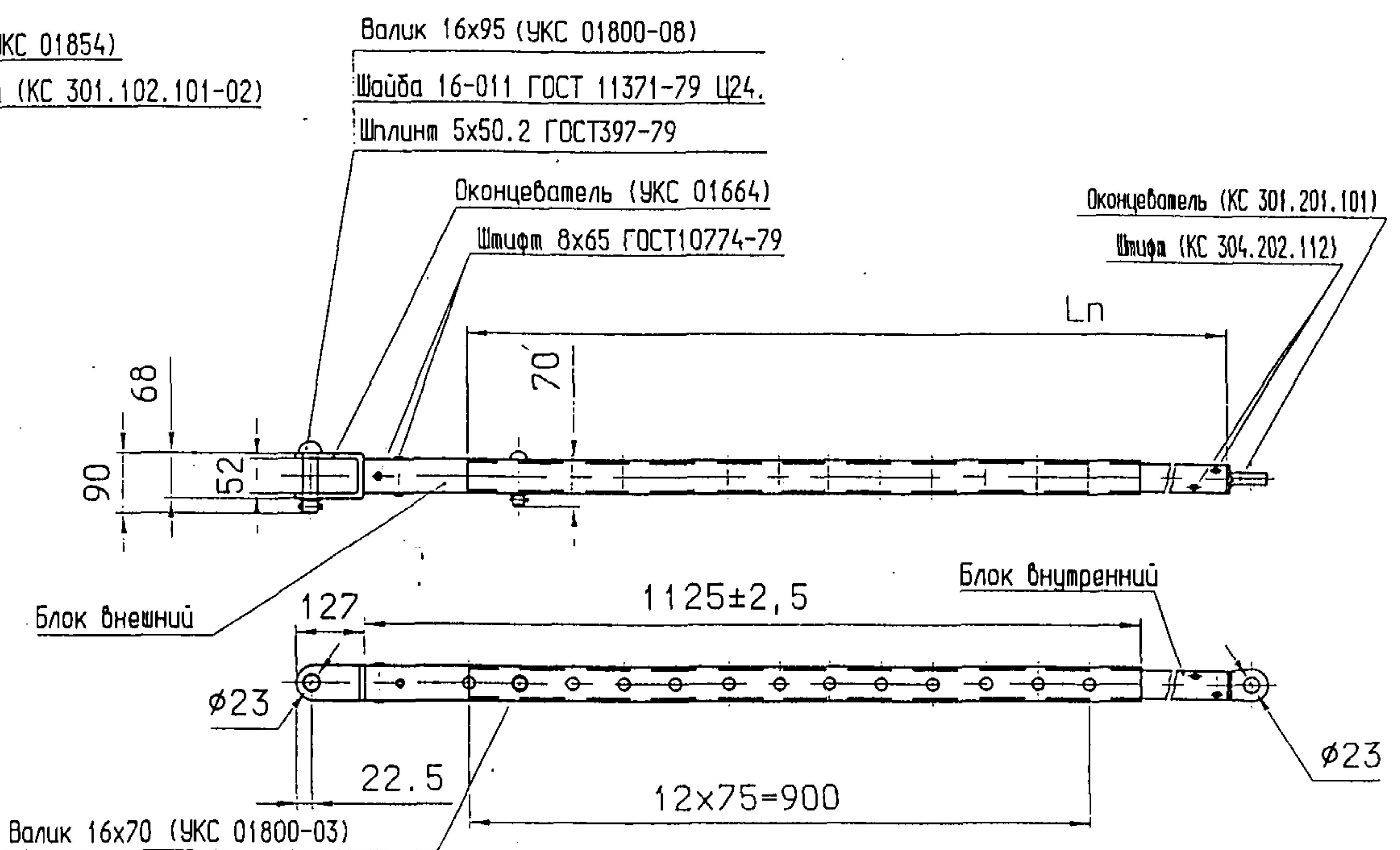
Переменное исполнение подкоса
