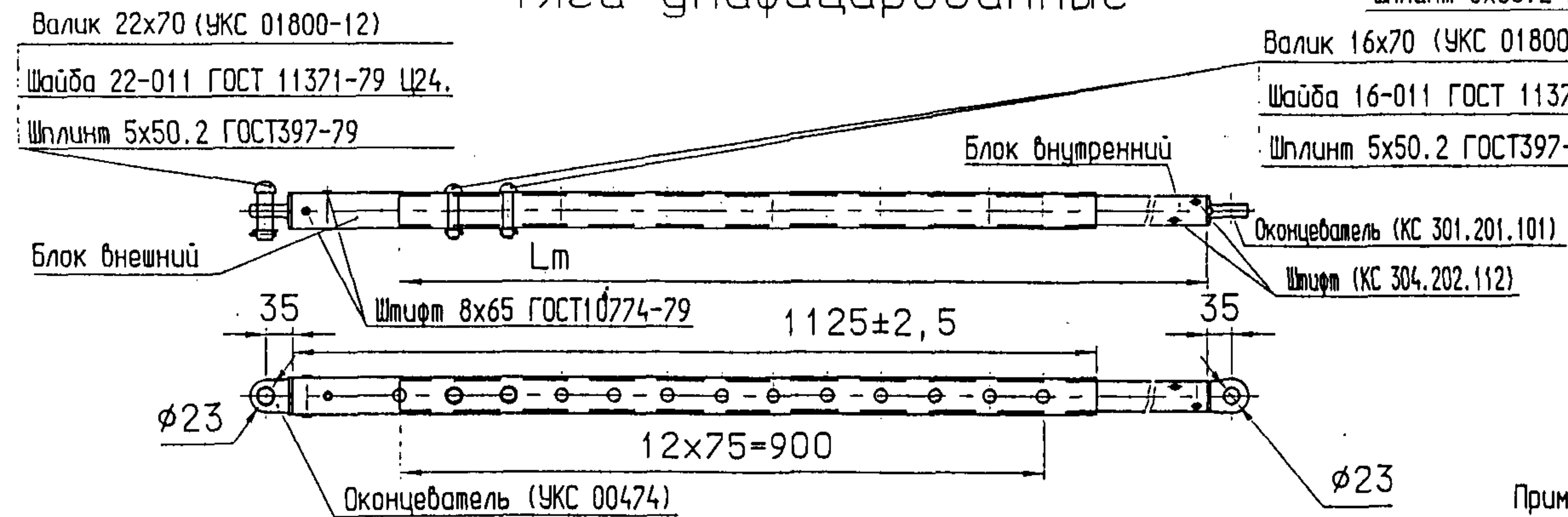
Переменное исполнение тяги унифицированной
