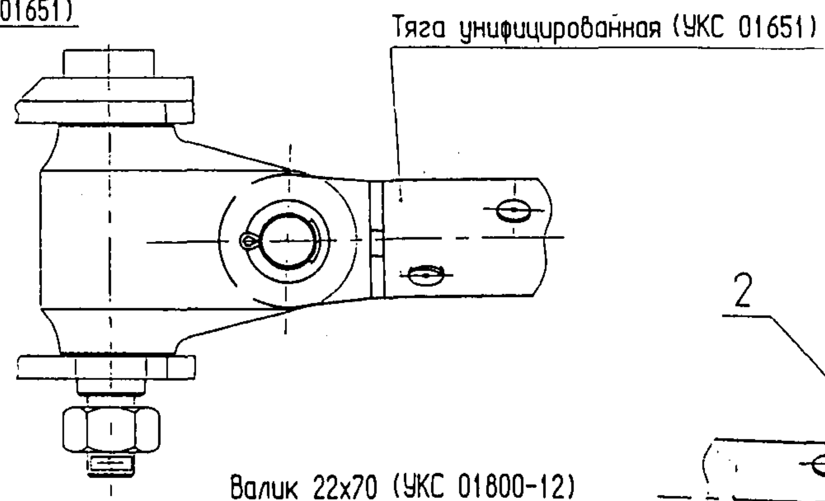
Г (Лист 15) консоль без подкоса
