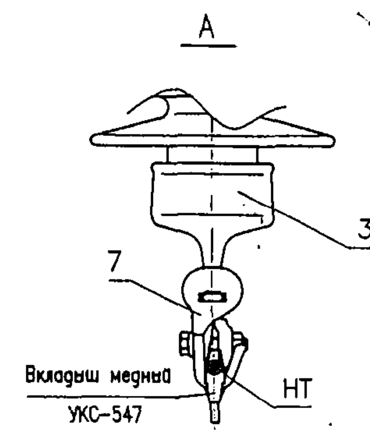
Вариант узла А с изолятором ПСФ 70-3,0/0.5-01 и седлом 008-1
