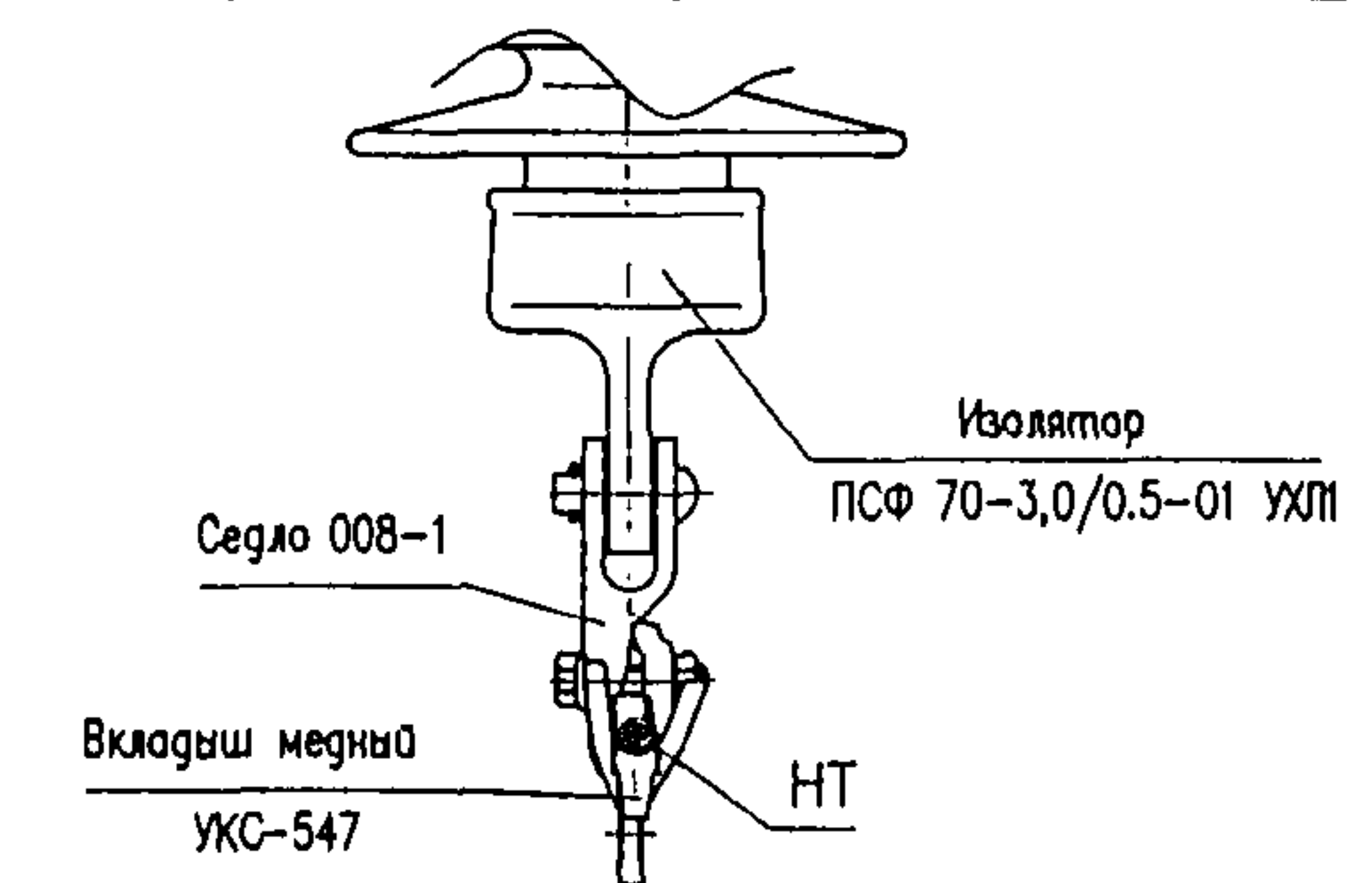
Вариант узла А с изолятором ПСФ 70-3,0/0.5-01 и седлом 008-1
