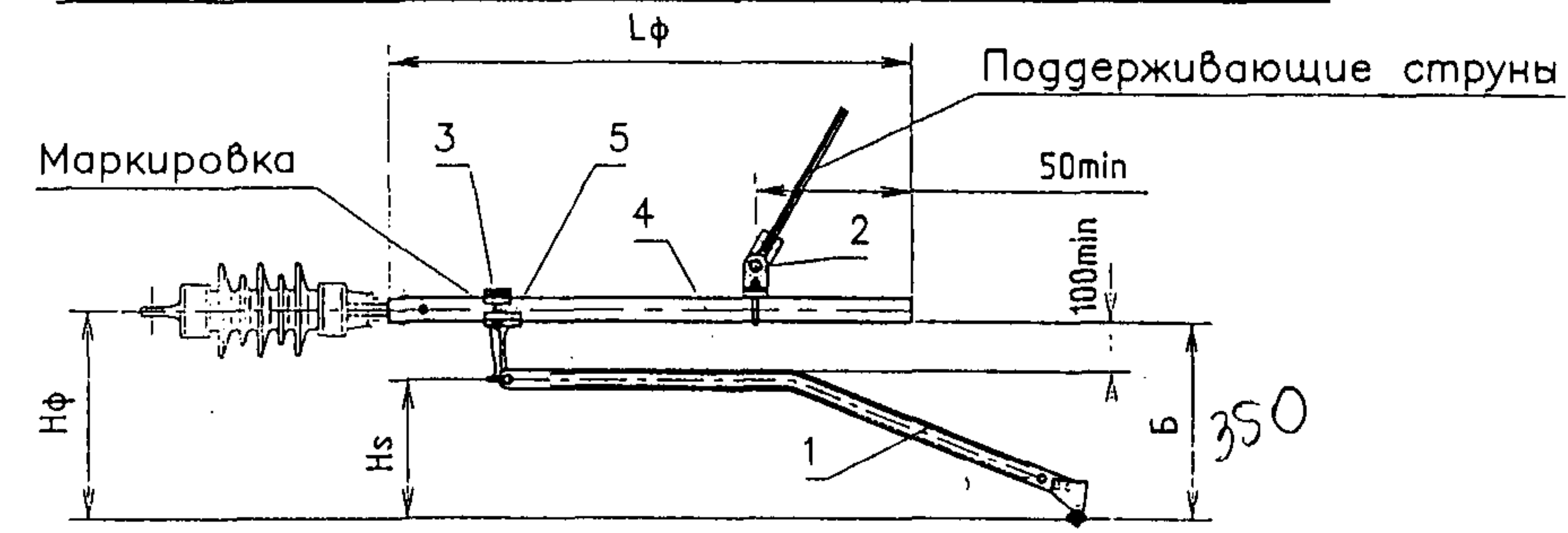
Расшифровка обозначений типов фиксаторов.
