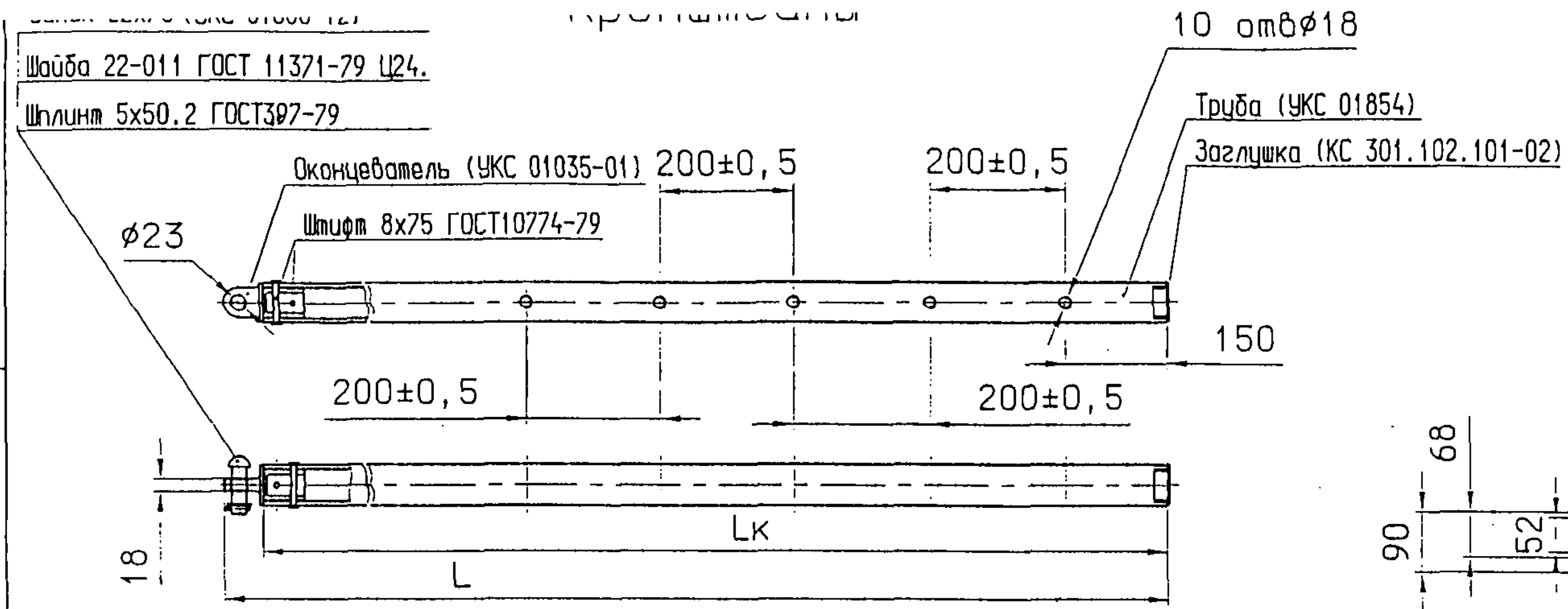
Переменные данные для исполнения конштейна
