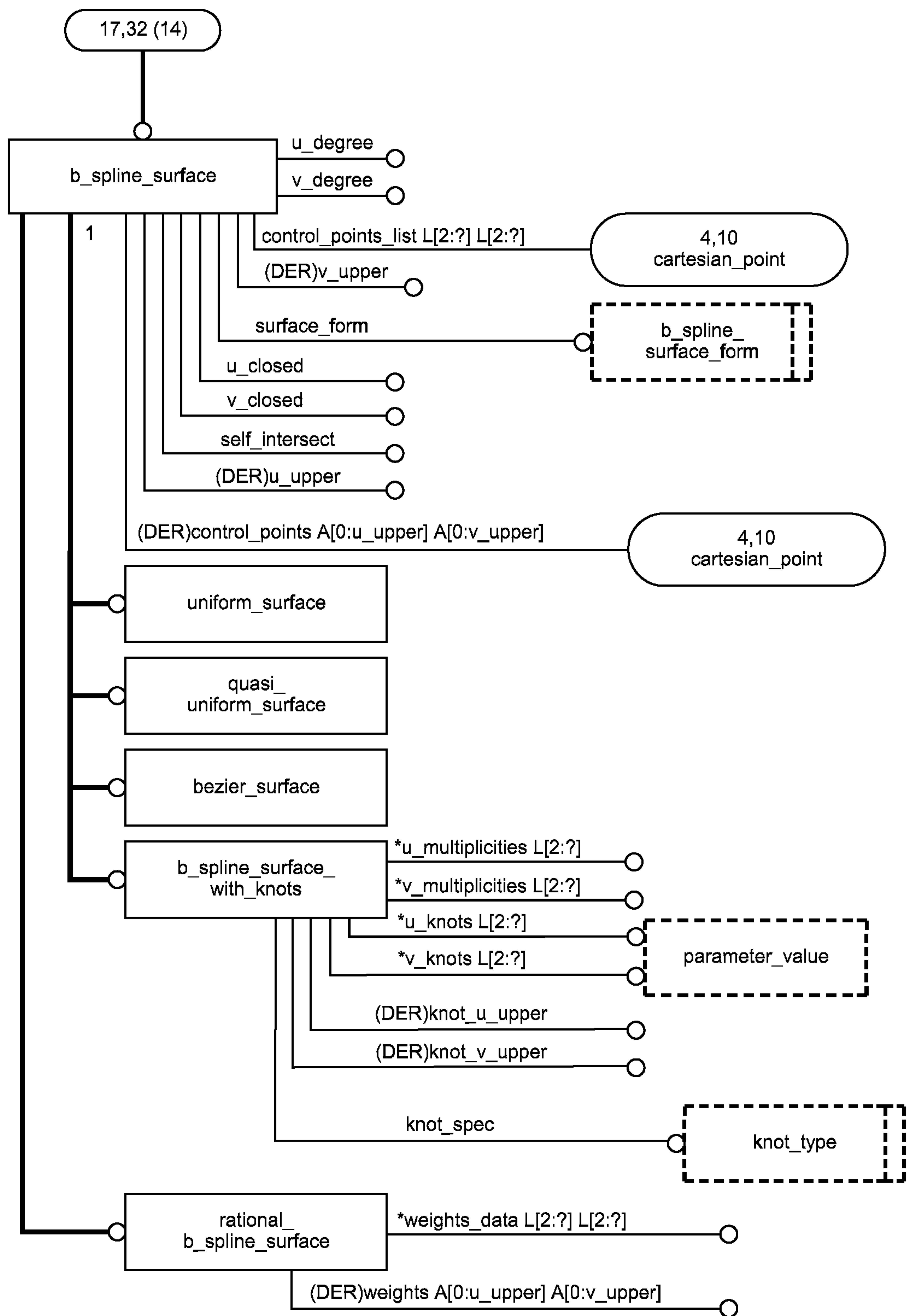
Рисунок С.17 — ПИК non_manifold_surface_shape_representation в формате EXPRESS-G (диаграмма 17 из 22)
