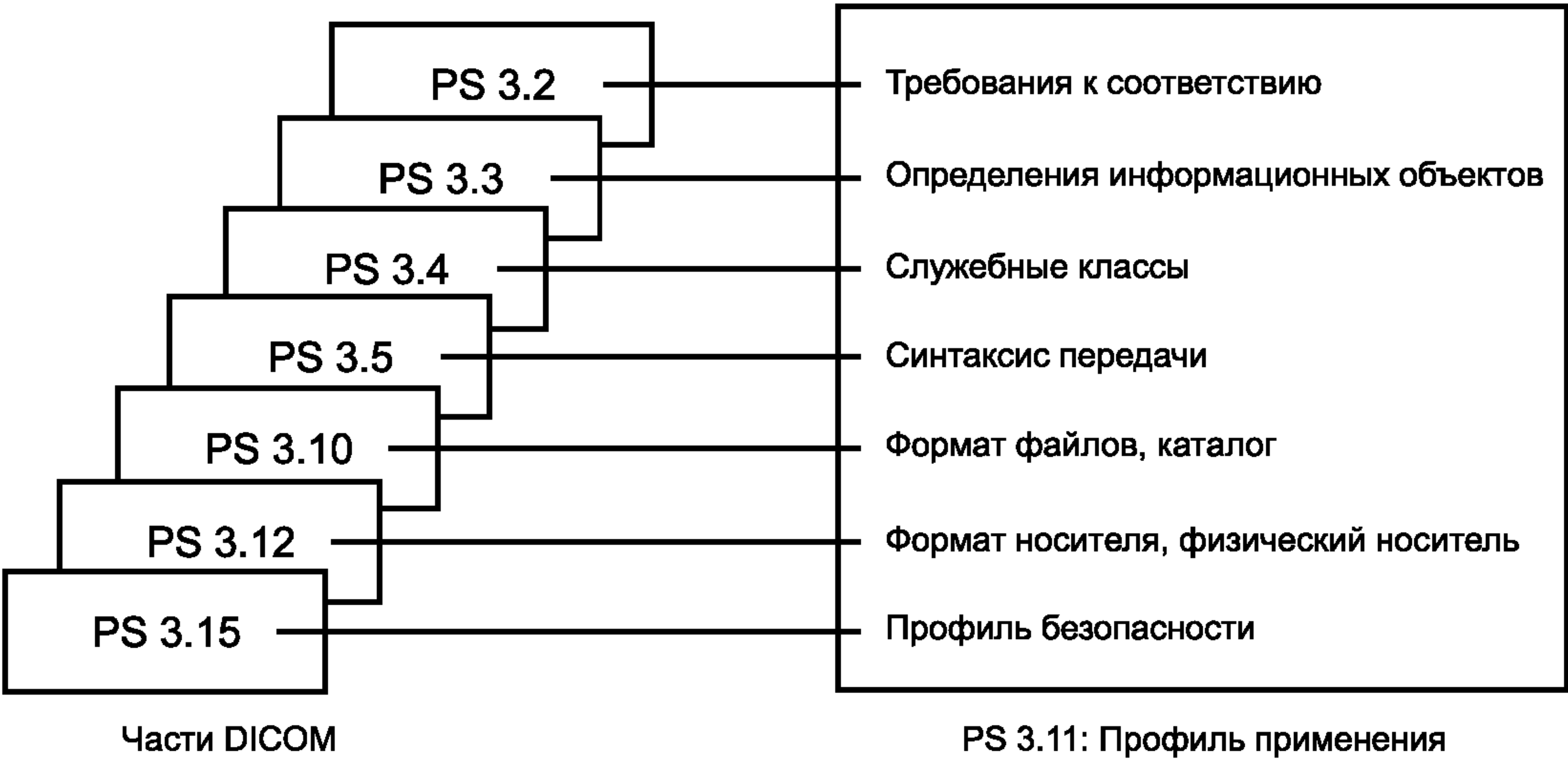
Рисунок 4 — Связь между профилем применения и частями DICOM
