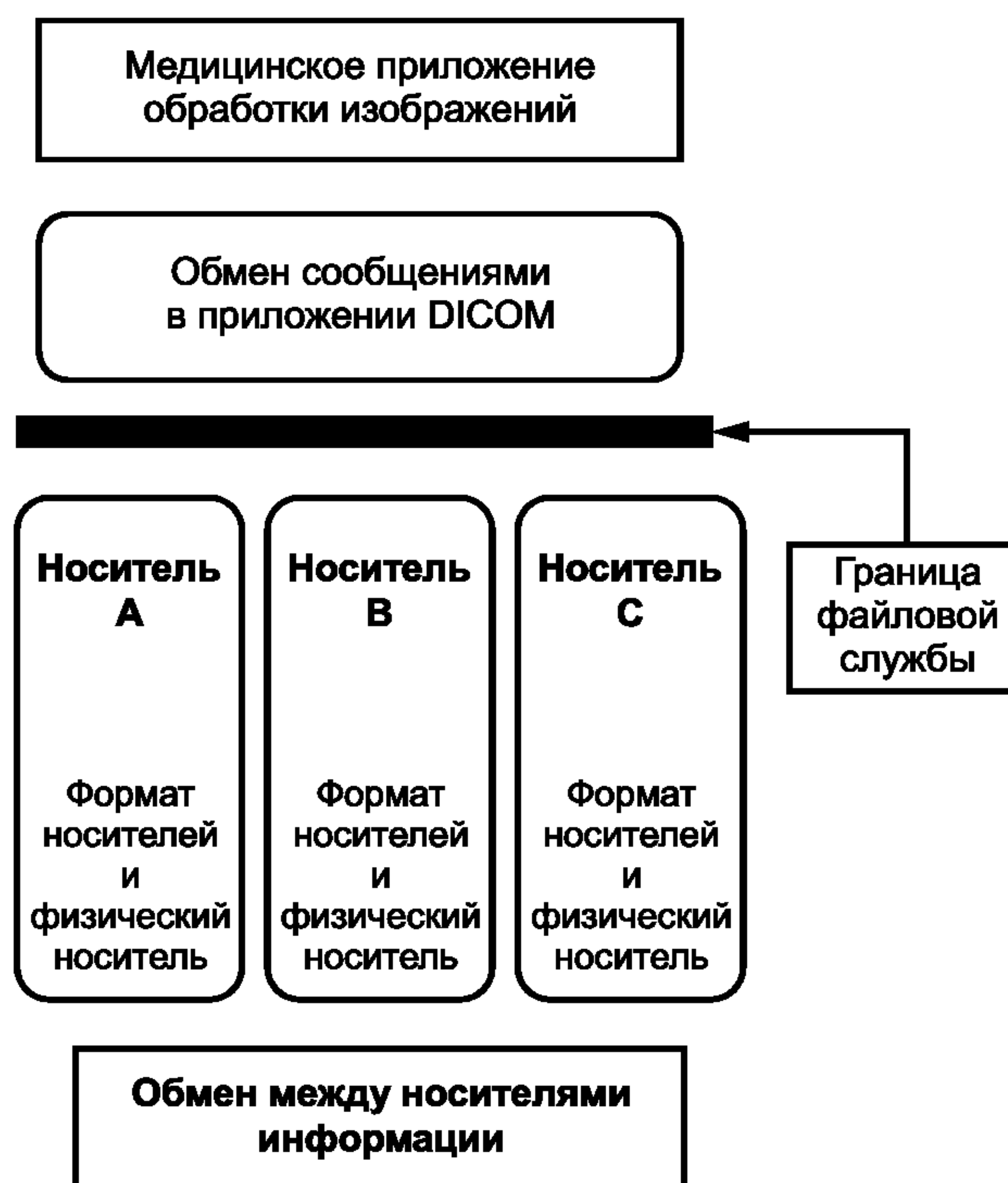
Рисунок 3 — Модель взаимосвязи между носителями DICOM
