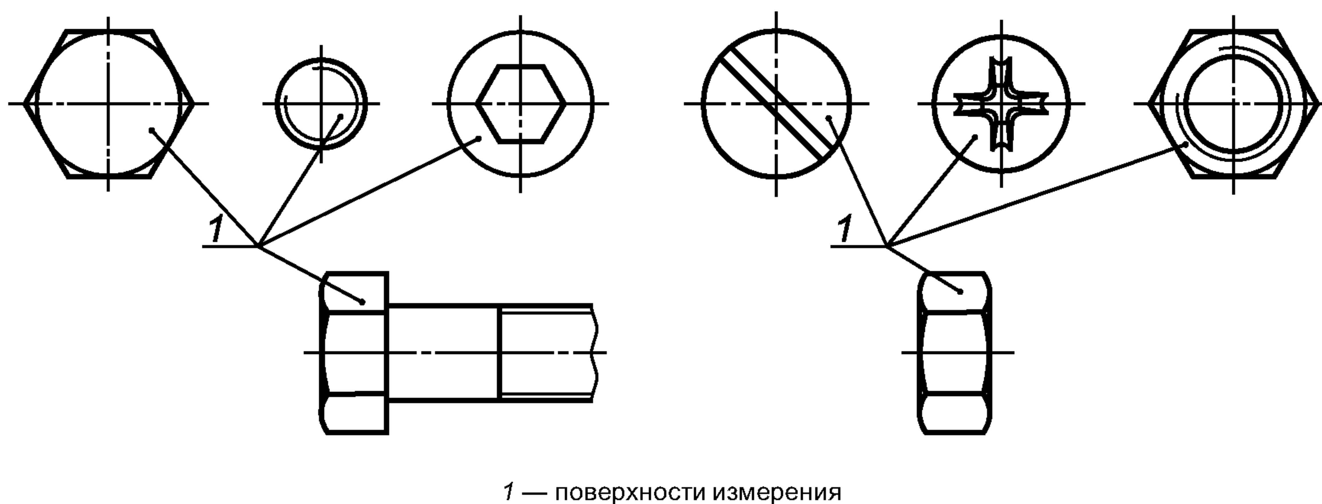
Рисунок 1 — Поверхности измерения локальной толщины покрытия на крепежных изделиях
