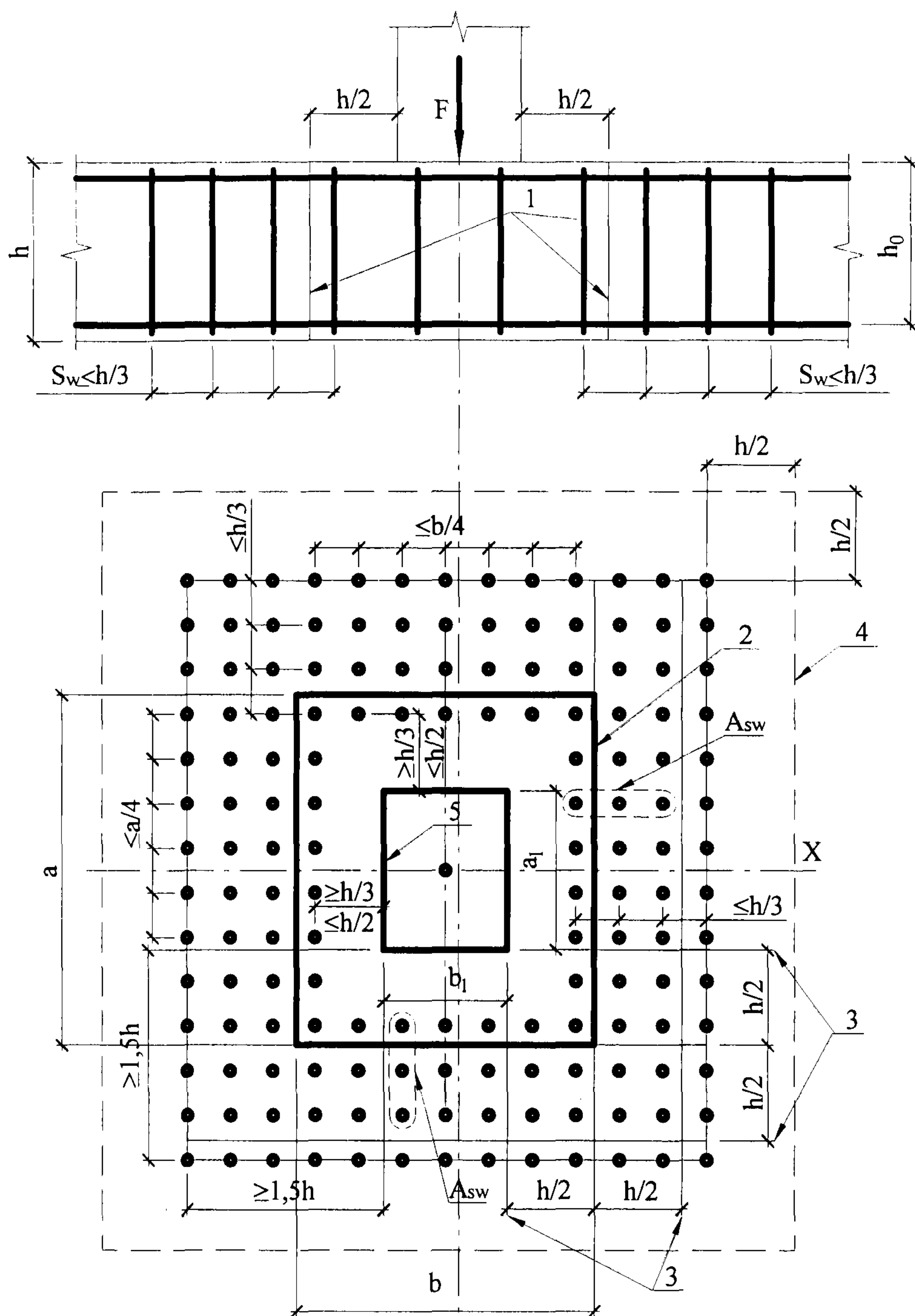
Рисунок 6.14 – Схема для расчета сталефибробетонных плит с вертикальной равномерно распределенной поперечной арматурой на продавливание: 1 – расчетное поперечное сечение; 2 – контур расчетного поперечного сечения; 3 – границы зоны, в пределах которых в расчете учитывается поперечная арматура; 4 – контур расчетного поперечного сечения без учета в расчете поперечной арматуры; 5 – контур площадки приложения нагрузки.
