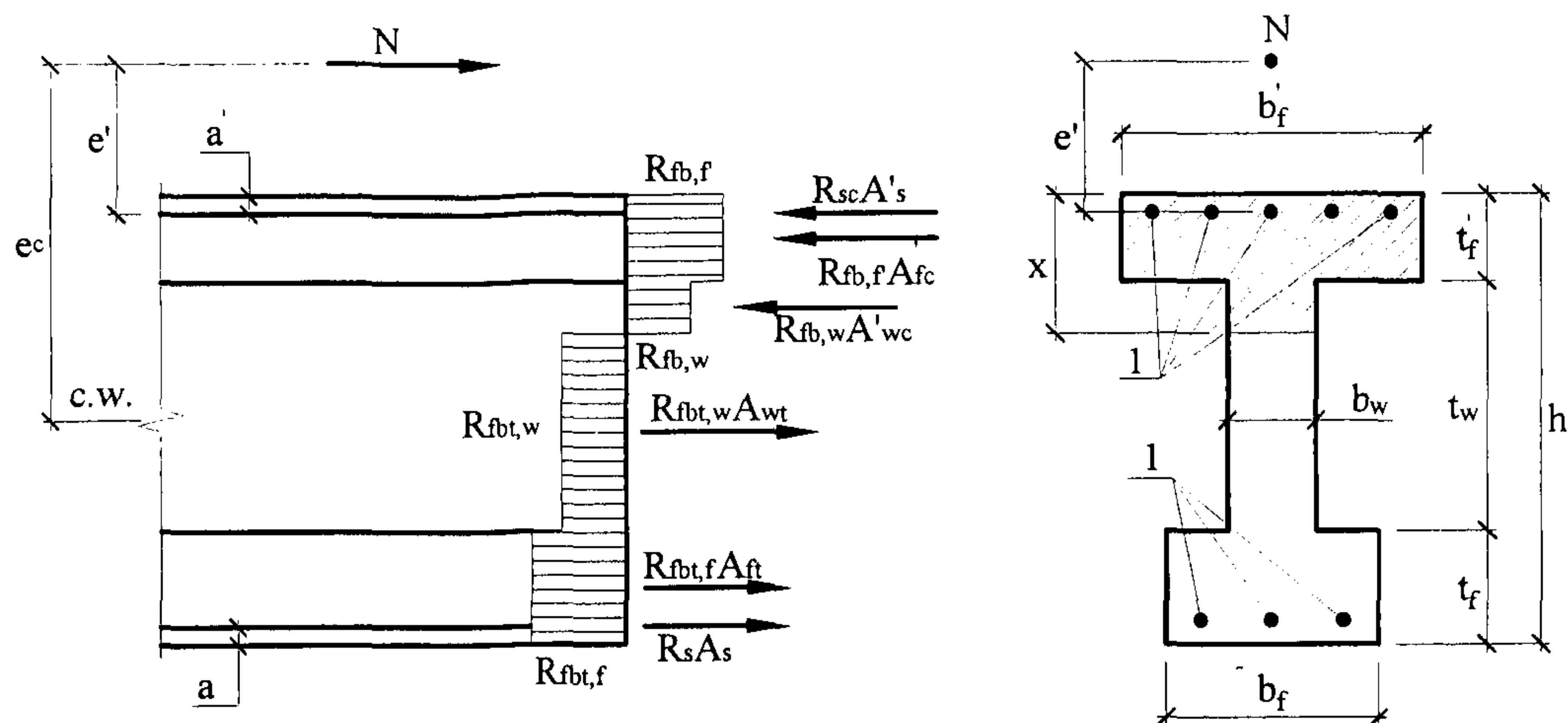
Рисунок 6.6 - Схема усилий и эпюра напряжений во внецентренно сжатых элементах двутаврового сечения при комбинированном армировании:
