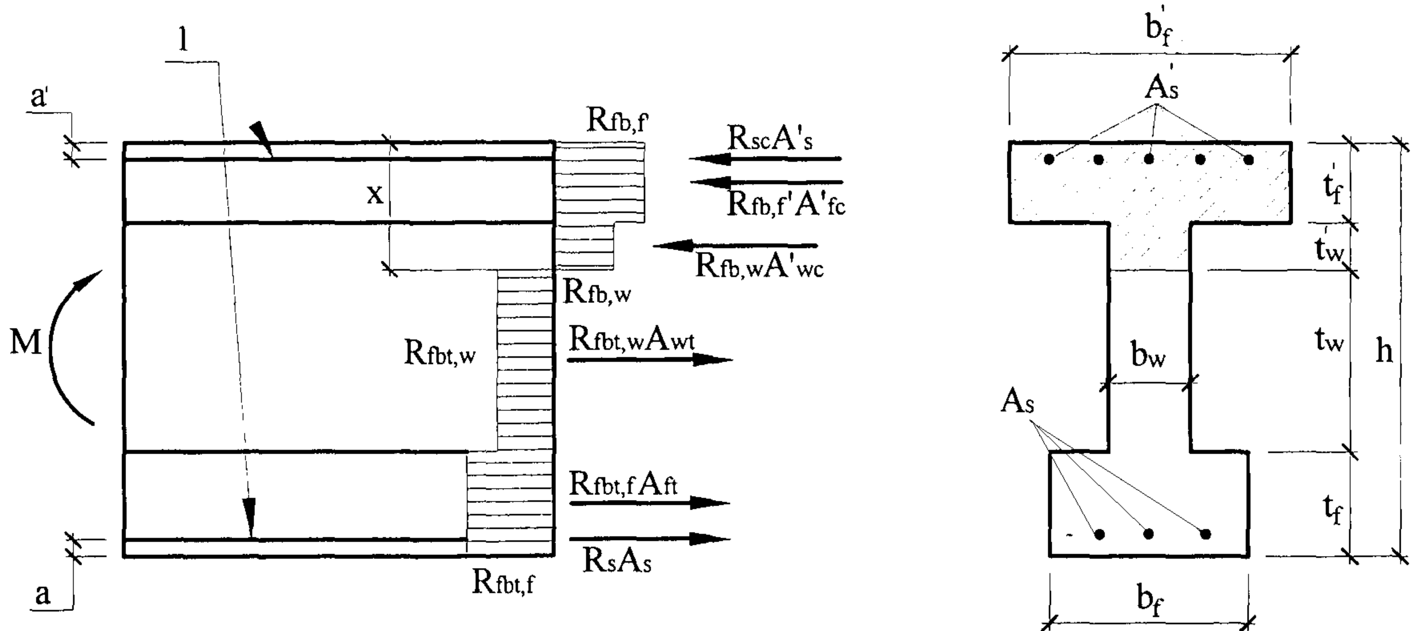
Рисунок 6.3 - Схема распределения усилий и эпюра напряжений в сечениях, нормальных к продольной оси изгибаемого элемента двутаврового сечения при комбинированном армировании а) – при x \leq t_f' ; б) – при x > t_f' ; 1 – стержневая арматура
