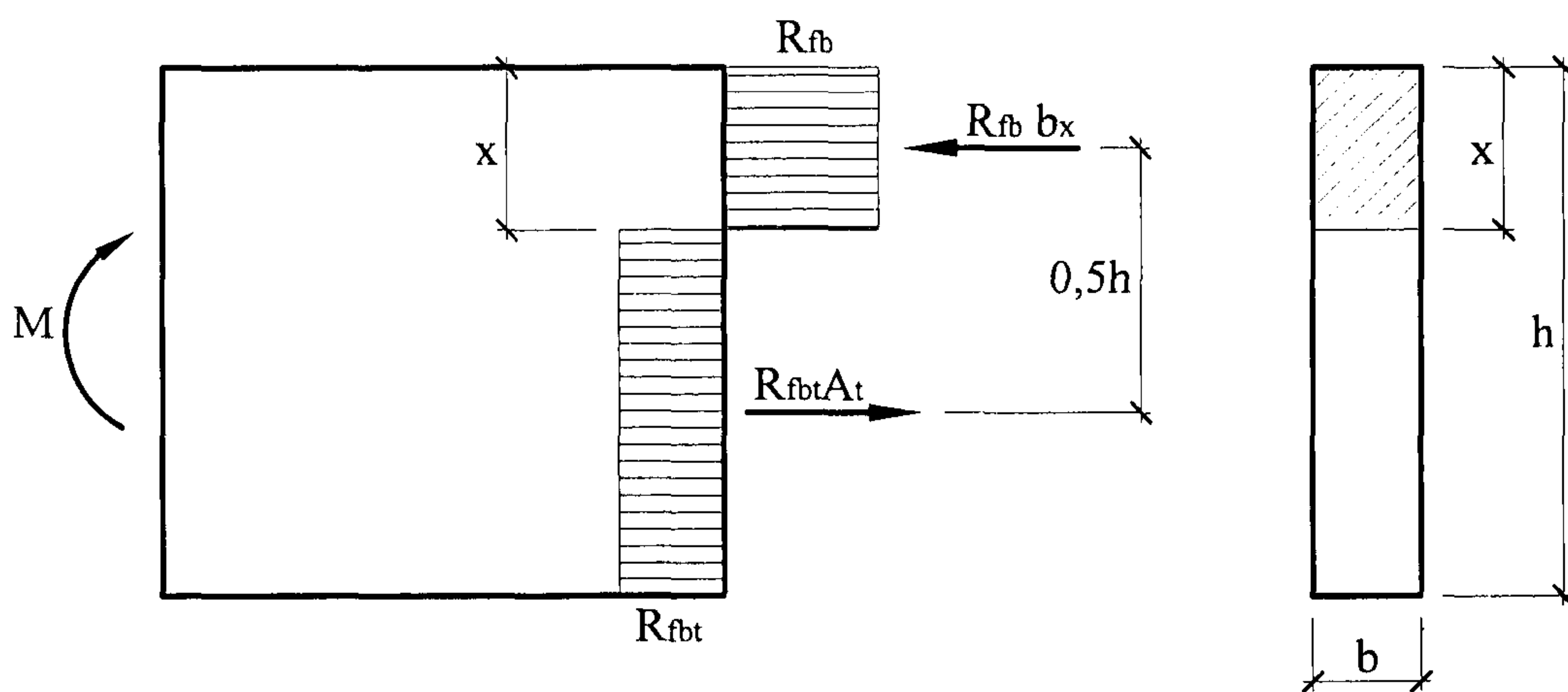
Рисунок 6.1 - Схема усилий и эпюра напряжений в сечении, нормальном к продольной оси изгибаемого сталефибробетонного элемента прямоугольного сечения, при его расчете по прочности (при фибровом
