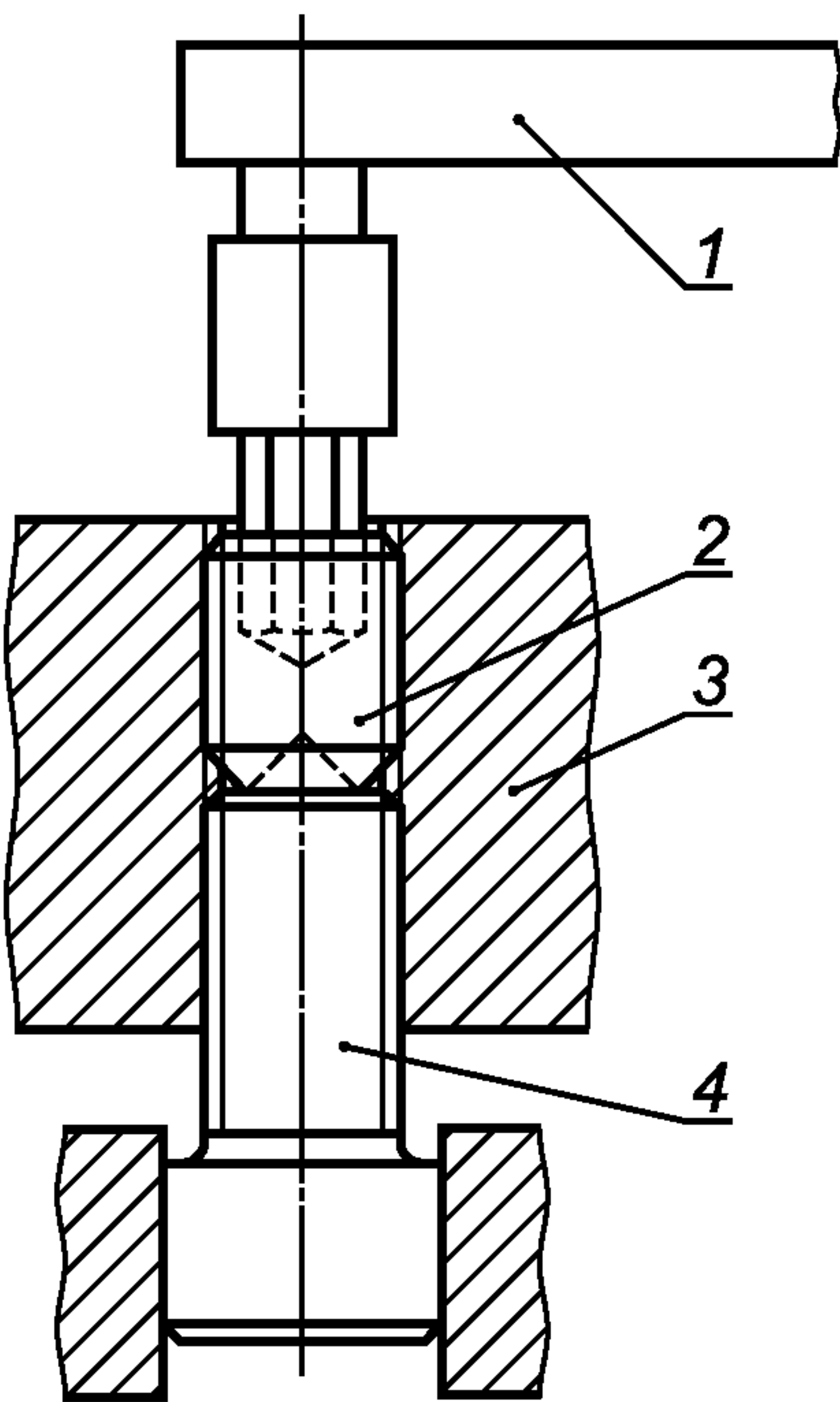
1 — гаечный ключ с ограничением по крутящему моменту; 2 — испытуемый винт; 3 — испытательный блок твердостью не менее 50 HRC с допуском 5H (по ИСО 965-3) для внутренней резьбы; 4 — опорный винт твердостью от 450 до 570 HV
