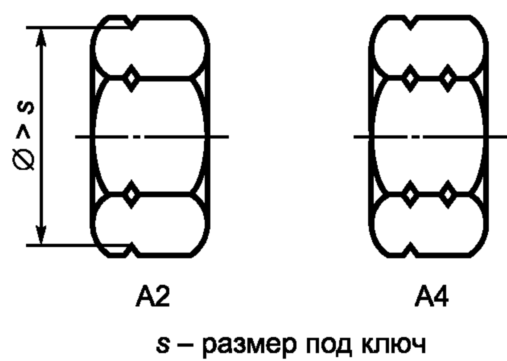
Вариант маркировки в виде бороздок (только для марок сталей А2 и А4) П р и м е ч а н и е — Маркировка левой резьбы — по ИСО 898-2. Рисунок 2 — Маркировка гаек
