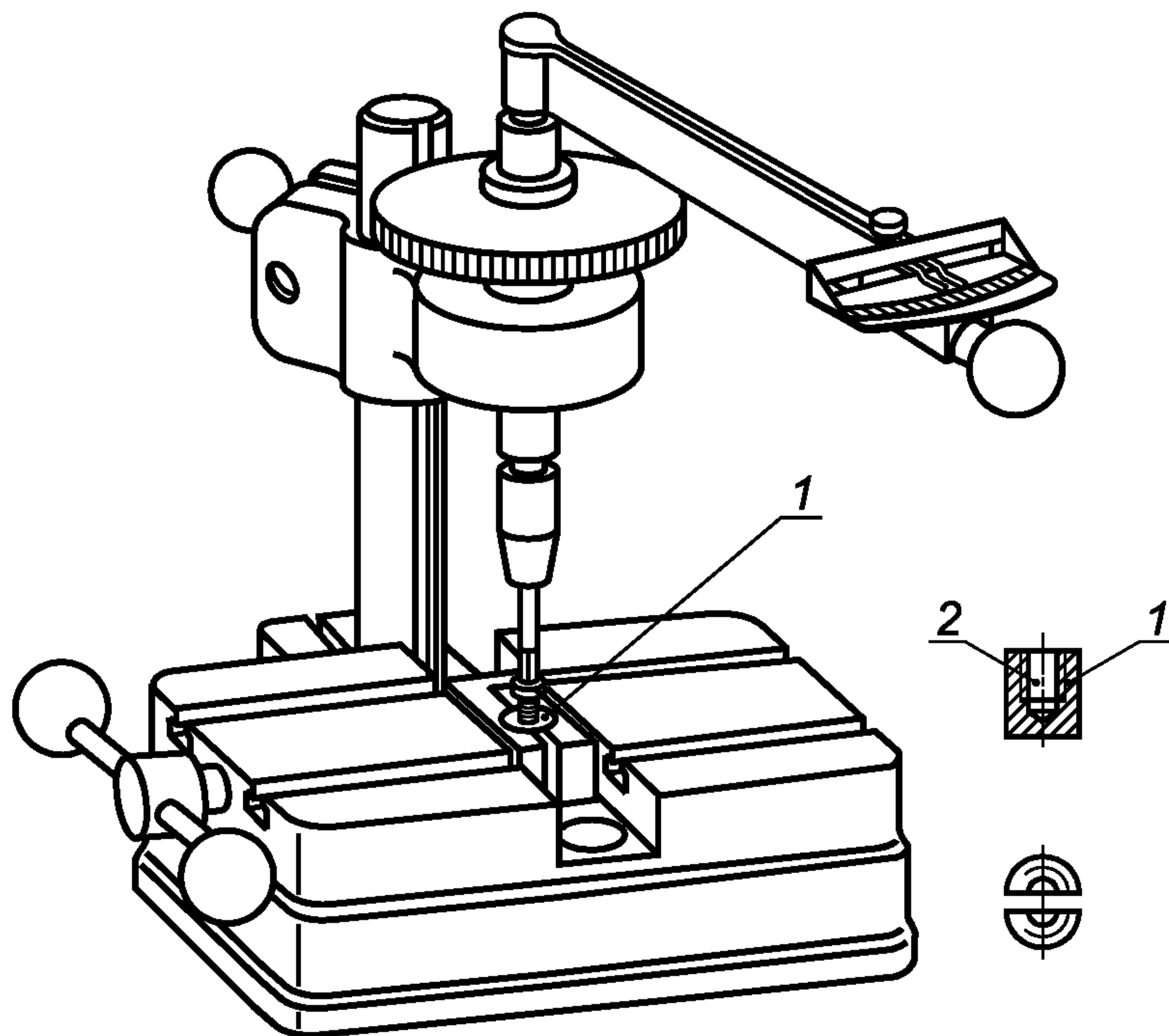
1 — разъемный зажим; 2 — глухое отверстие
