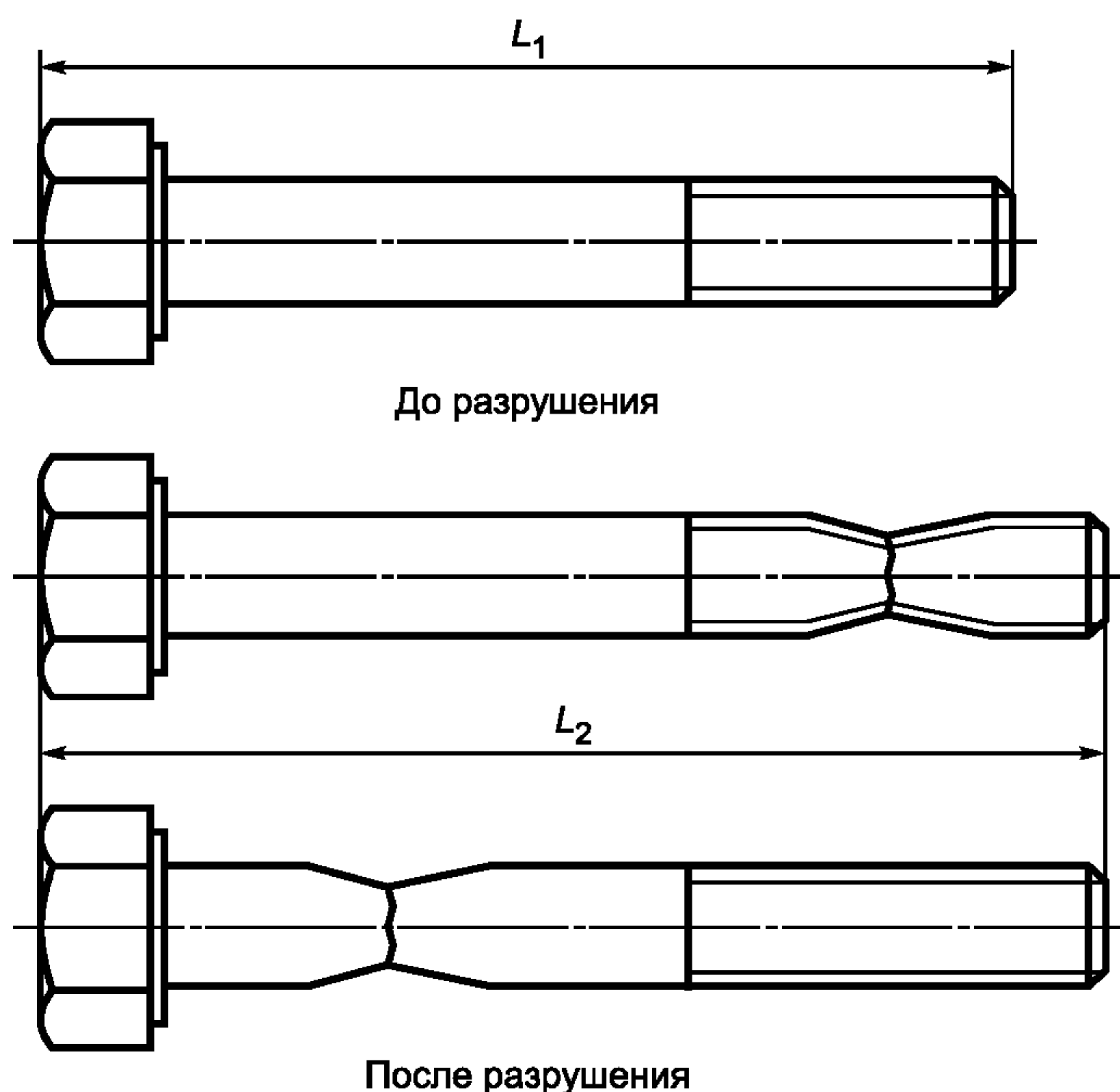
Рисунок 5 — Определение удлинения при разрыве A (см. 6.2.4)
