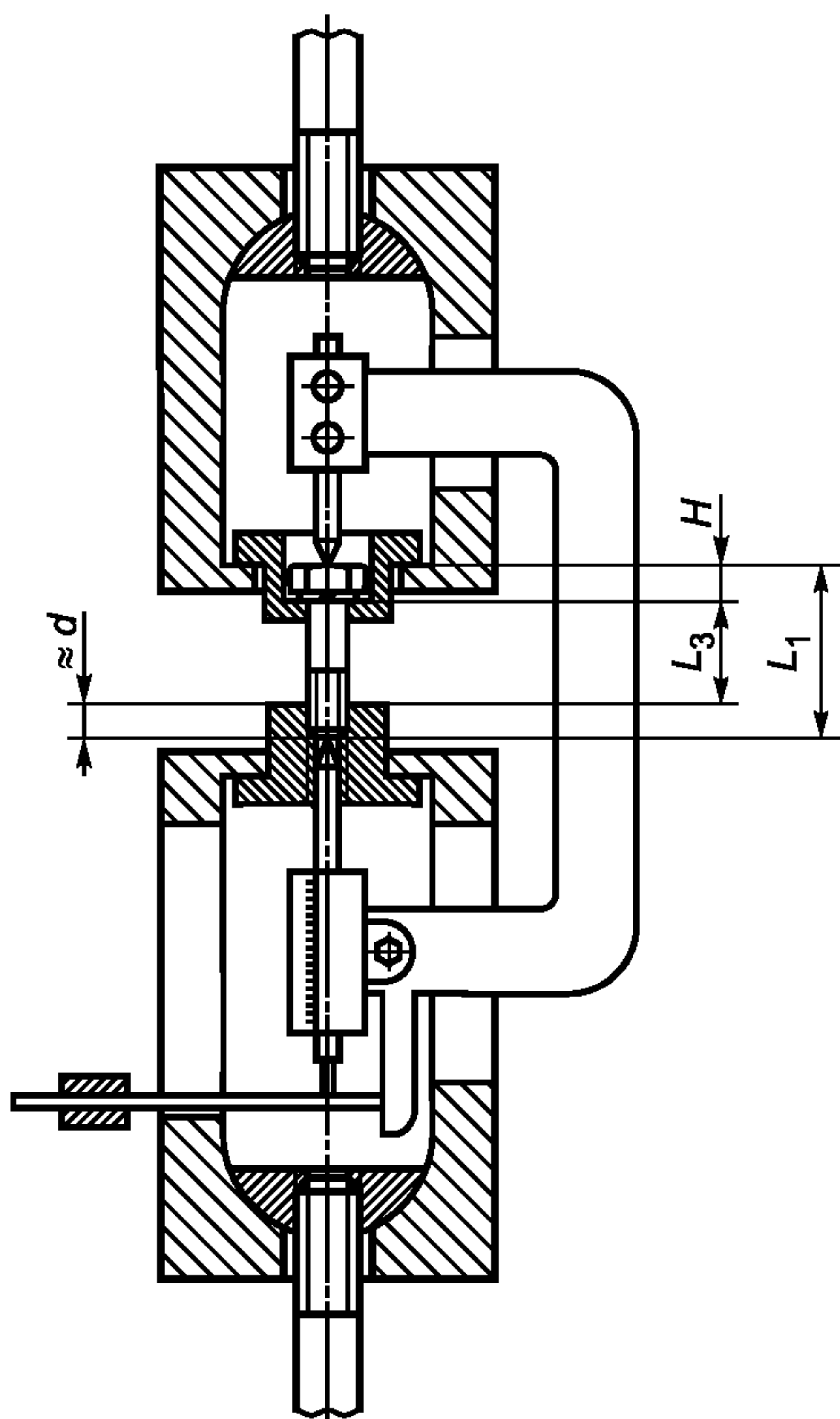
Рисунок 3 — Тензометр, установленный на болт в самоцентрирующих зажимах
