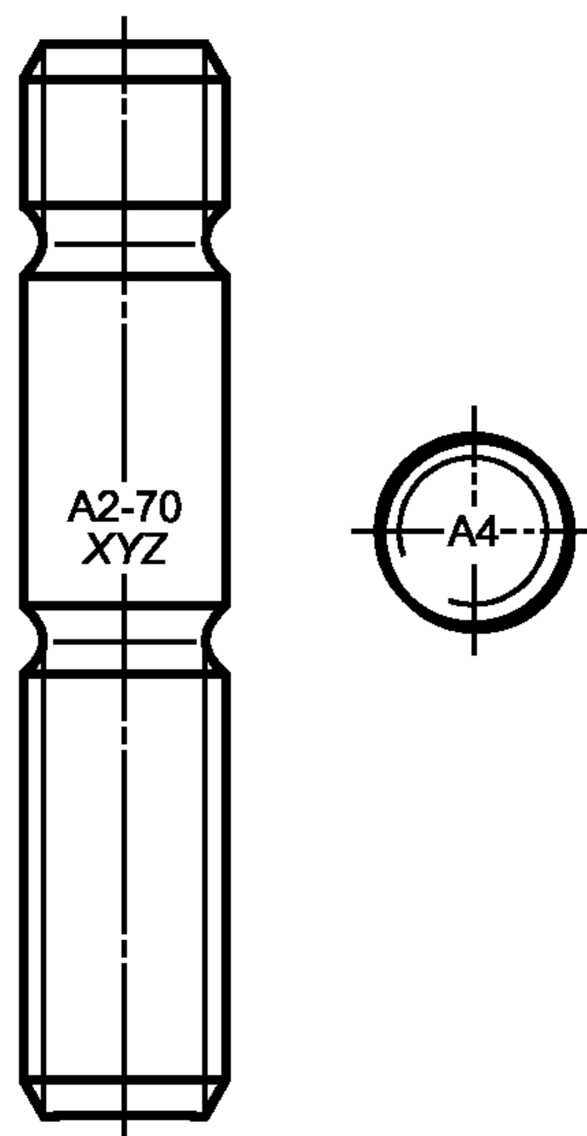
Маркировка шпилек
