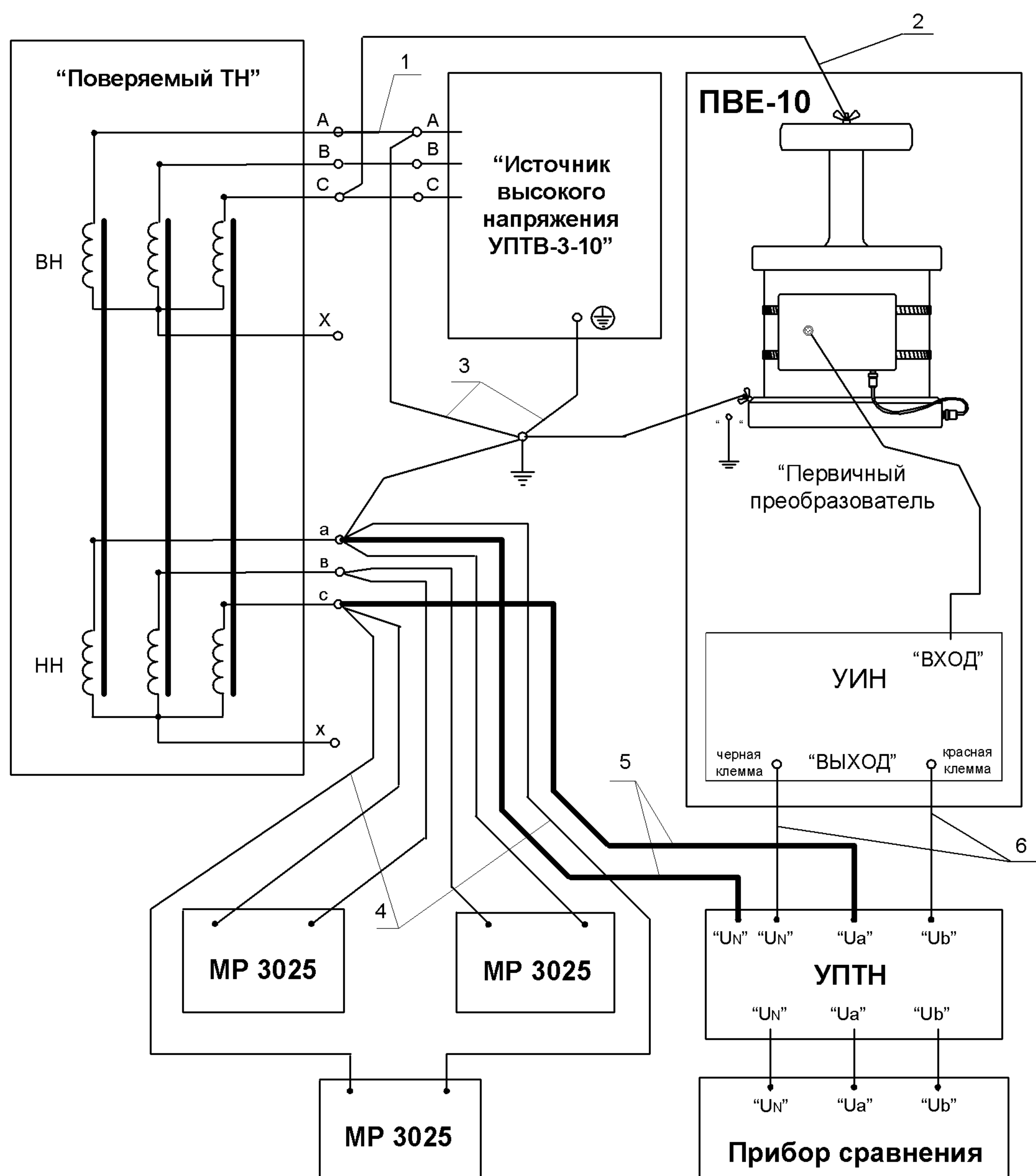
Рис.7. Схема поверки трехфазного ТН обмотки «с-а».
