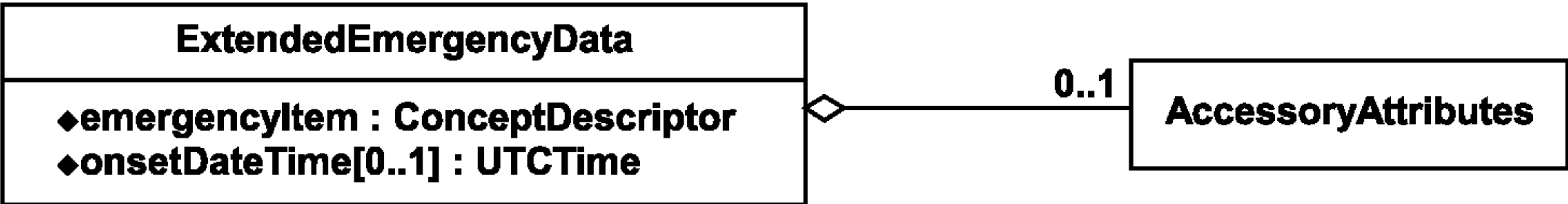
Рисунок 5 — Структура класса ExtendedEmergencyData
