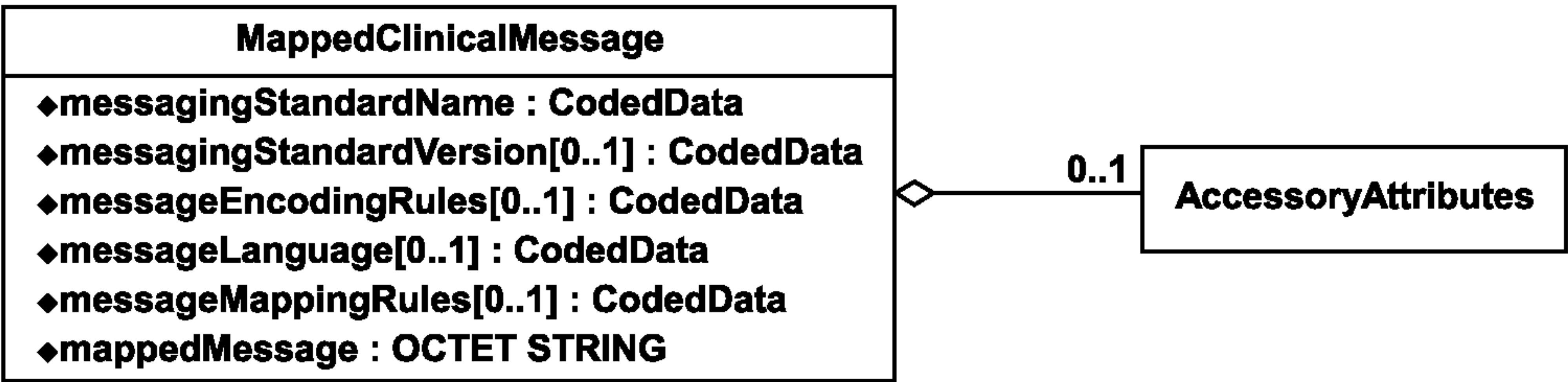
Рисунок 4 — Структура класса MappedClinicalMessage
