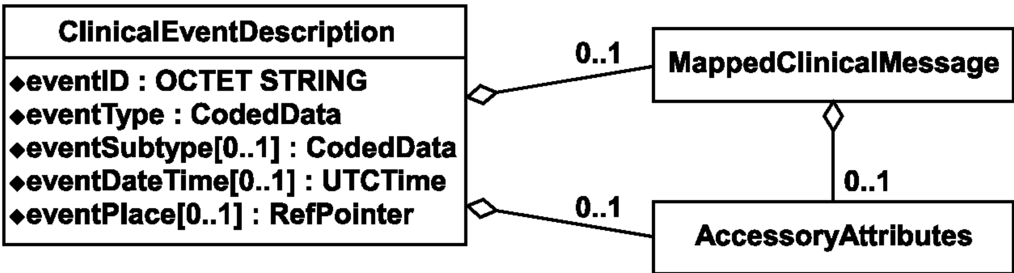
Рисунок 3 — Структура класса ClinicalEventDescription
