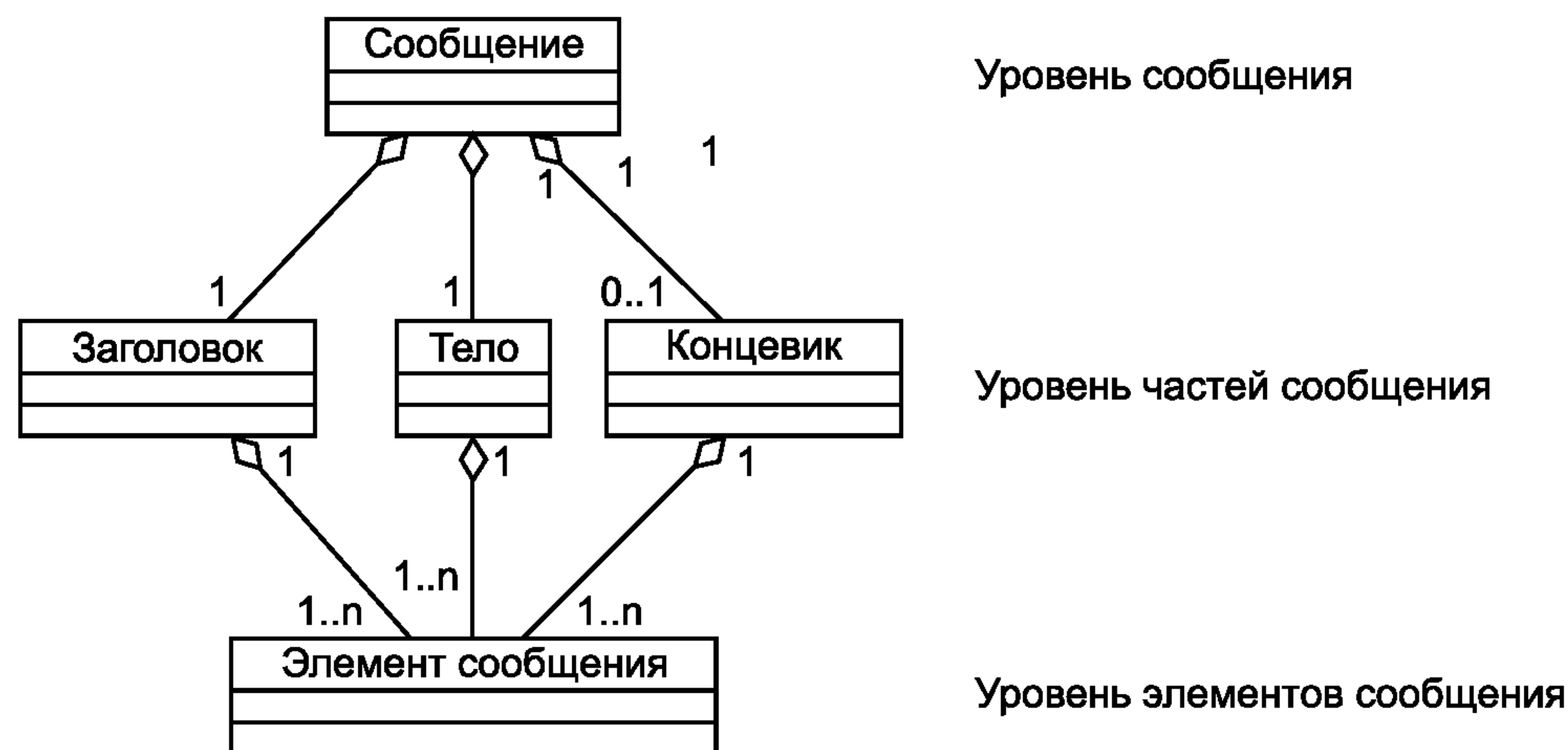
Рисунок В.3 — Уровни структуры сообщения
