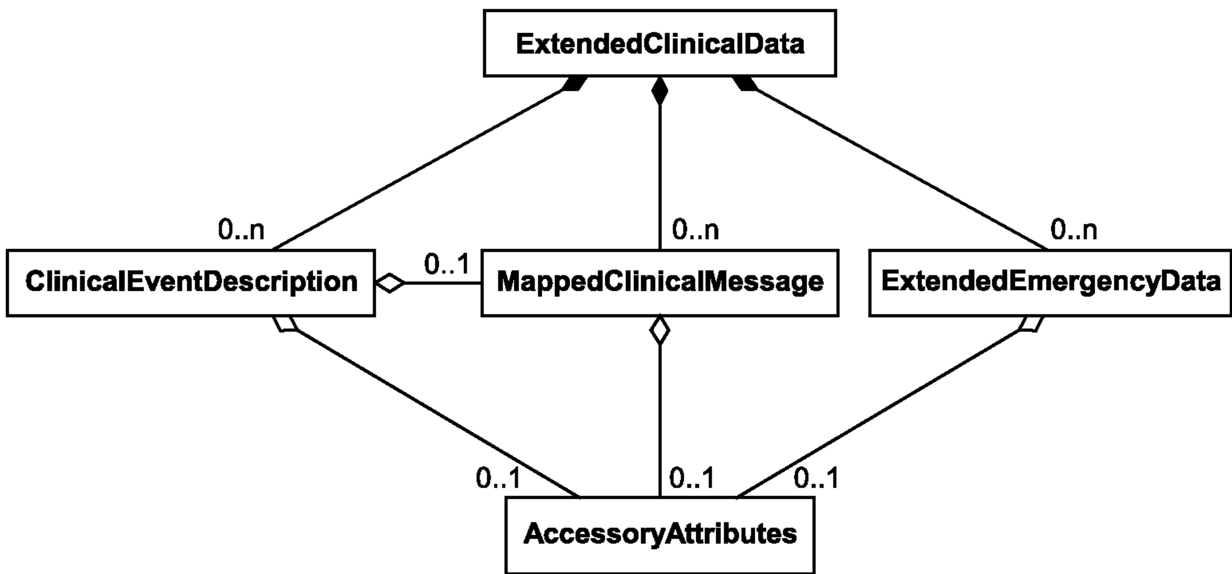
Рисунок 2 — Структура класса ExtendedClinicalData
