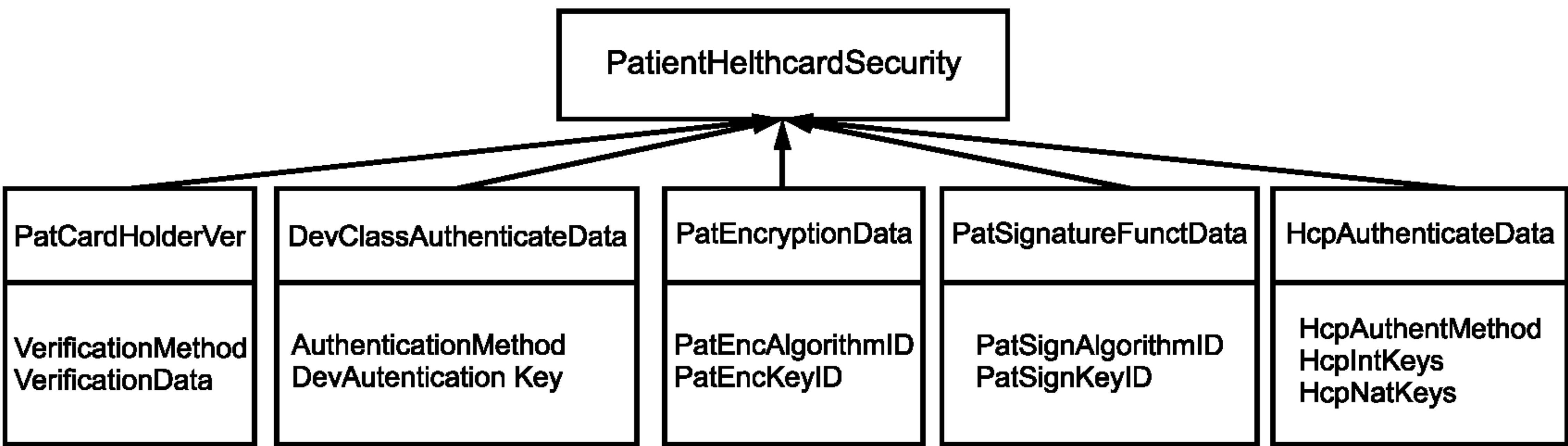
Рисунок 6 — Структура класса информационных объектов «PatientHealthcardSecurity»
