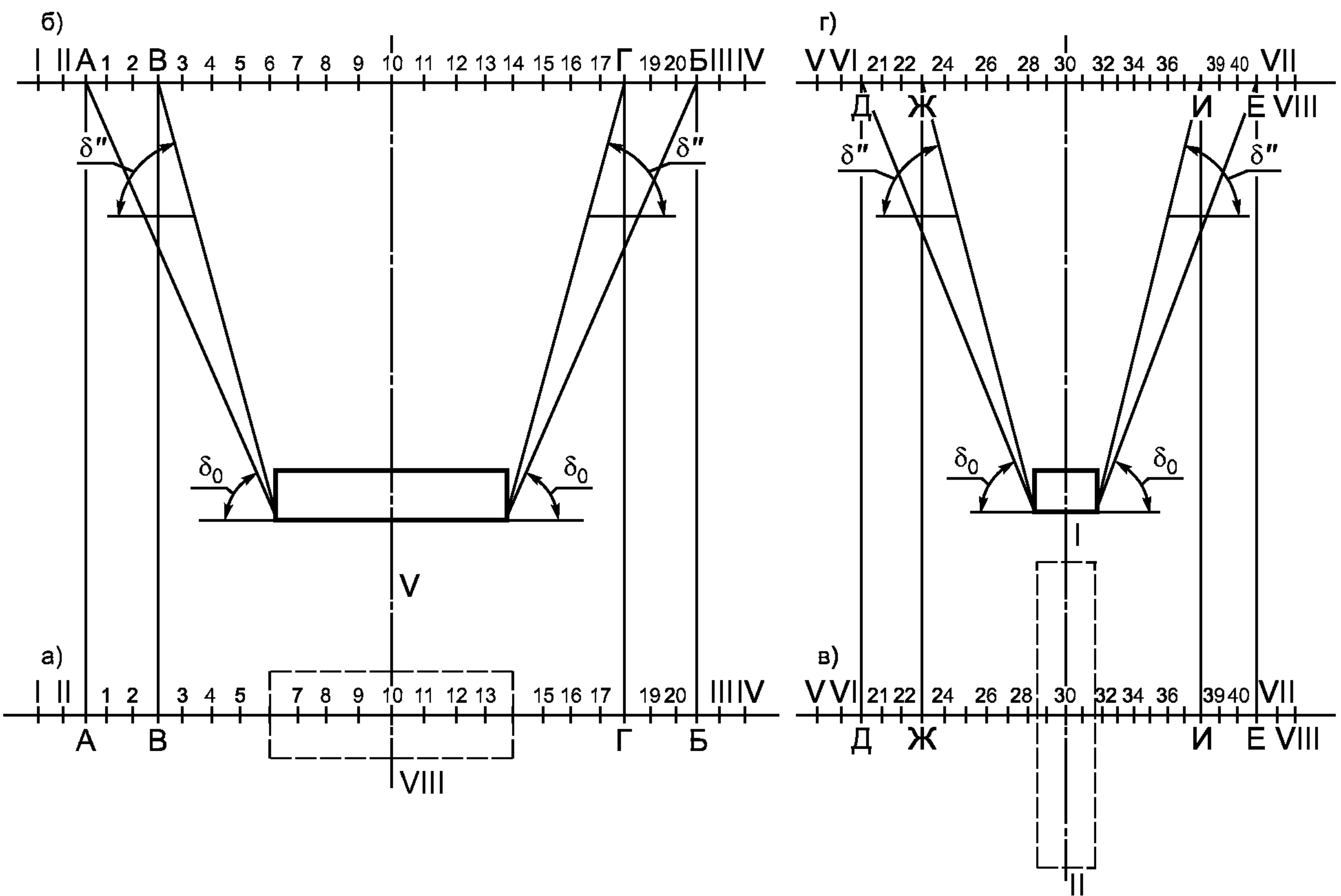
а) и б) — на плане и разрезе вдоль сооружения; в) и г) — на плане и разрезе поперек сооружения; I, II, III, IV, V, VI, VII, VIII — опорные реперы; 1, 2, 3 ... 40 — рабочие реперы; АБ и ДЕ — зоны влияния подземного сооружения на земную поверхность; ВГ и ЖИ — зоны возможного образования трещин
