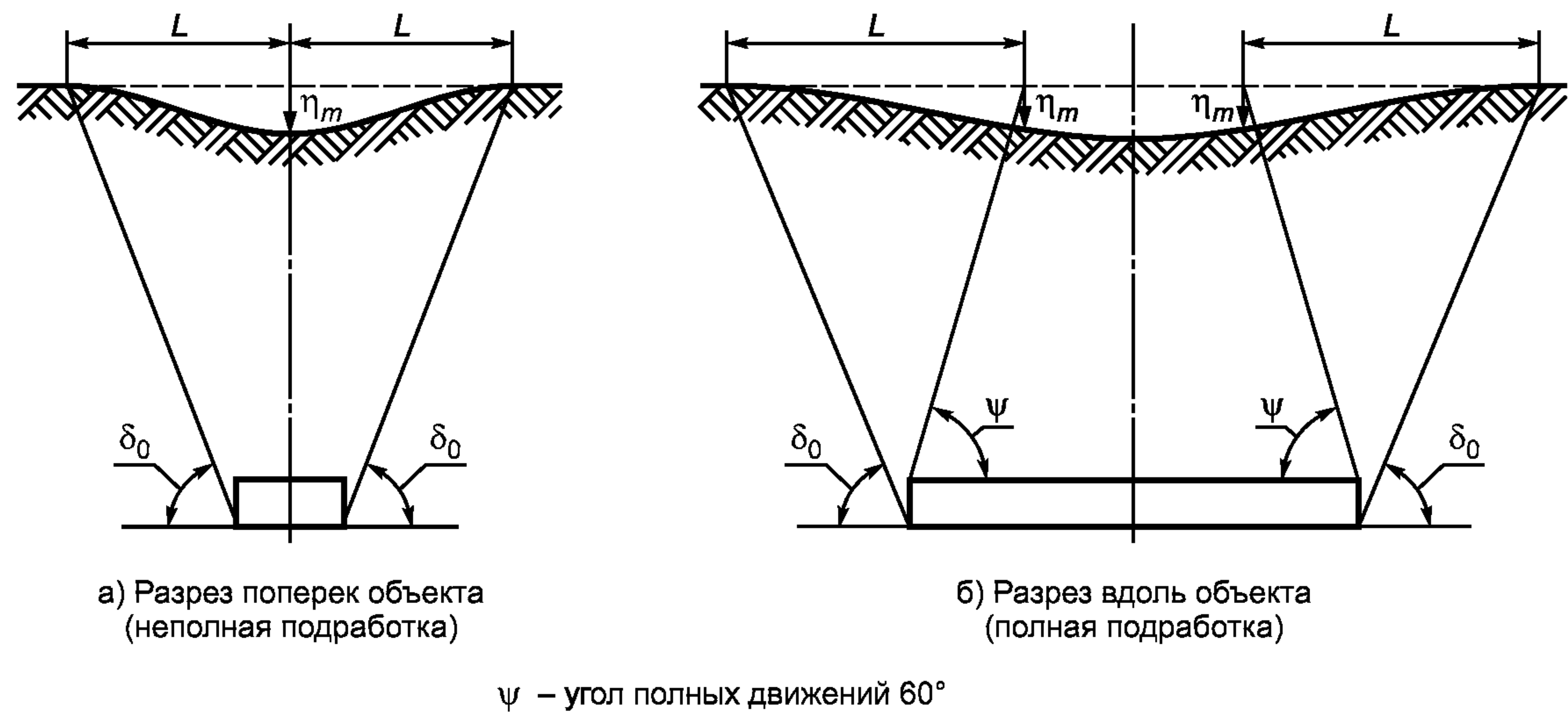
Рисунок С.1 — Основные параметры мульды сдвижения
