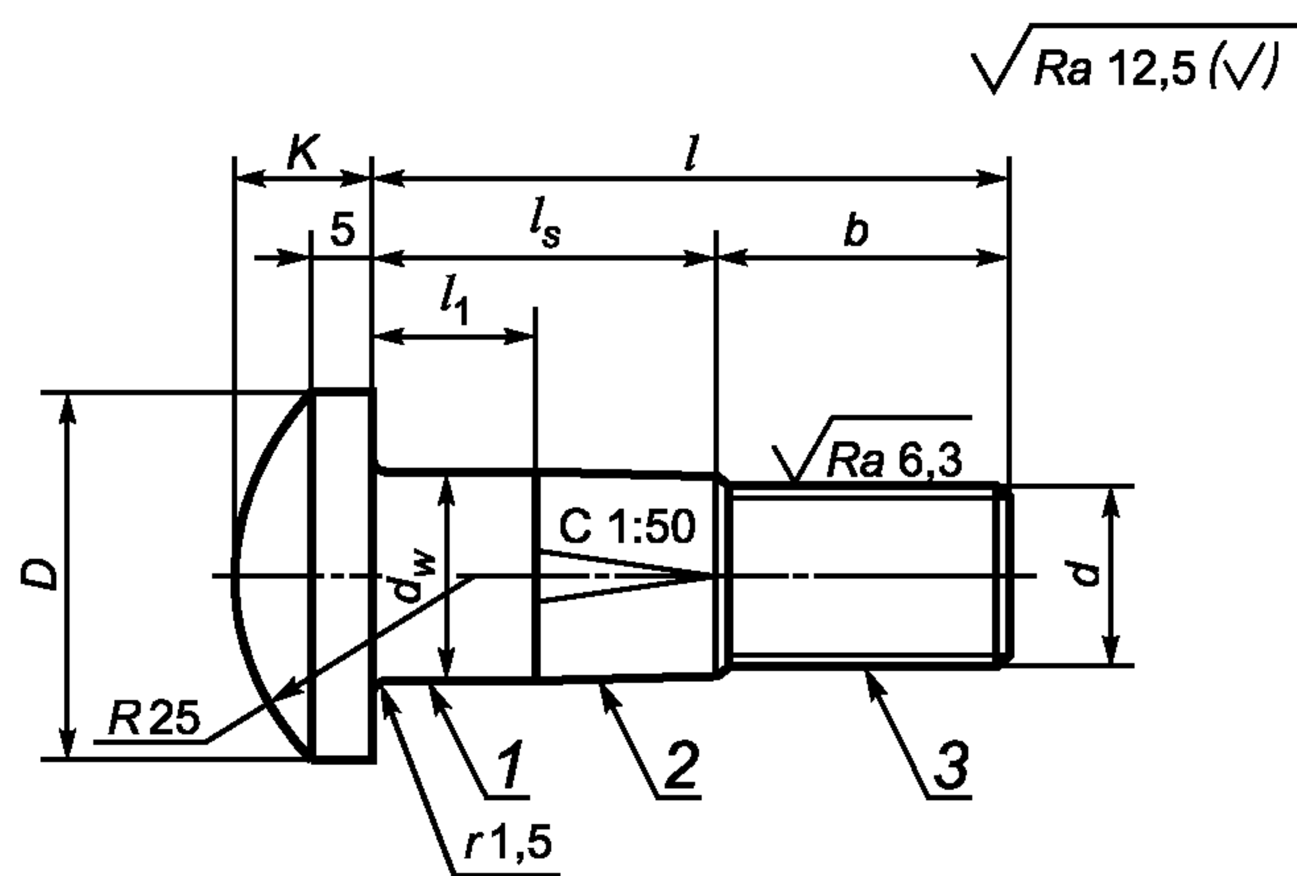
1 — цилиндрическая часть; 2 — коническая часть; 3 — резьба
