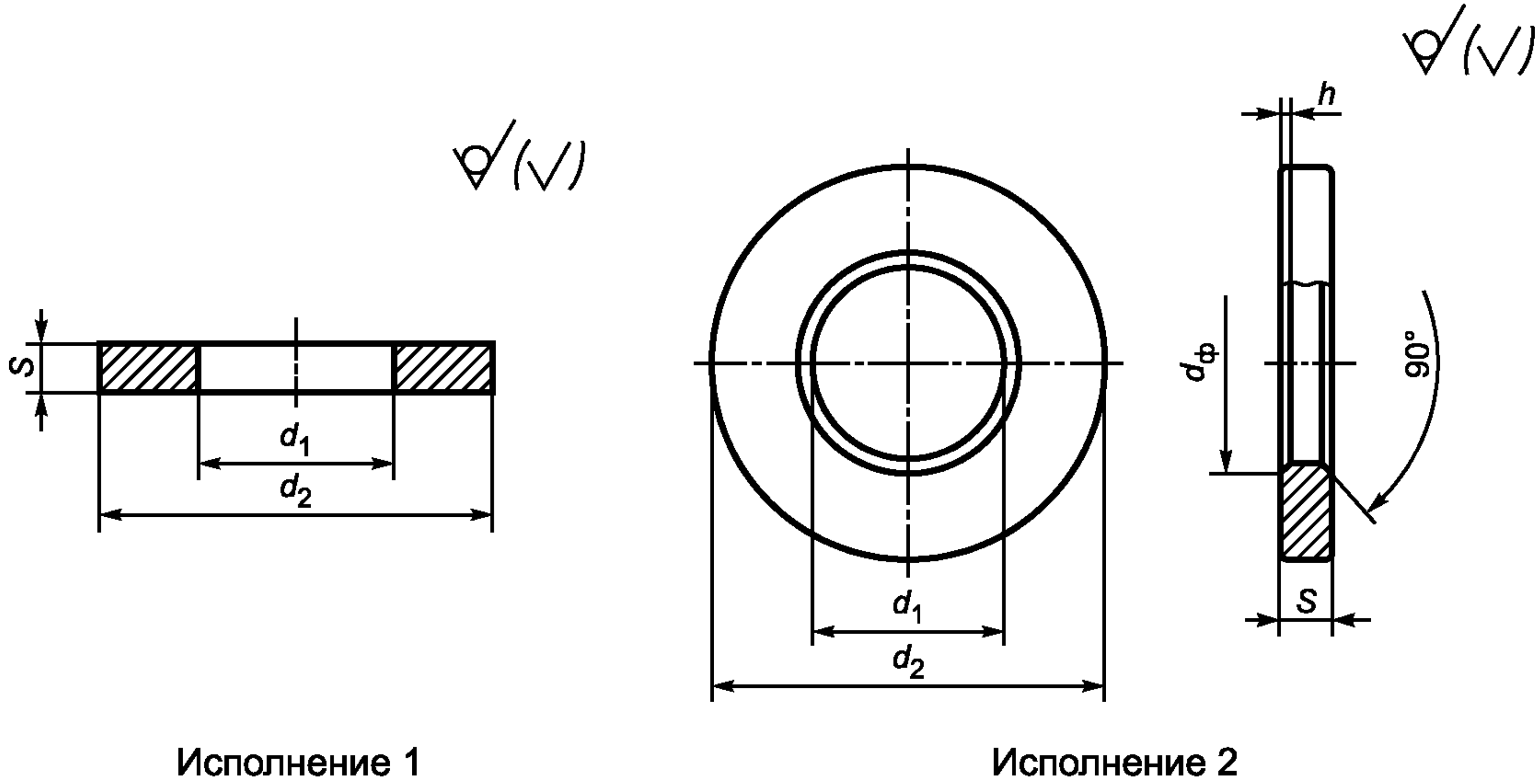
Рисунок 4 — Конструкция шайб
