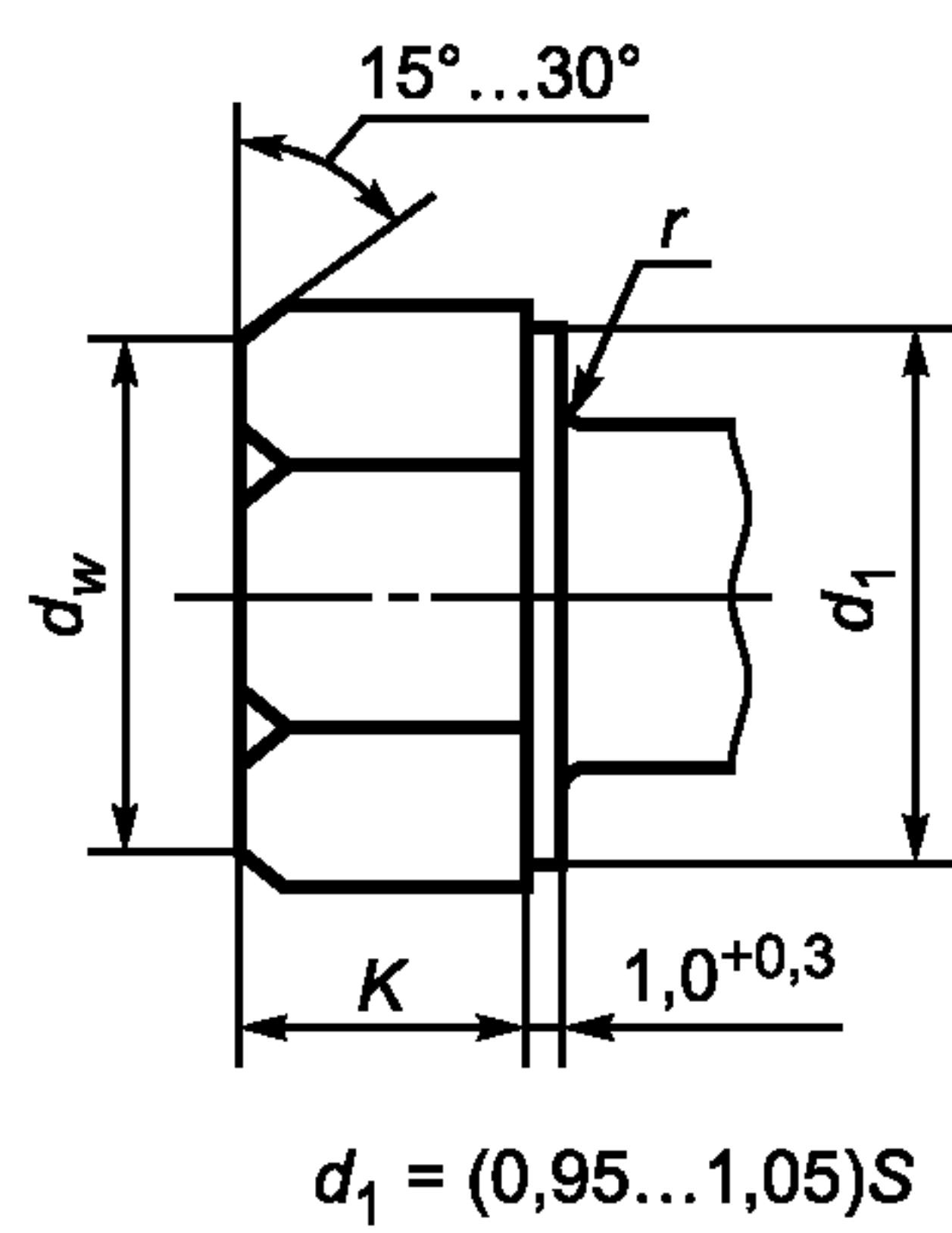
Исполнение 3 головки болта
