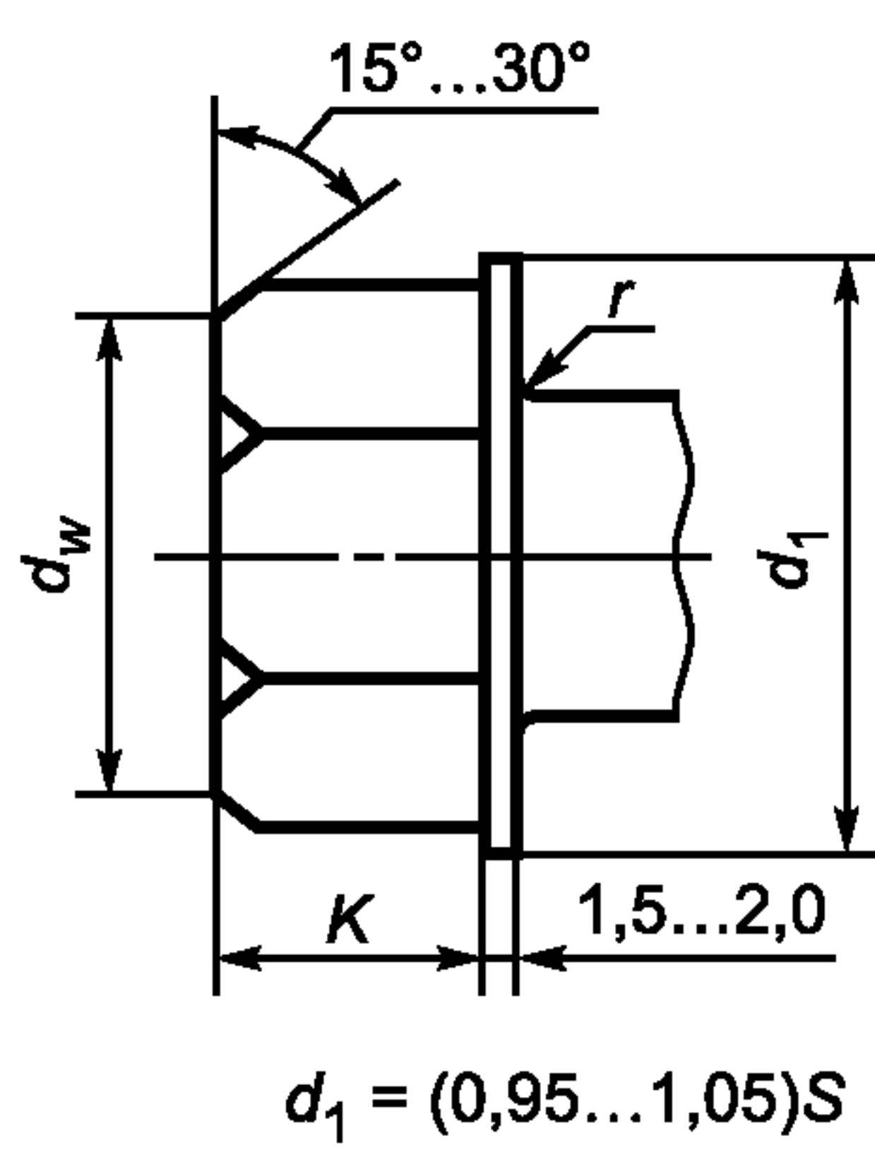
Исполнение 4 головки болта
