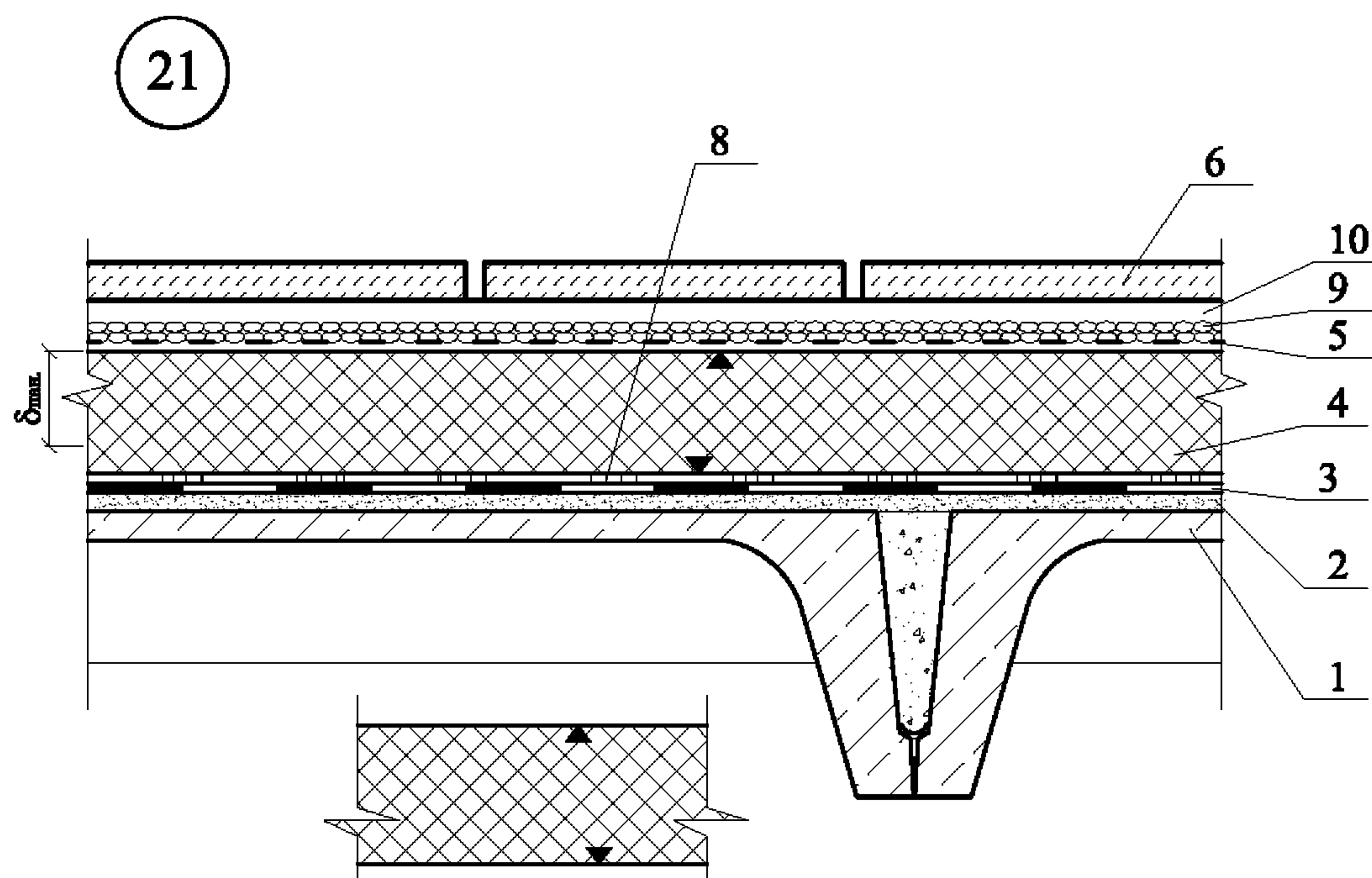
ориентация покровных слоев панели при монтаже
