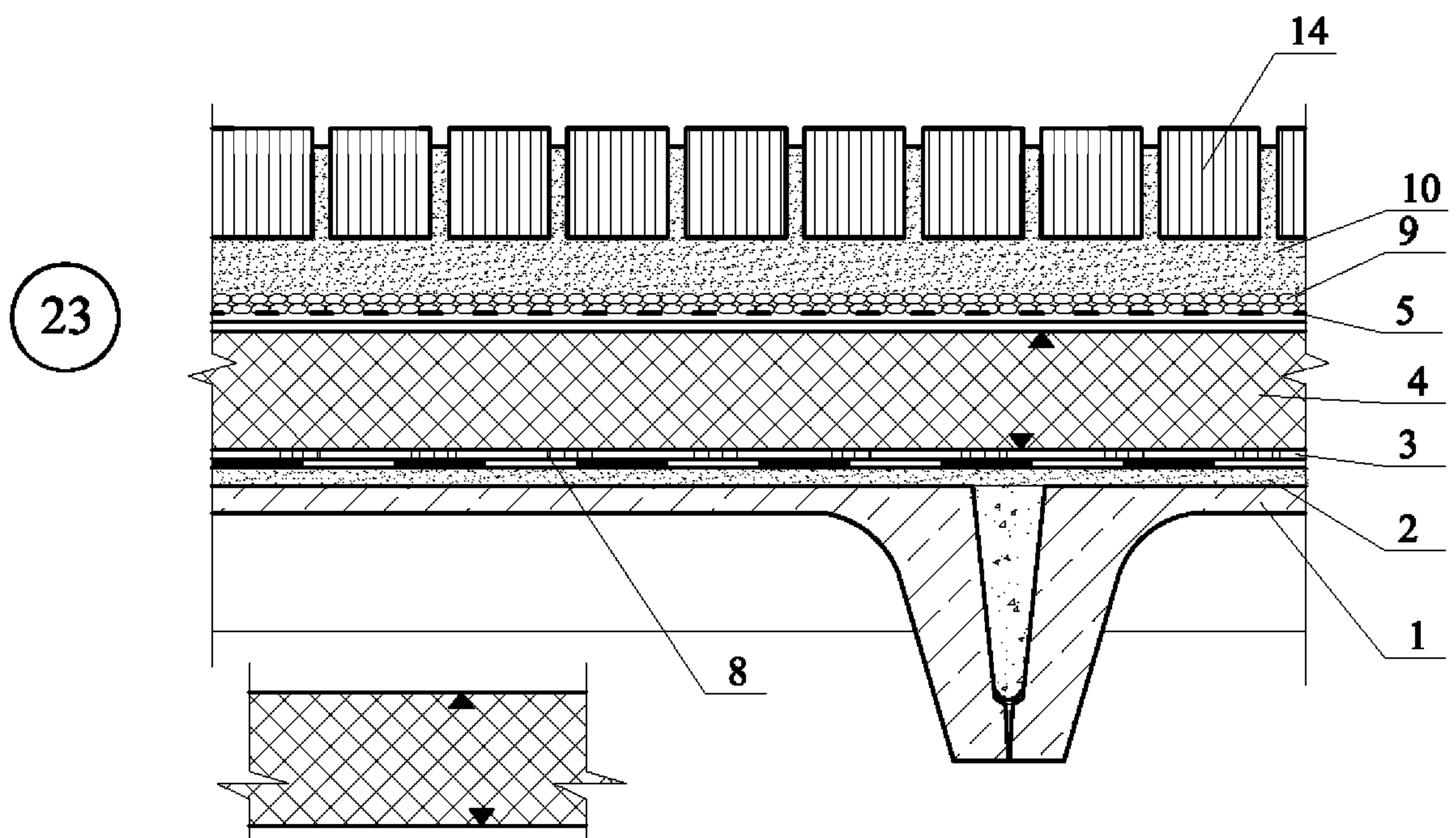
ориентация покровных слоев панели при монтаже
