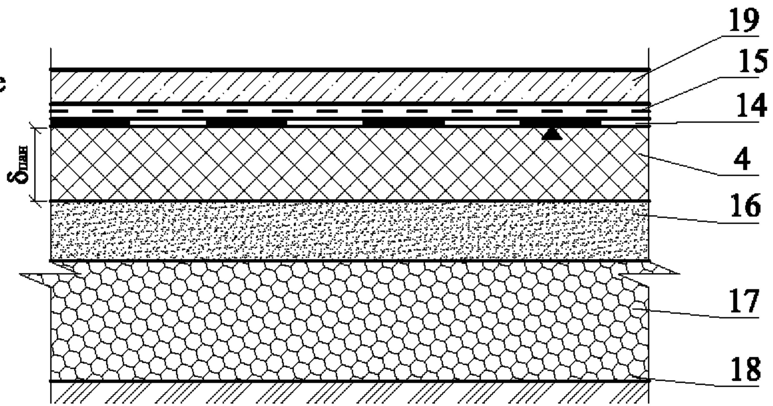
ориентация покровных слоев панели при монтаже
