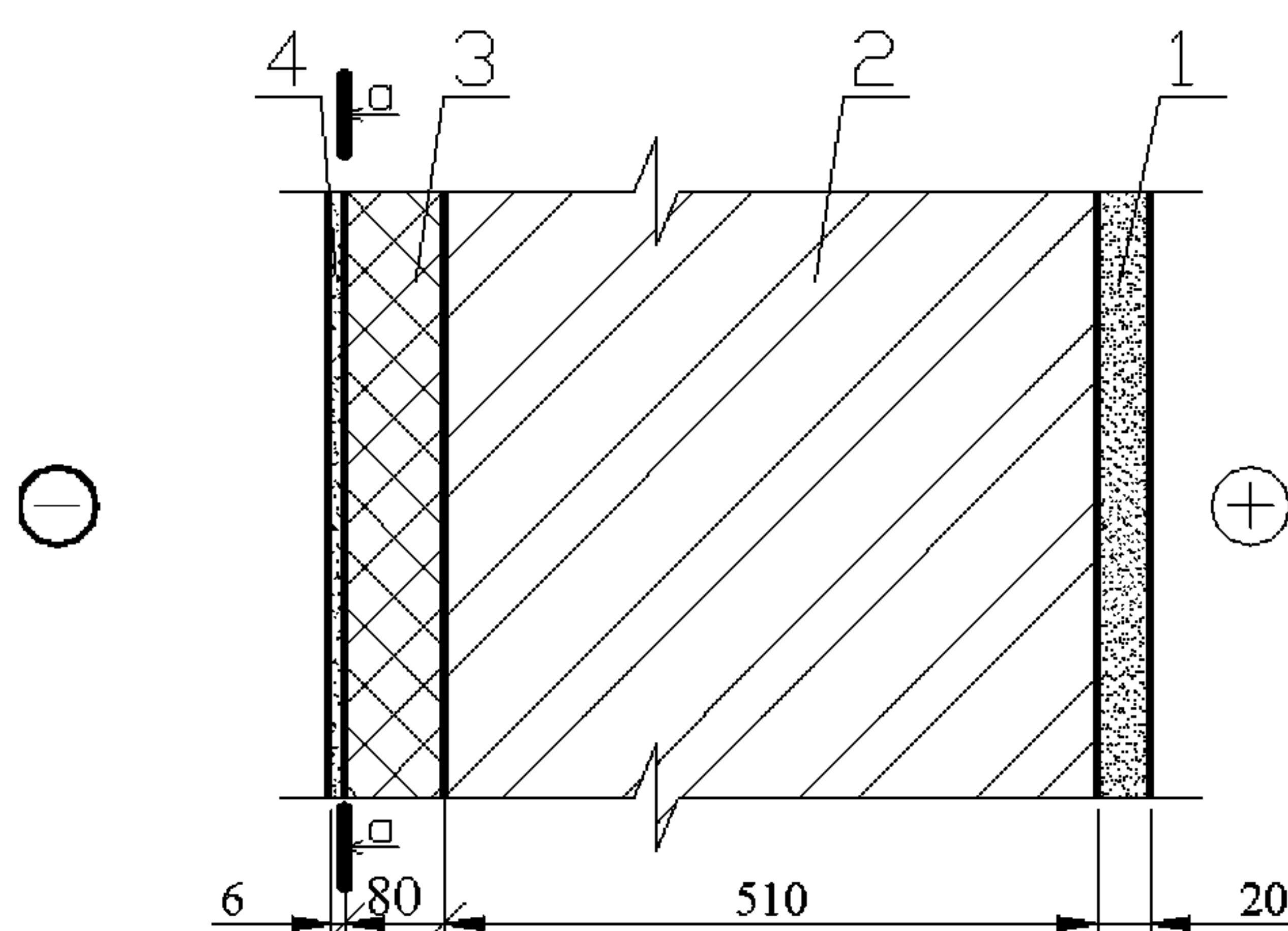
а-а – плоскость возможной конденсации
