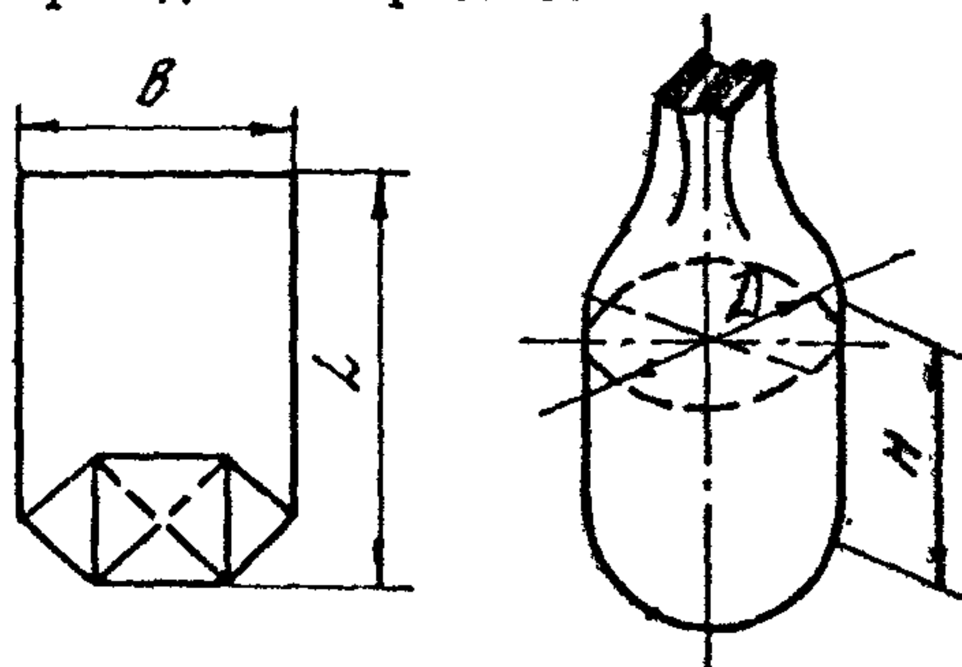
Рис. 3. Мешок типа МКР-I, ММ
