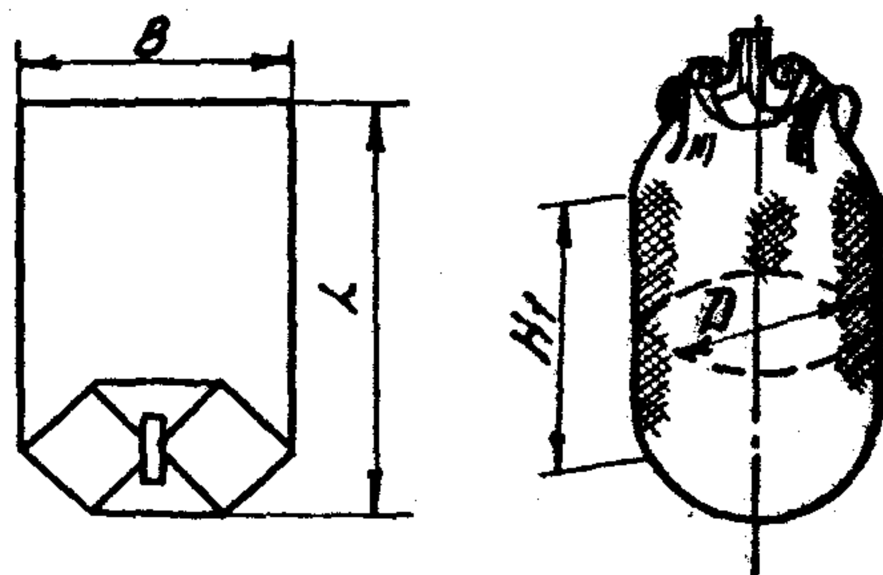
Рис. 2. Мешок типа МКР-I, СС
