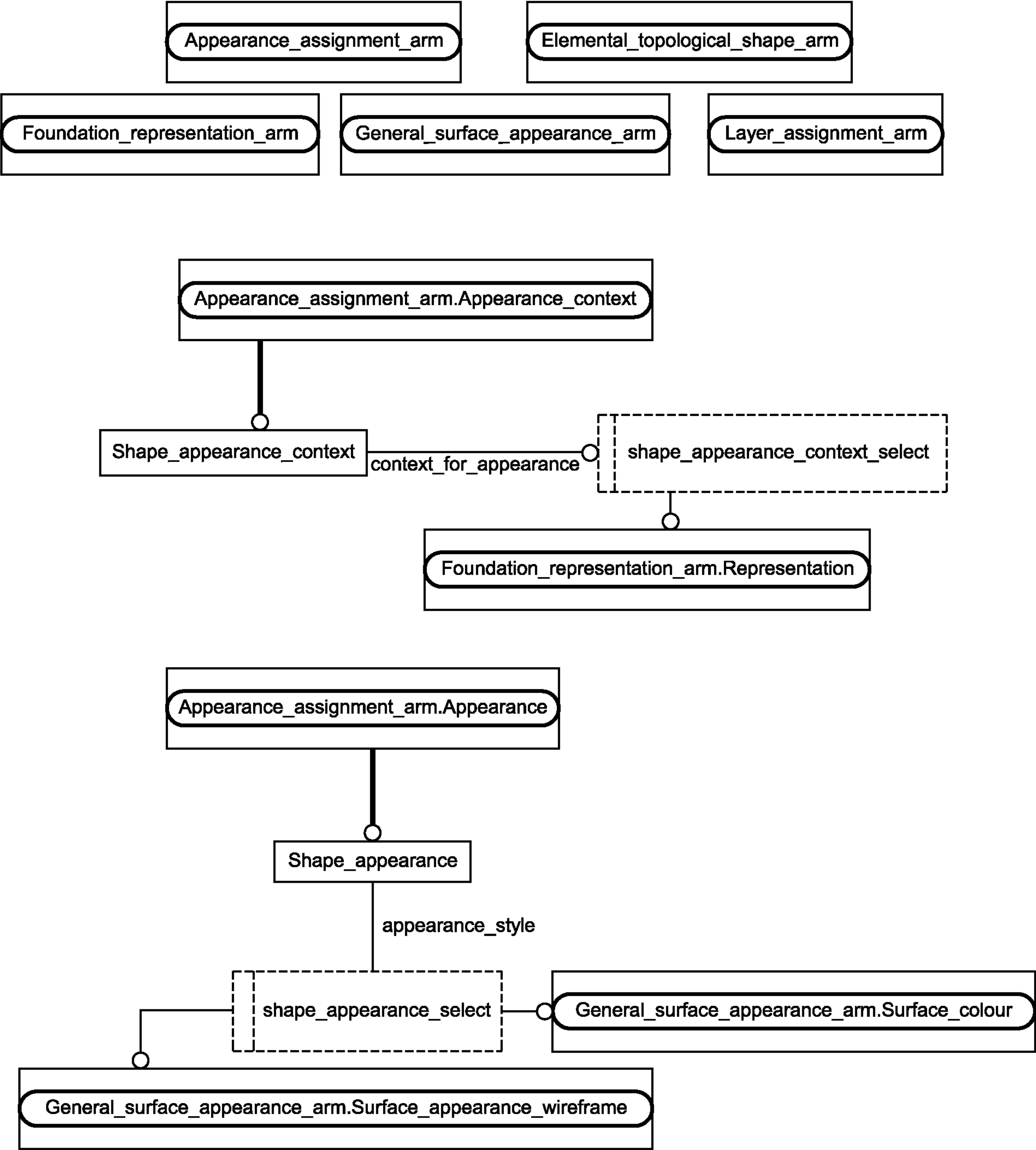
Рисунок С.1 — EXPRESS-G диаграмма ПЭМ
