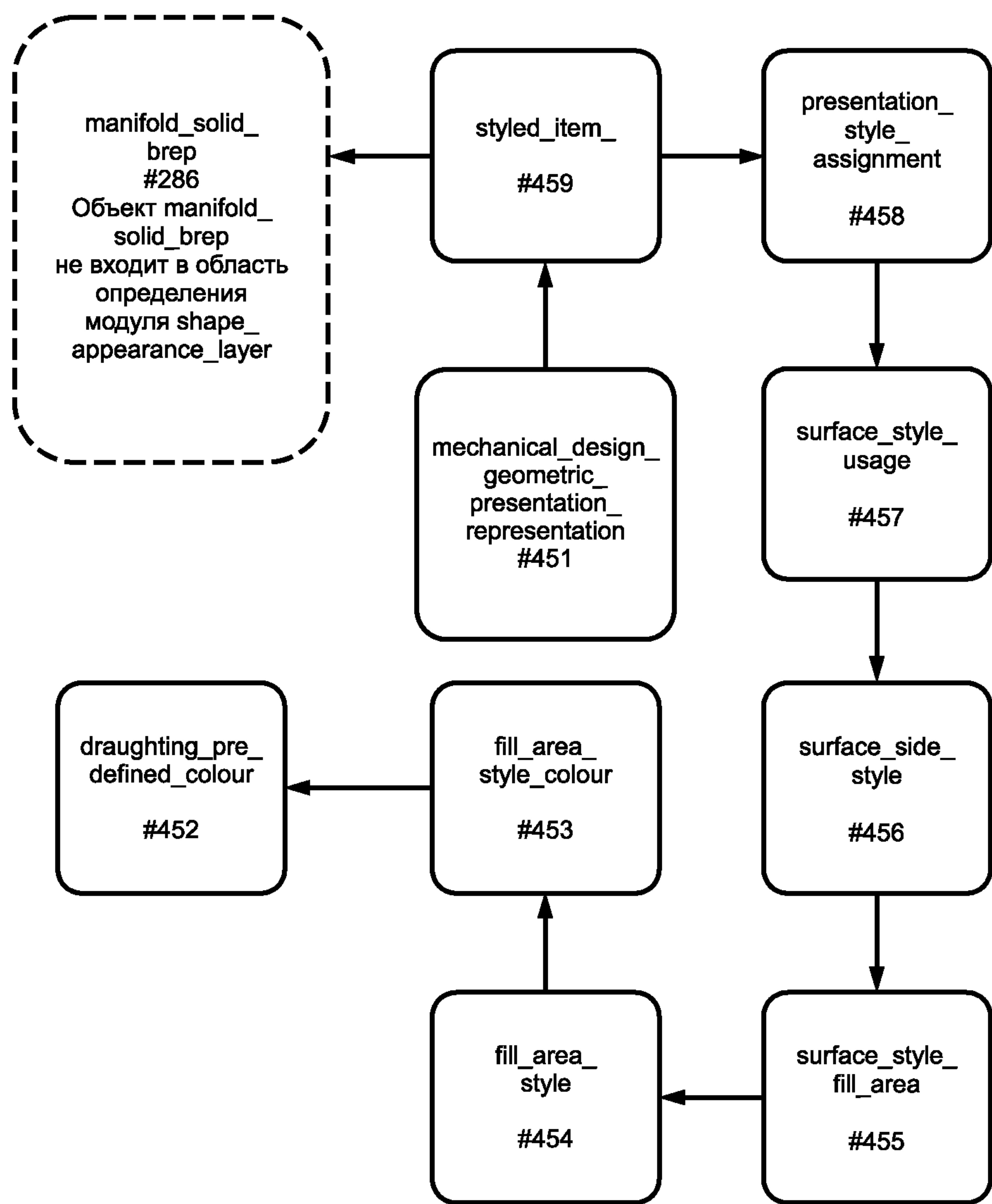
Рисунок F.4 — Задание цвета геометрической модели
