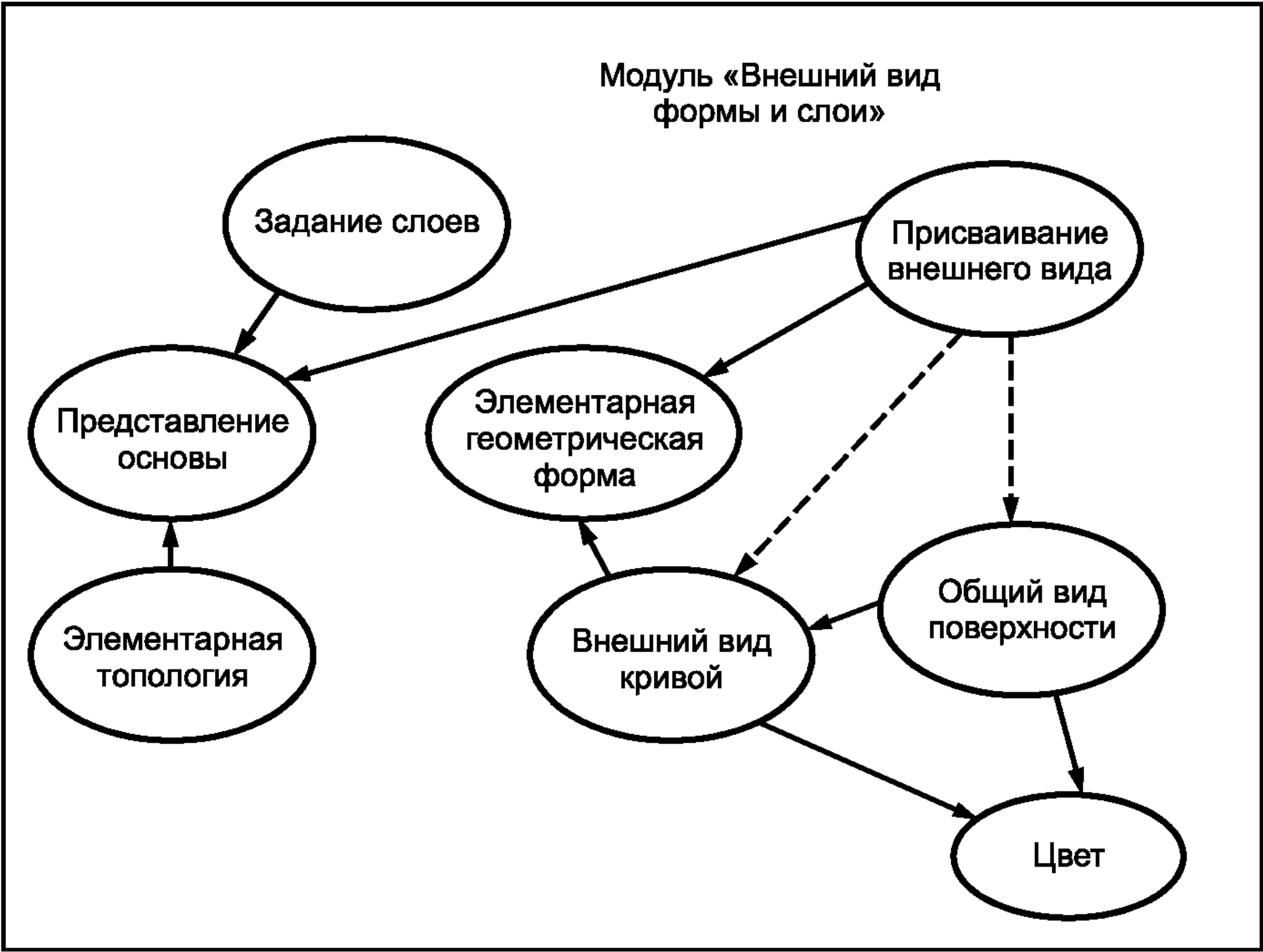
Рисунок F.1 — Связи прикладного модуля Shape_appearance_layer
