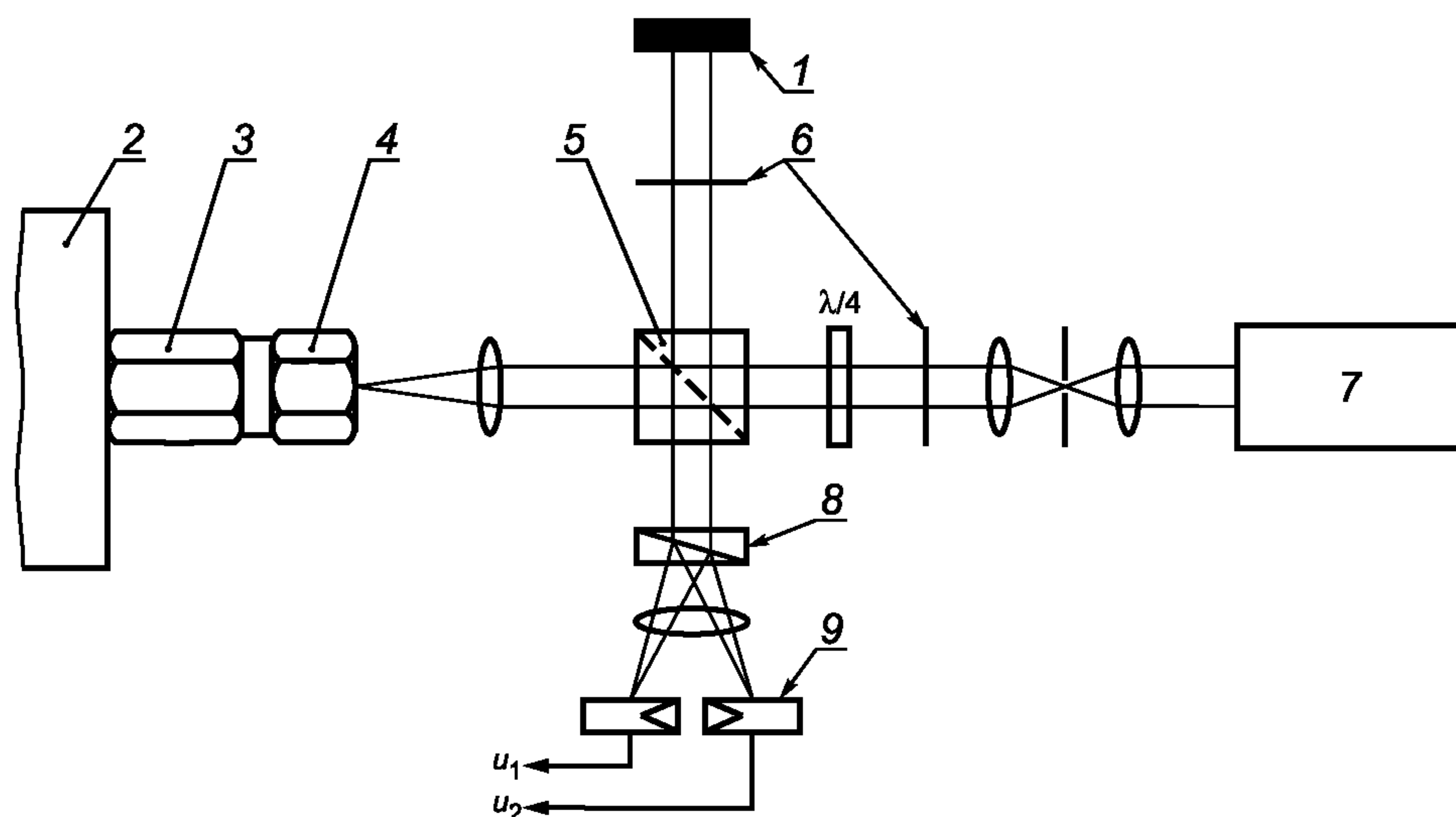
1 — опорное зеркало; 2 — подвижная система вибростенда; 3 — акселерометр; 4 — имитатор; 5 — светодетектор; 6 — поляризатор; 7 — лазер; 8 — призма Волластона; 9 — фотодетекторы
