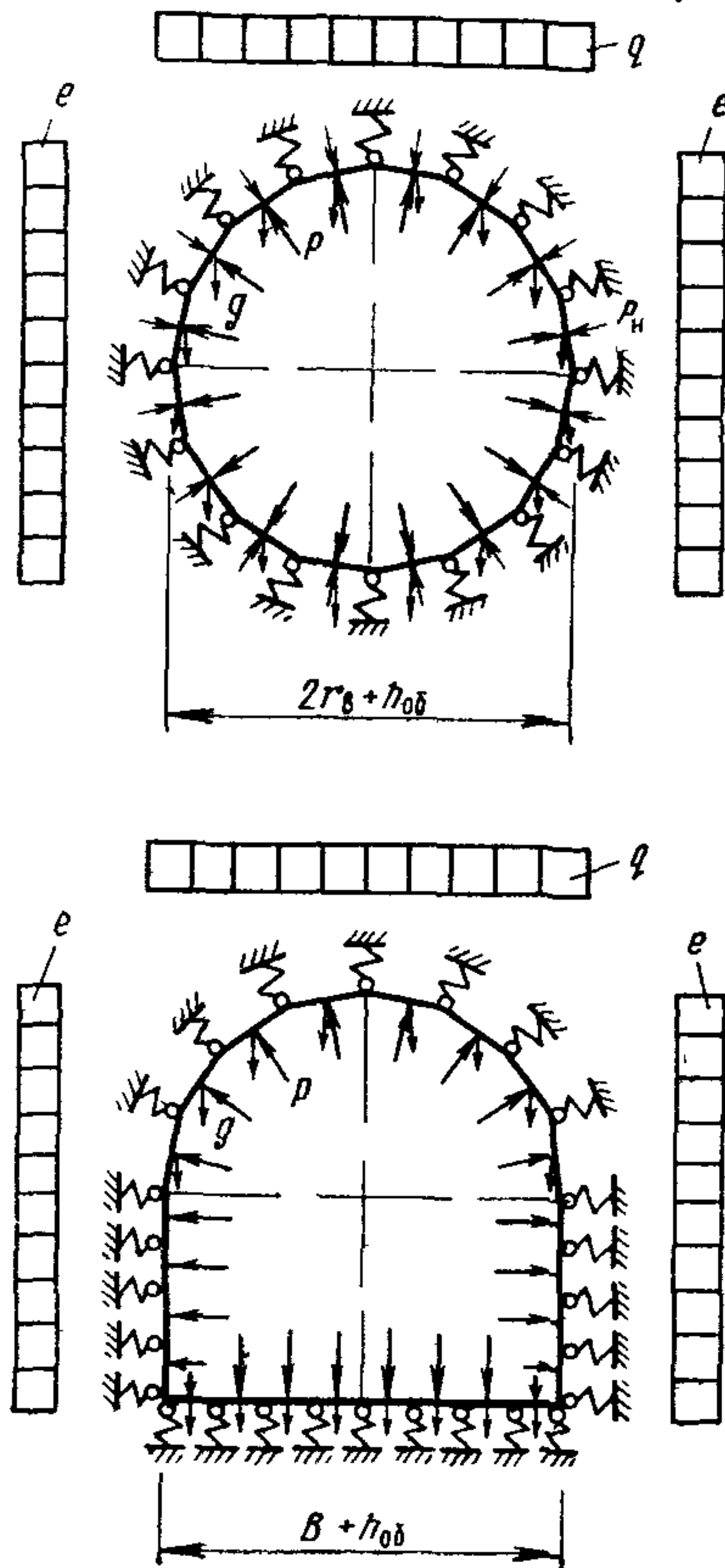
Рис. 3. Расчетные схемы обделок туннелей
