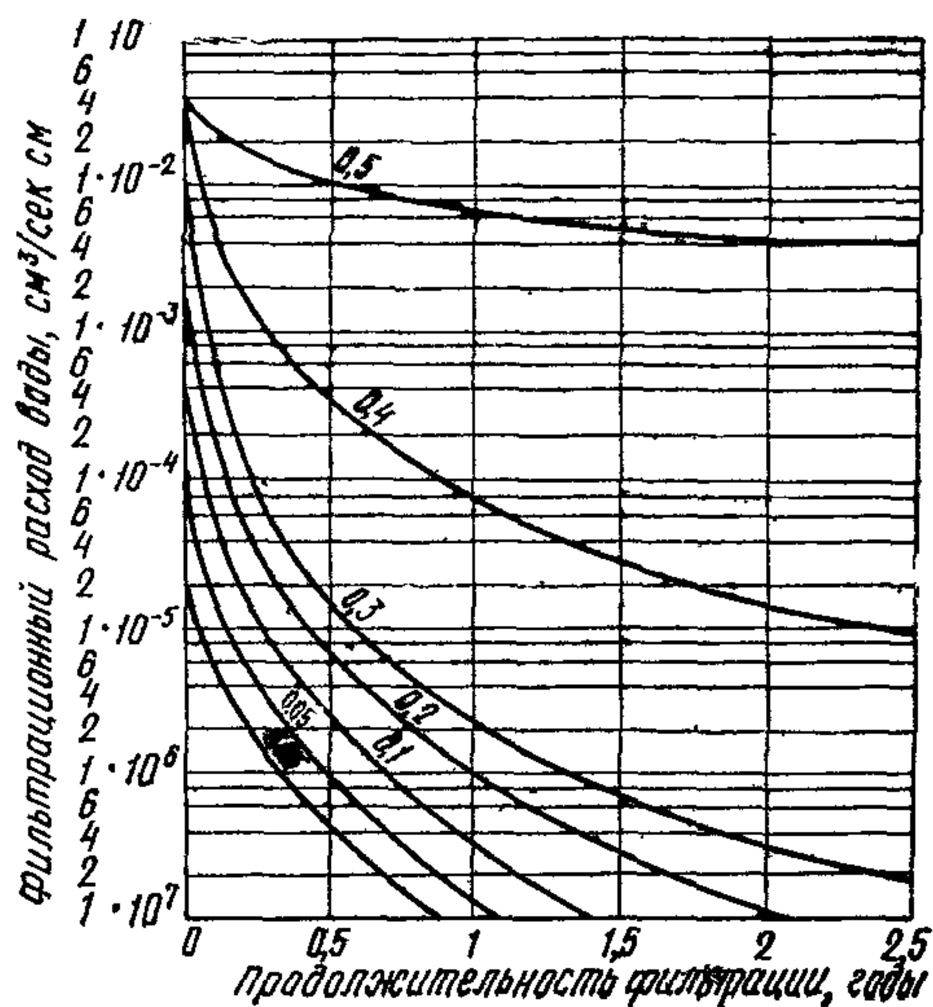
Рис. 5. Расчетные кривые самоуплотнения трещин в бетоне (цифрами у кривых обозначены величины раскрытия трещин в мм)
