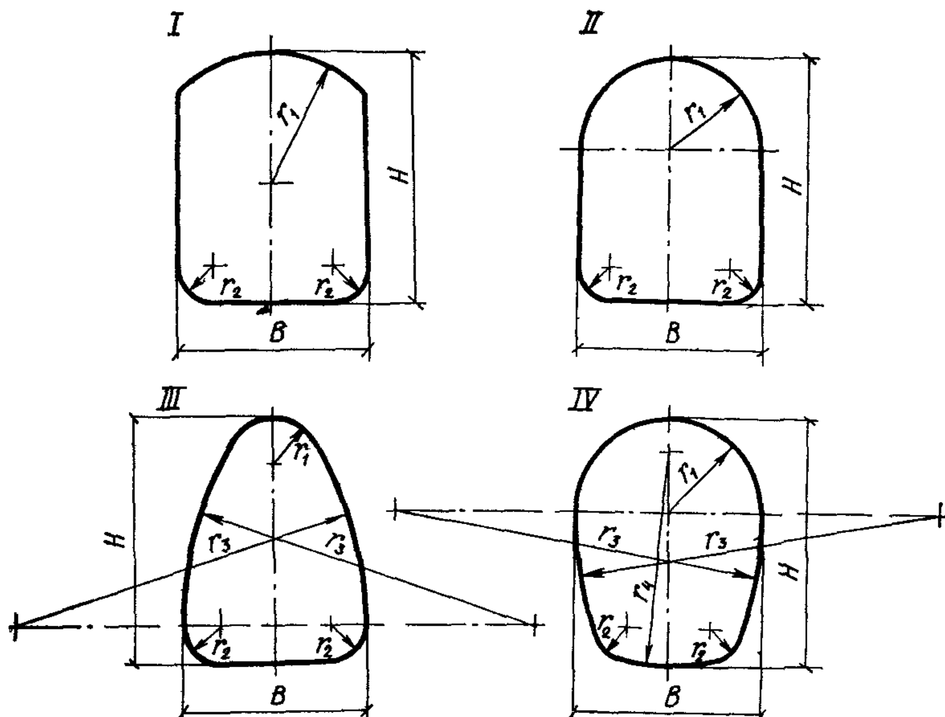
Рис 4. Поперечные сечения туннелей в свету
