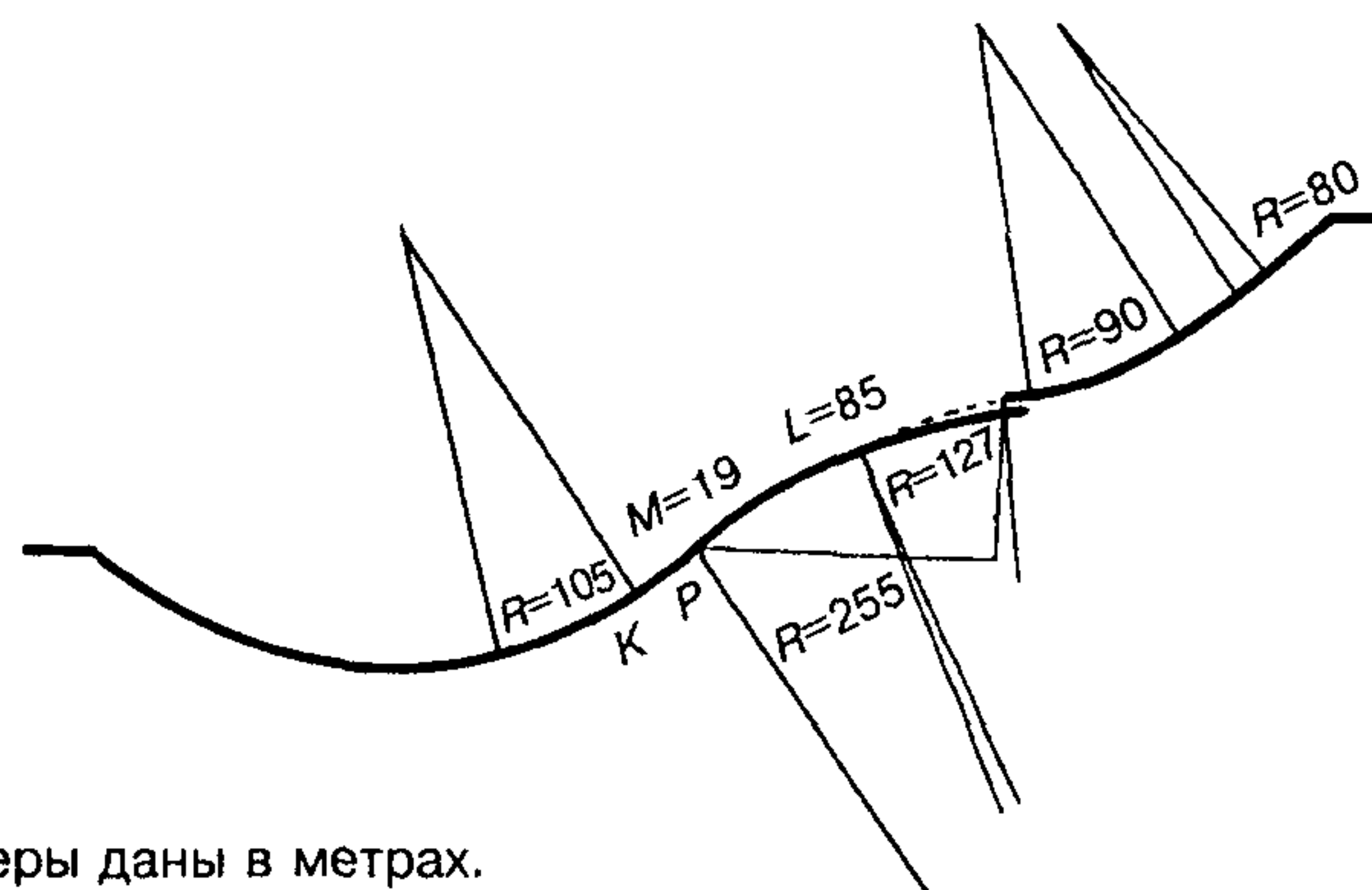
Профиль трамплина
