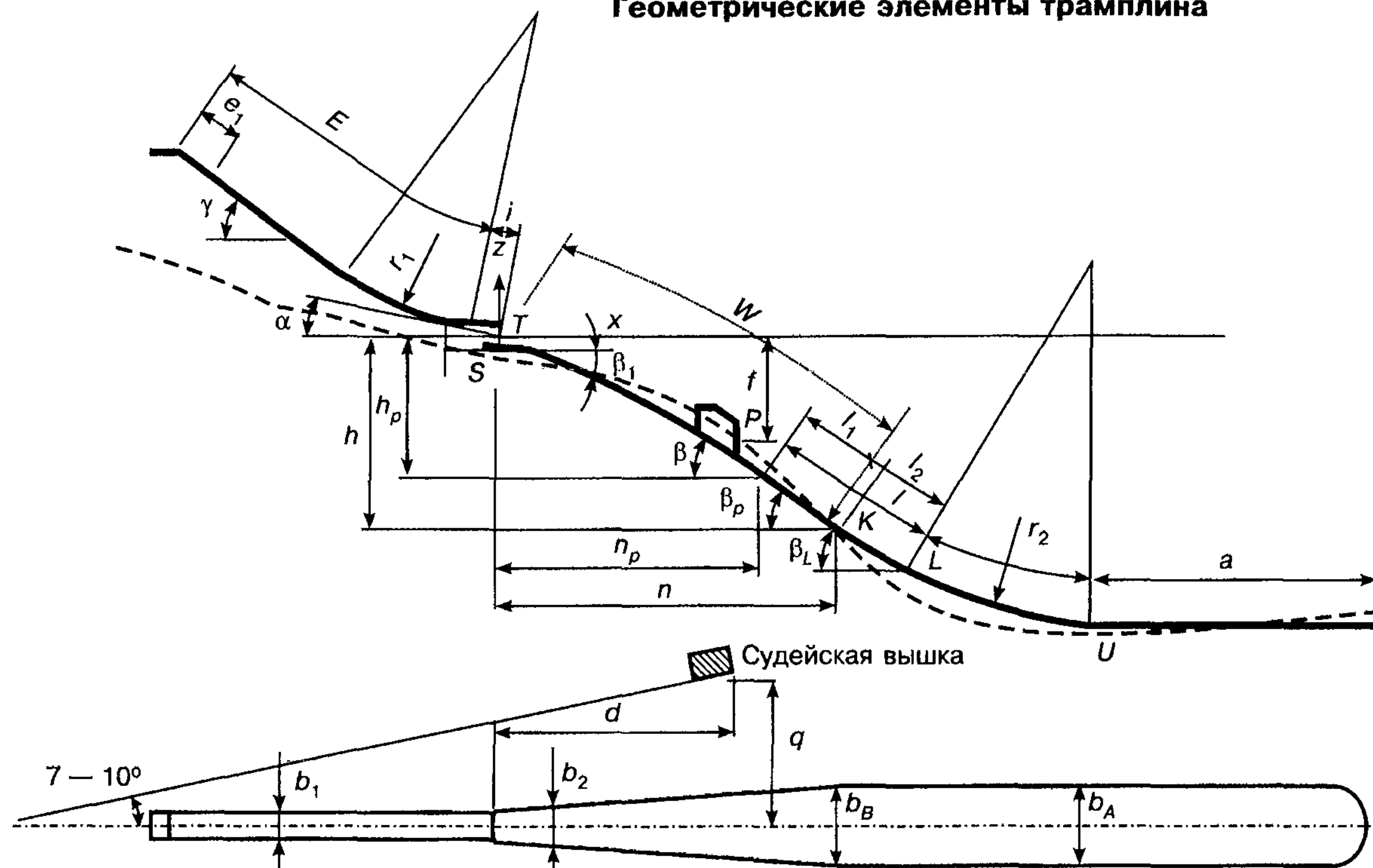
Геометрические элементы трамплина
