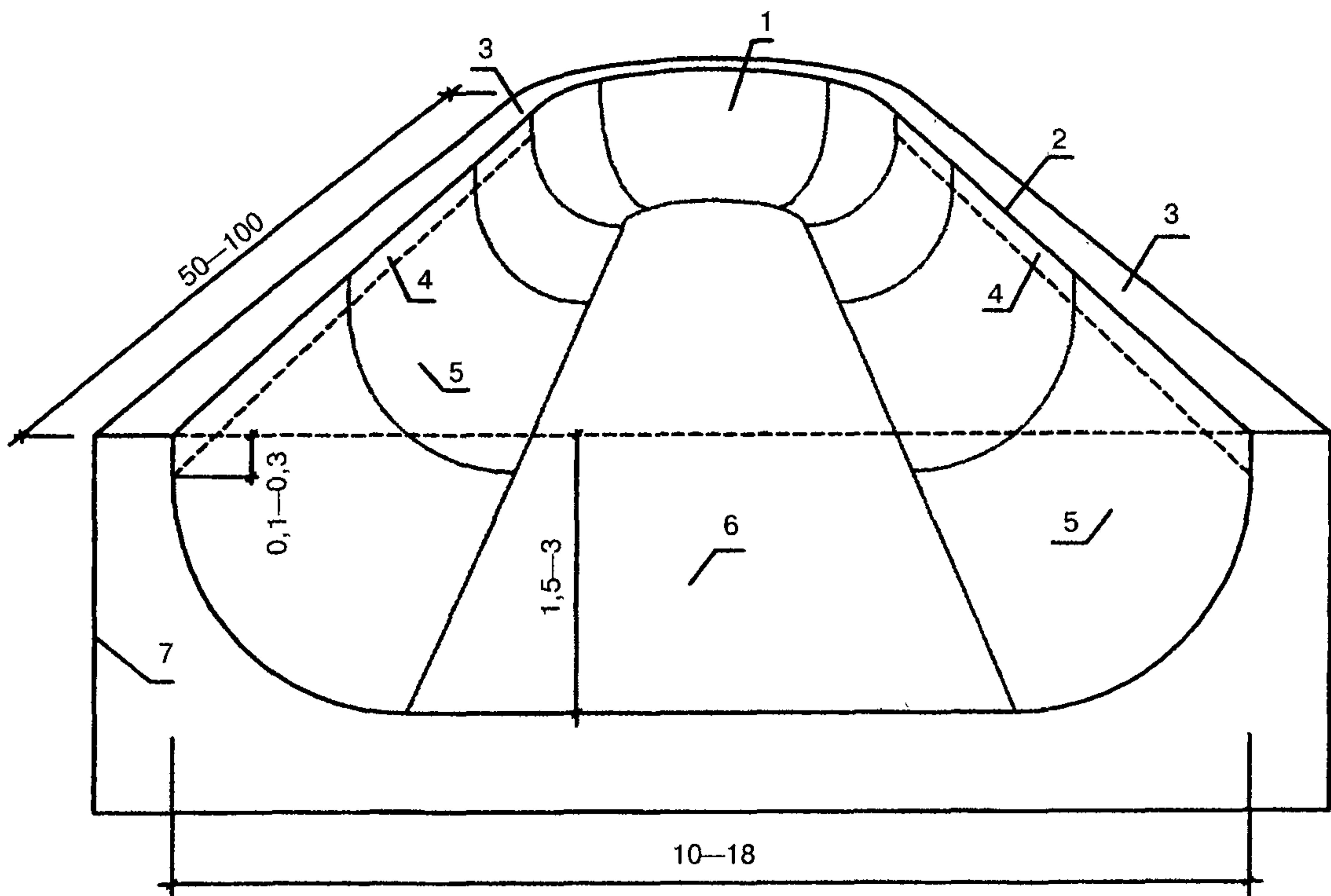
Б. ТРАДИЦИОННАЯ ТРУБА
