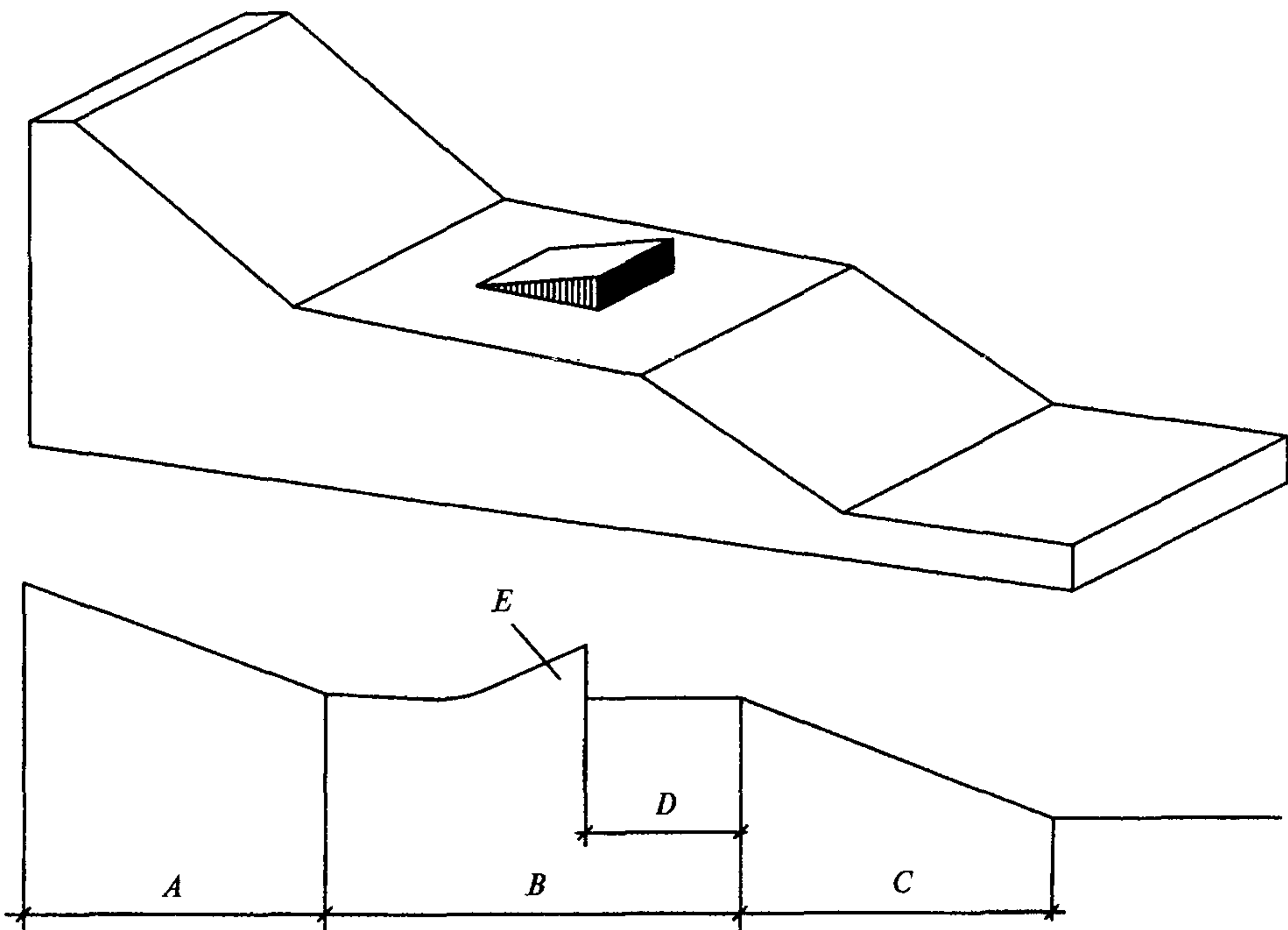
А. СХЕМА СКЛОНА ДЛЯ ЛЫЖНОЙ АКРОБАТИКИ
