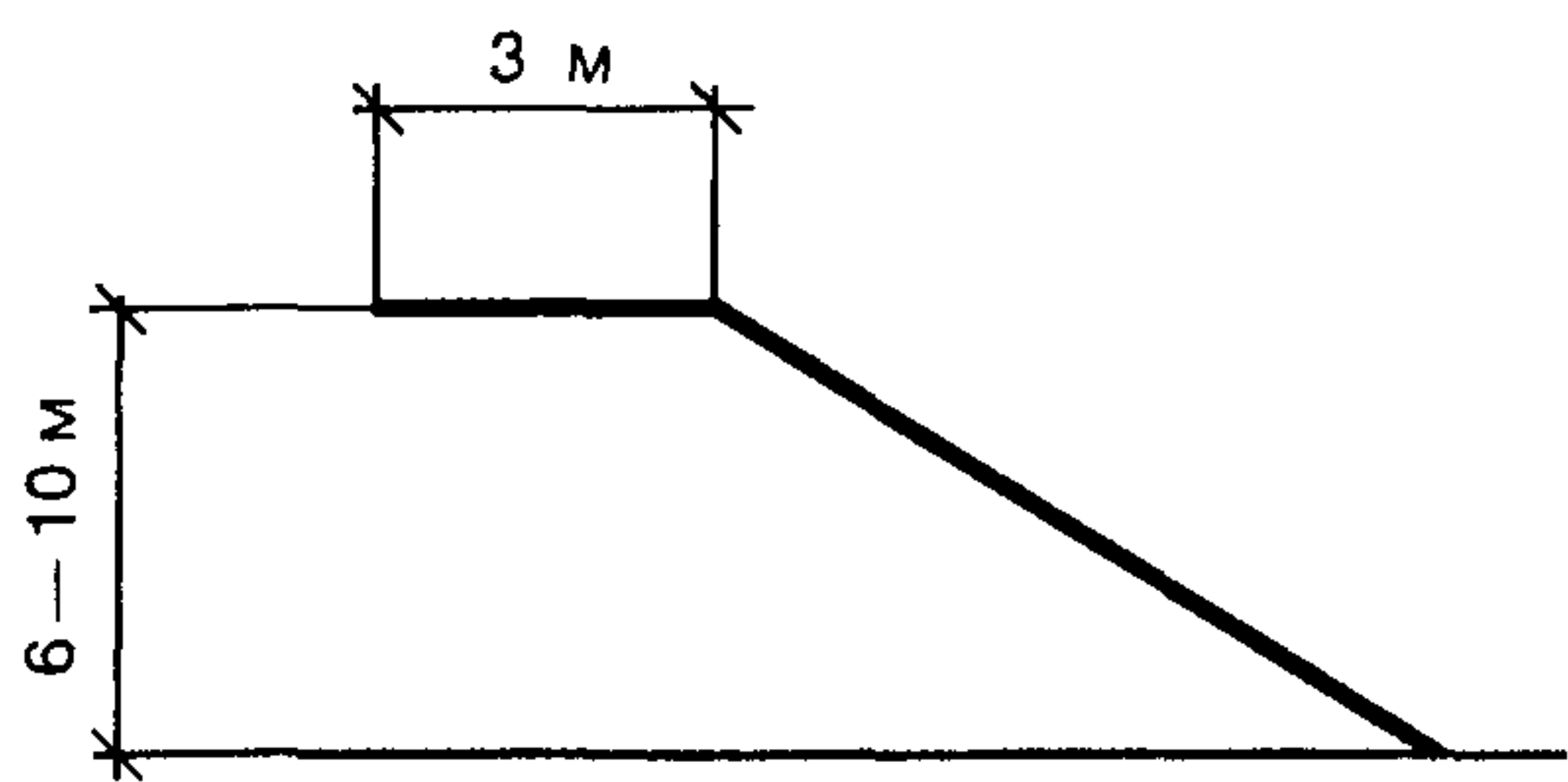
Профиль зоны
