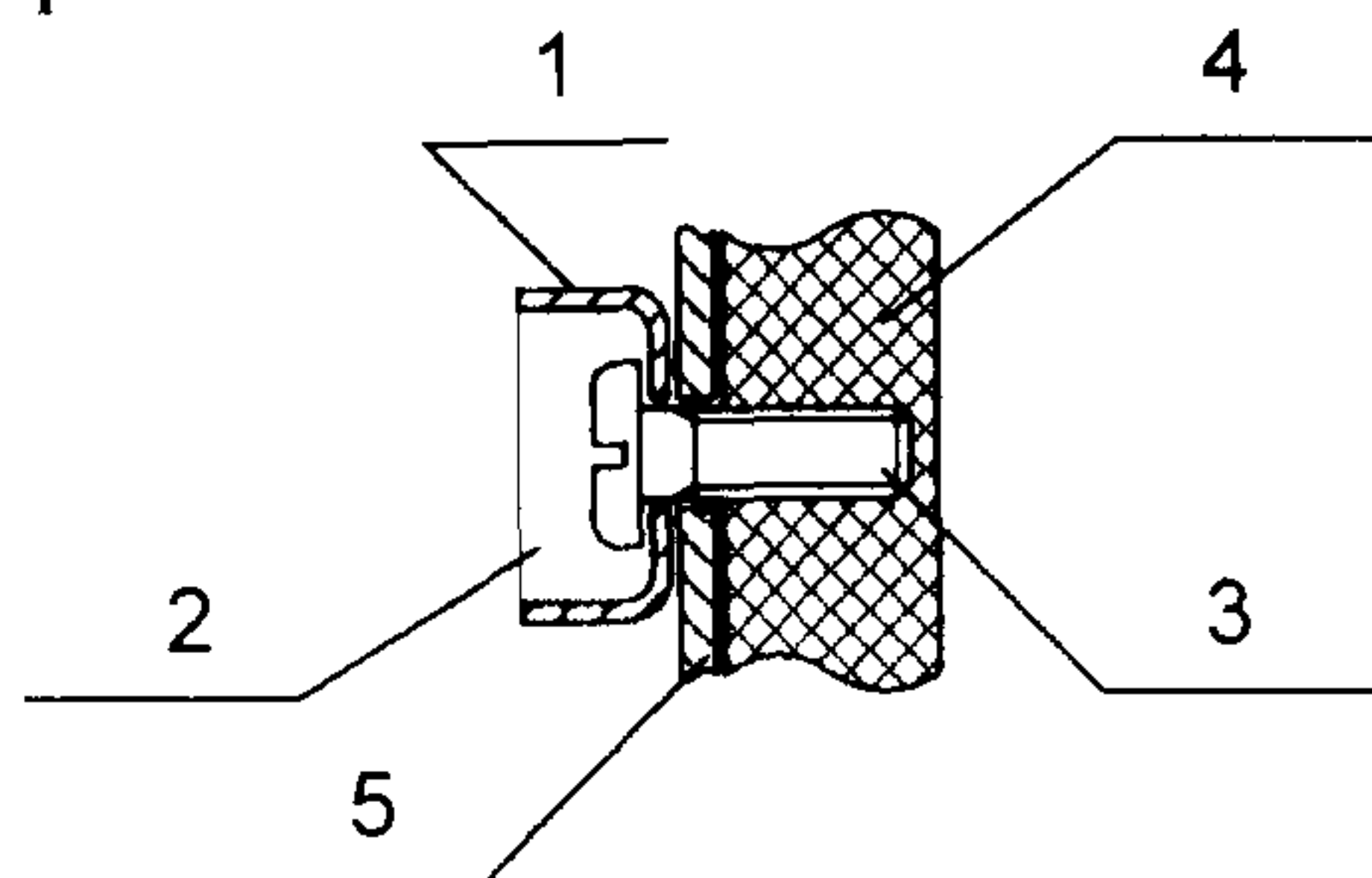
Вариант 1 пломбирования
