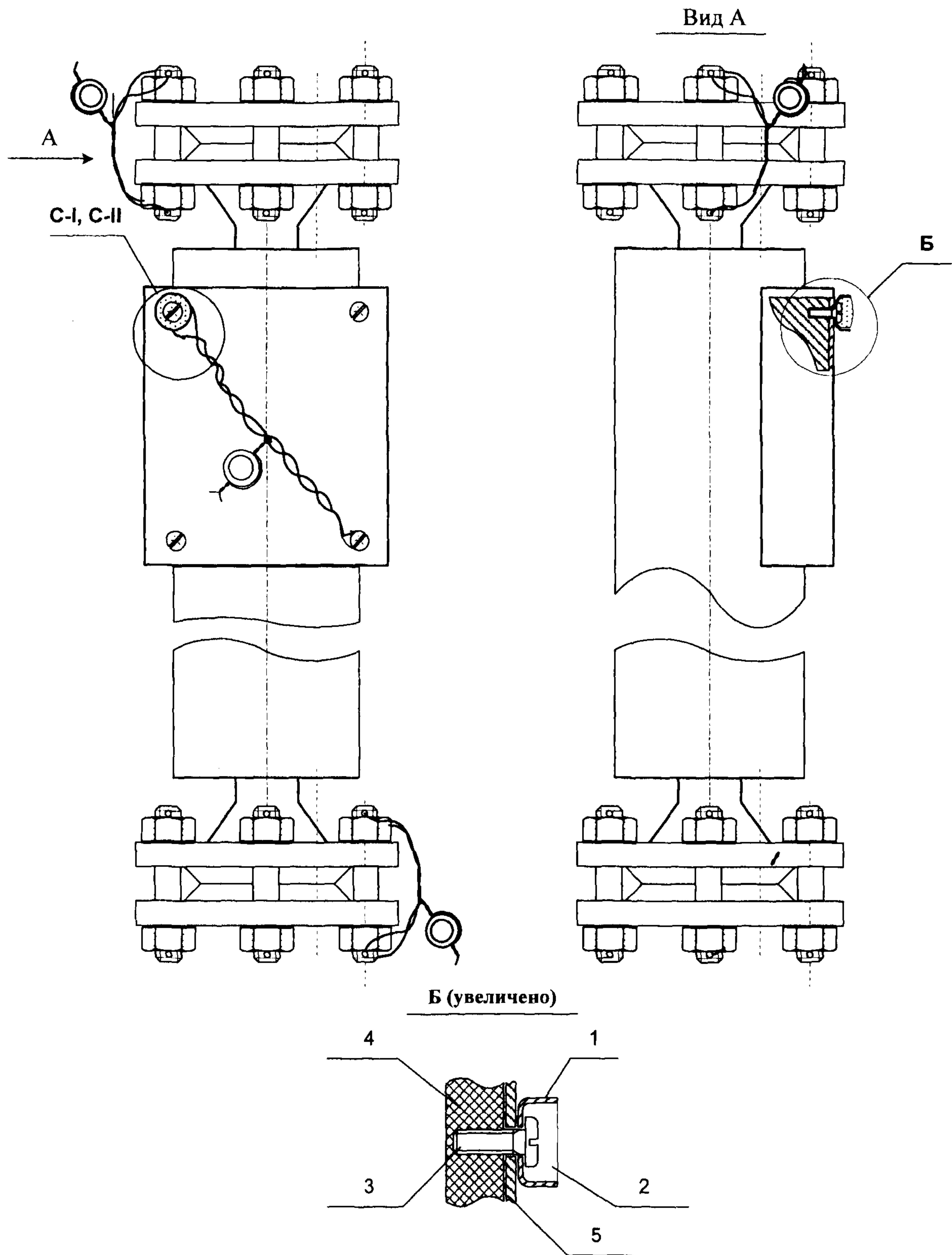
Рисунок Б.30 – Преобразователь плотности жидкости измерительный модели 7835 фирмы «Solatron Mobrey Limited»
