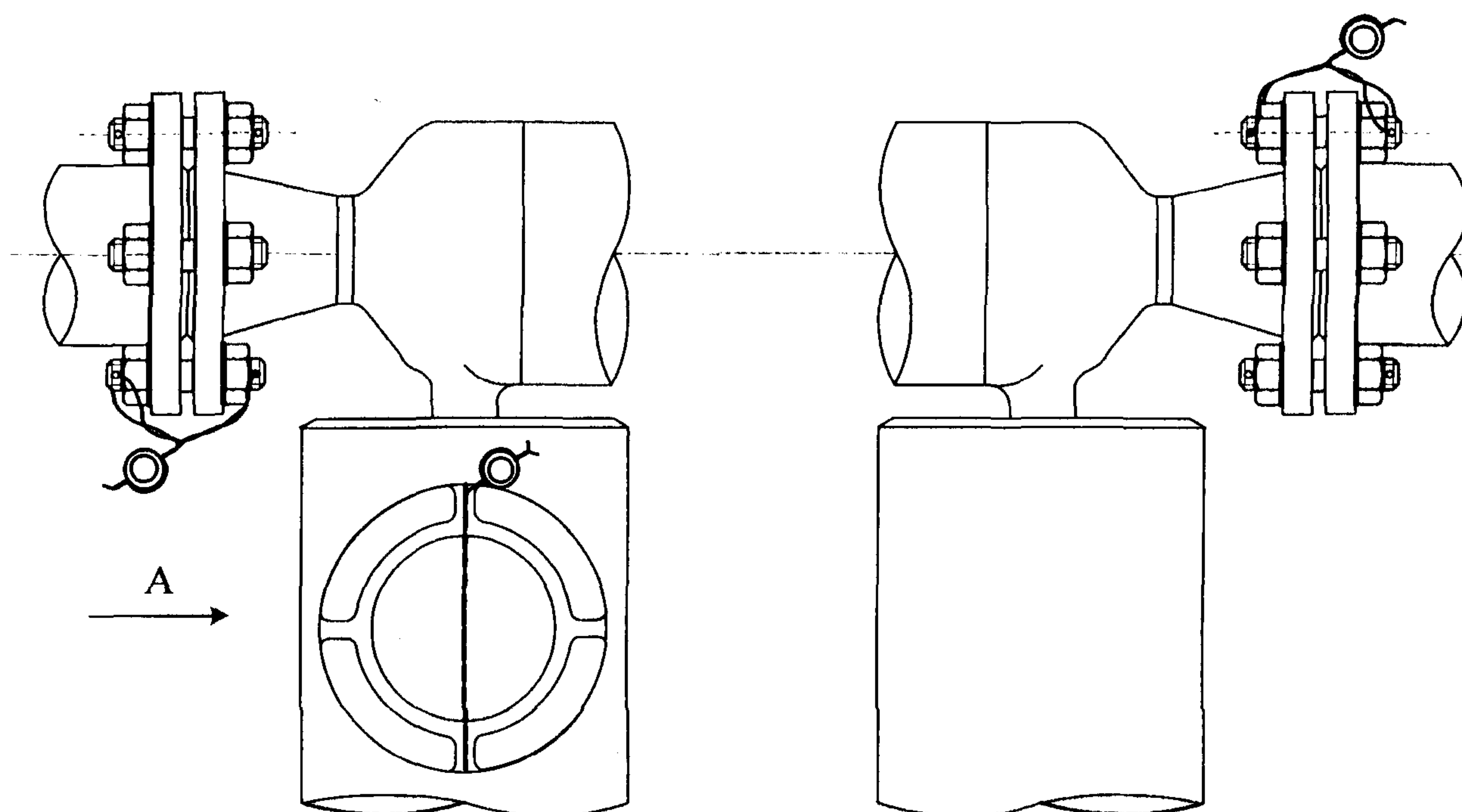
Вид А
