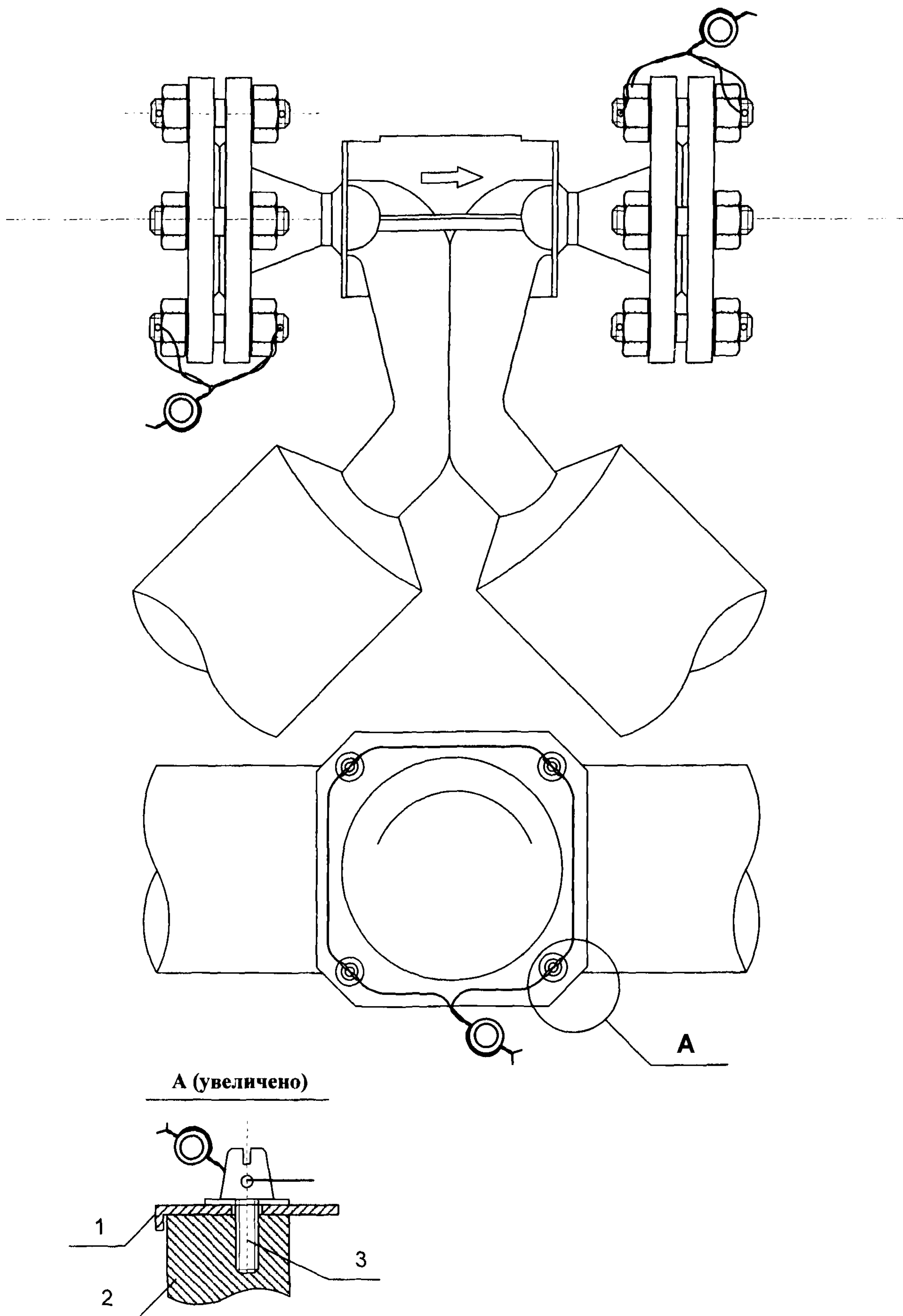
Рисунок Б.5 – Счетчик-расходомер массовый Micro Motion модель CMF 025 (050, 100) серии Elite, выполненный с соединительной коробкой, фирмы «Emerson Process Management, Fisher-Rosemount»
