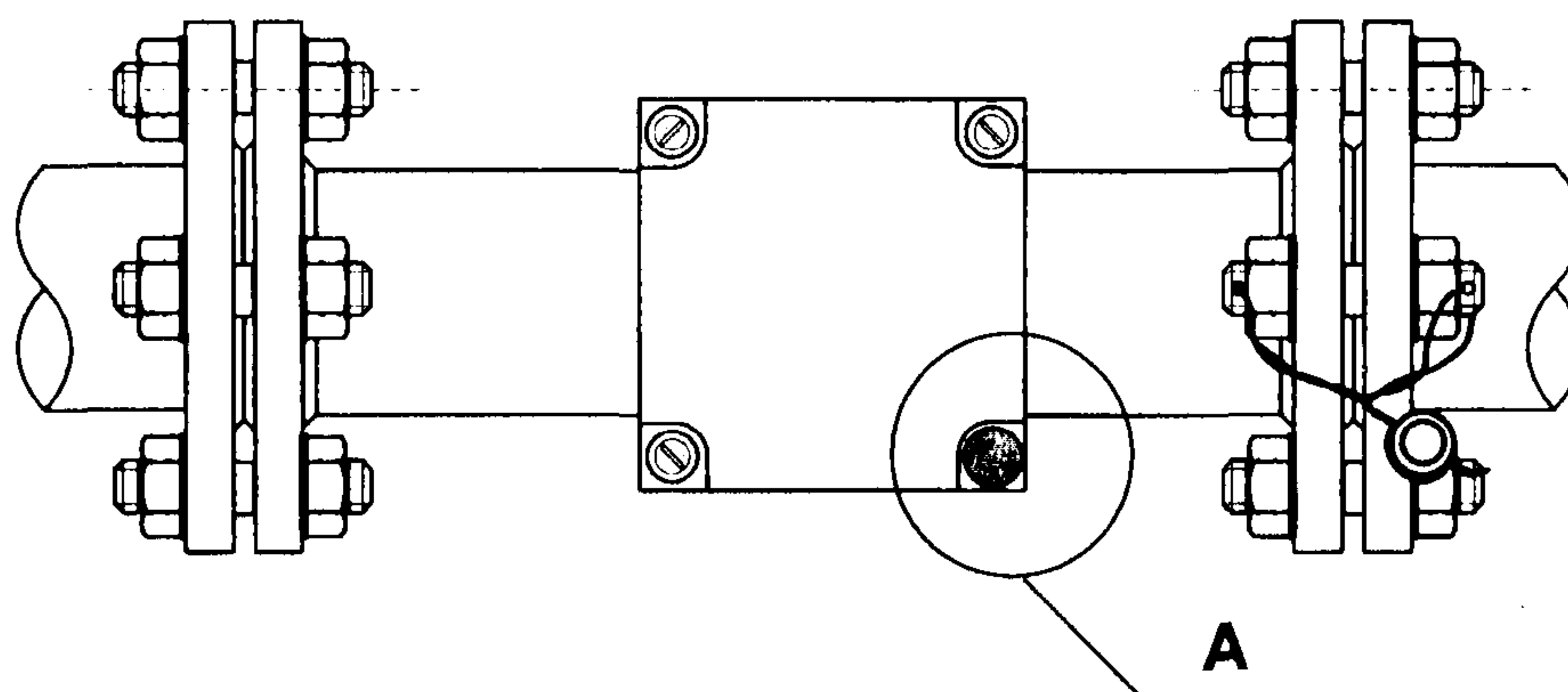
Вид А
