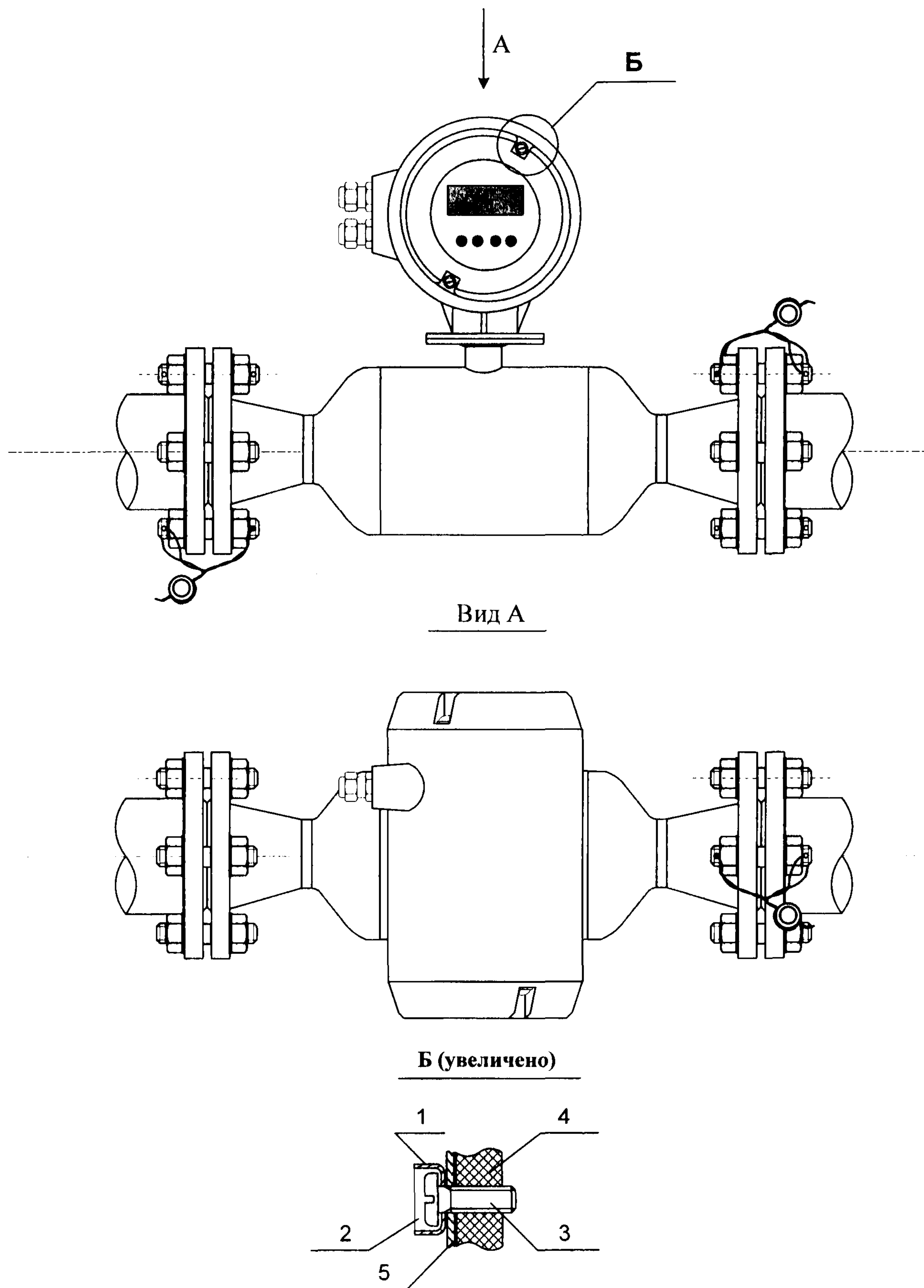
Рисунок Б.3 – Счетчик ультразвуковой серии UFM с вторичным преобразователем UFC 500F производства «КРОНЕ-Автоматика»
