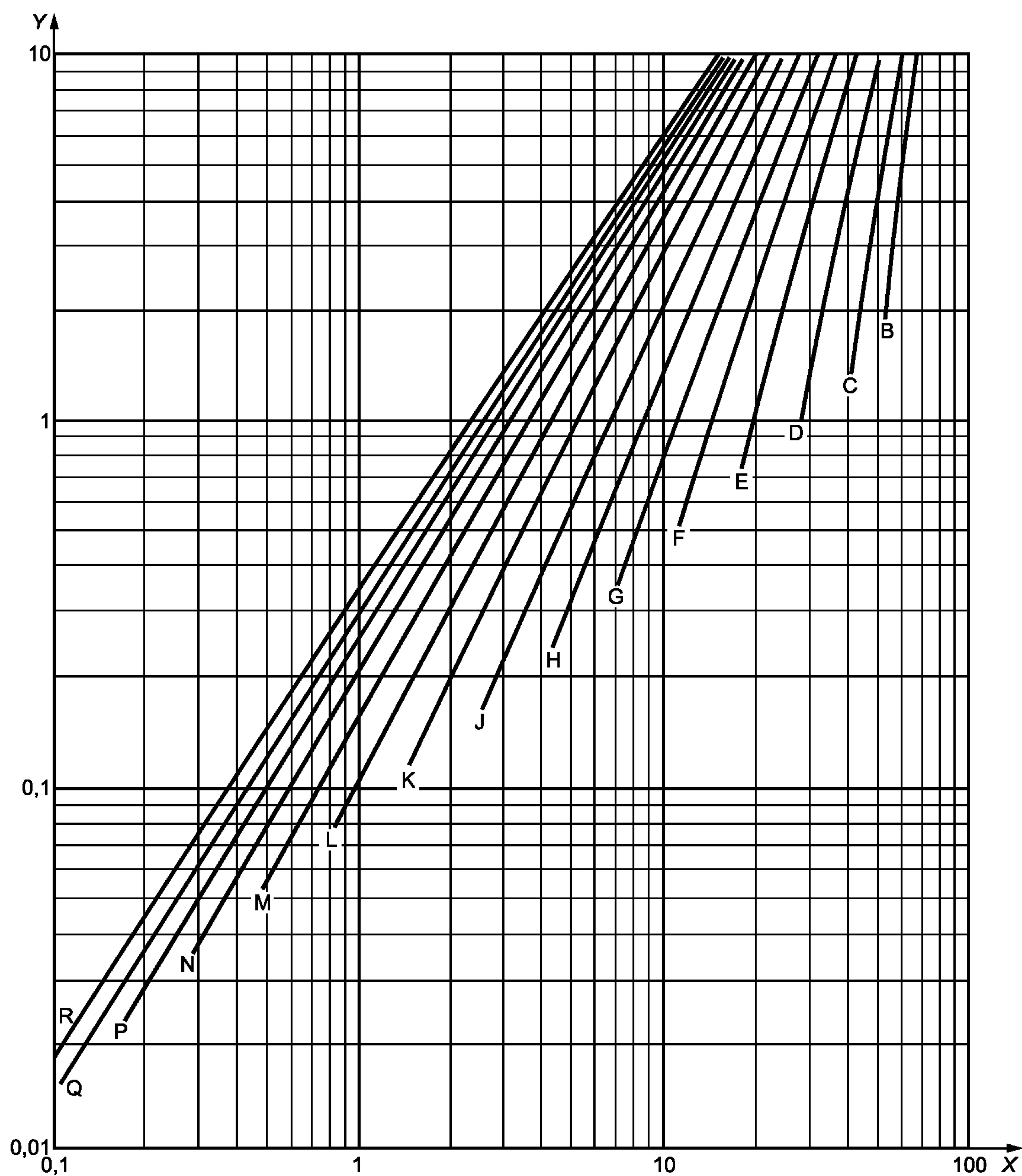
X — предельный уровень качества, т. е. уровень несоответствий, соответствующий вероятности приемки 10 % в виде процента несоответствующих единиц продукции; Y — уровень несоответствий в процентах несоответствующих единиц продукции, соответствующий вероятности приемки 95 %; Коды объема выборки показаны полужирным шрифтом.
