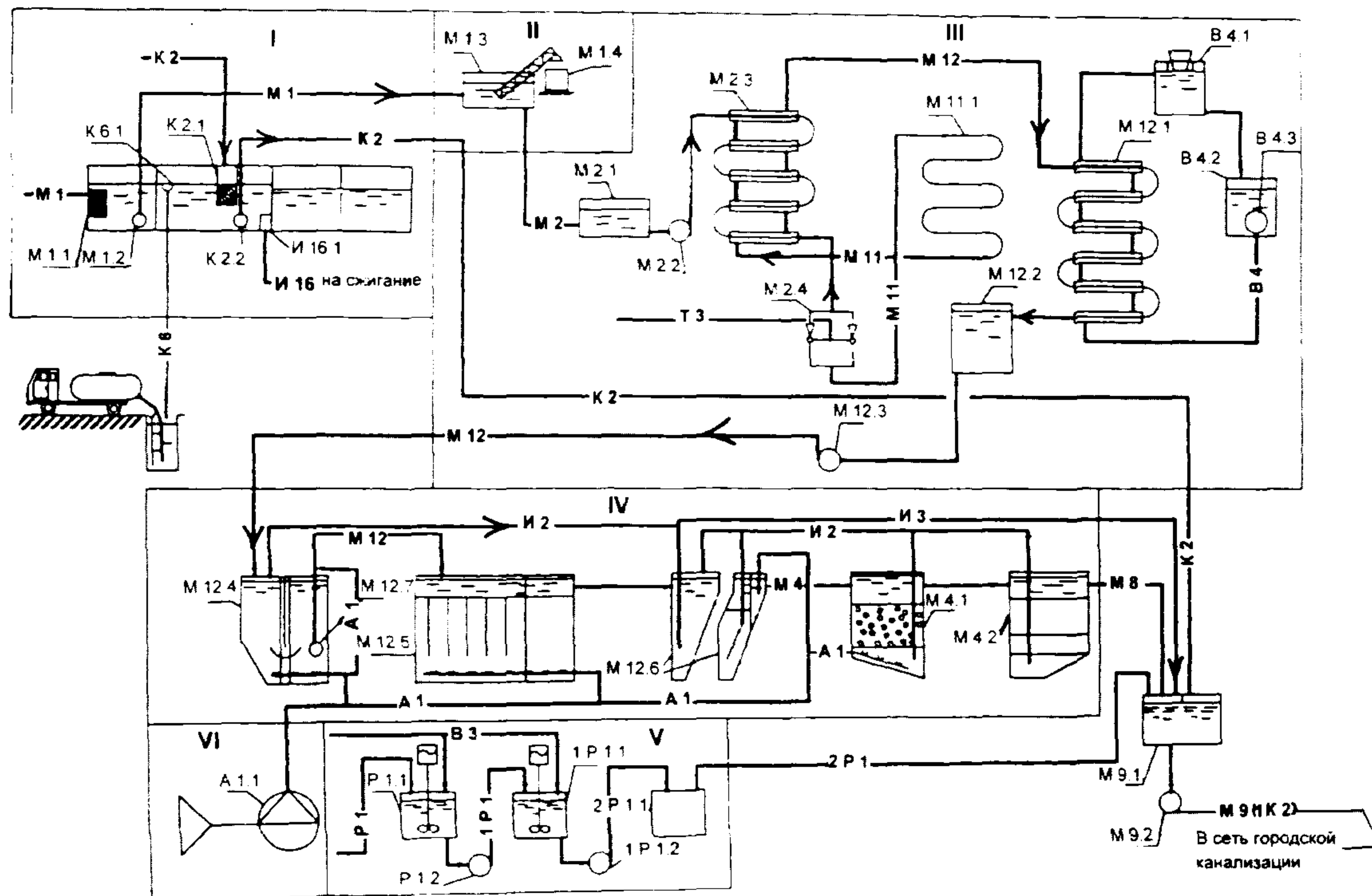
Рис. В.1 – Технологическая схема очистки сточных вод
