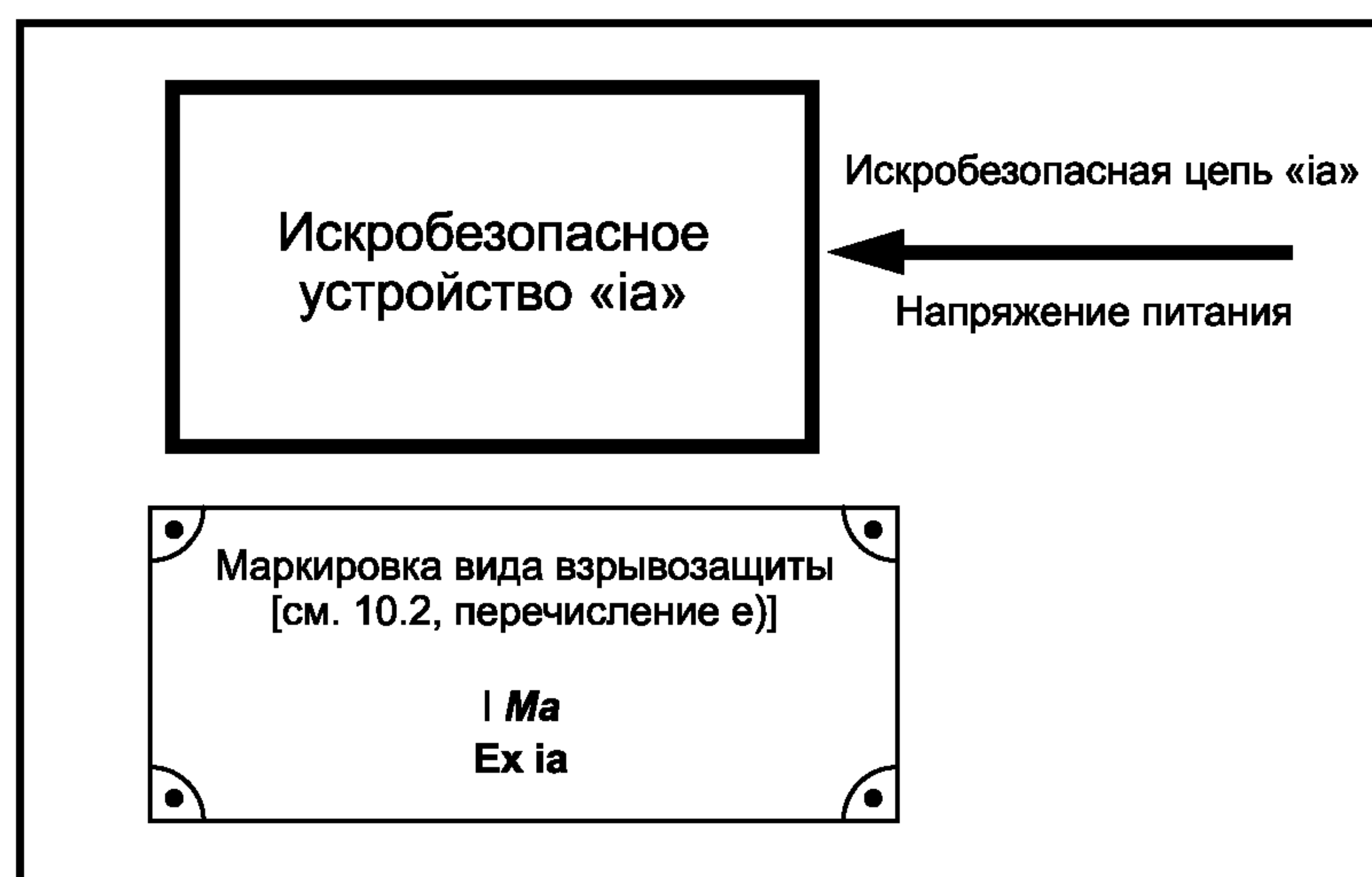
Рисунок 1 — Оборудование уровня взрывозащиты Ma (искробезопасная цепь «ia»)
