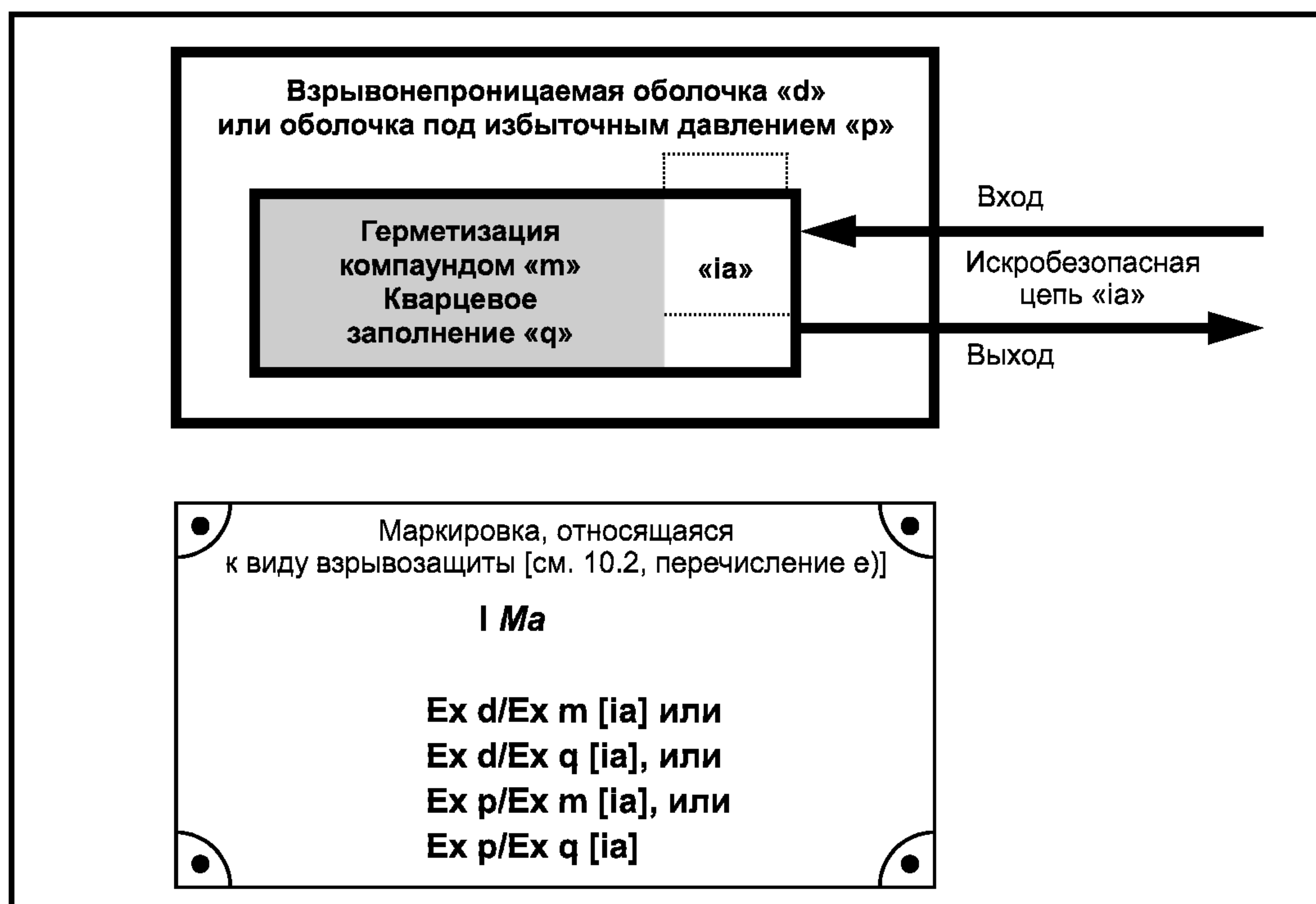
Рисунок 3 — Оборудование уровня взрывозащиты Ma (герметизация компаундом «т» или кварцевое заполнение «q» внутри взрывонепроницаемой оболочки «d» или оболочки под избыточным давлением «р»)
