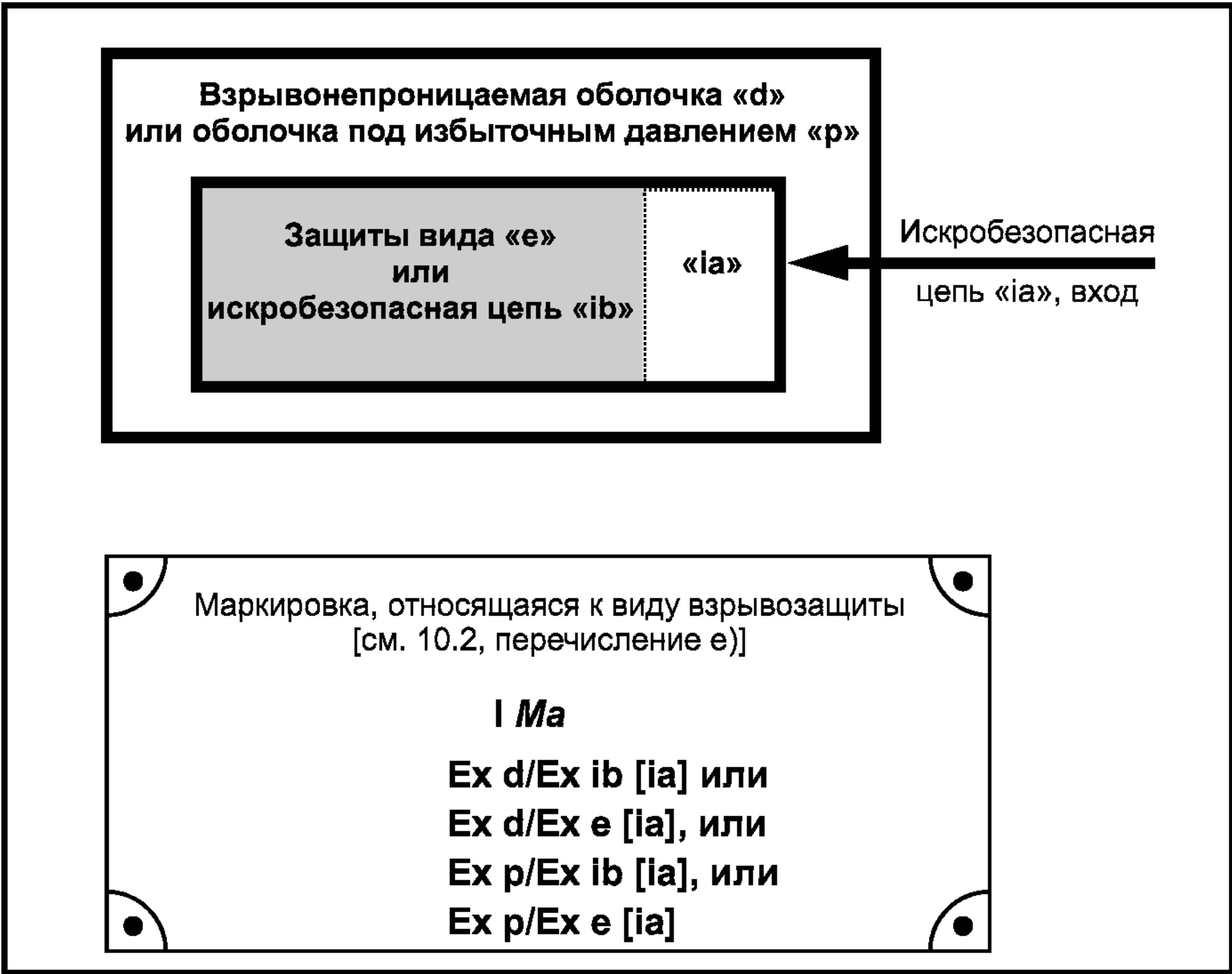
Рисунок 4 — Оборудование уровня взрывозащиты Ma (защита вида «е» или искробезопасная цепь «ib» внутри взрывонепроницаемой оболочки «d» или оболочки под избыточным давлением «р»)
