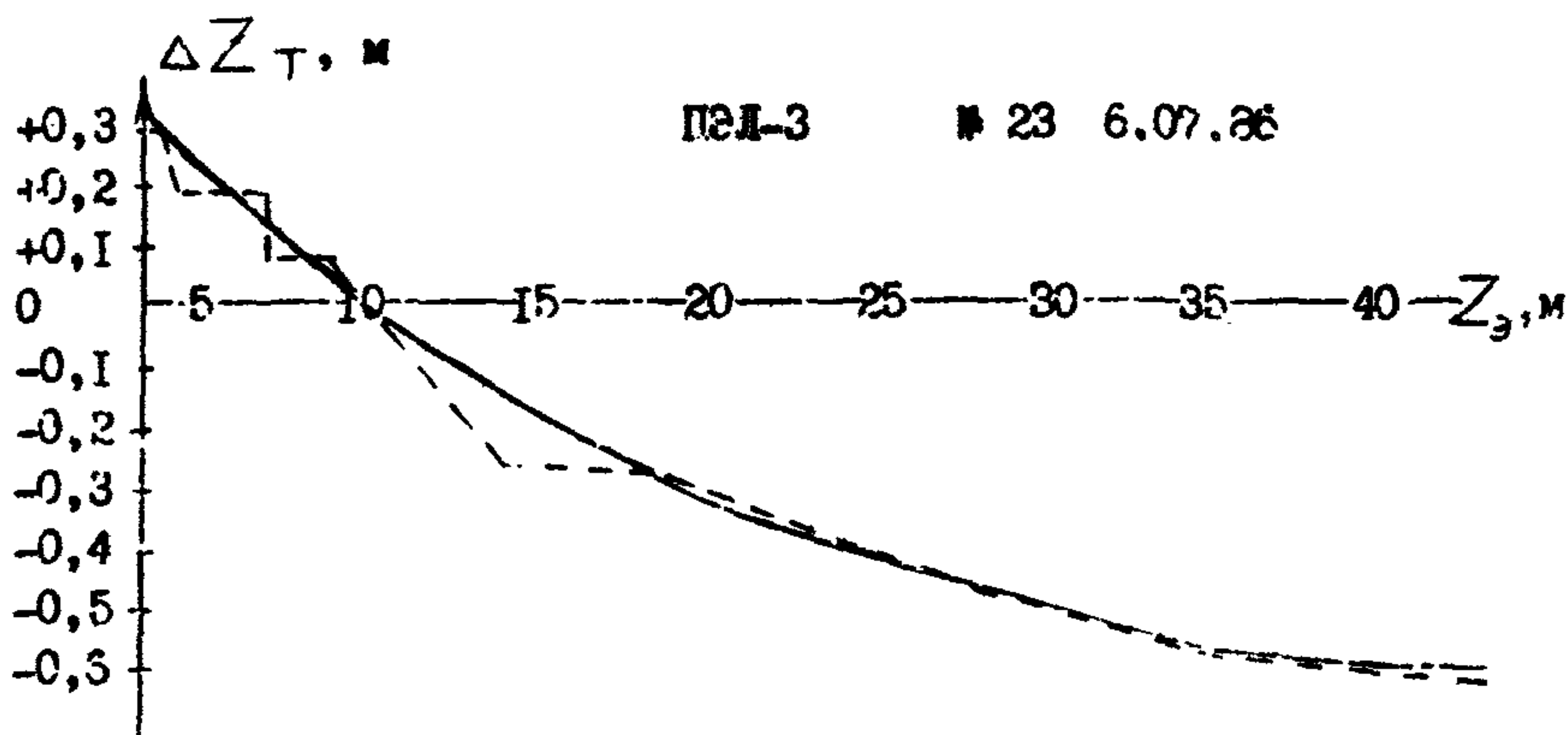
График тарирования эхолота
