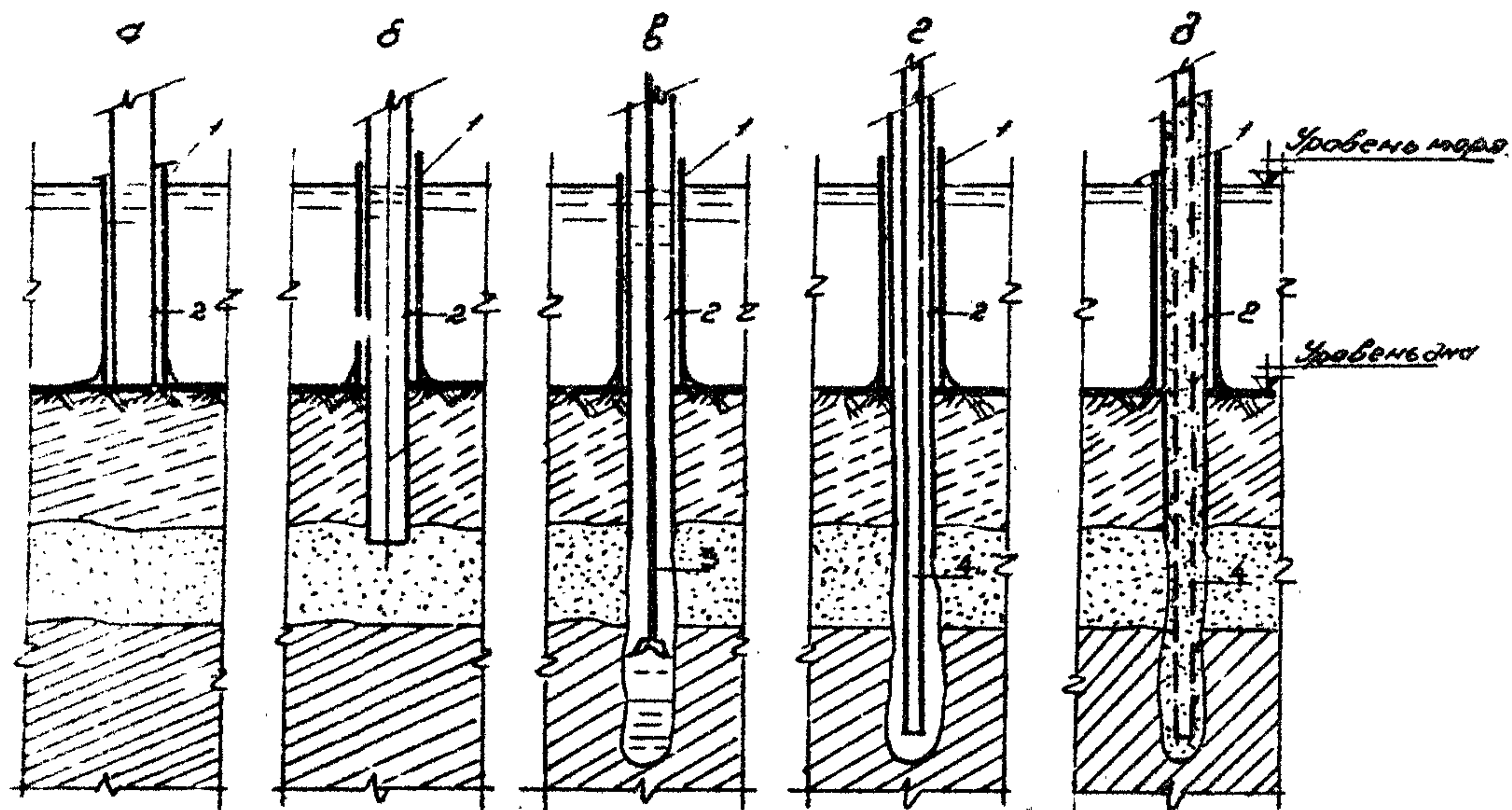
Рис. 5 схема устройства бурозаливной сваи
