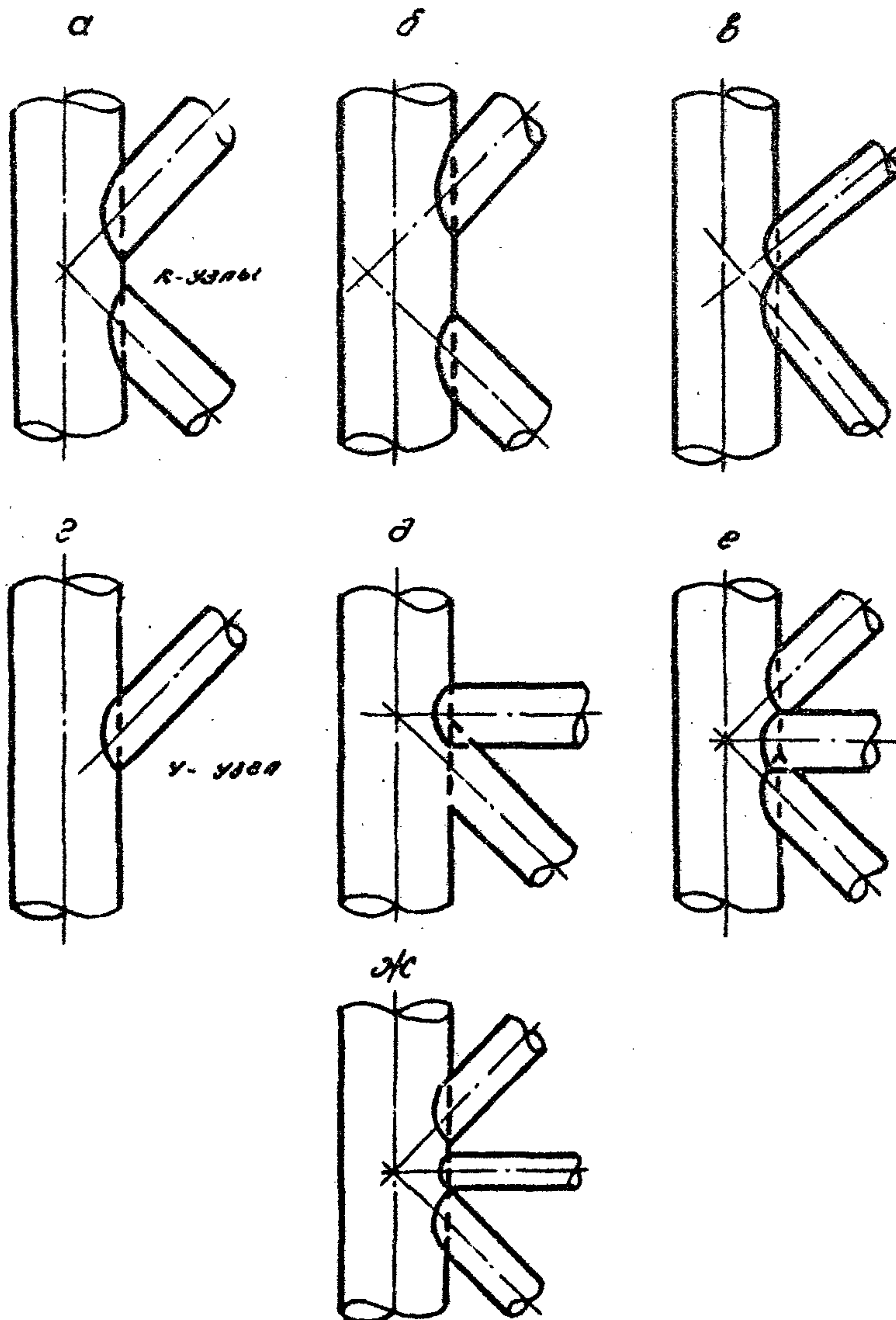
Рис. 3 Основные конструкции сесфазовочных узлов из труб
