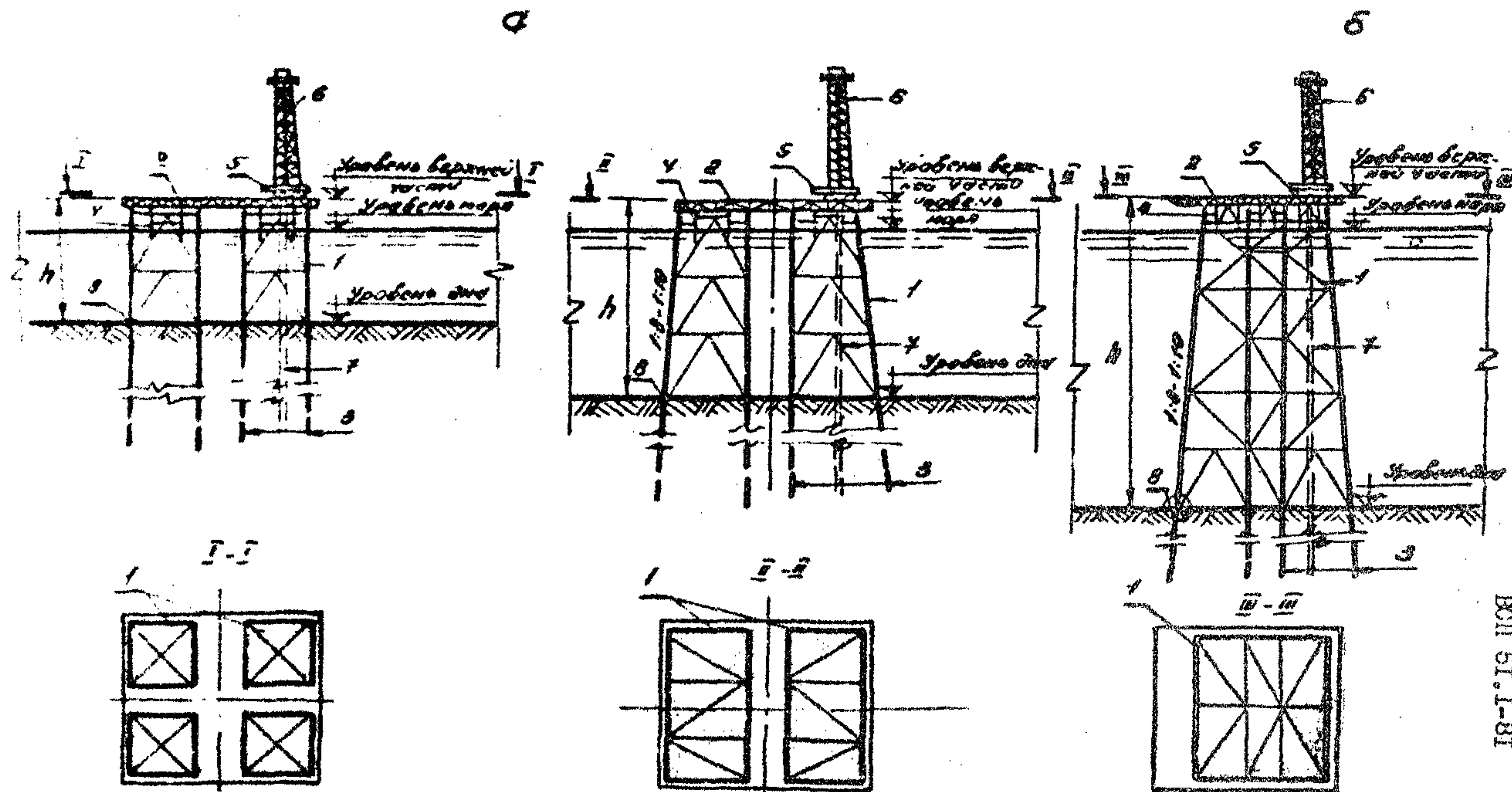
Рис. 1 Основные виды конструкций МНТС: а - многоблочные, б - одноблочные 1 - опорный блок, 2 - верхнее строение, 3 - свайный фундамент, 4 - причально-посадочное устройство, 5 - подрывные конструкции, 6 - буровая вышка, 7 - сбрасывающая колонна, 8 - опорный узел
