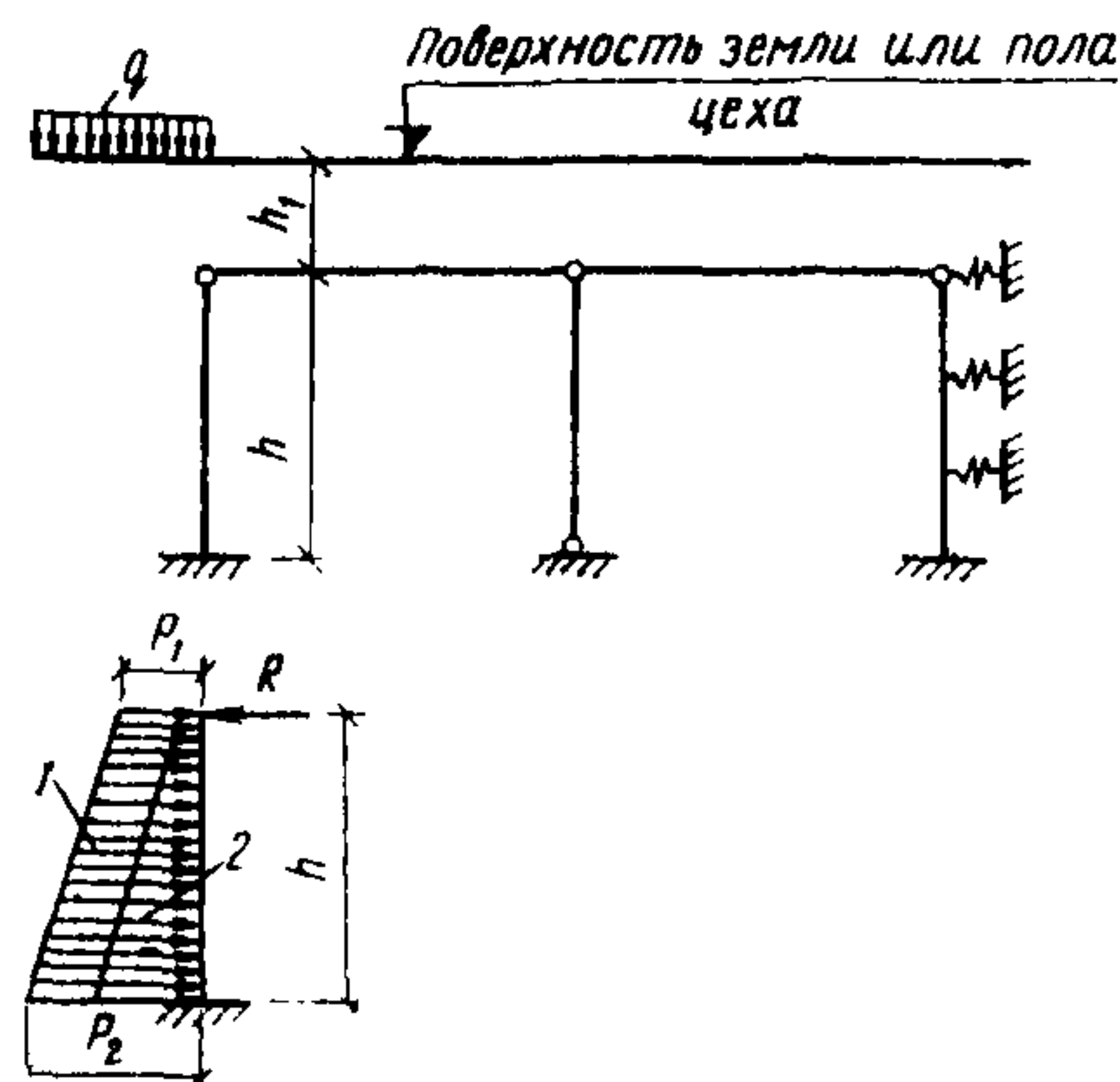
Рис. 1. Расчетная схема подвала при одностороннем загрузке временной вертикальной нагрузкой
