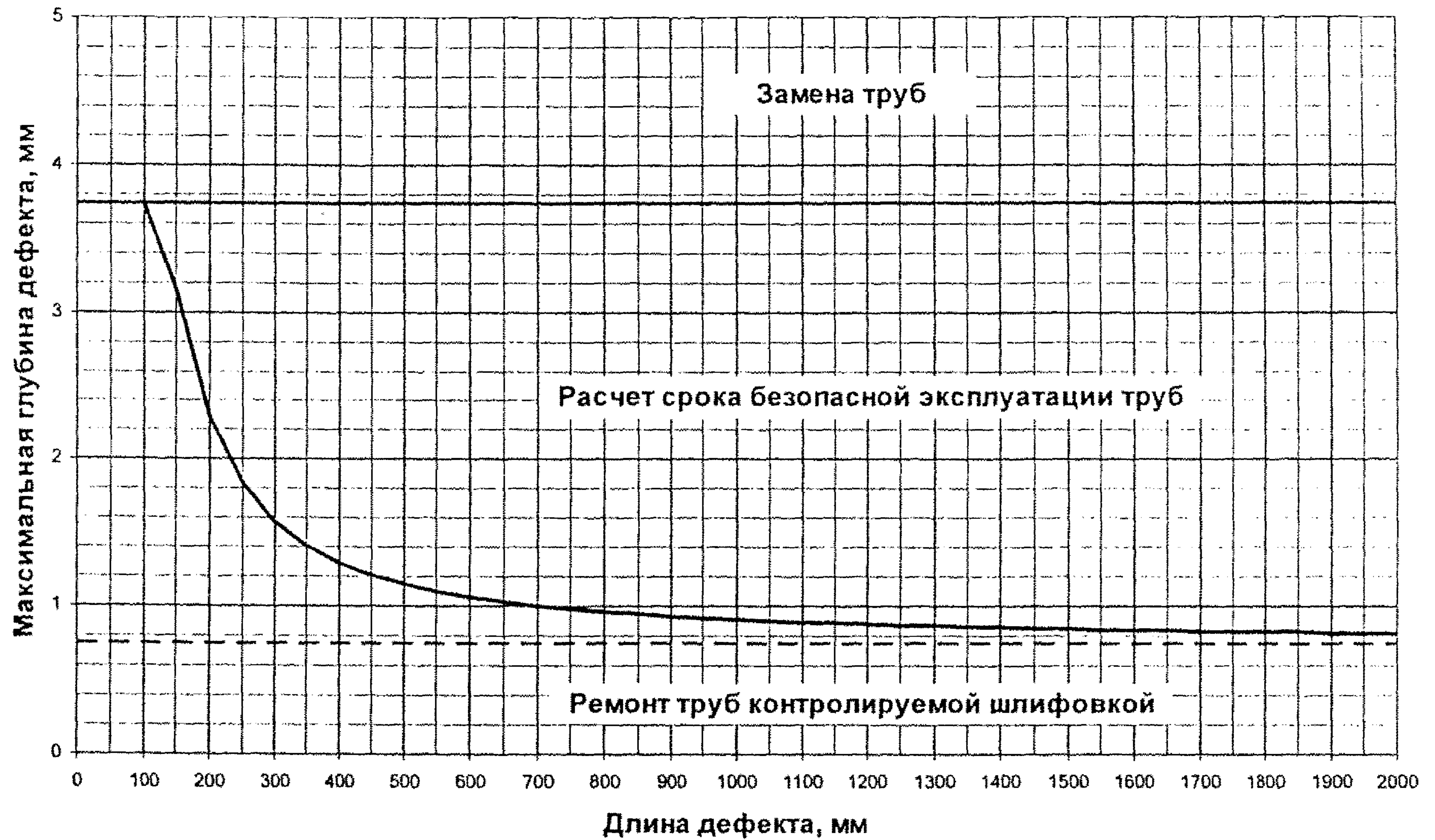
Рис.3.3.4п. График зависимости максимальной глубины дефектов от их длины для труб толщиной стенки 18,7 мм, на которых будут обнаружены стресс-коррозионные дефекты.
