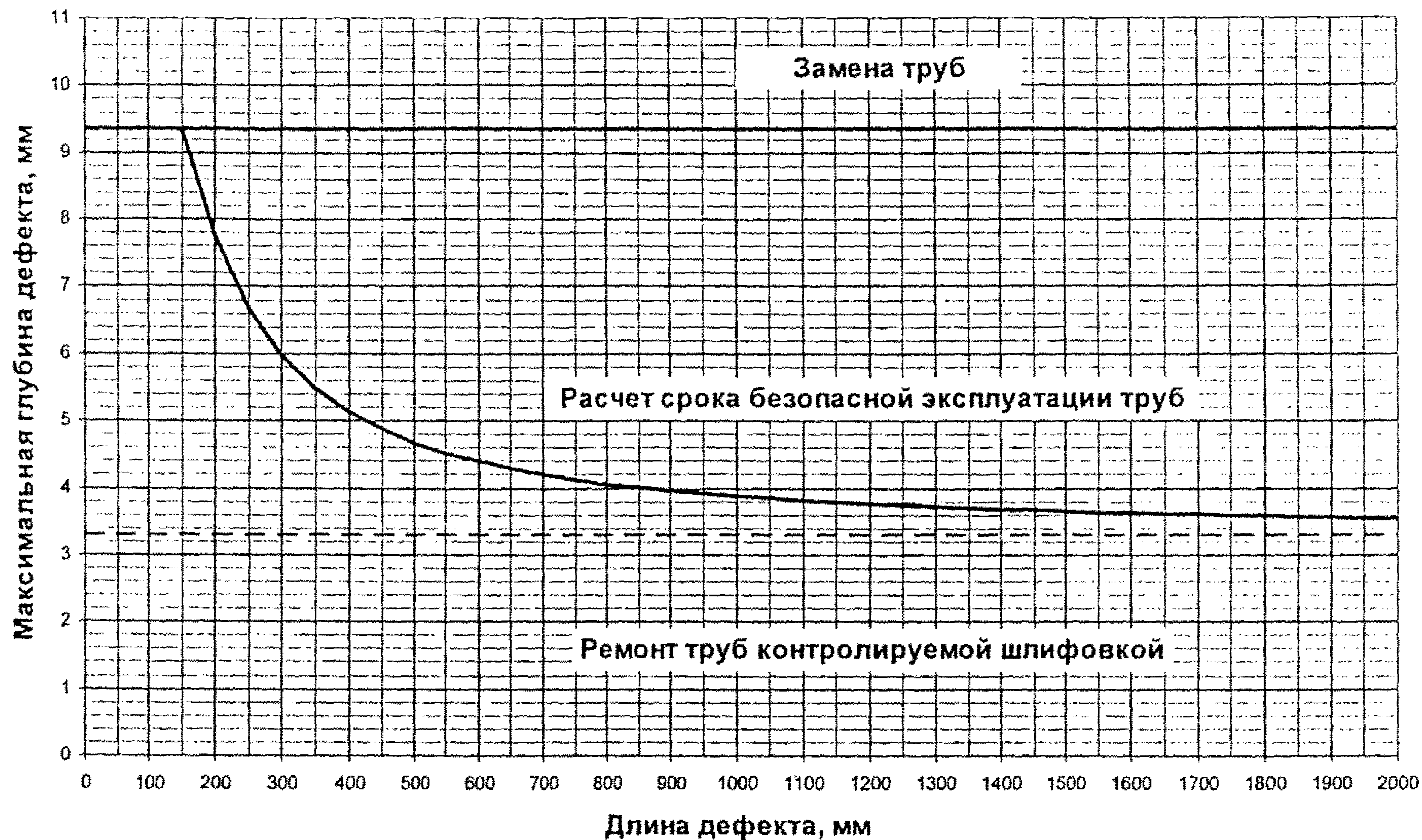
Рис.3.3.2п. График зависимости максимальной глубины дефектов от их длины для труб толщиной стенки 18,7 мм, на которых не будут обнаружены стресс-коррозионные дефекты.
