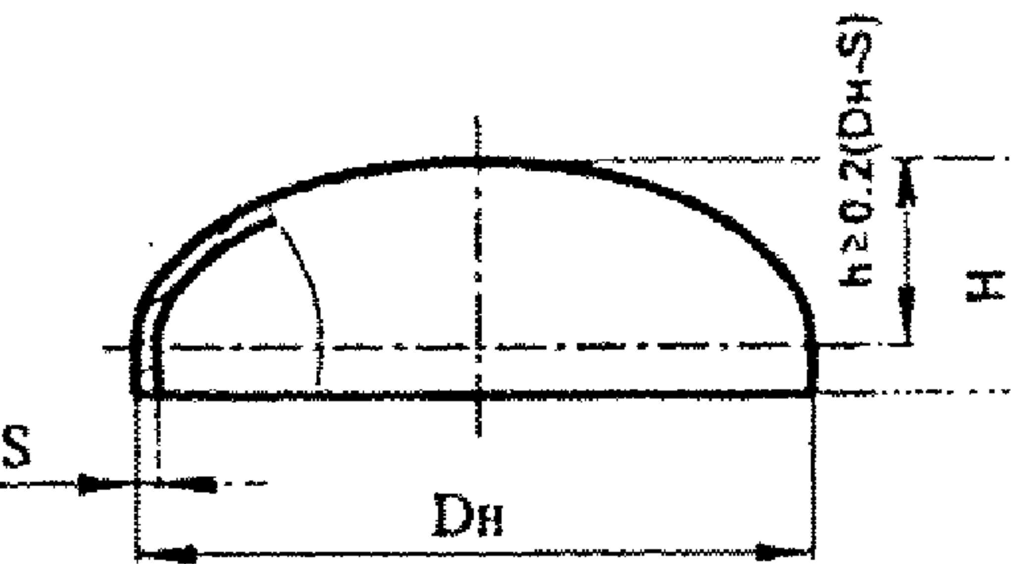
Днища (заглушки) штампованные эллиптические (ДШ)
