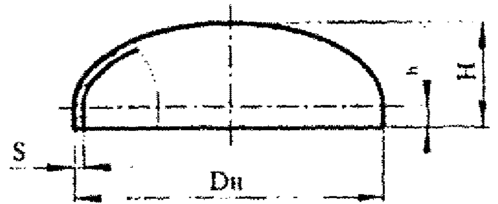
Днища (заглушки) штампованные эллиптические (ДШ)
