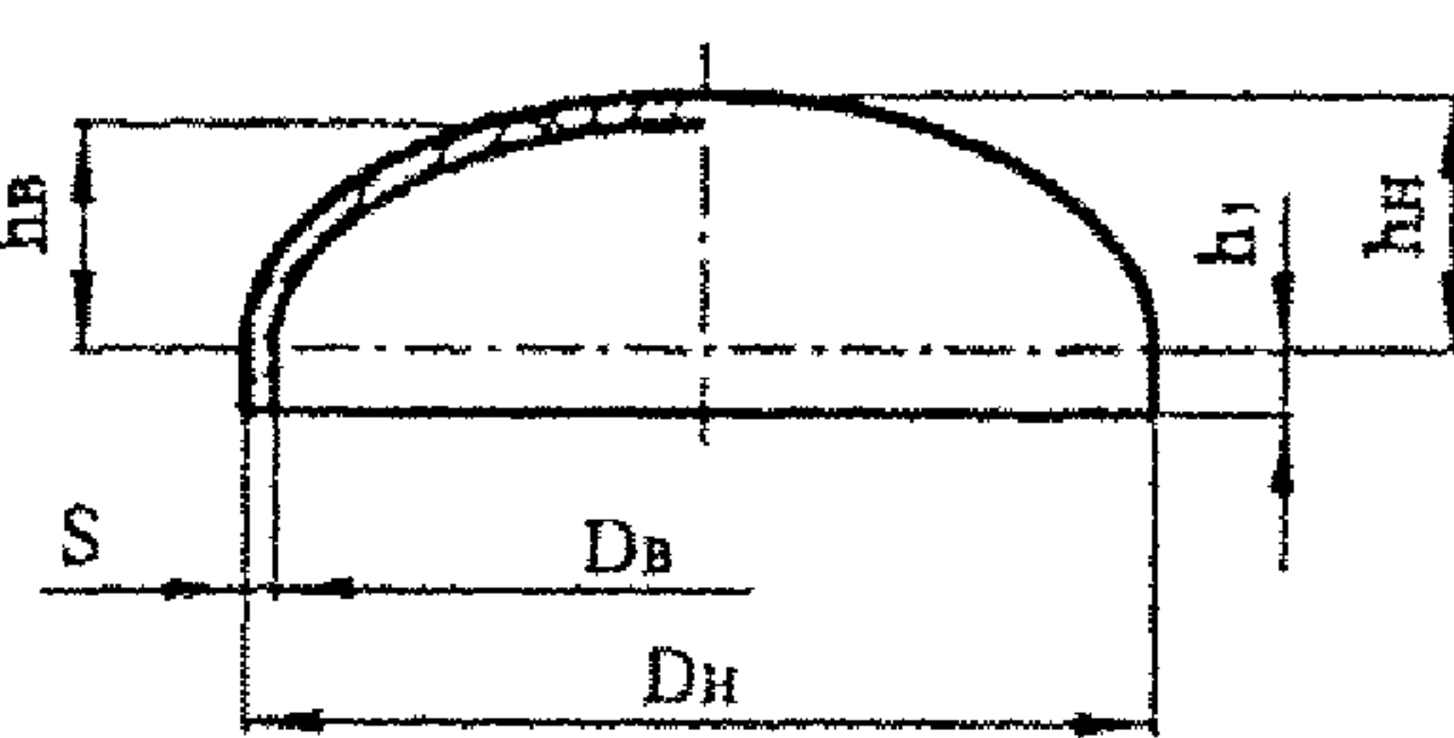
Днища (заглушки) отбортованные эллиптические (ДШ)
