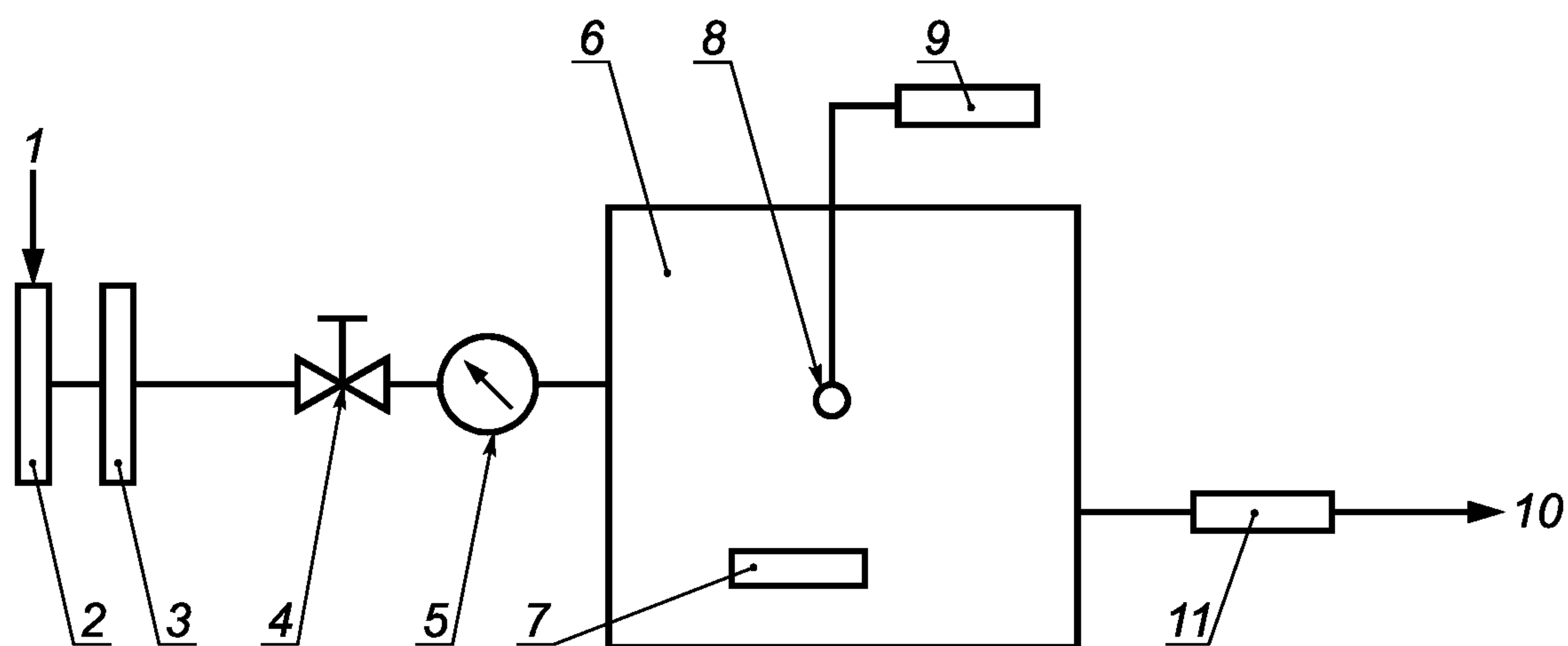
Схема установки с испытательной камерой
