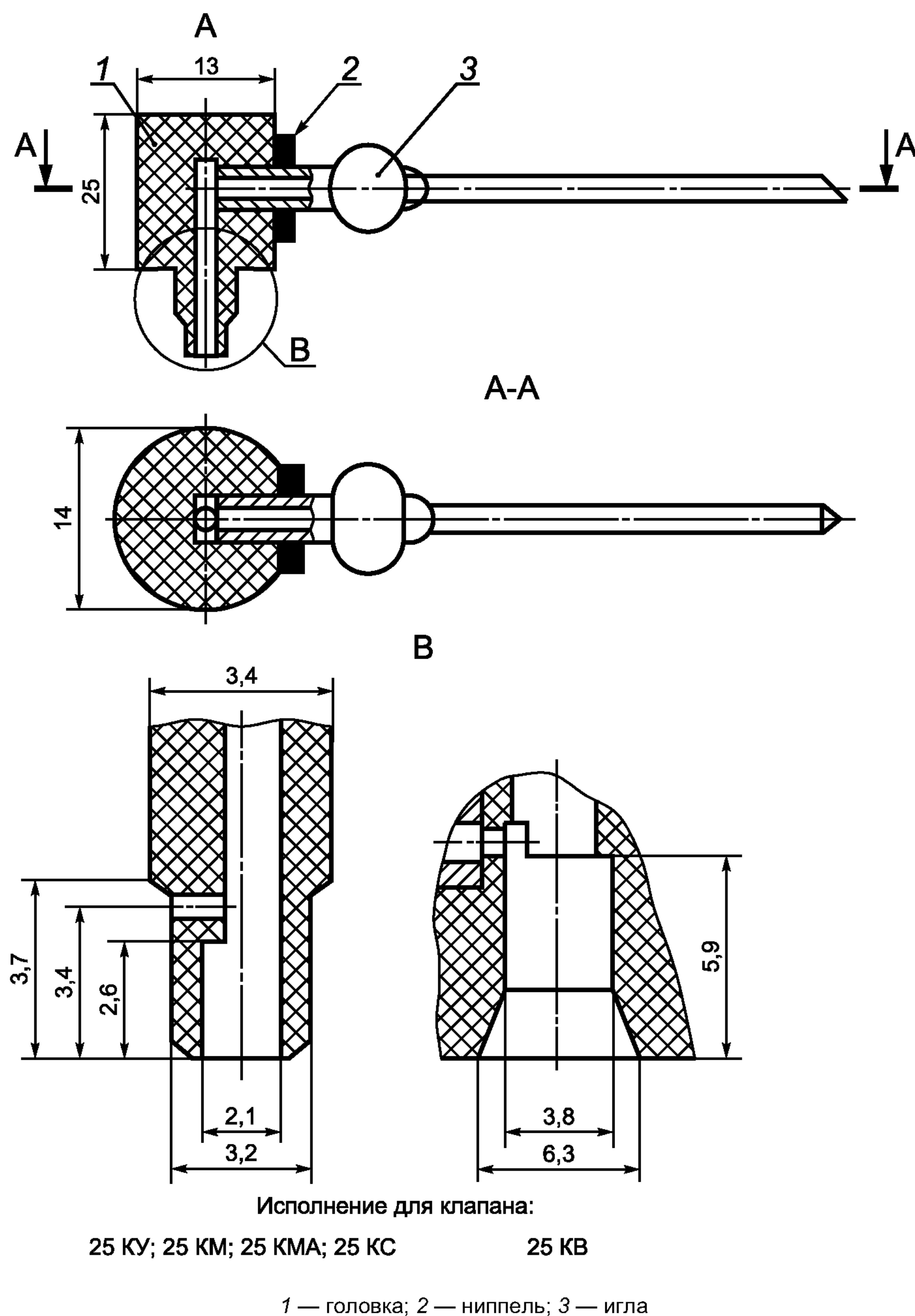
Рисунок 1 — Распылительная головка с инъекционной иглой
