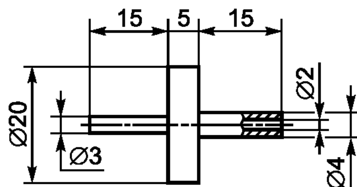
Рисунок 3 — Переходник латунный
