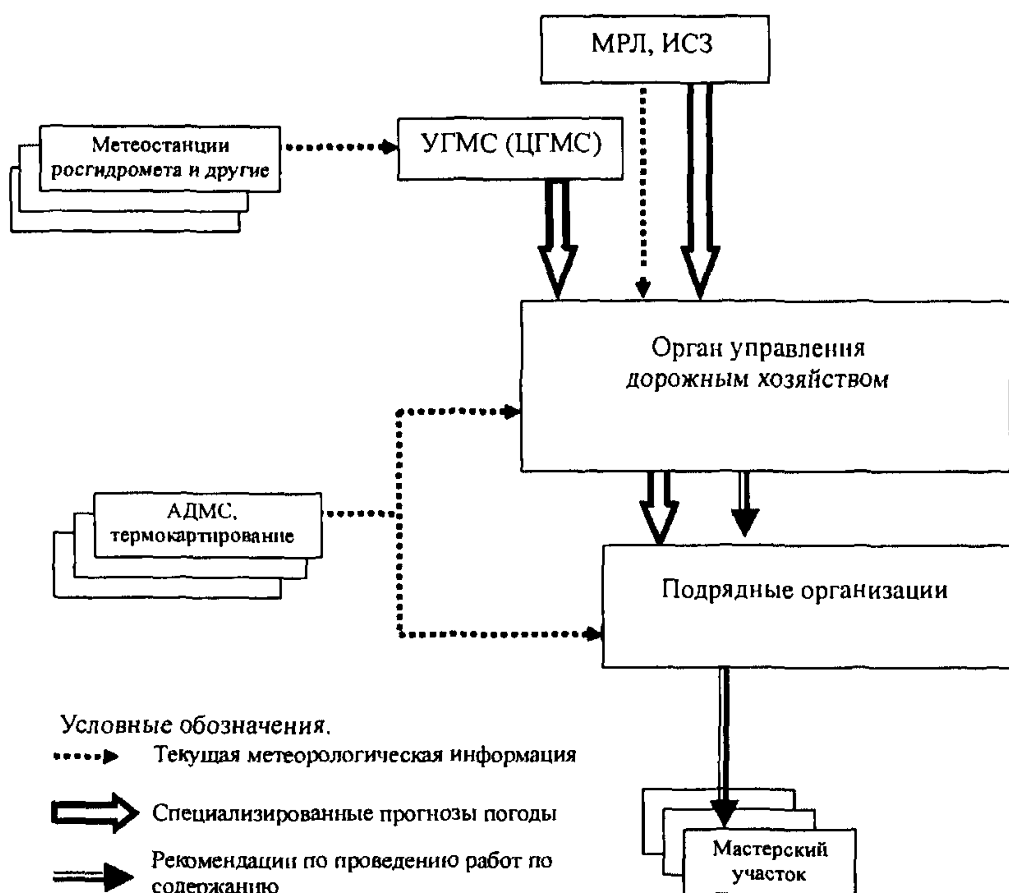
Рисунок 1. Схема получения специализированной гидрометеорологической информации в дорожном хозяйстве
