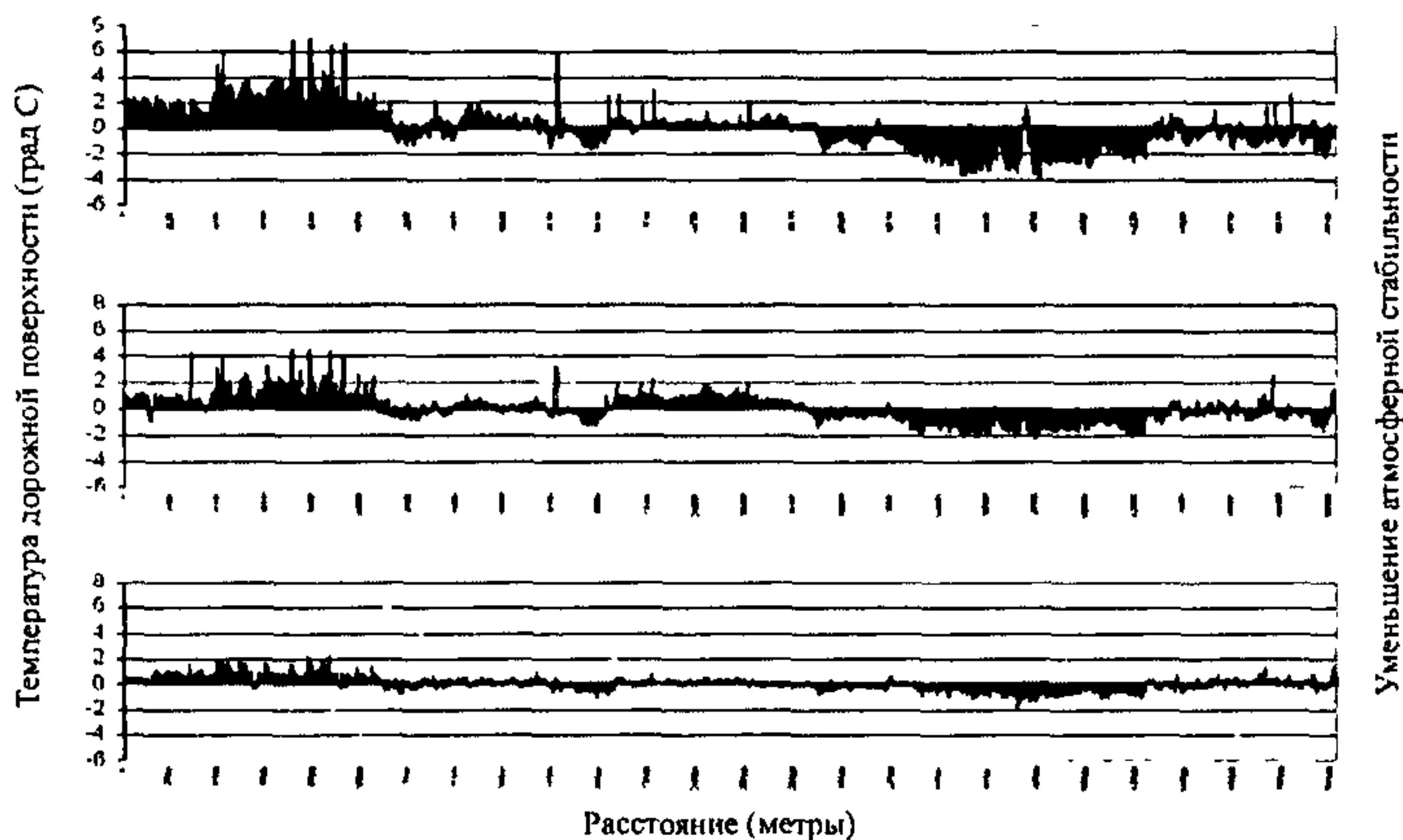
Рисунок Г.1. Пример измерения температуры дорожной поверхности
