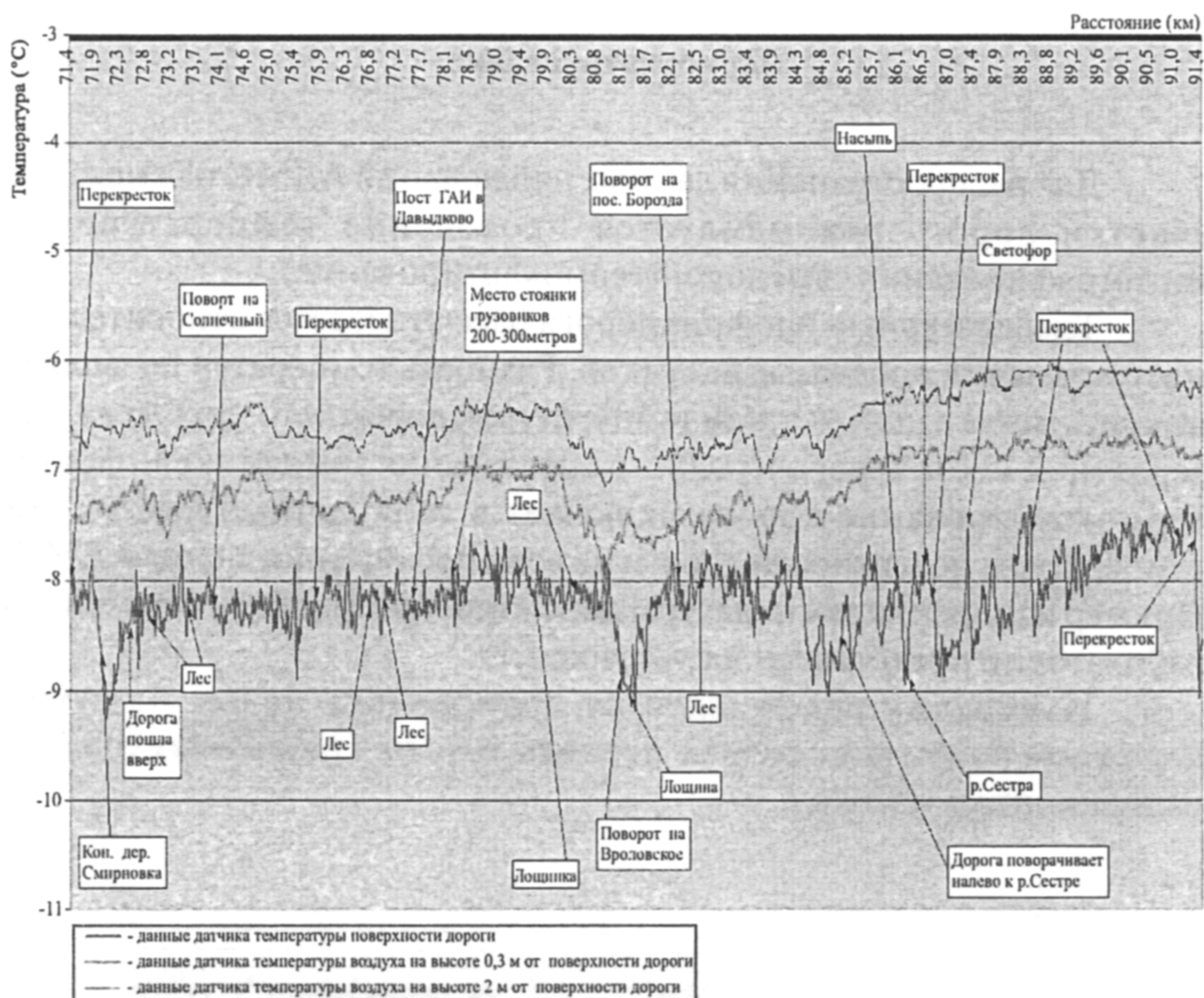
Рисунок Г.2. Вид первичной, расшифрованной термокарты (термопрофиль)
