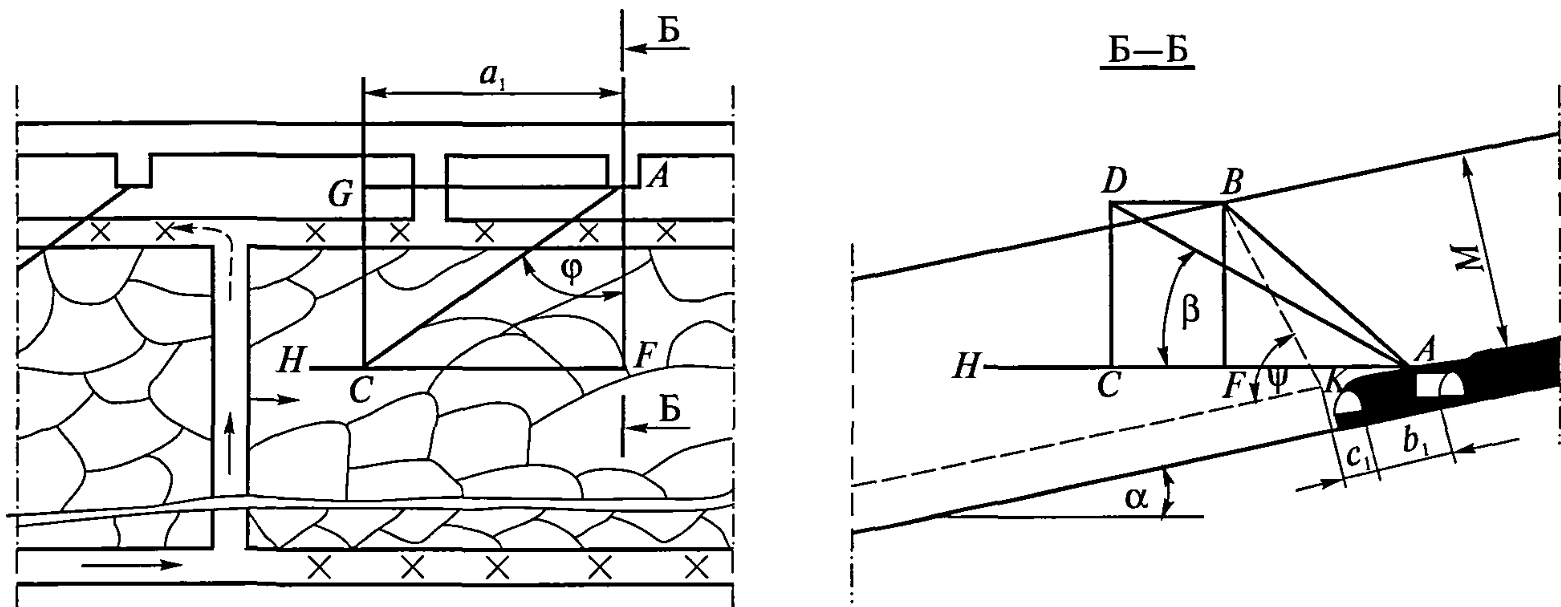
Рис. 1. Графическое определение параметров скважин, буримых на подрабатываемый пласт
