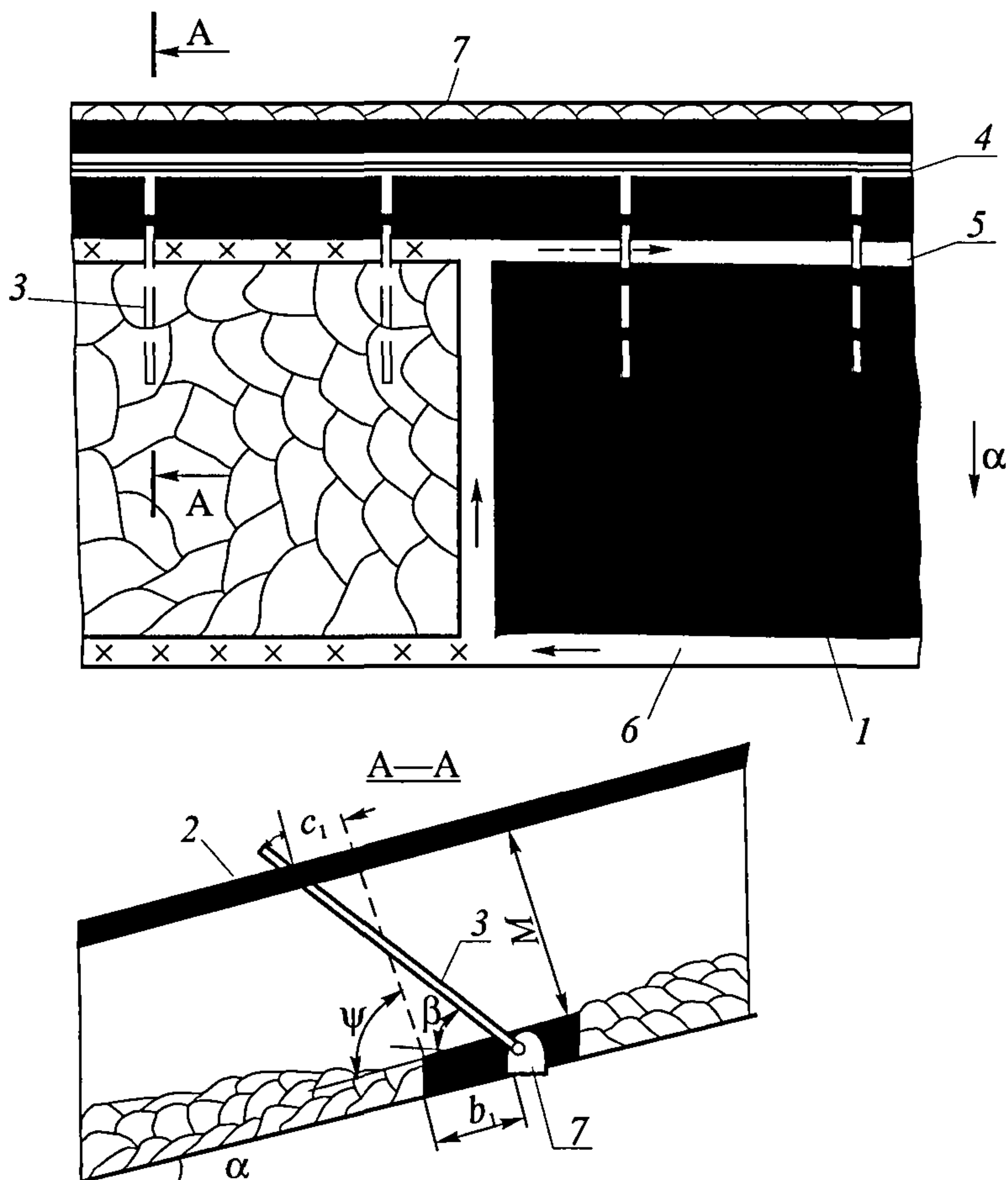
Рис. 1. Схема дегазации подрабатываемых сближенных пластов скважинами, пробуренными из охраняемой целиком угля выработки (схема 1):
