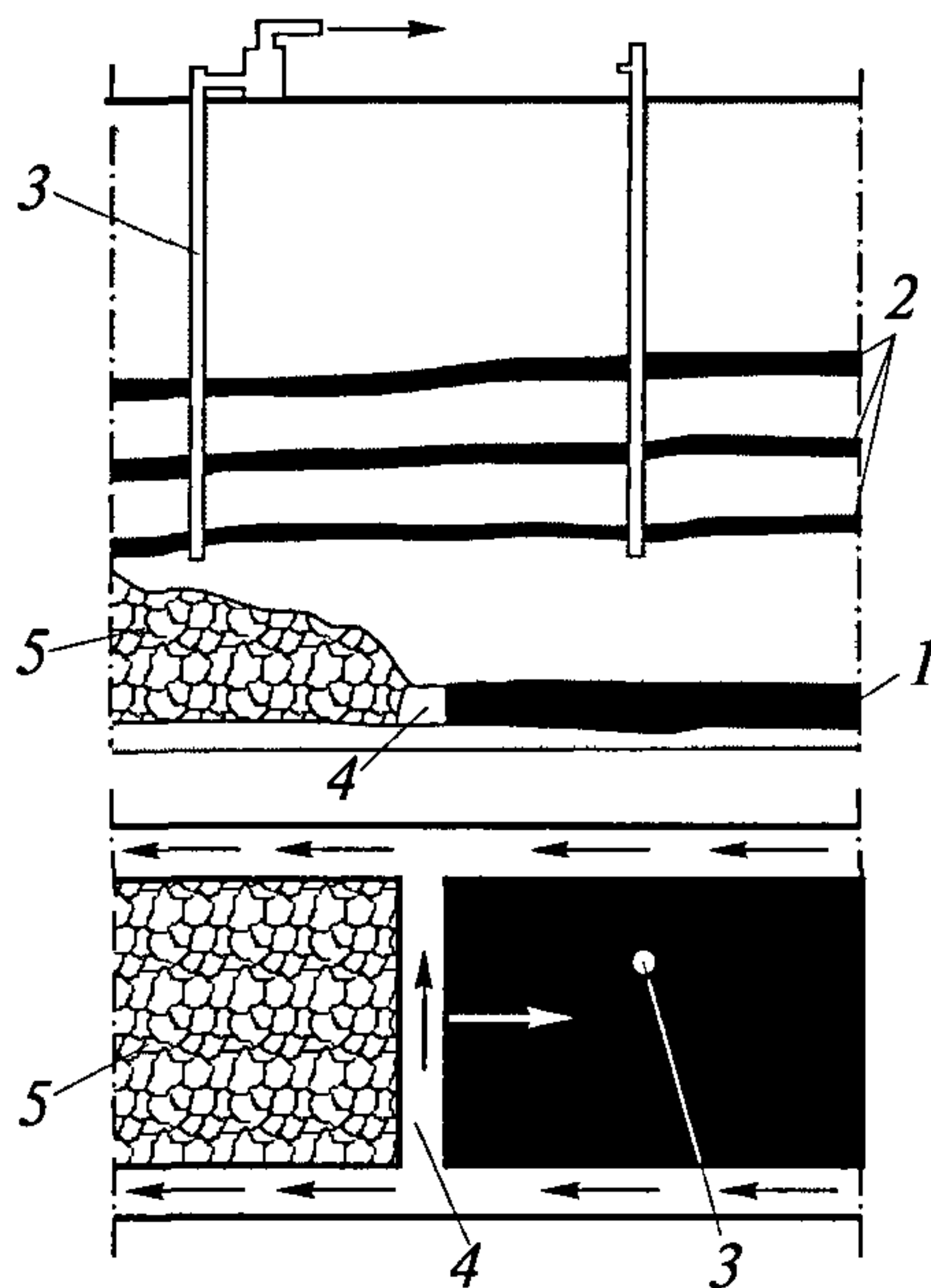
Рис. 2. Схема дегазации сближенных пластов скважинами, пробуренными с поверхности: 1 — разрабатываемый пласт; 2 — сближенные пласты; 3 — скважина; 4 — очистной забой; 5 — выработанное пространство
