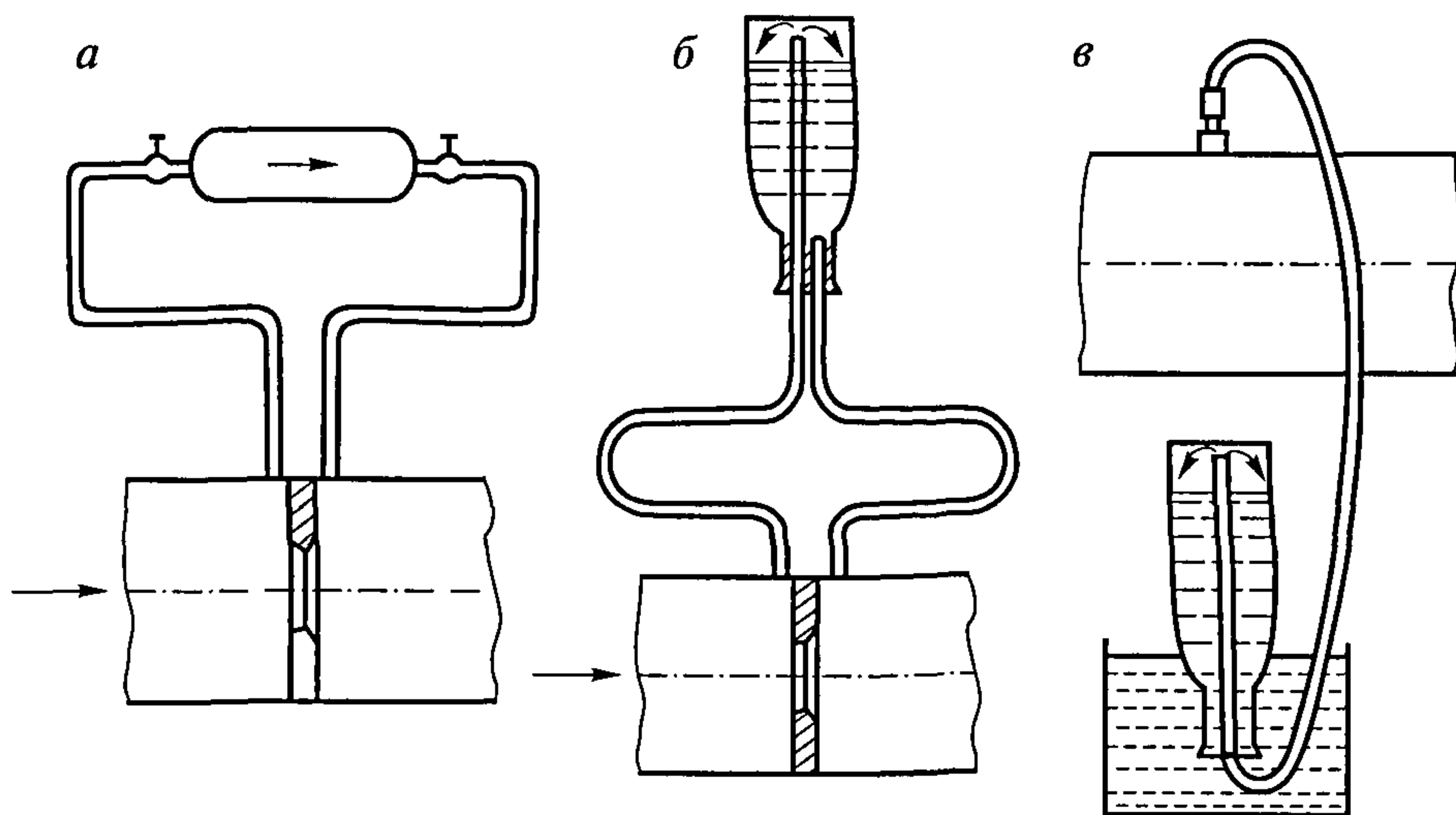
Рис. 7. Схема отбора проб газовой воздушной смеси из газопровода: а — бюреткой Зегера; б — бутылкой при вакууме; в — бутылкой при давлении выше атмосферного
