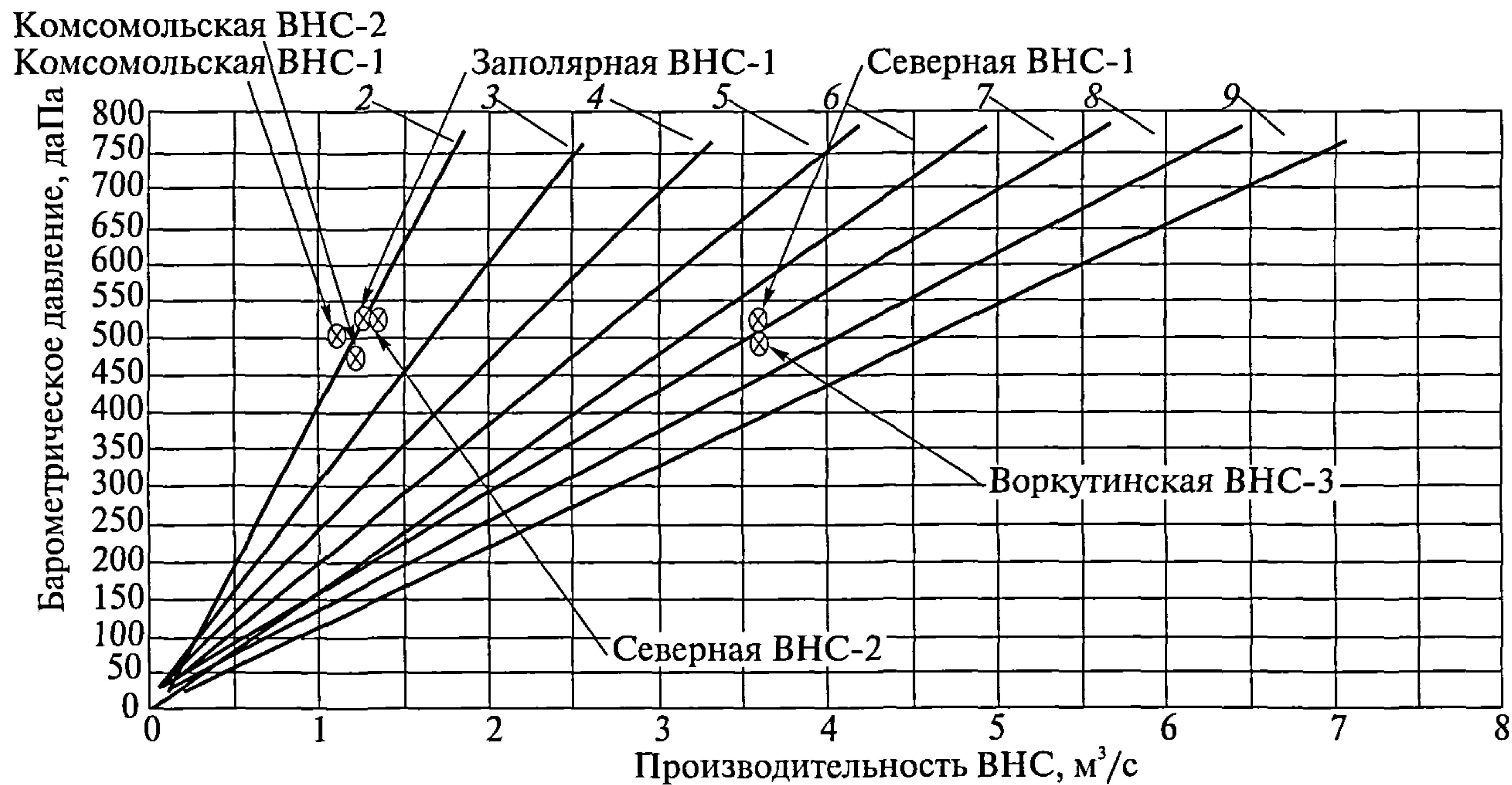
Рис. 6. Характеристики вакуум-насосных станций
