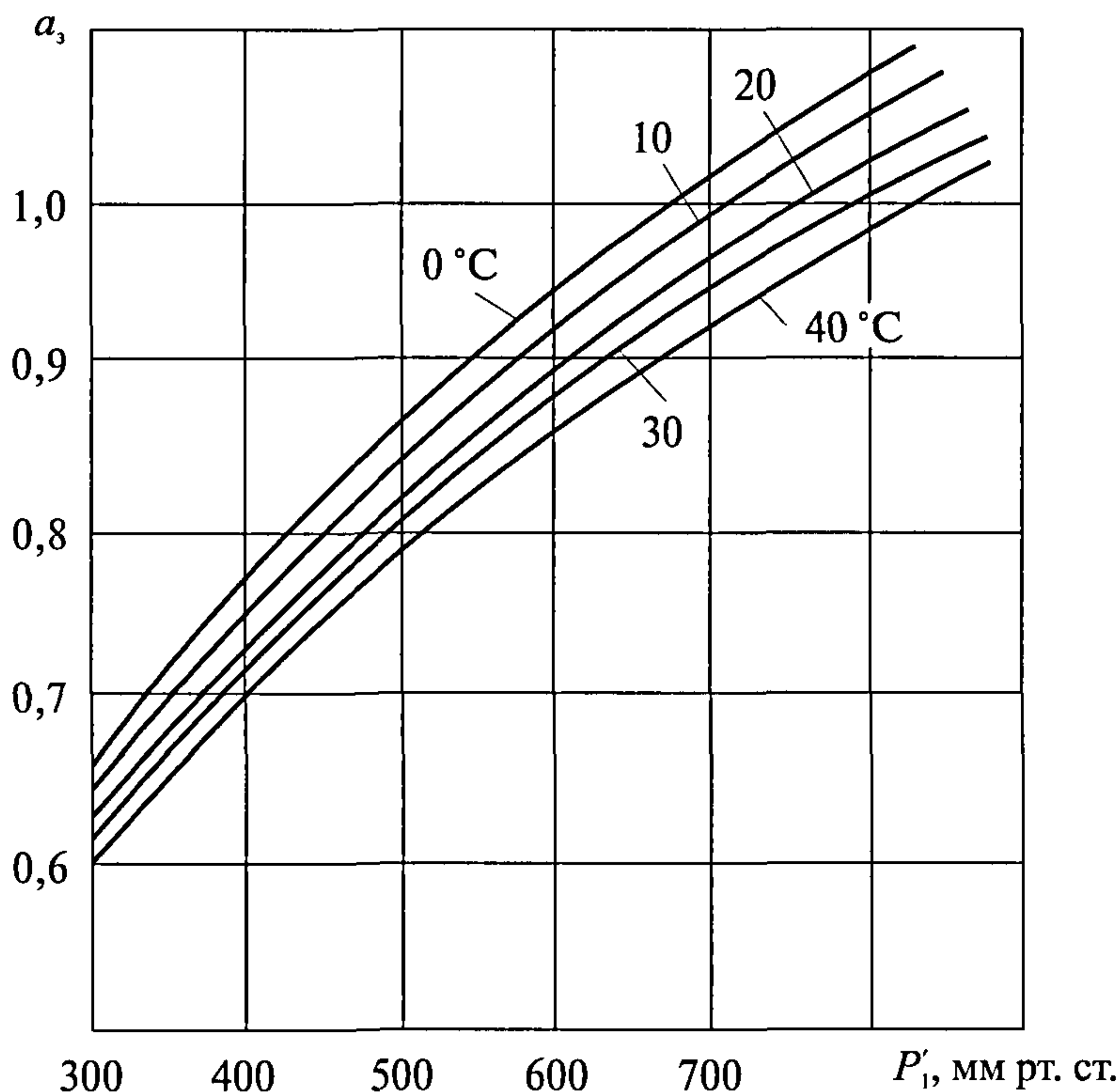
Рис. 4. Определение поправочного коэффициента a_3
