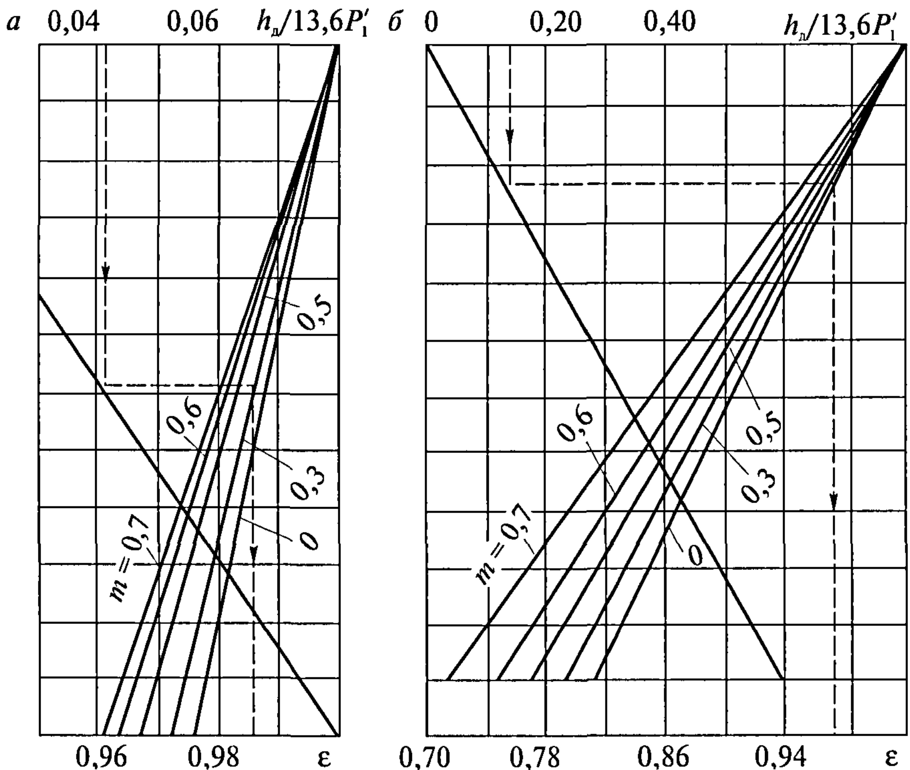
Рис. 3. Определение коэффициента \varepsilon при малых (а) и при больших (б) значениях h_d / 13,6 P'_1
