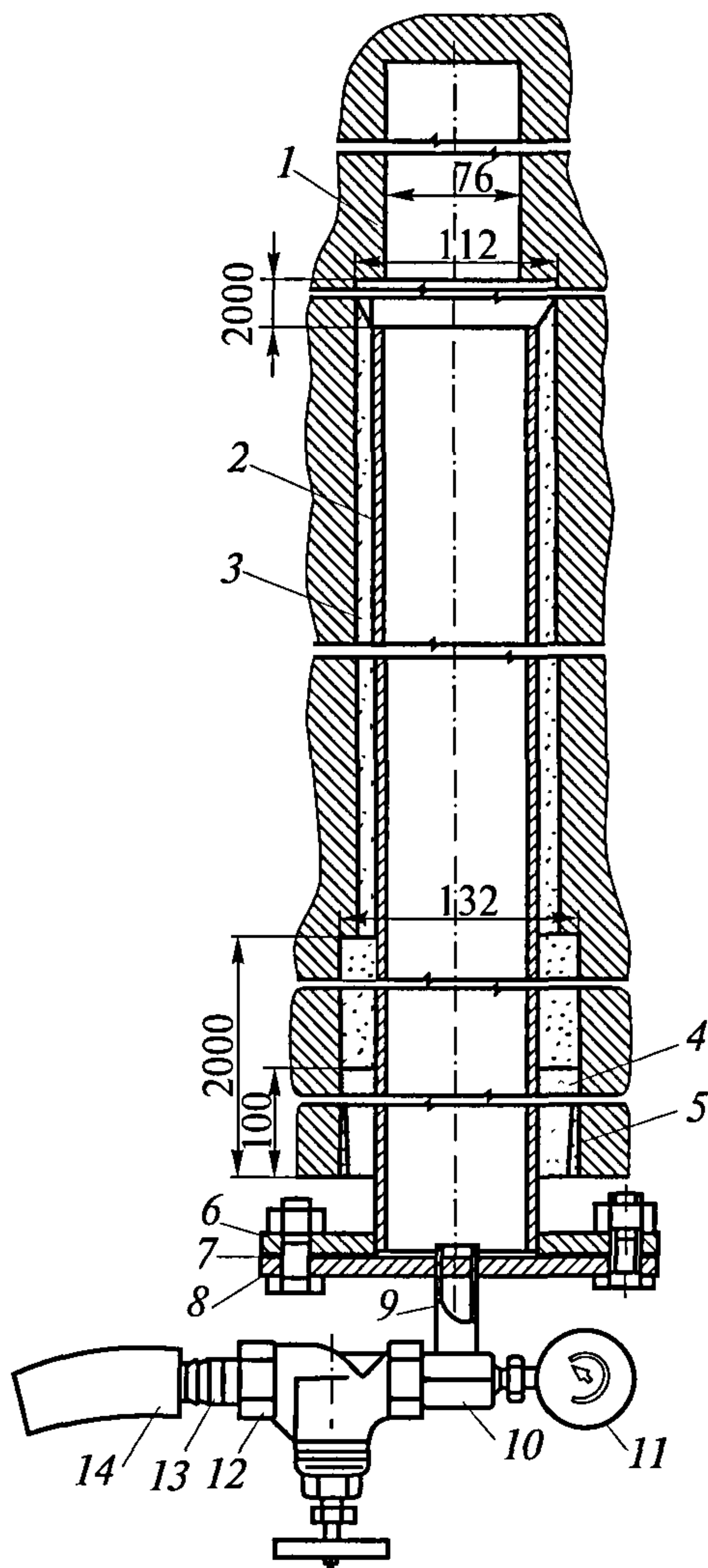
Рис. 2. Приспособление для контроля герметичности скважины:
