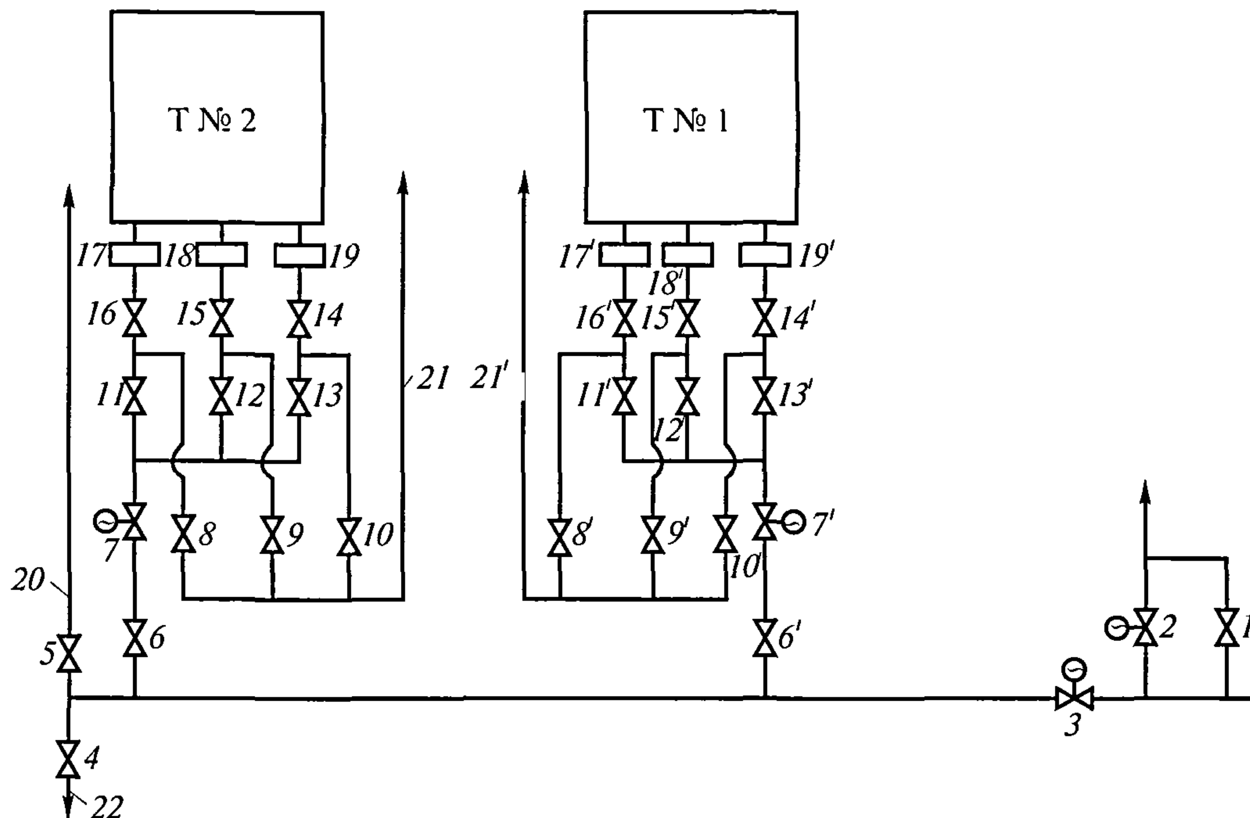
Рис. 2. Упрощенная технологическая схема газопроводов АГВН:
