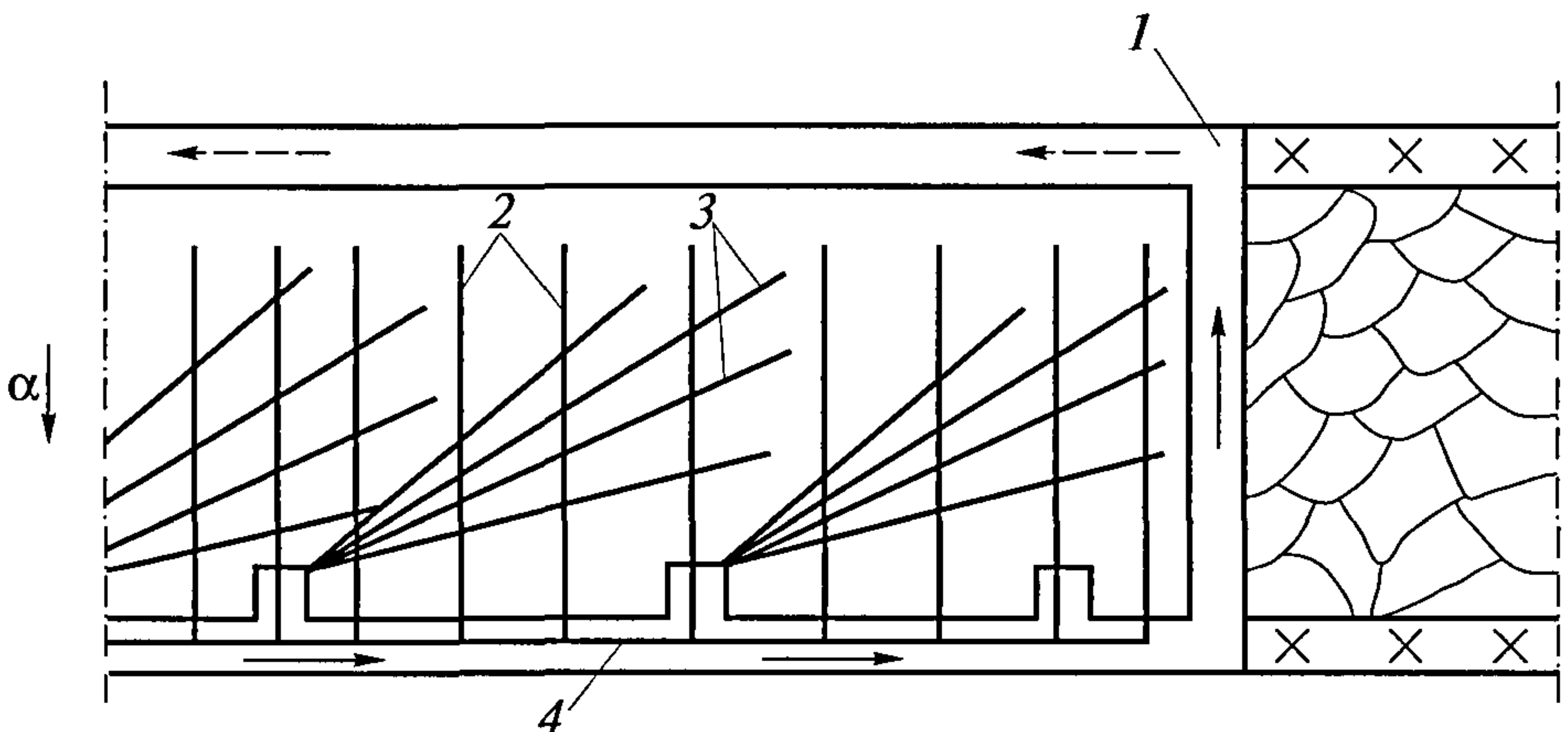
Рис. 11. Схема дегазации пласта параллельными и веерными, ориентированными на очистной забой скважинами: 1 — очистной забой; 2 — параллельные очистному забою скважины; 3 — веерные скважины, ориентированные на очистной забой; 4 — дегазационный трубопровод; \alpha — угол падения пласта
