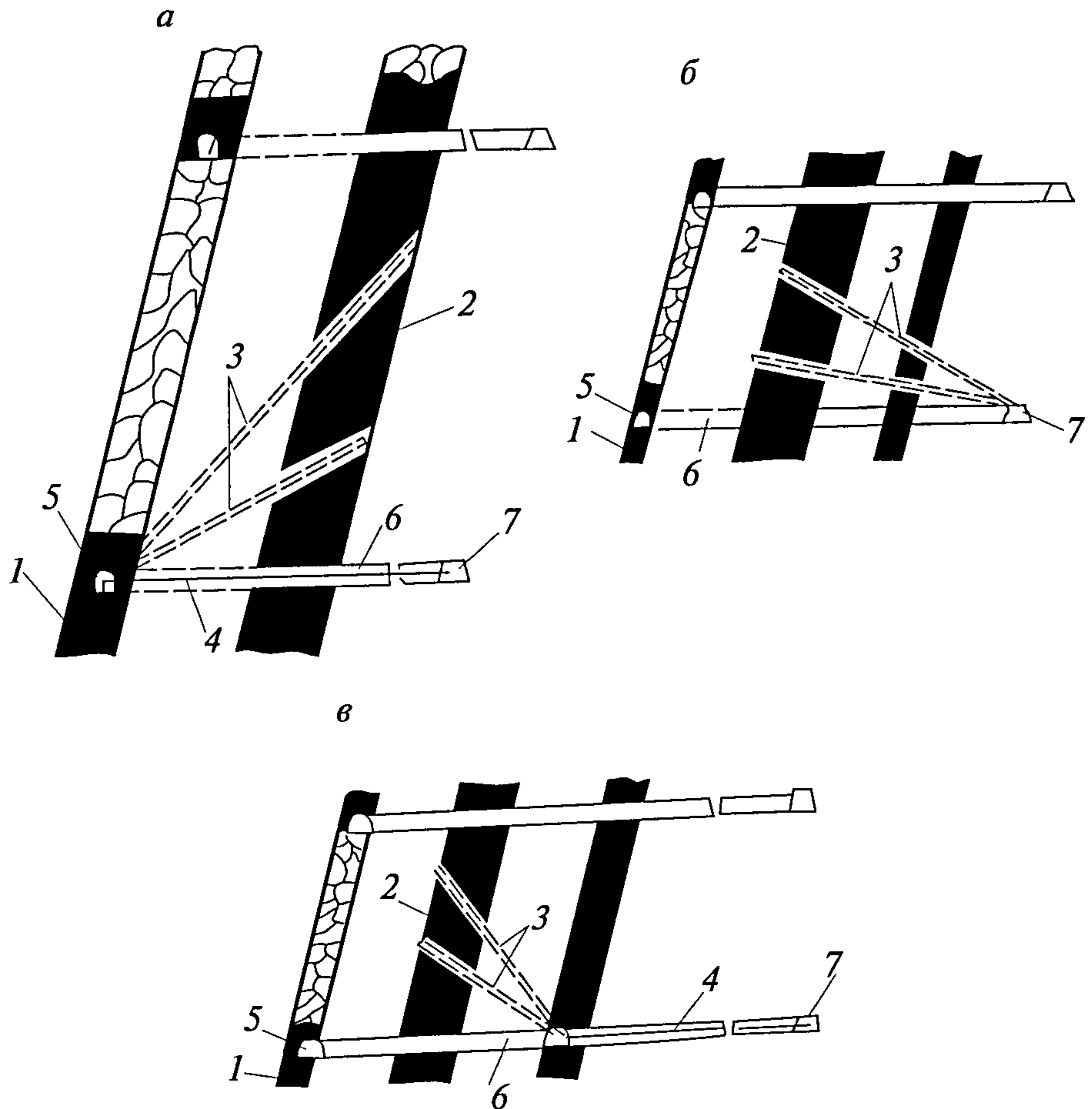
Рис. 1. Схема дегазации надрабатываемого крутого пласта скважинами, пробуренными веером вкрест его залегания:
