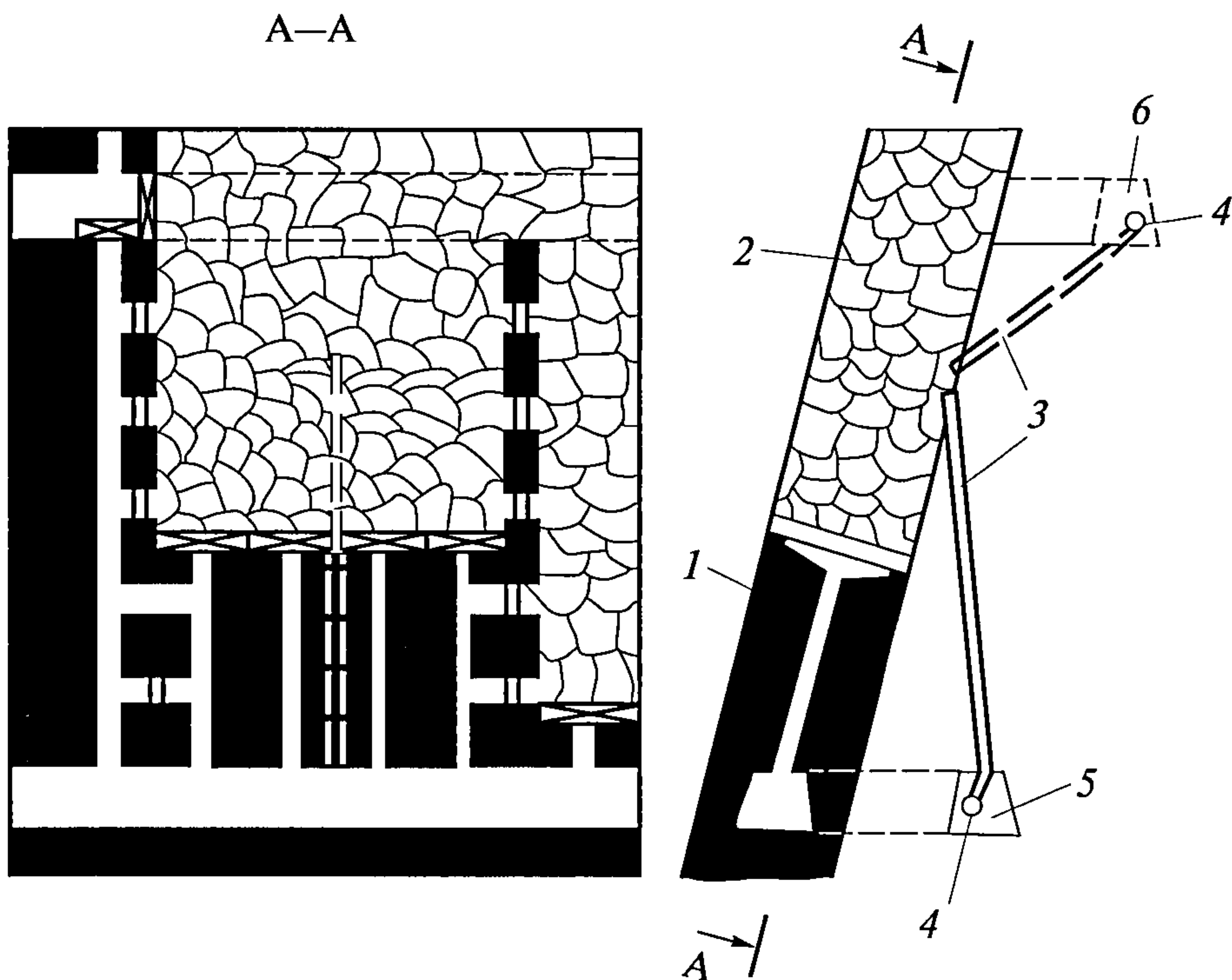
Рис. 2. Схема дегазации выработанных пространств мощных крутых пластов скважинами, пробуренными из полевых выработок: 1 — разрабатываемый пласт; 2 — выработанное пространство; 3 — дегазационные скважины; 4 — дегазационный трубопровод; 5 — полевой штрек откаточного горизонта; 6 — полевой штрек вентиляционного горизонта
