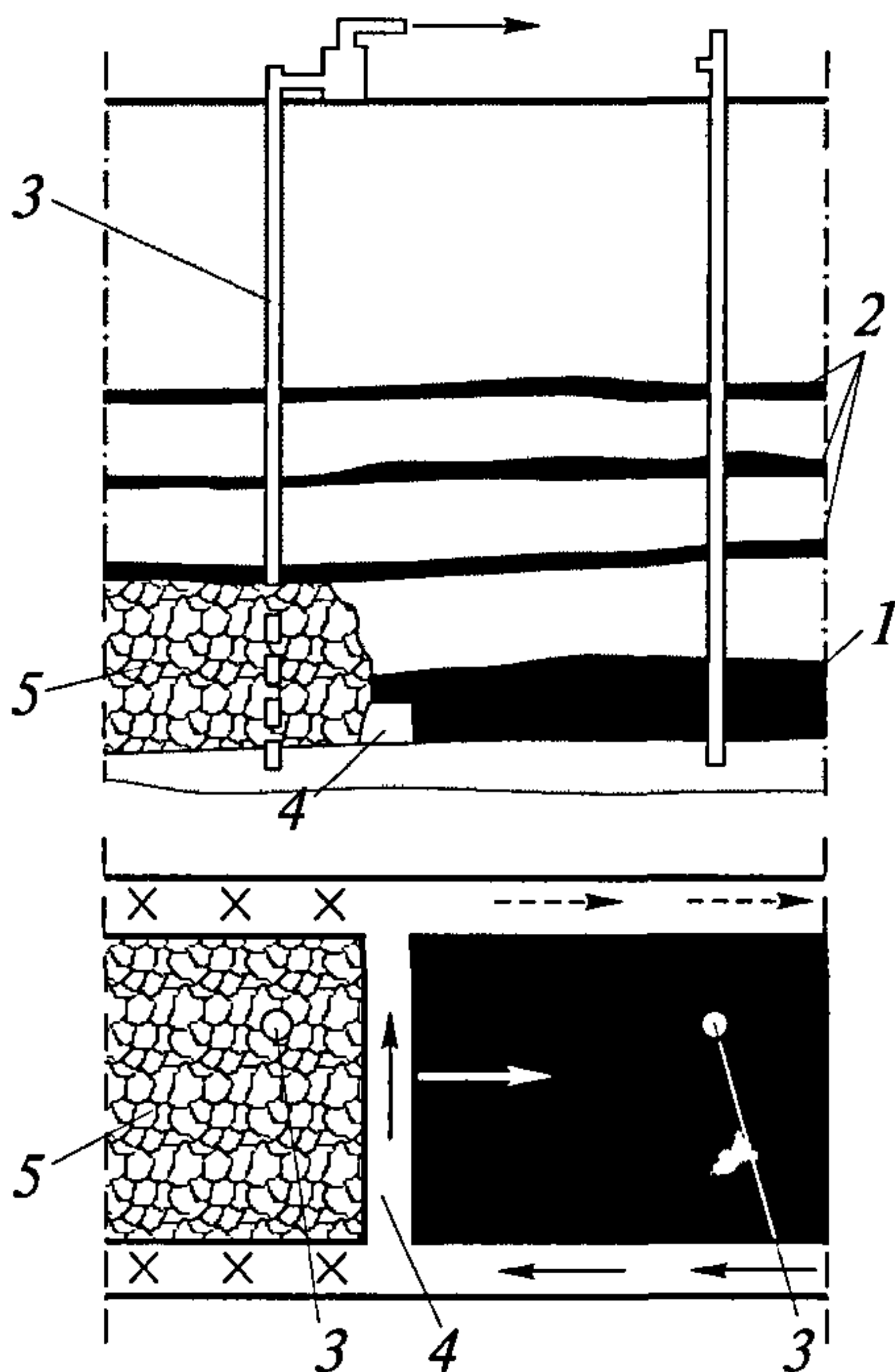
Рис. 1. Схема дегазации сближенных пластов и выработанного пространства скважинами, пробуренными с поверхности: 1 — разрабатываемый пласт; 2 — сближенные пласты; 3 — скважина; 4 — очистной забой; 5 — выработанное пространство
