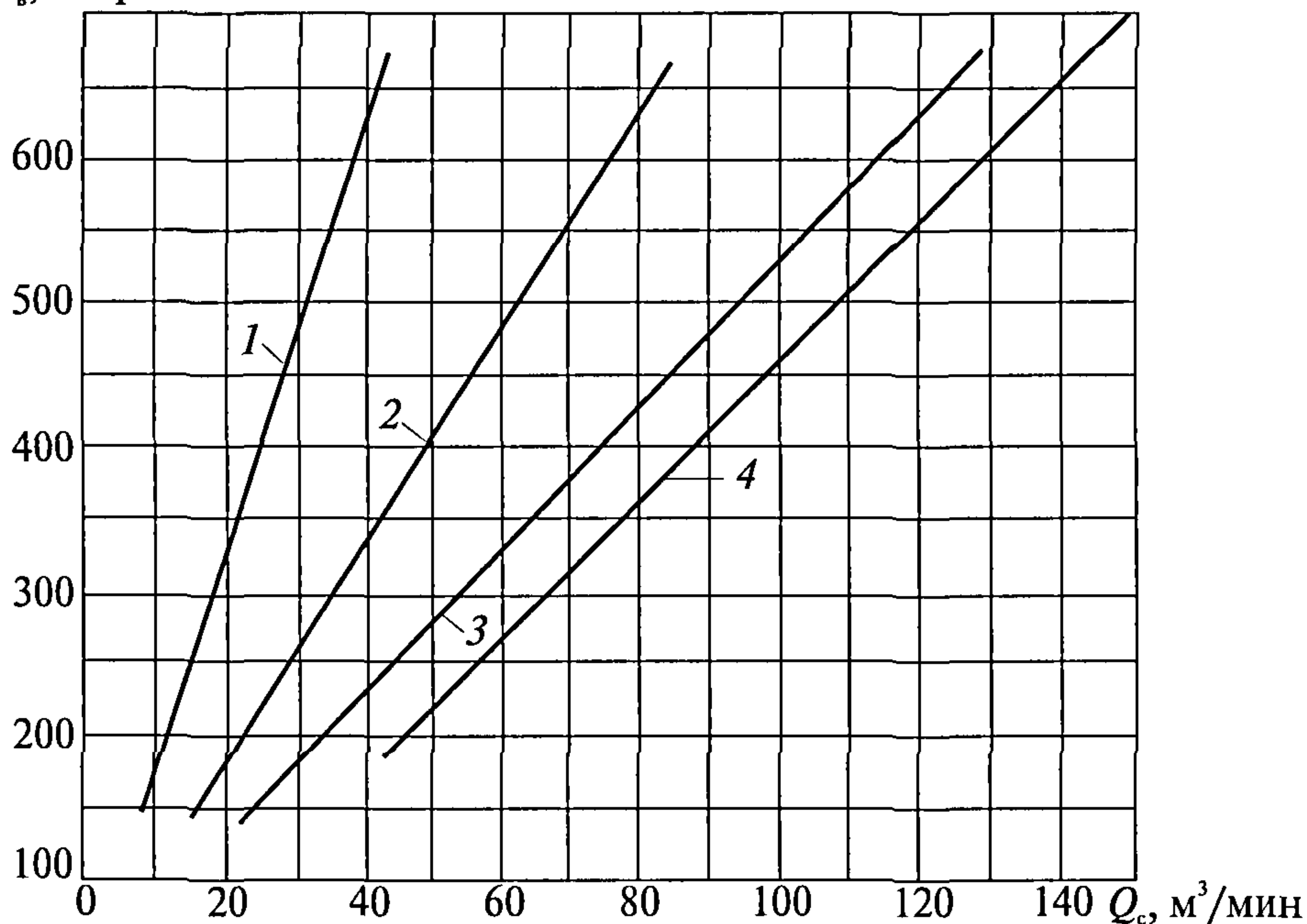
Рис. 3. Характеристика вакуум-насосов, работающих в режиме всасывания:
