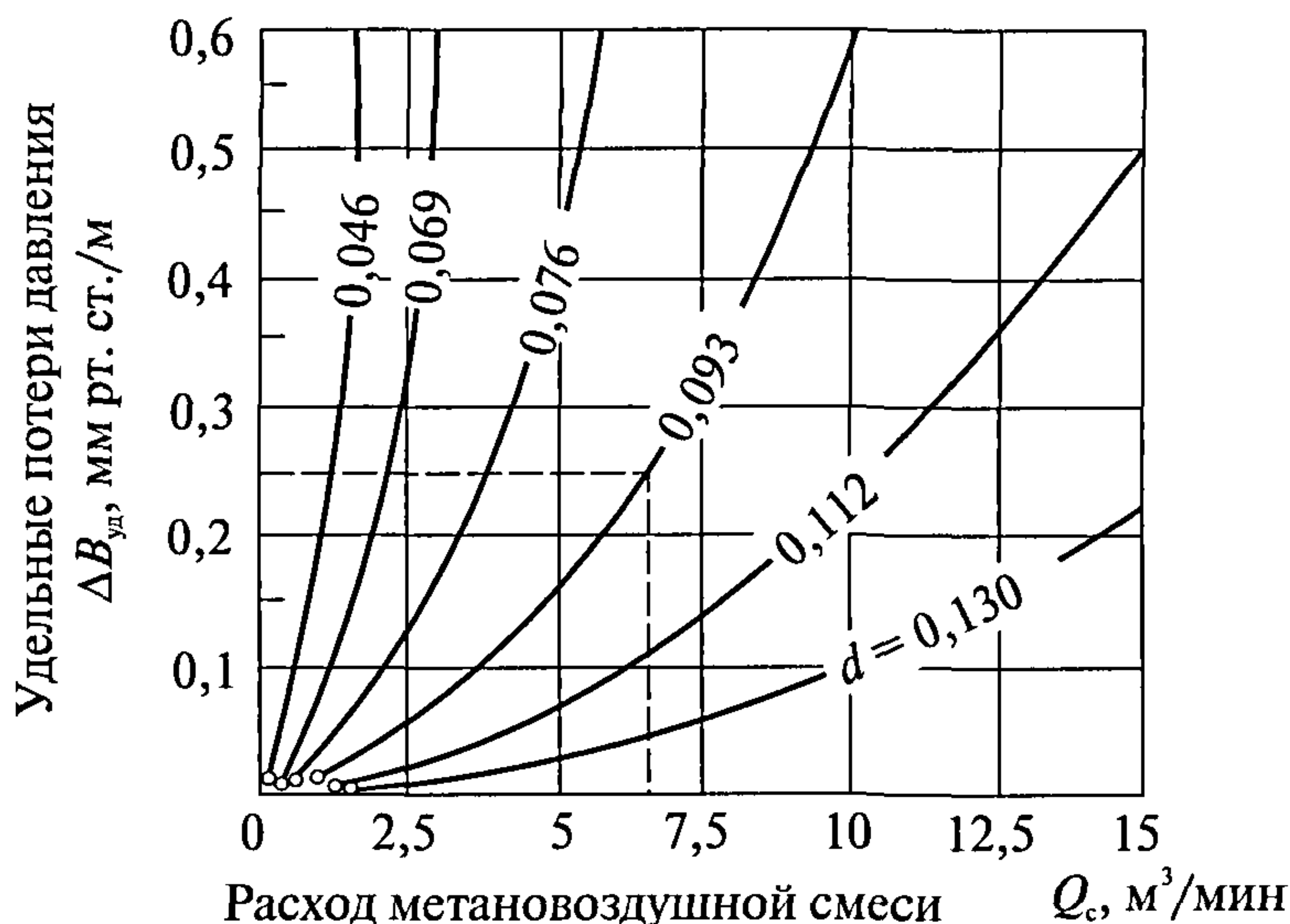
Рис. 2. Определение удельных потерь давления в скважине
