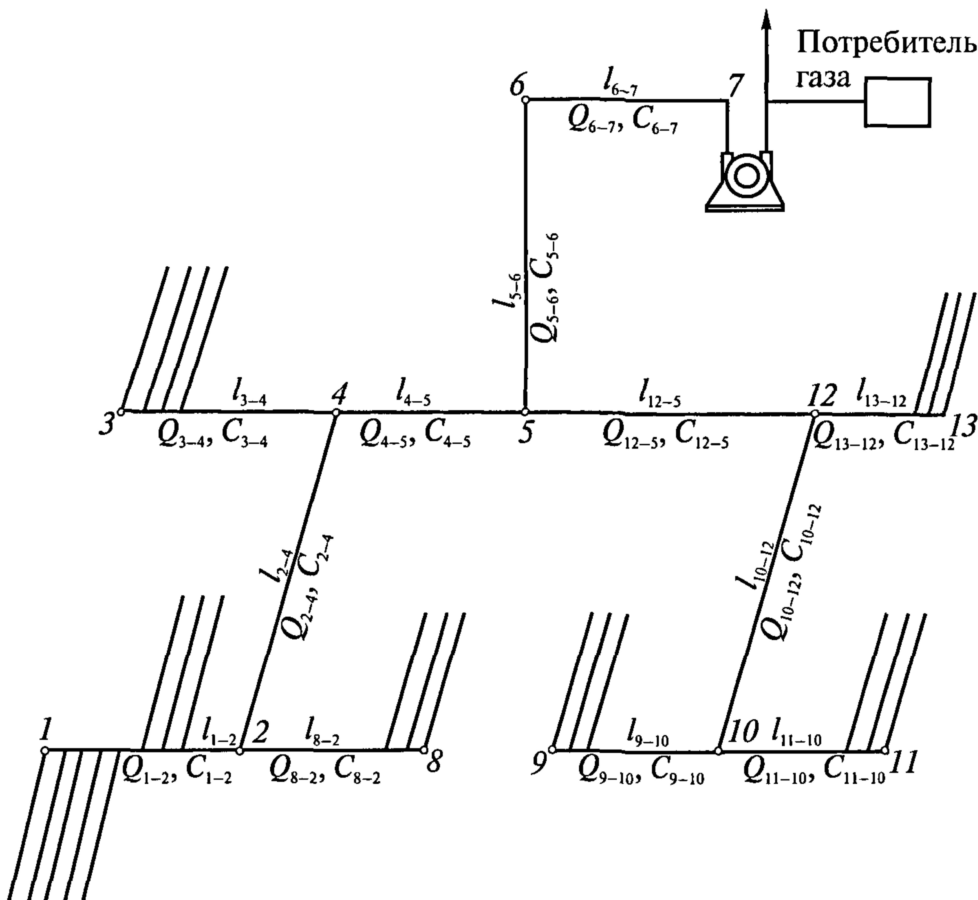
Рис. 1. Схема для расчета газопроводов
