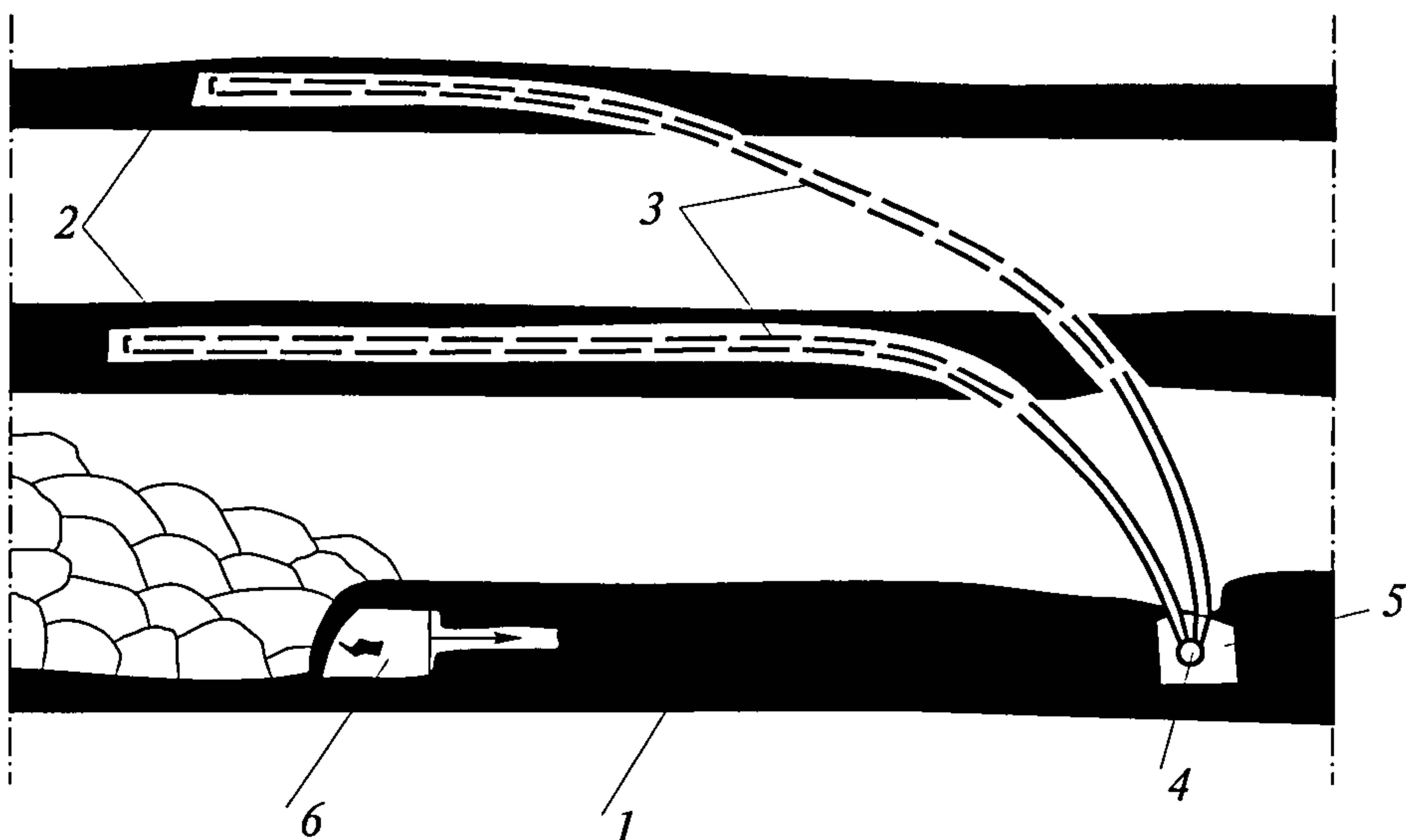
Рис. 6. Схема дегазации сближенного пласта скважинами, пробуренными вдоль столба из фланговой выработки (схема 5а): 1 — разрабатываемый пласт; 2 — сближенные пласты; 3 — дегазационные скважины; 4 — дегазационный трубопровод; 5 — фланговая выработка; 6 — очистной забой
