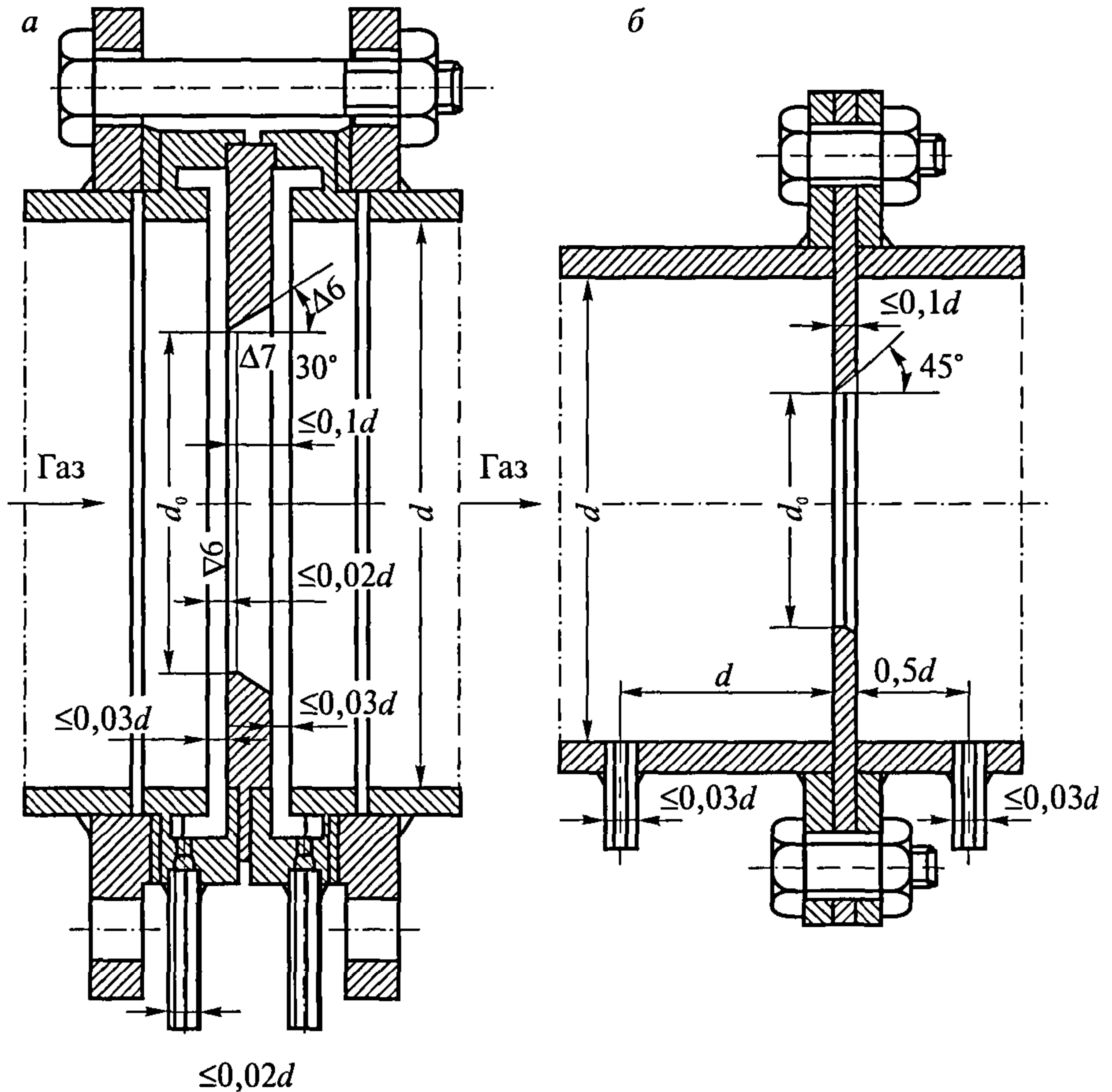
Рис. 1. Диафрагмы для замера расхода газа: а — нормальная; б — дисковая; \Delta 6 , \Delta 7 — чистота обработки поверхности диска
