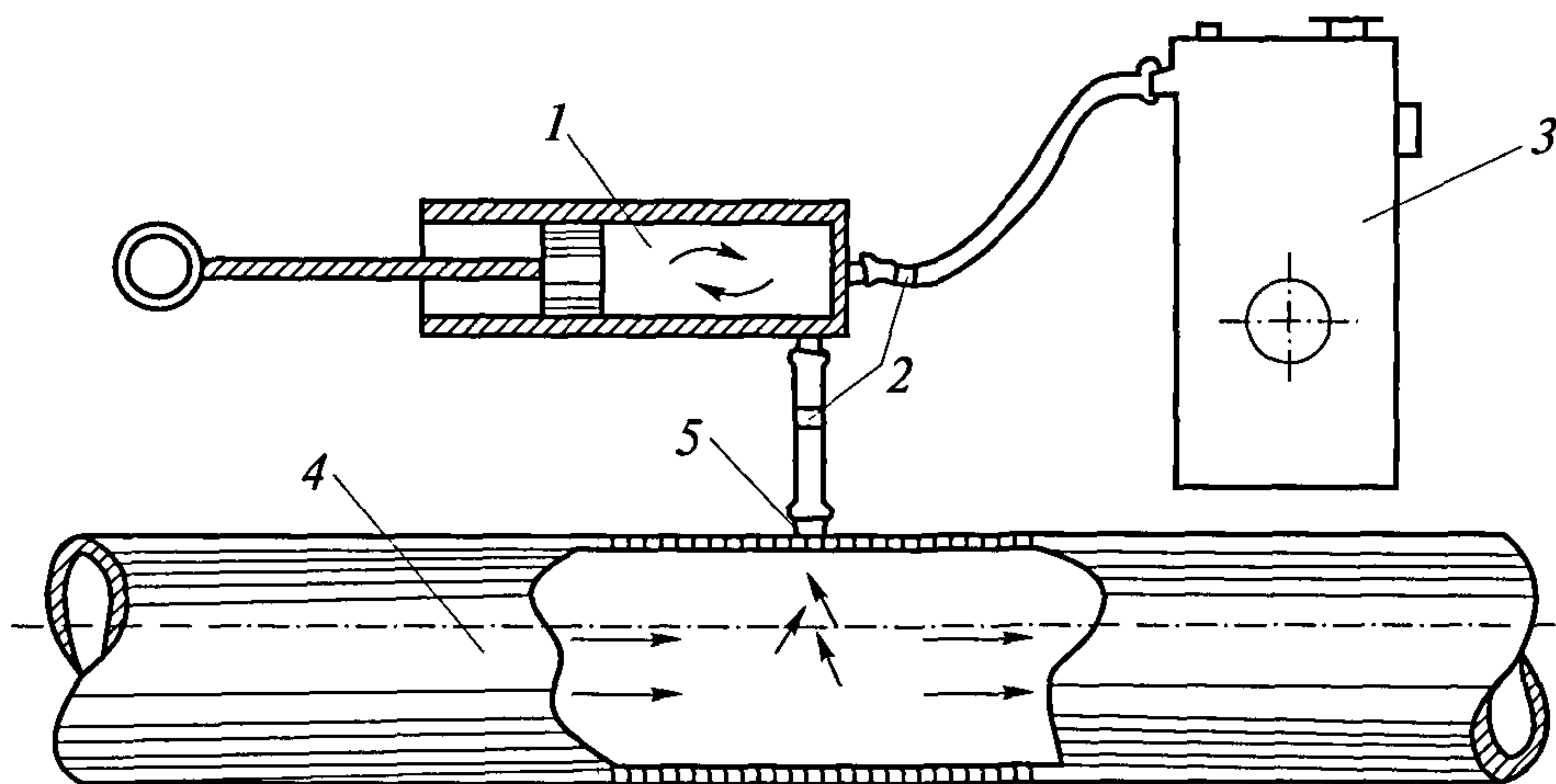
Рис. 2. Схема отбора проб газовой смеси: 1 — насос ручной; 2 — обратный клапан; 3 — интерферометр; 4 — газопровод; 5 — штуцер для отбора пробы
