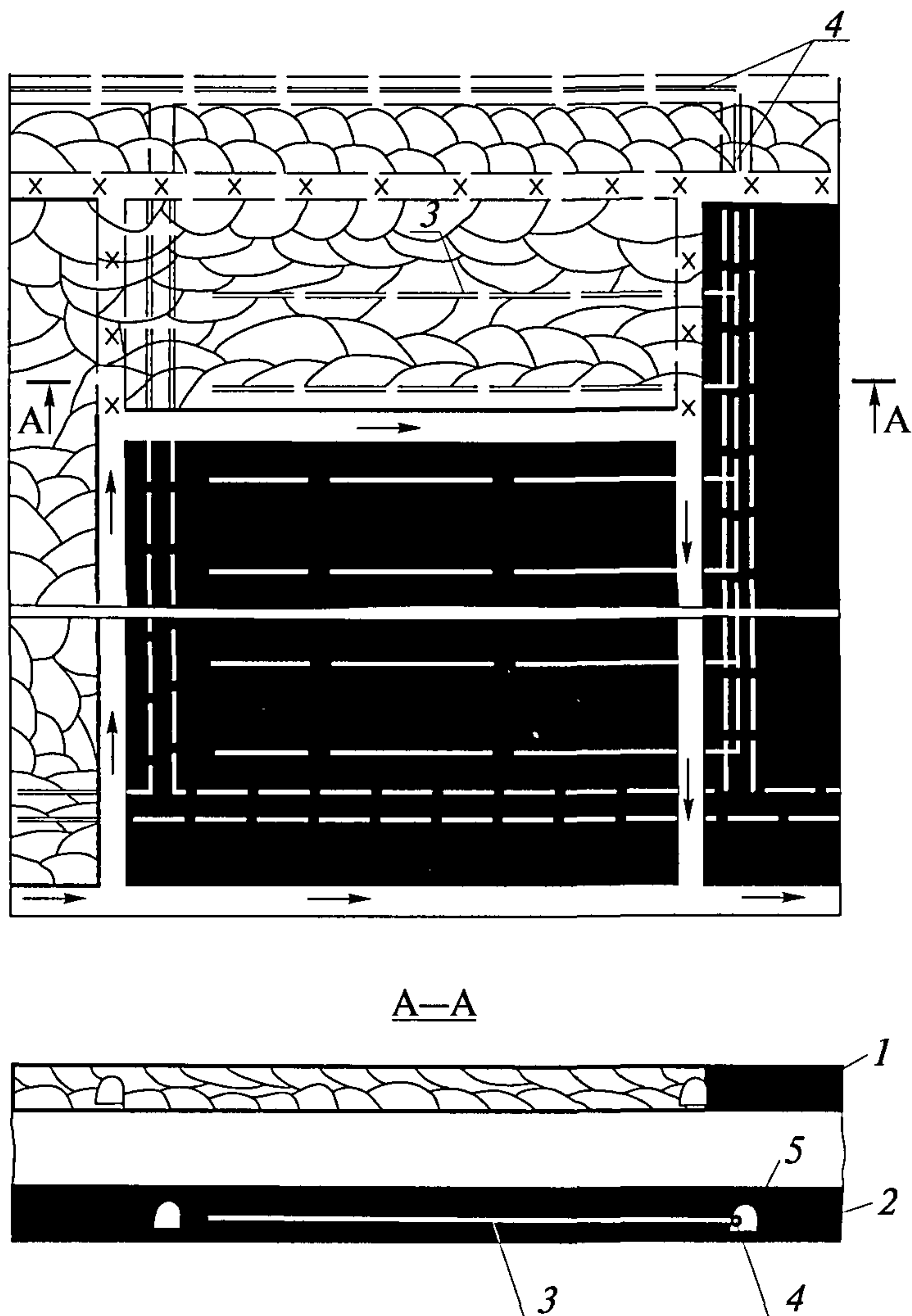
Рис. 3. Схема дегазации надрабатываемого угольного пласта пластовыми скважинами:
