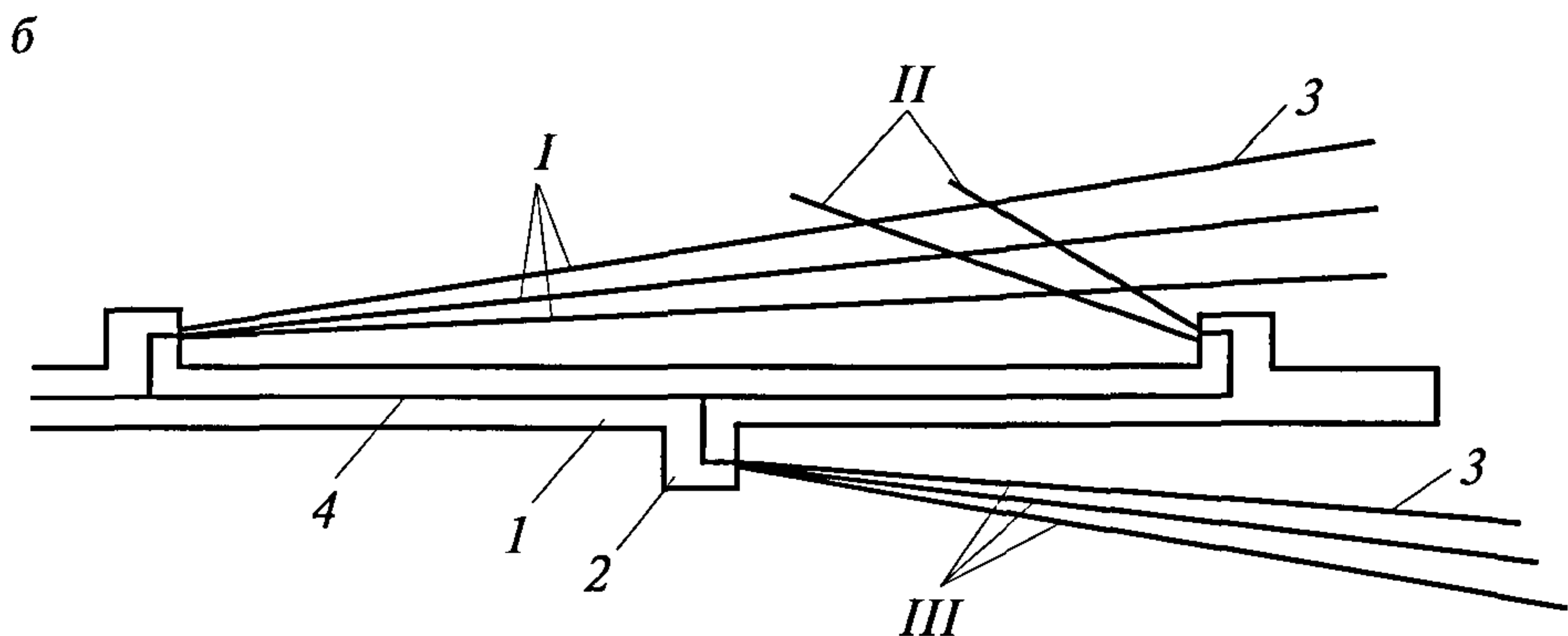
Рис. 5. Схема дегазации пласта барьерными скважинами: a — одиночные скважины; б — перекрещивающиеся скважины; I и II — серии перекрещивающихся барьерных скважин; III — серия барьерных скважин; 1 — штрек; 2 — камера; 3 — скважина; 4 — газопровод; \alpha — угол падения пласта
