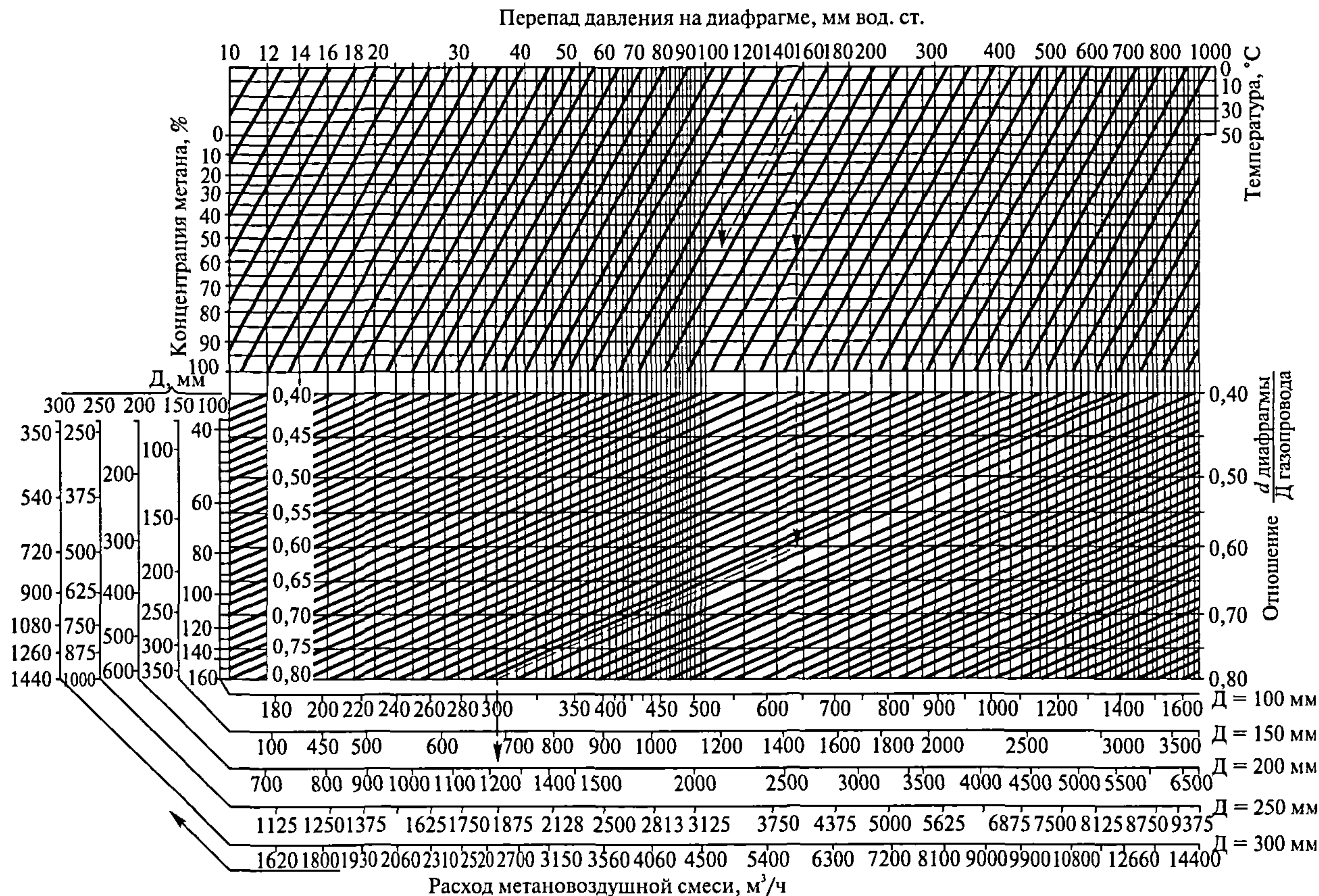
Рис. 6. Определение расхода газа Q_r , м³/ч
