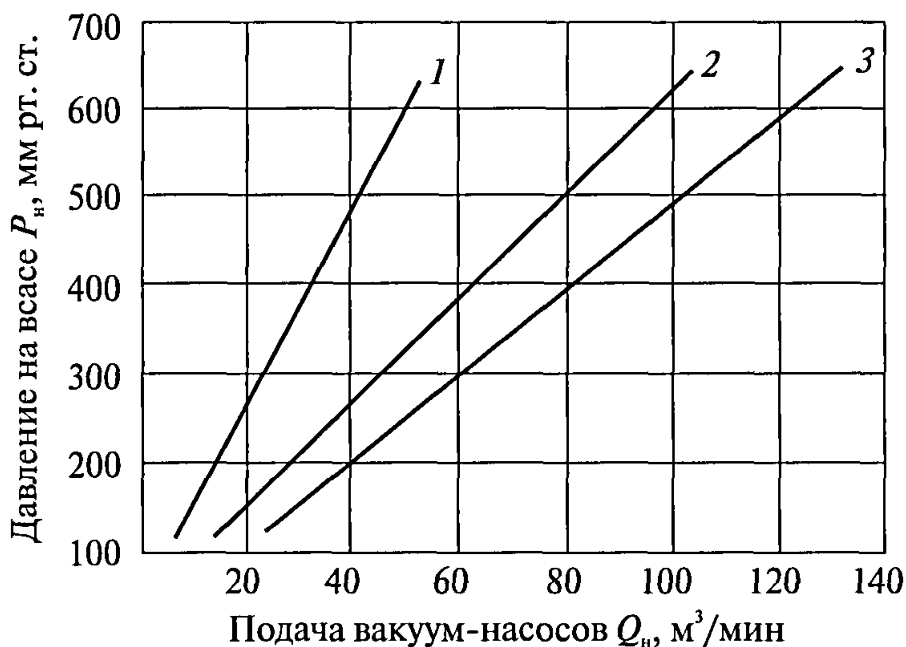
Рис. 3. Характеристика вакуум-насосов:
