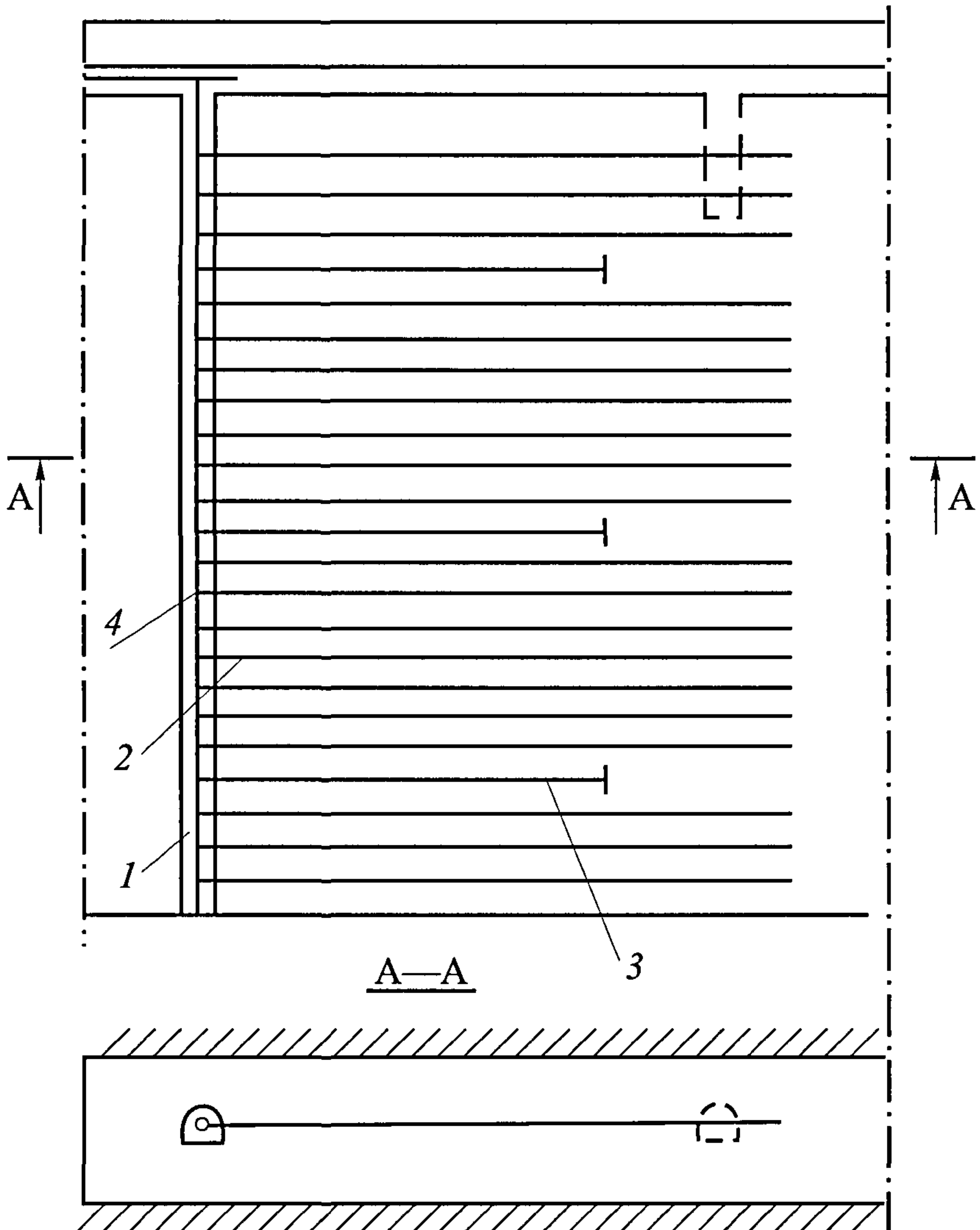
Рис. 17. Схема дегазации с предварительным гидроразрывом пласта через скважины, пробуренные из пластовой выработки: 1 — конвейерный бремсберг; 2 — дегазационная скважина; 3 — скважина гидроразрыва; 4 — дегазационный трубопровод
