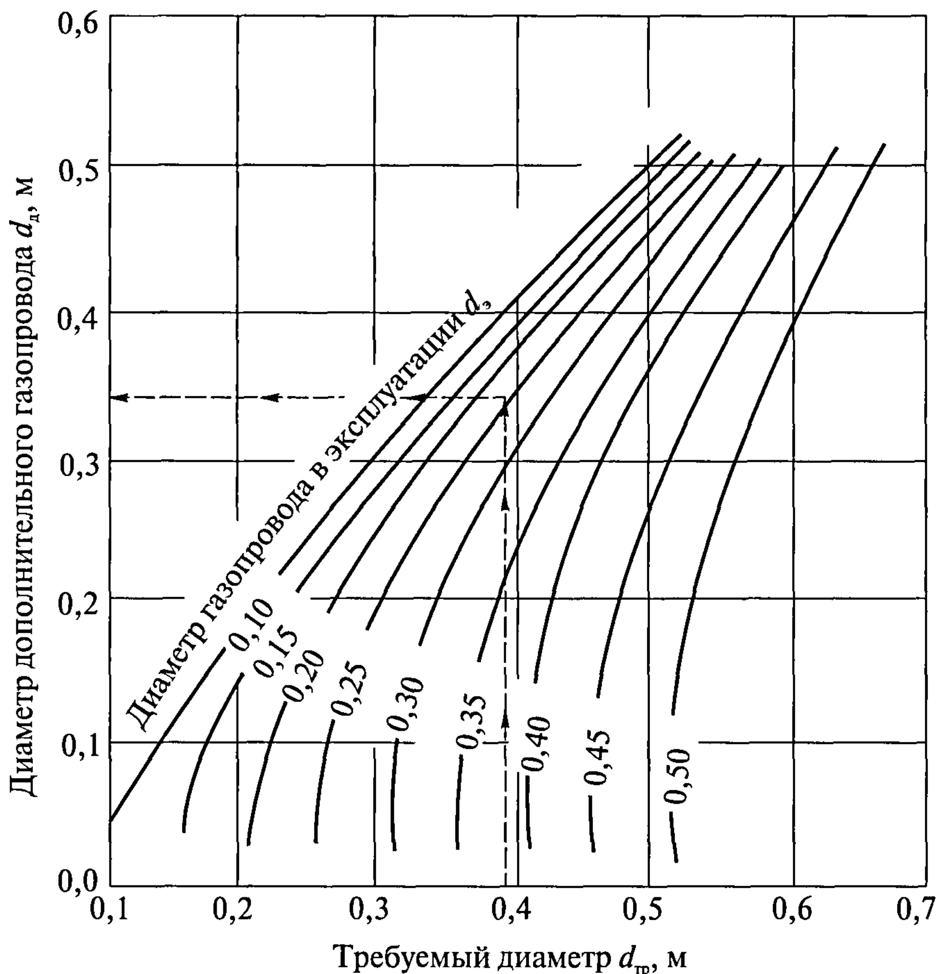
Рис. 5. Определение диаметра дополнительного газопровода
