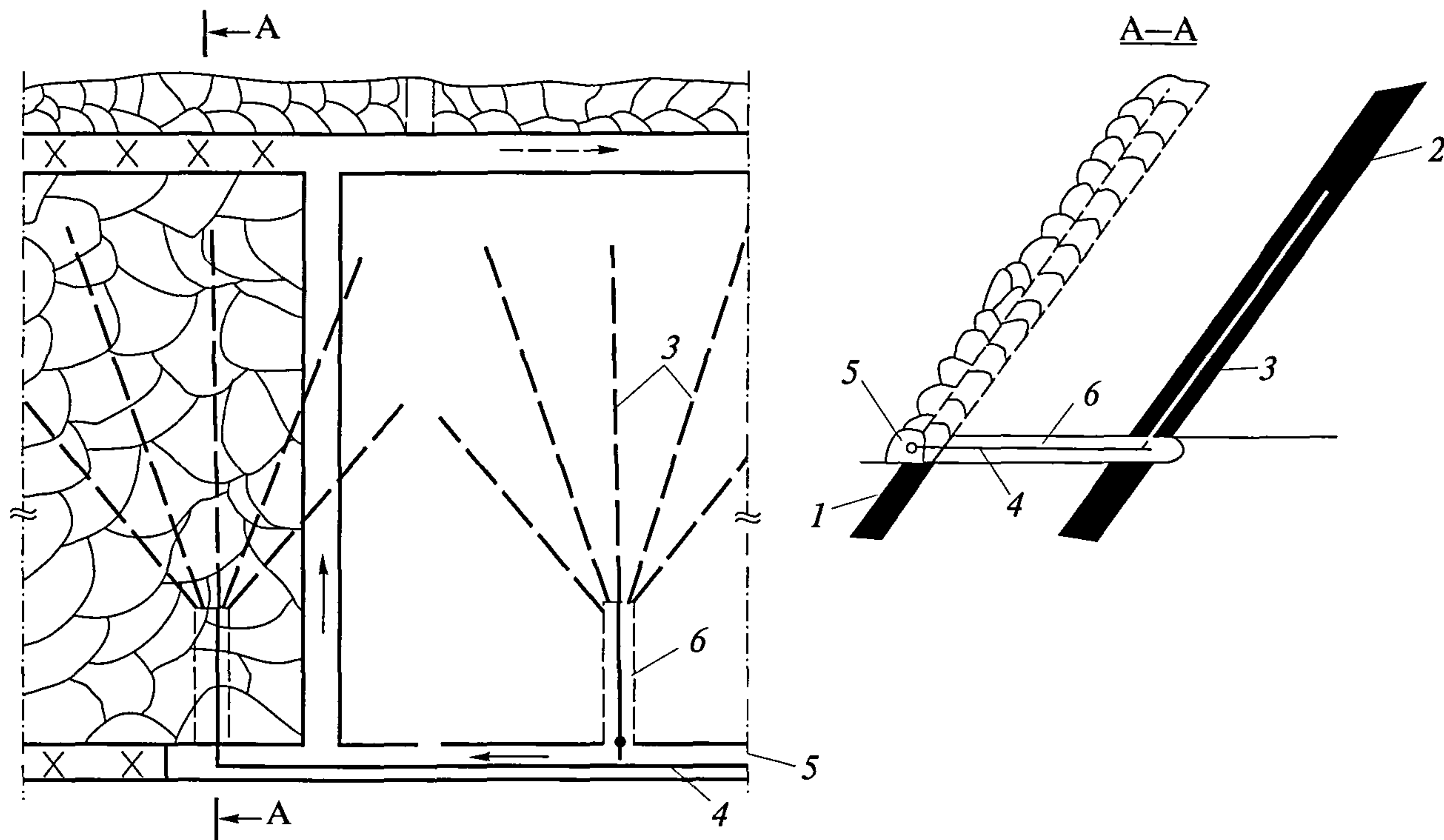
Рис. 3. Схема дегазации надрабатываемого пласта скважинами, пробуренными веером из промежуточного квершлага:
