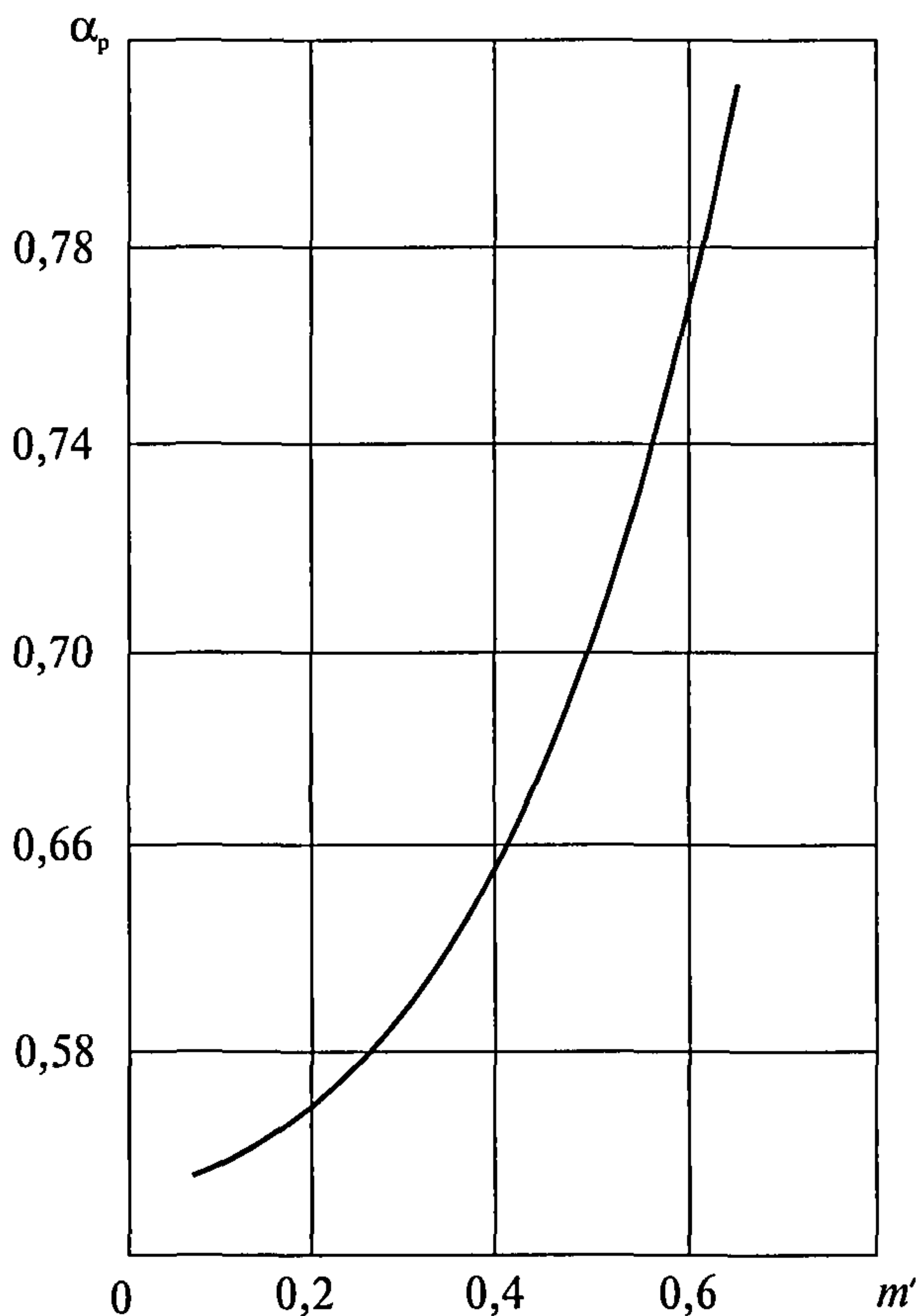
Рис. 5. Зависимость коэффициента расхода \alpha_p от m' = d_0^2/d^2
