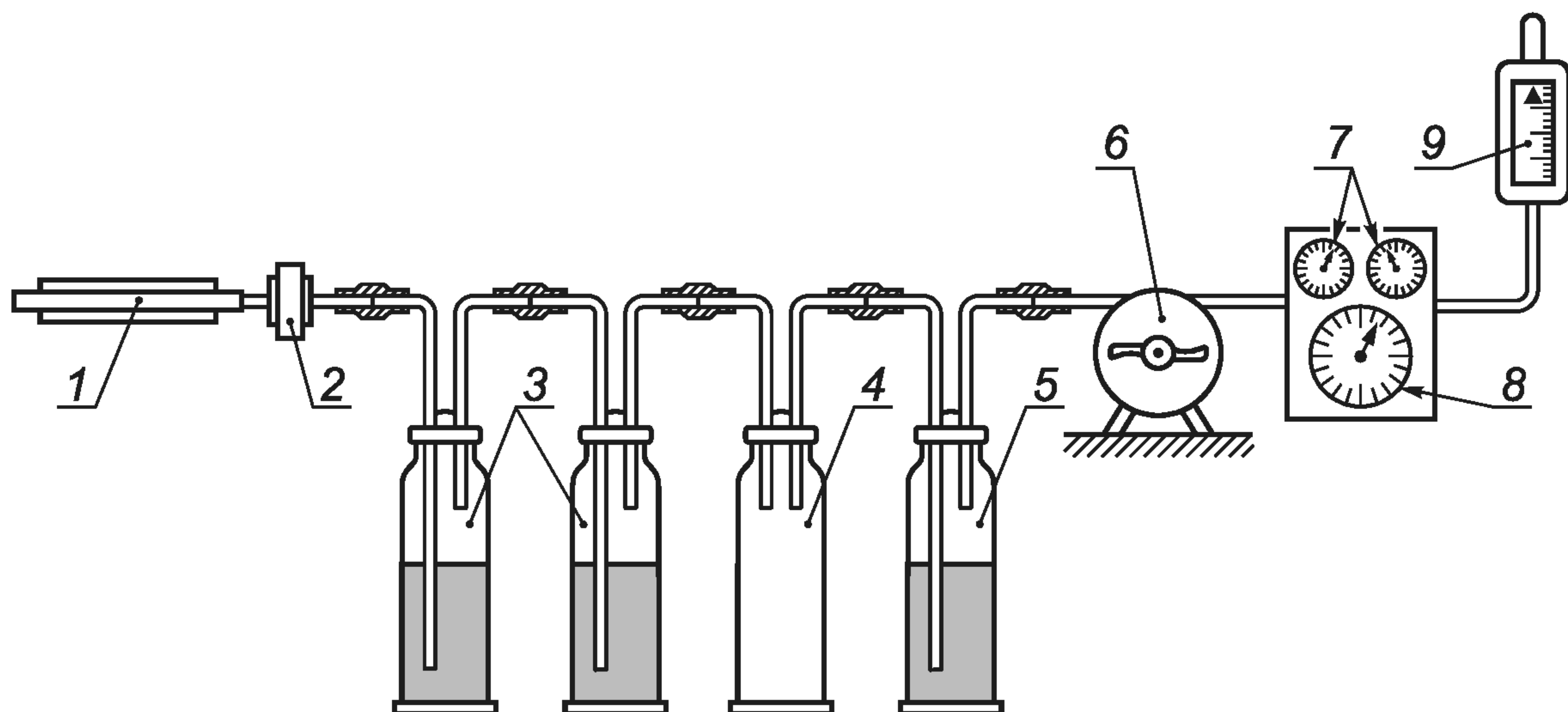
1 — подогреваемый зонд; 2 — фильтр и корпус фильтра; 3 — поглотительные сосуды с раствором NaOH концентрацией 0,1 моль/л; 4 — ловушка; 5 — поглотительный сосуд с силикагелем или осушительная трубка; 6 — насос; 7 — термометр и манометр; 8 — газовый счетчик; 9 — ротаметр
