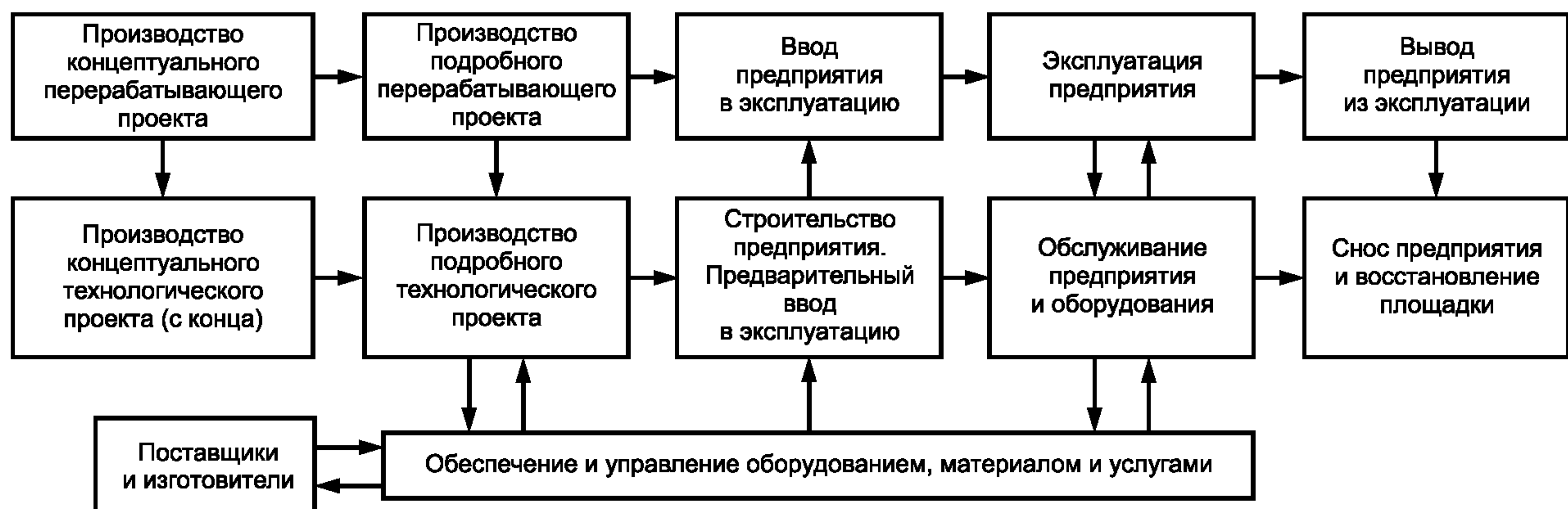
Рисунок 1 — Модель деятельности жизненного цикла перерабатывающего предприятия
