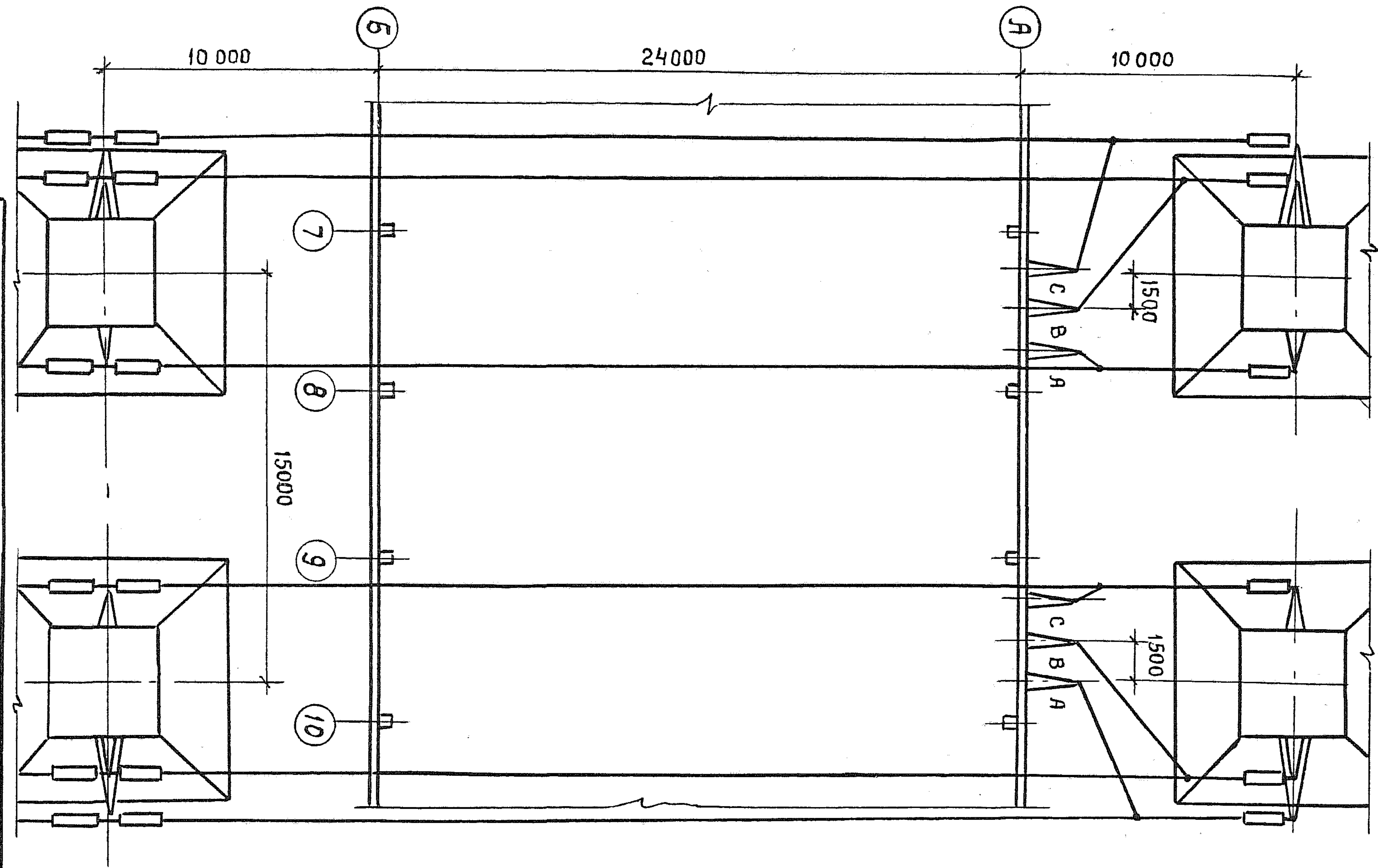
Пример перехода ошиновки над зданием ЗРУ. План (вариант с унифицированными анкерно-угловыми опорами типа УИГО-I+4)
