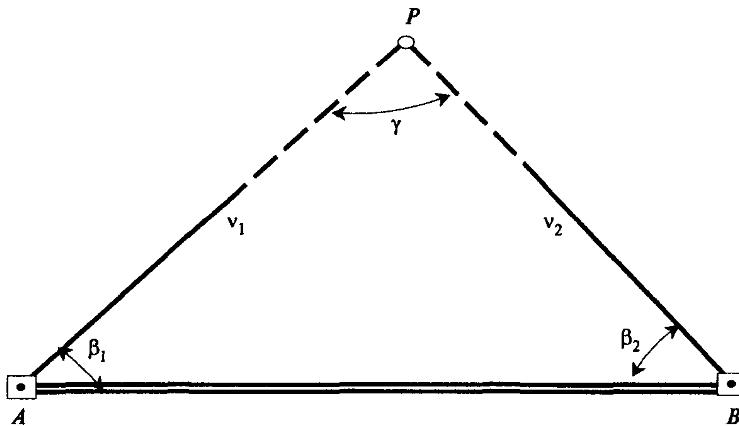
Рис. 2.2. Схема способа прямой угловой засечки
