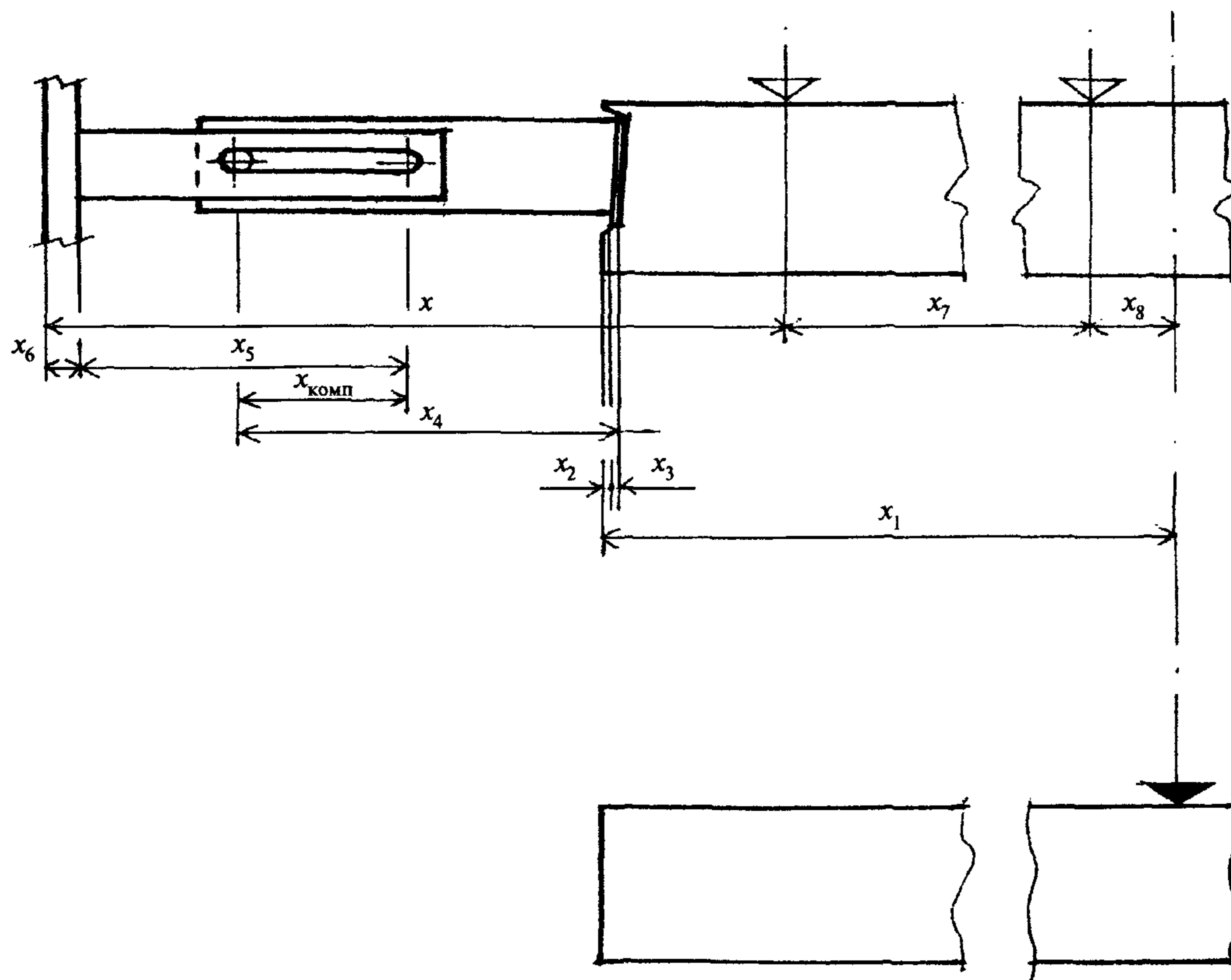
Рисунок 7.1. Расчетная схема
