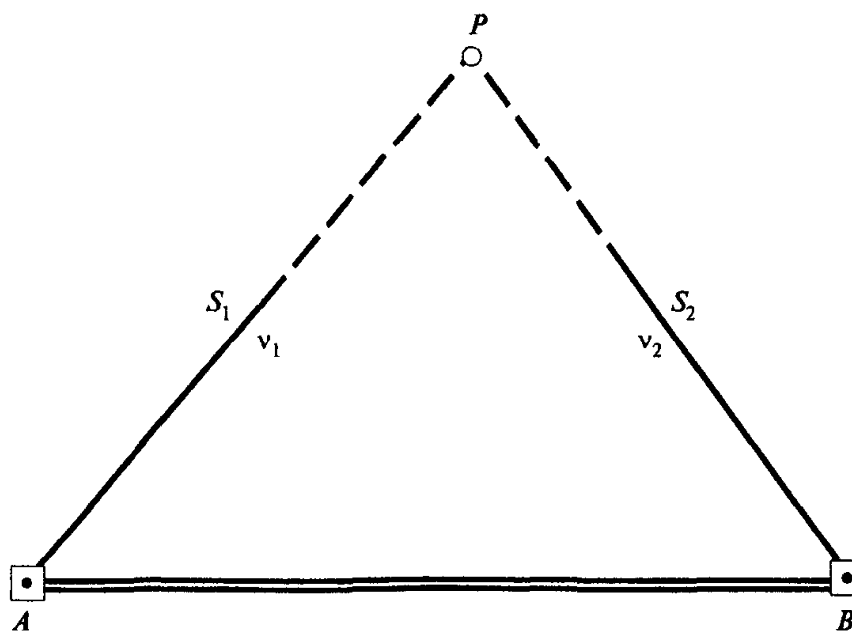
Рис. 2.3. Схема способа линейной засечки
