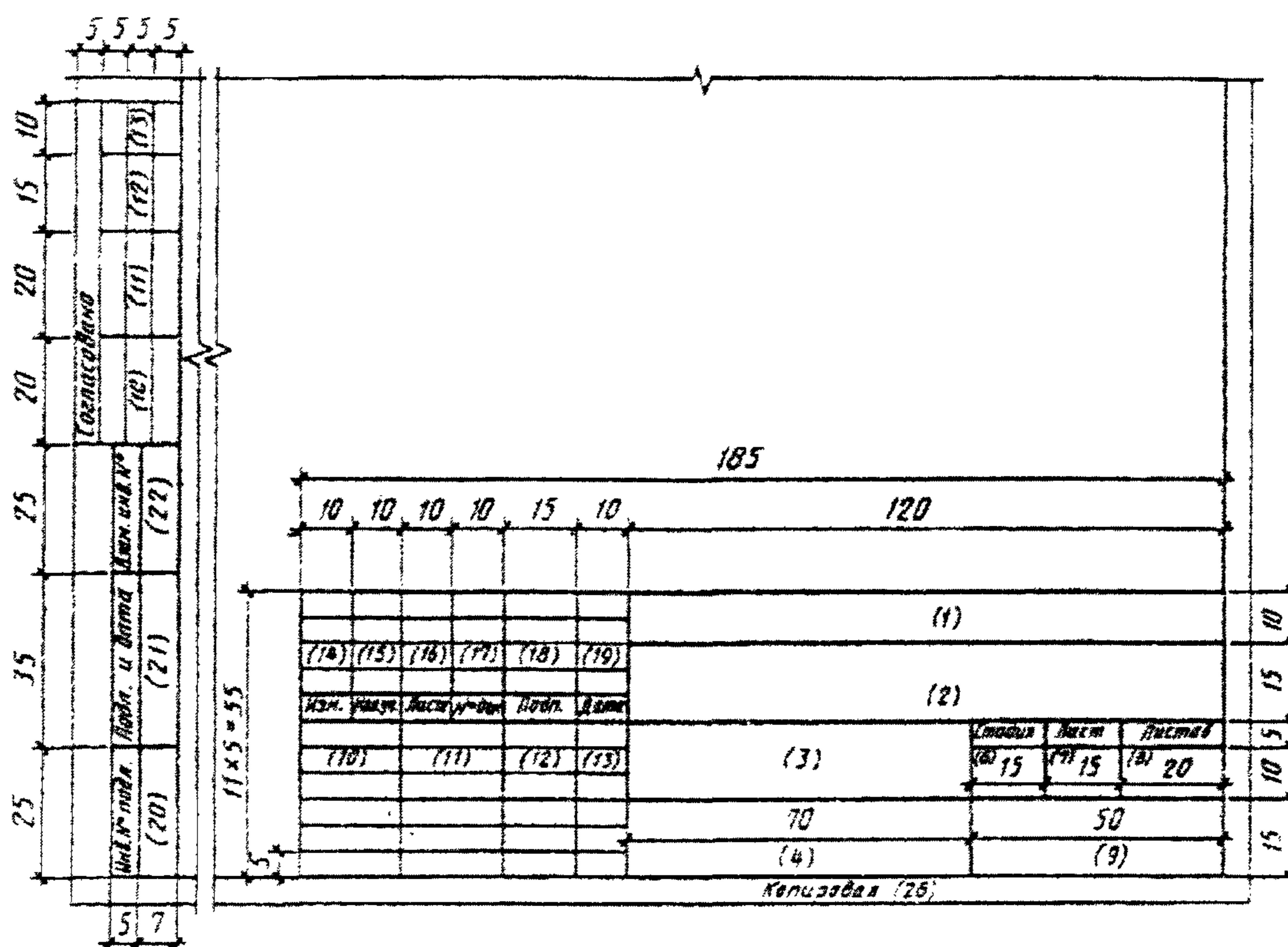
Рисунок 14.1. Основная надпись по ГОСТ 21.101—97
