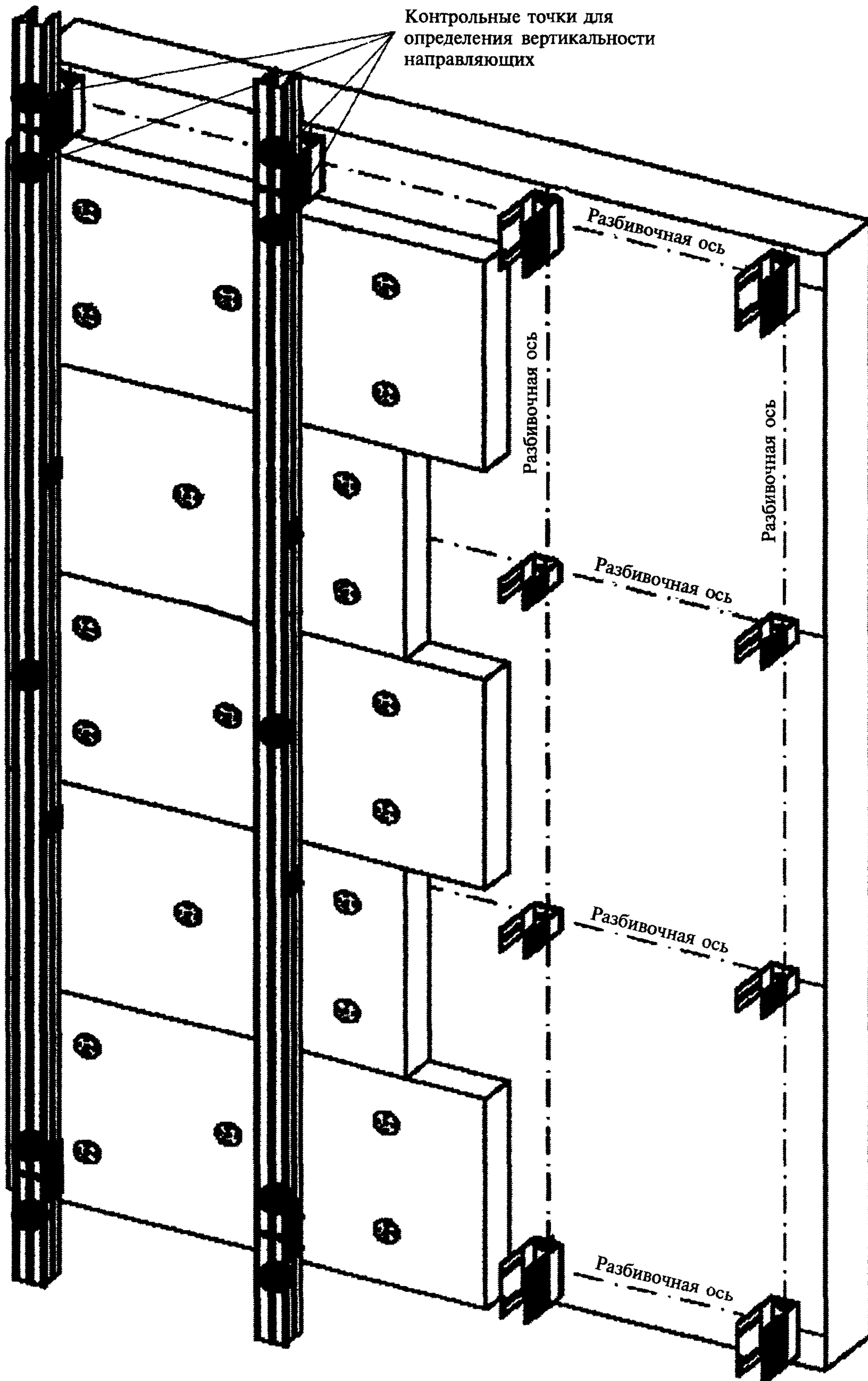
Рисунок 12.1. Схематическое расположение точек для контроля вертикальности направляющих
