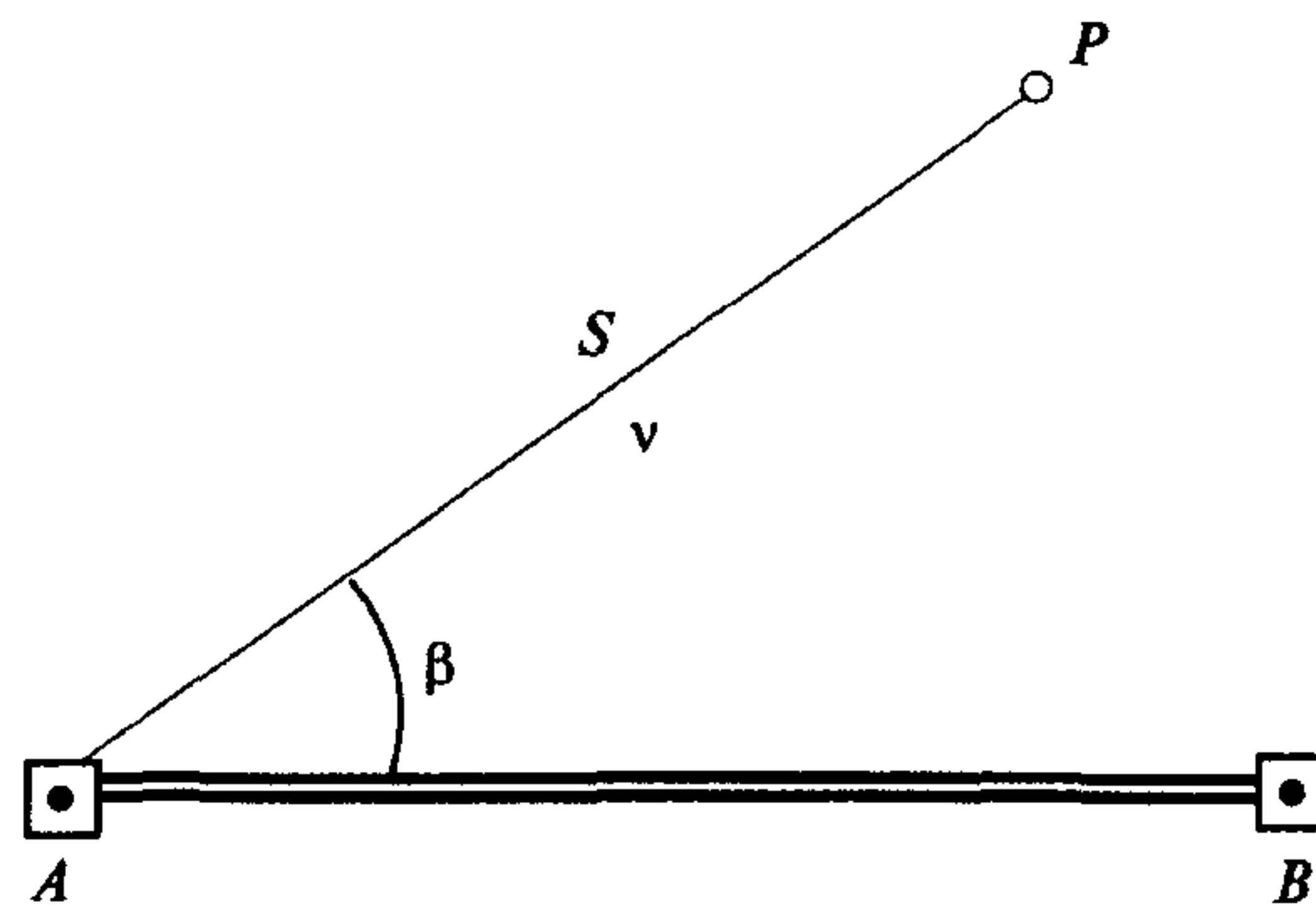
Рис. 2.1. Схема способа полярных координат
