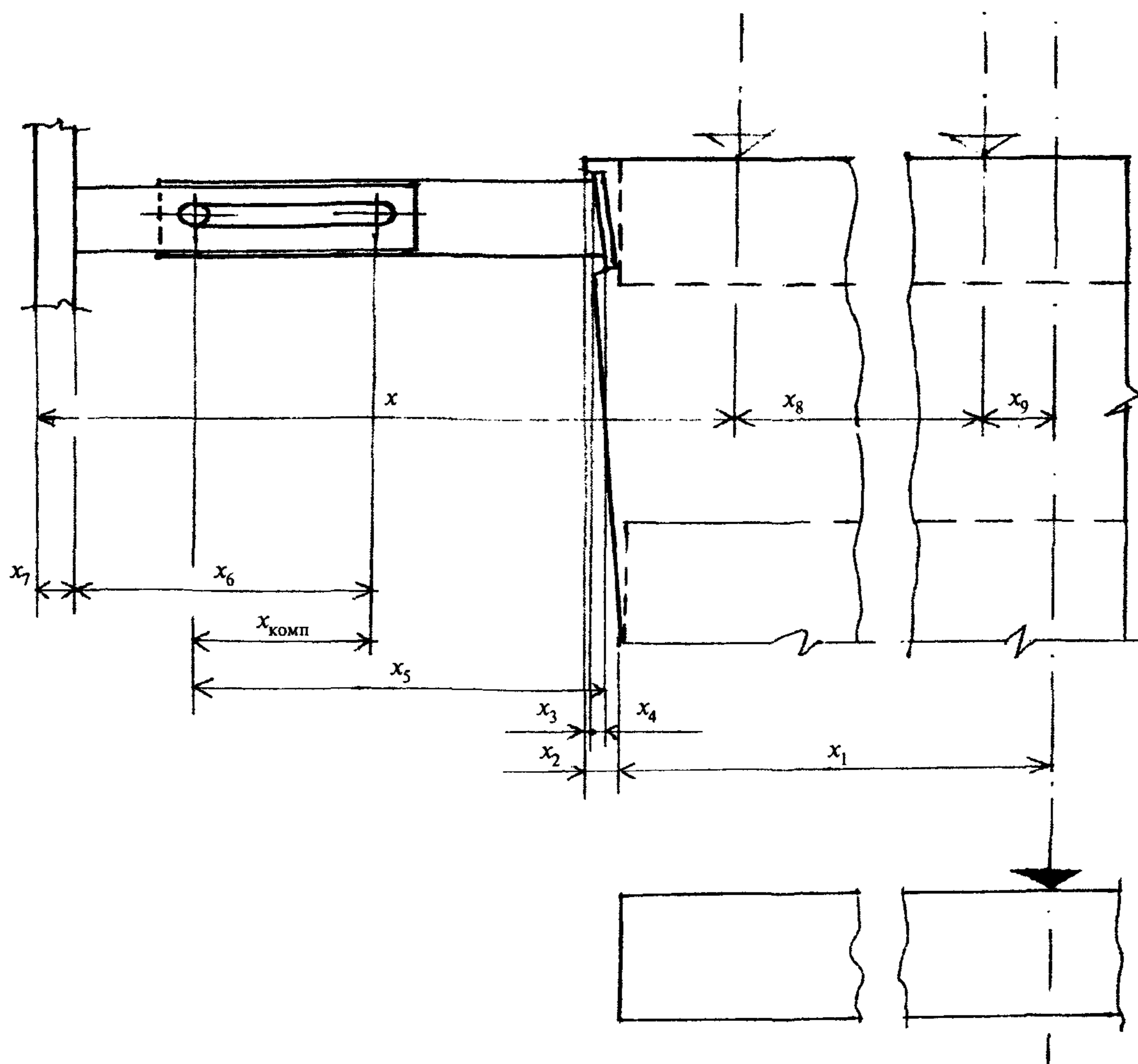
Рисунок 7.2. Расчетная схема
