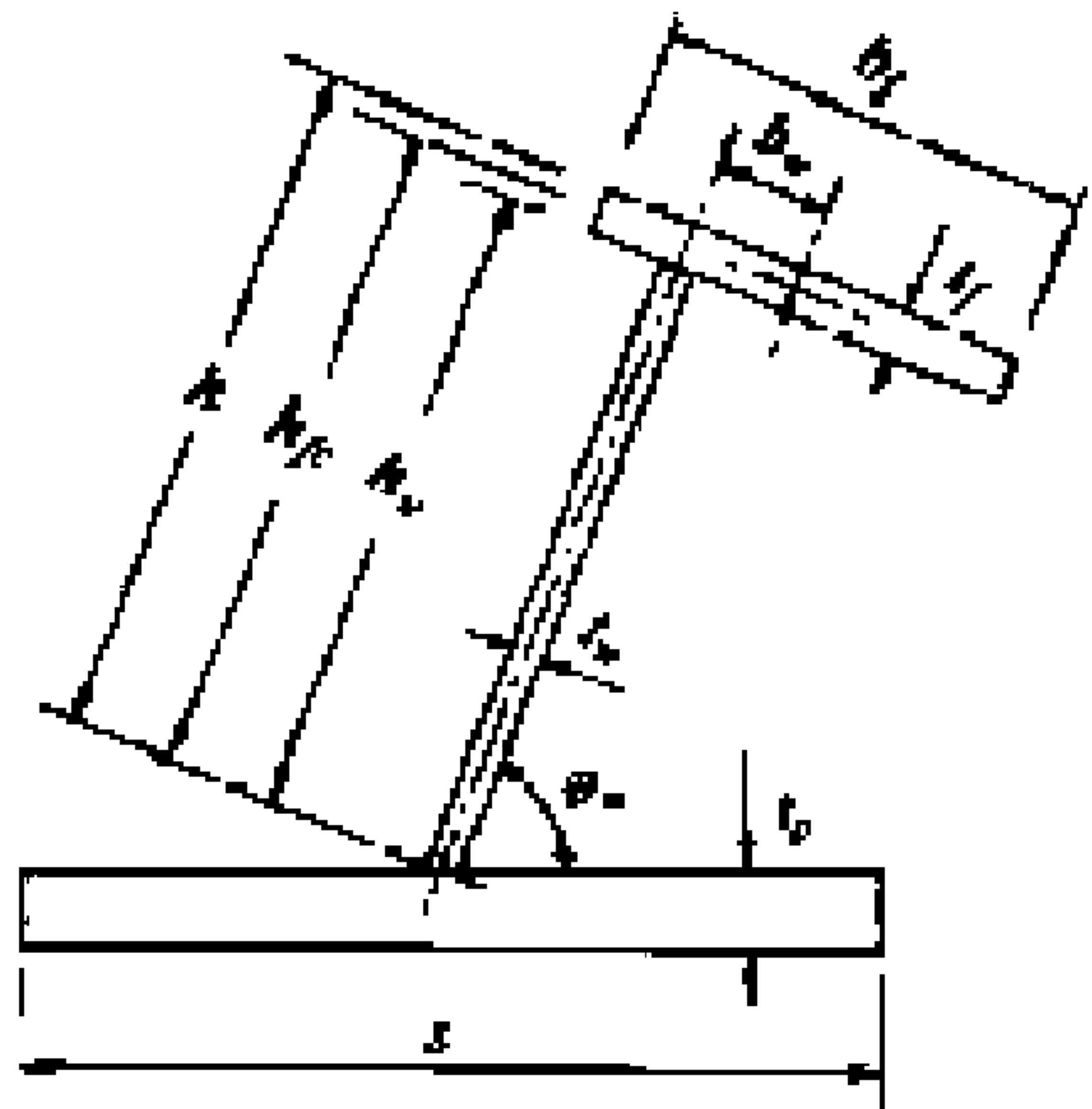
Рис. 1.2.5.7 Геометрия ребра жесткости
