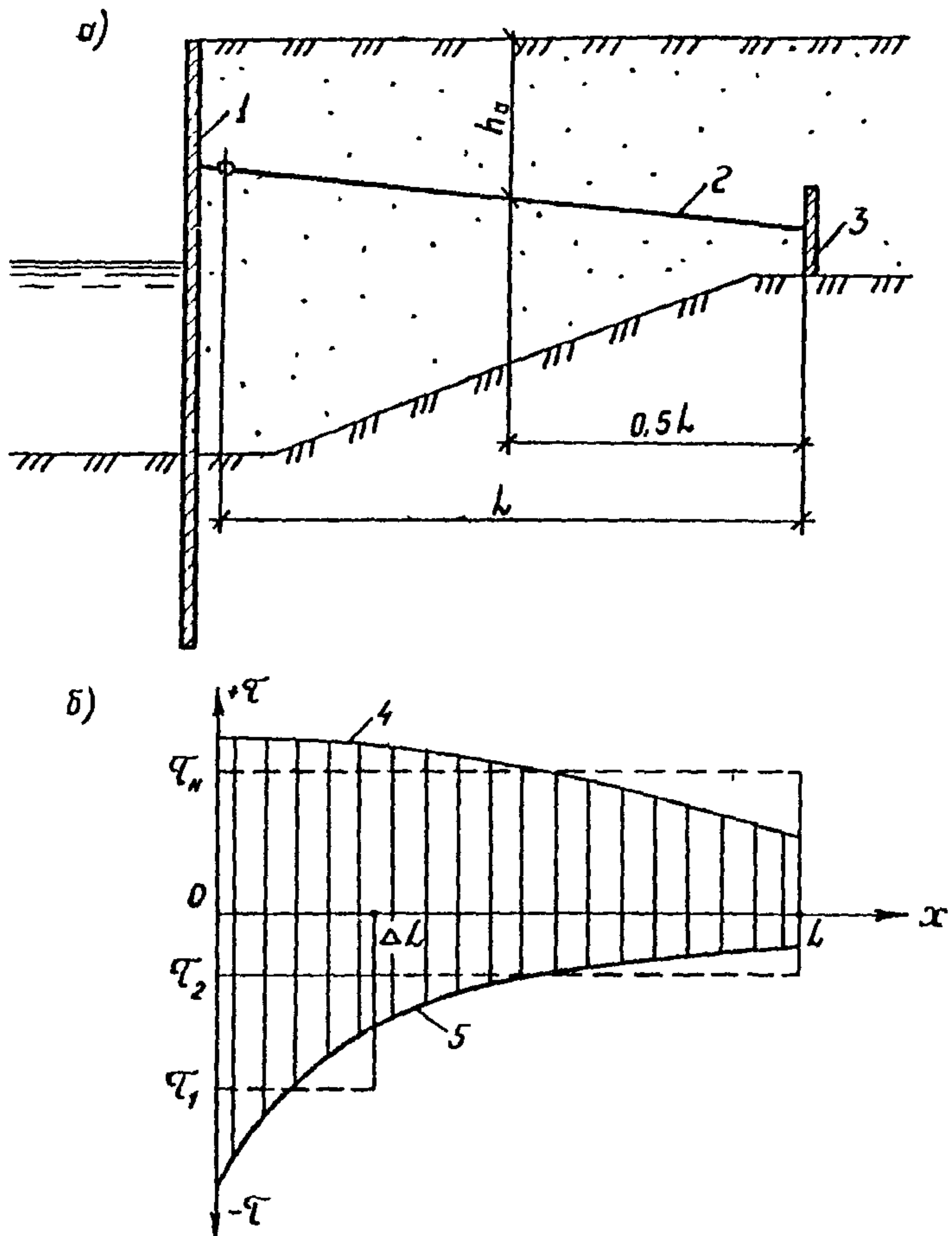
Рис. 3. Схемы к определению \Delta T_q
